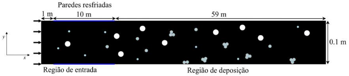
Figura 5.5: Esquema conceitual dos casos simulados com as dimensões geométricas do canal.
