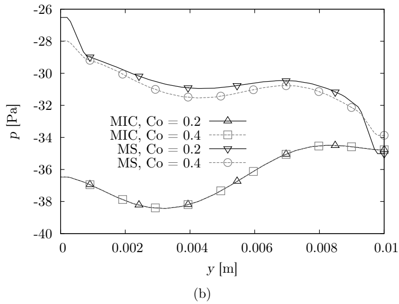
Figura 4.3: Comparação dos perfis de pressão ao longo de uma linha vertical na geometria BFS usando as metodologias MS e MIC. Figura (a) mostra os resultados estacionários do solver pUC para diferentes malhas no caso BFS1, enquanto a Figura (b) mostra os resultados obtidos para diferentes números de Courant para o caso BFS2.
