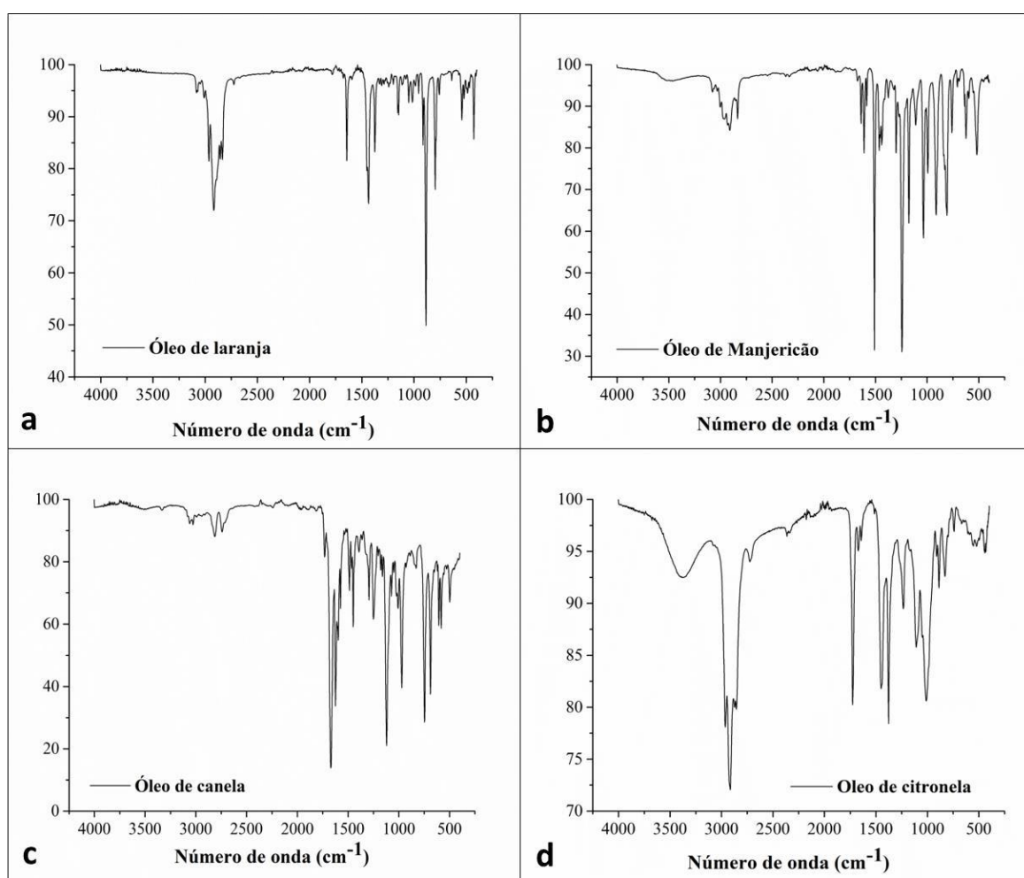
Figura 4. 54. Espectros de FTIR dos óleos essenciais: óleo de laranja, manjerição, canela e citronela
