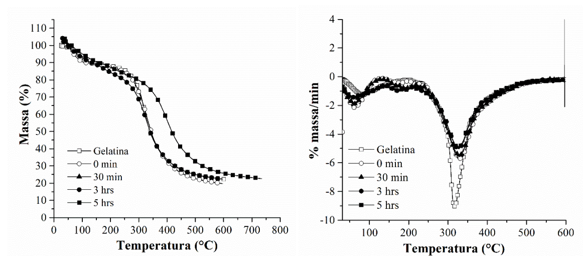
Figura 4. 21. Termogramas de TGA de partículas de gelatina obtidas na reação padrão: a) decomposição térmica; b) derivada da curva de TGA (DTG).
