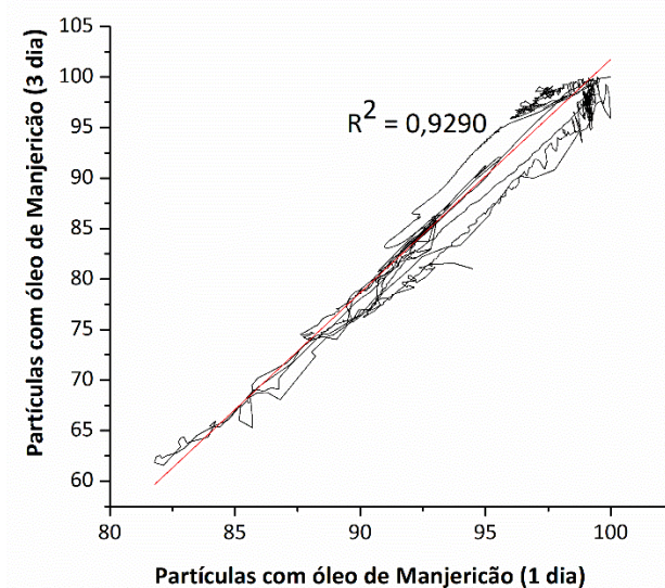
Figura 4. 84. Ensaio de liberação de partículas de gelatina dopadas com óleo de manjerição em 5 horas de reação.
