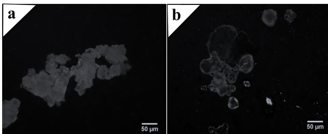
Figura 4. 10. Micrografias de partículas de gelatina obtidas na reação em meio alcalino (NaOH): a) 30 mim e b) 3 horas.
