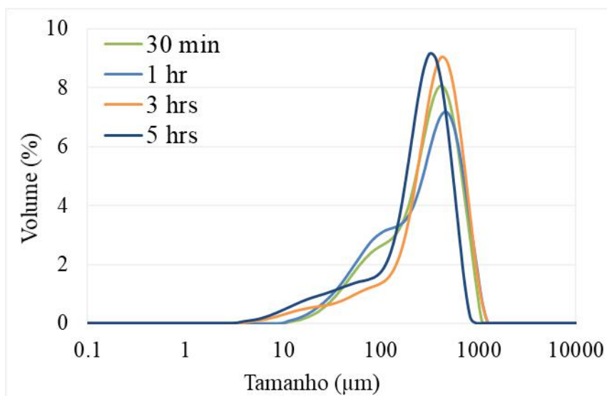
Figura 4. 88. Distribuições de tamanhos de partícula de amido obtidas da reação A2.
