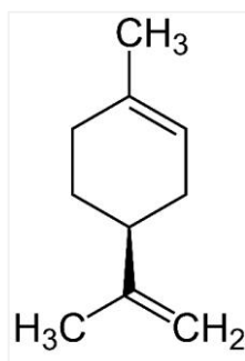
Figura 4. 39. Estrutura molecular do limoneno.
