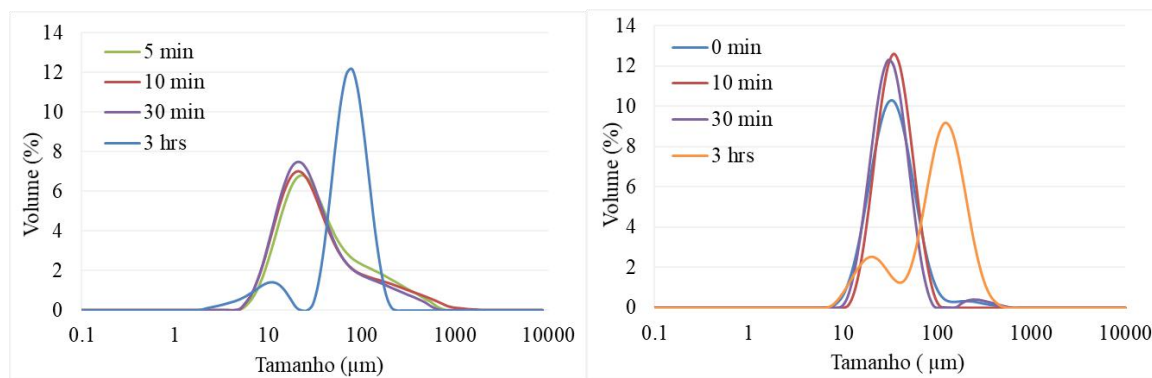
Figura 4. 35. Distribuições dos tamanhos das partículas de gelatina de reações conduzidas com extrato natural de erva cidreira. A) sem controle de pH; b) com controle de pH ( \text{Ca(OH)}_2 ).
