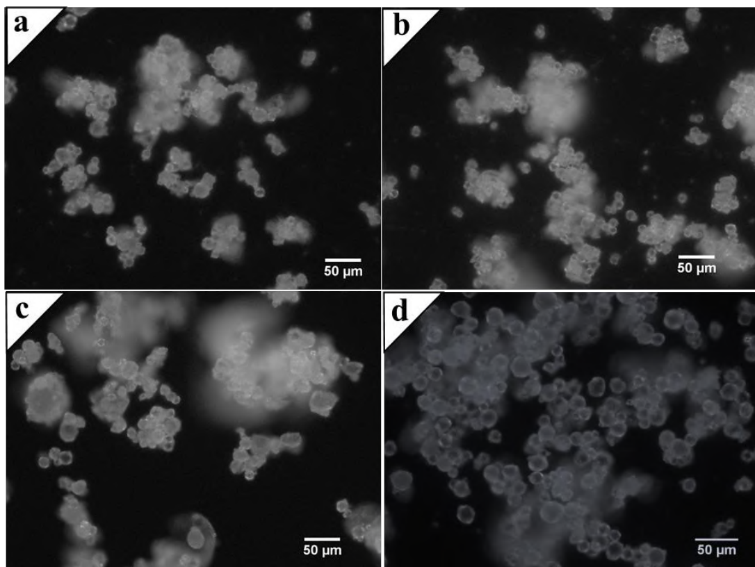
Figura 4. 11. Micrografias de partículas de gelatina obtidas na reação em meio alcalino ( \text{Ca(OH)}_2 ): a) 0 min, b) 30 min, c) 2 horas e d) 3 horas.
