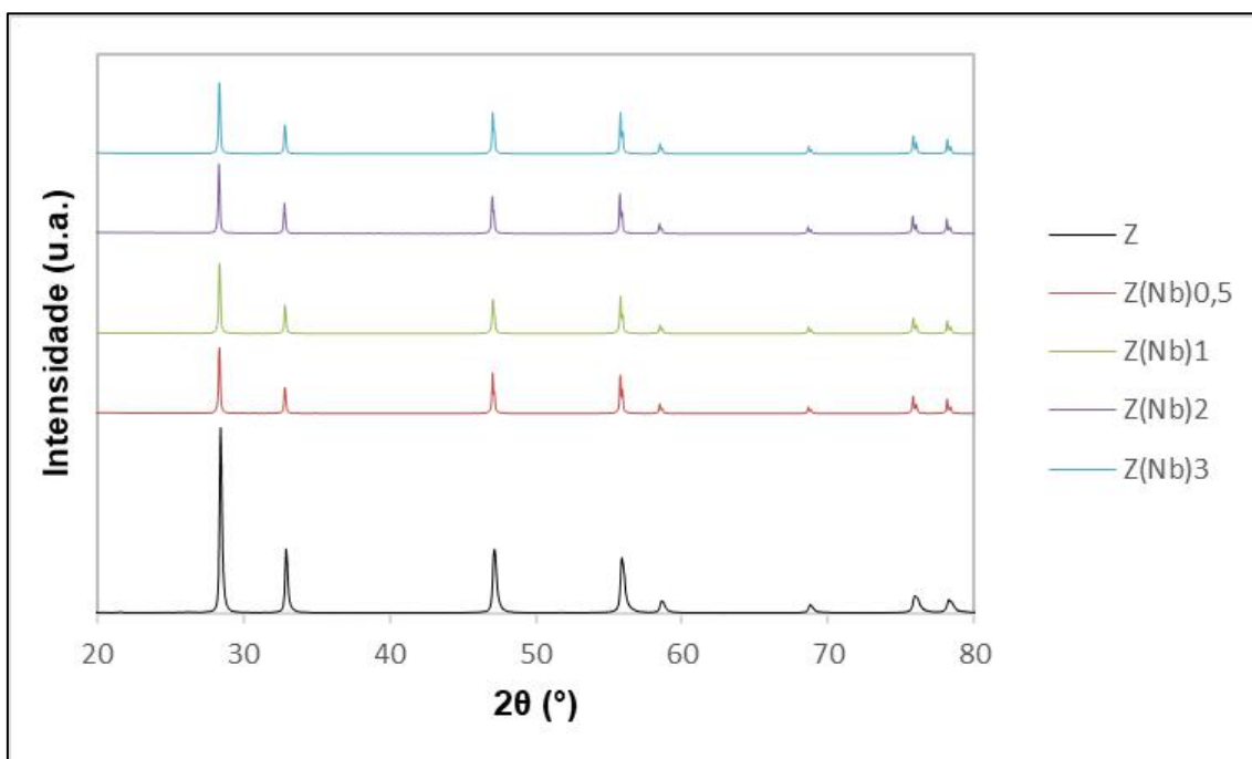
Figura 51: Difratomogramas de raios-X das amostras Z, Z(Nb)0,5; Z(Nb)1, Z(Nb)2 e Z(Nb)3.
