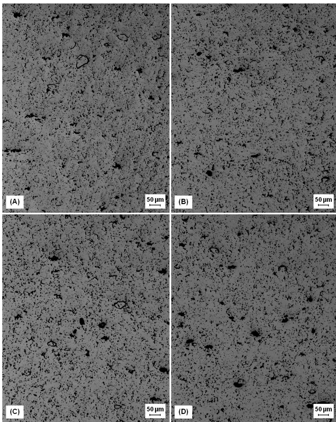
Figura 59: Estrutura de poros das pastilhas de \text{UO}_2 polidas, obtidas por microscopia óptica com aumento de 100x, das amostras (A) Z(\text{Al})_{0,5} ; (B) Z(\text{Al})_1 , (C) Z(\text{Al})_2 e (D) Z(\text{Al})_3 .
