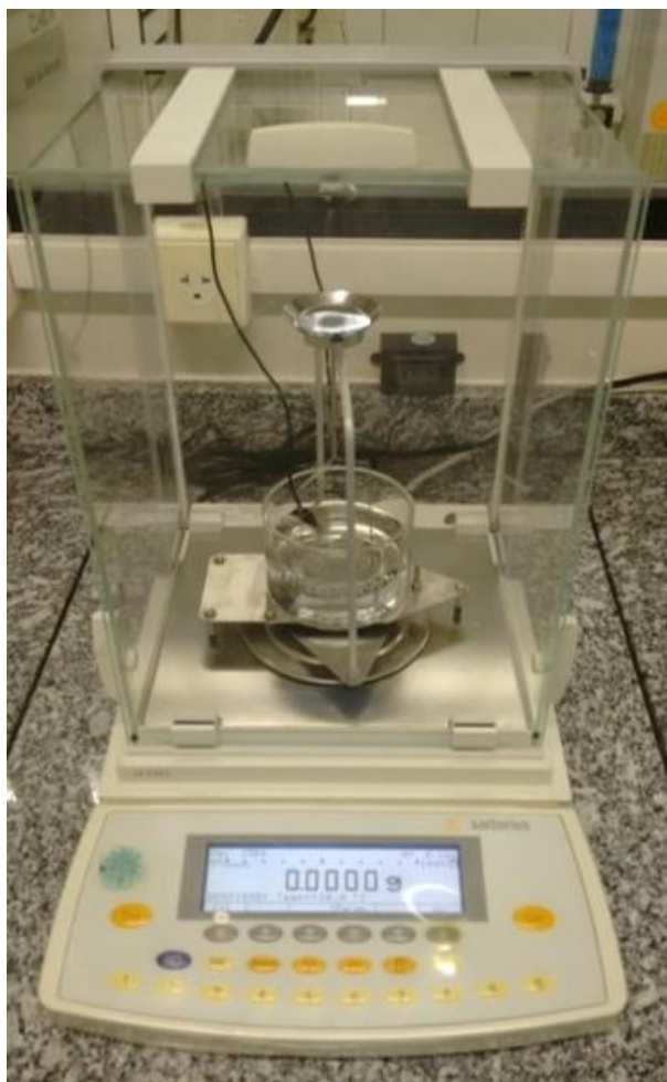
Figura 42: Balança analítica SARTORIUS com monitoração da temperatura do meio e programa computacional SARTO CONNECT para medição de densidade sinterizada pelo método de imersão.
