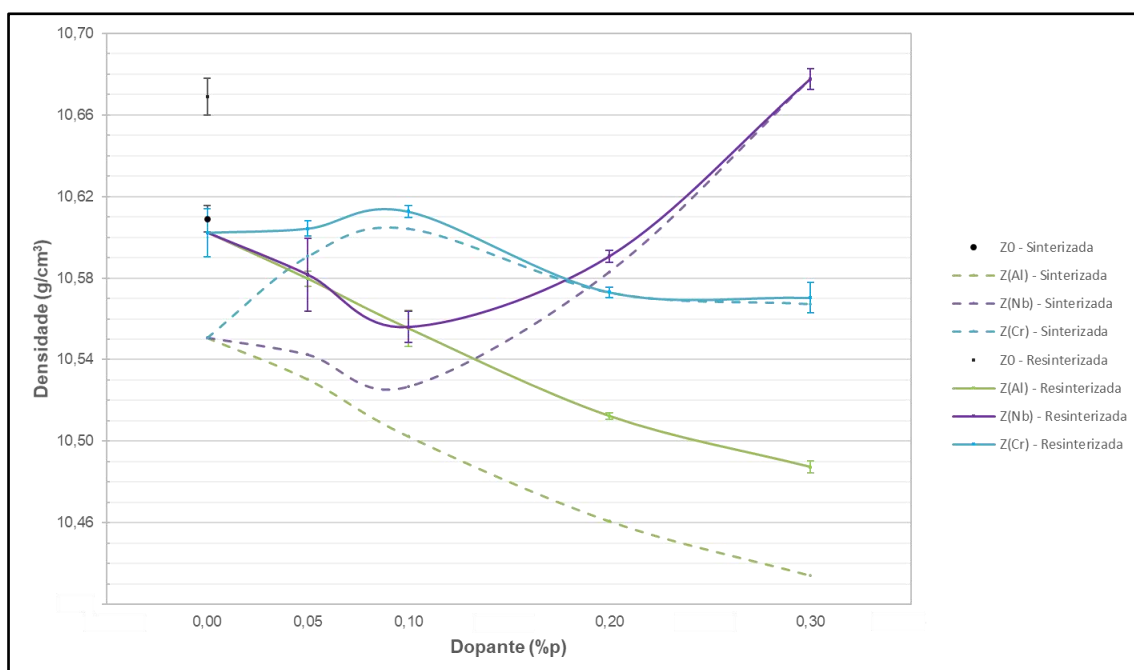
Figura 75: Variações das densidades sinterizadas (1760°C, 5 h, H 2 umidificado) e resinterizadas (1708°C, 24 h, H 2 puro) das amostras Z0, Z, Z(Al), Z(Nb) e Z(Cr) em função da adição dos dopantes (%p = µg Metal/g U).
