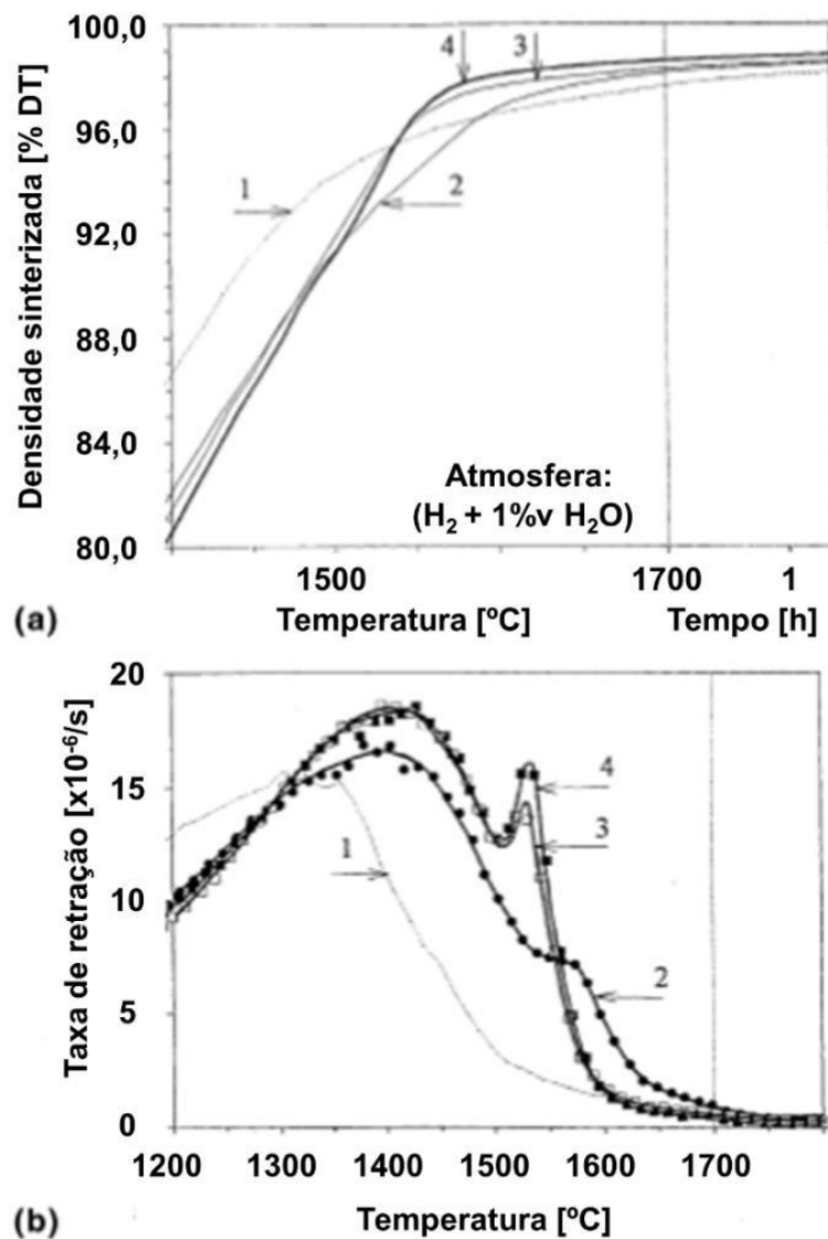
Figura 19: (a) Curvas de retração de pastilhas compactadas em atmosfera de \text{H}_2 + 1\% \text{v H}_2\text{O} : (1) amostra padrão, (2) \text{UO}_2 + 0,05\% \text{p Cr}_2\text{O}_3 , (3) \text{UO}_2 + 0,075\% \text{p Cr}_2\text{O}_3 e (4) \text{UO}_2 + 0,10\% \text{p Cr}_2\text{O}_3 . (b) Taxas de retrações em função da temperatura. Adaptado de [10].
