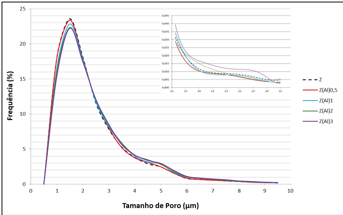
Figura 55: Distribuição dos tamanhos de poros ( \mu\text{m} ) das amostras Z, Z(Al)0,5; Z(Al)1, Z(Al)2 e Z(Al)3 para as regiões de 0 a 10 \mu\text{m} e de 15 a 31 \mu\text{m} .
