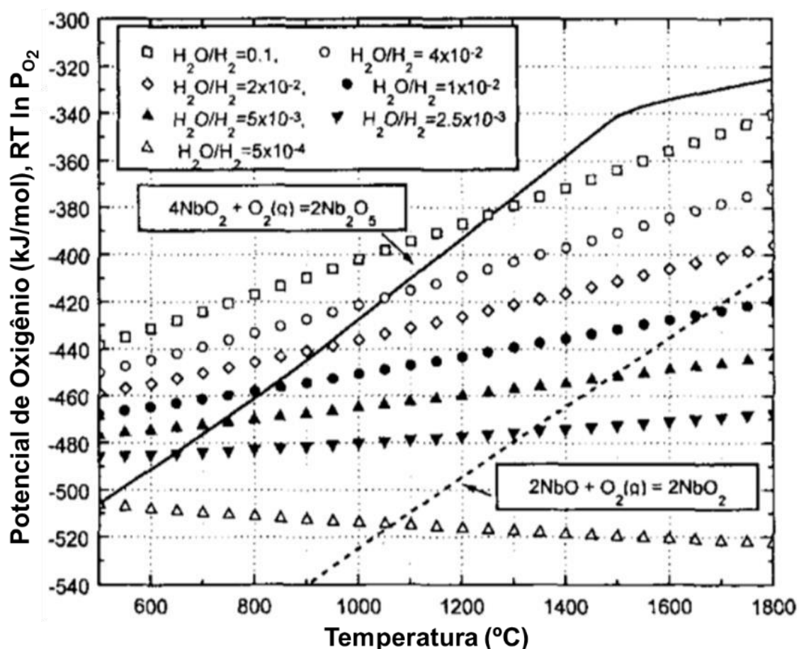
Figura 12: Potenciais de oxigênio dos óxidos de nióbio e várias misturas gasosas ( \text{H}_2\text{O}/\text{H}_2 ) em função da temperatura. Adaptado de [28].
