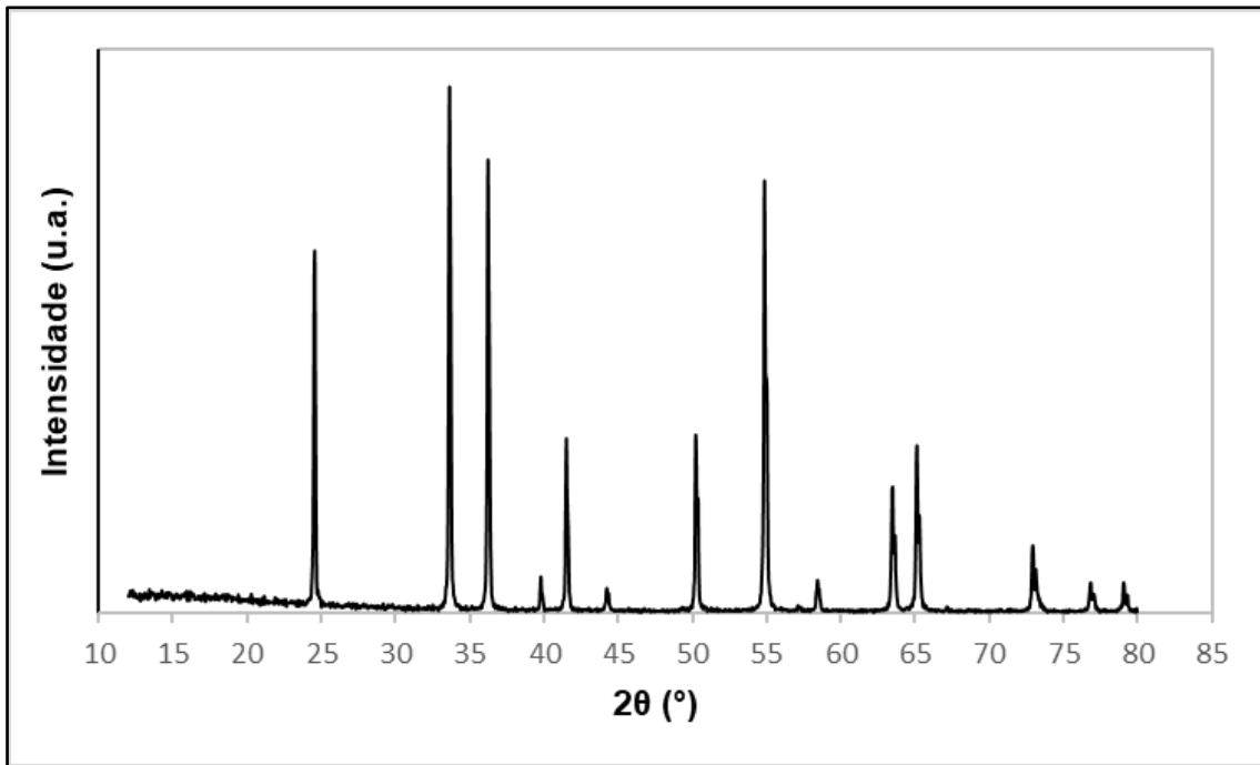
Figura 32: Difratoograma de raios-X da crômia utilizada como dopante.
