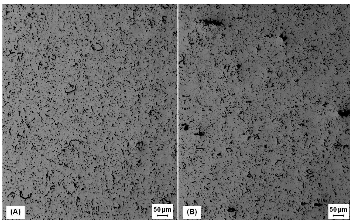
Figura 58: Estruturas de poros das pastilhas de \text{UO}_2 polidas, obtidas por microscopia óptica com aumento de 100x, das amostras (A) Z0 e (B) Z.
