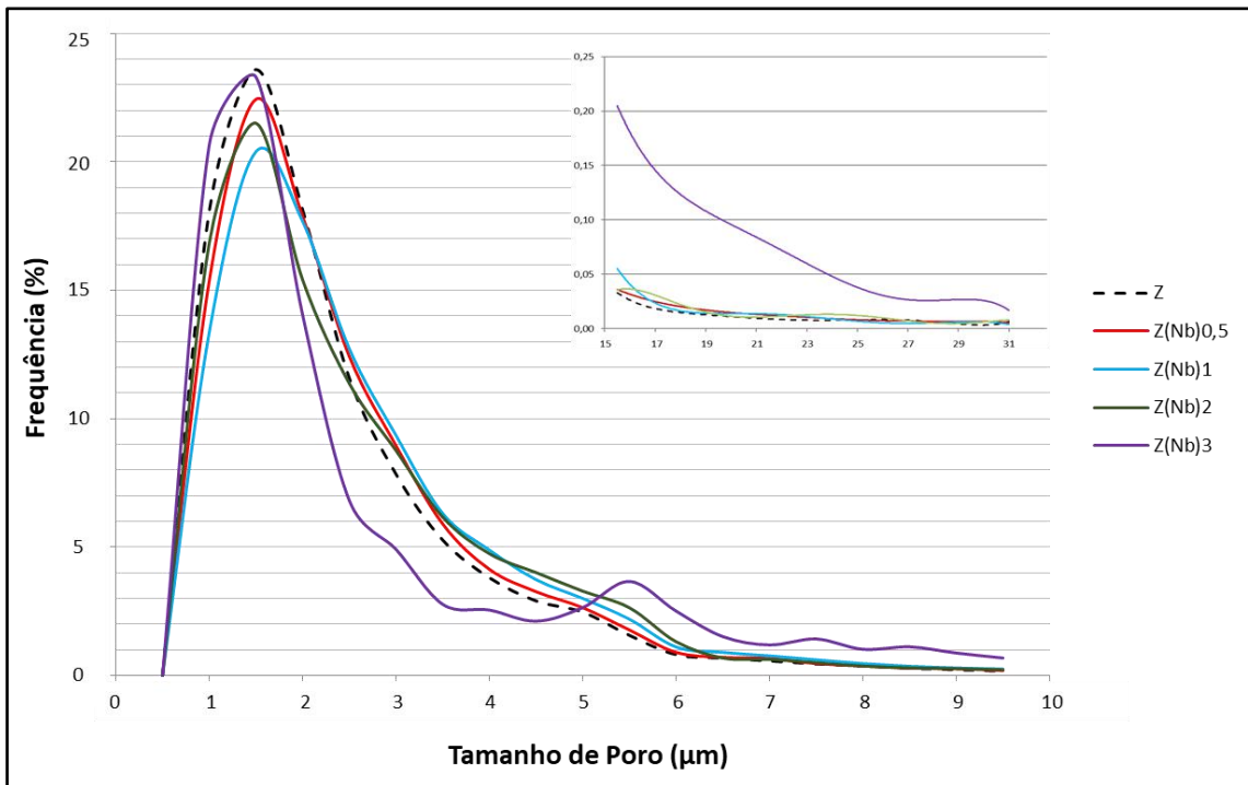
Figura 56: Distribuição dos tamanhos de poros ( \mu\text{m} ) das amostras Z, Z(Nb)0,5; Z(Nb)1, Z(Nb)2 e Z(Nb)3 para as regiões de 0 a 10 \mu\text{m} e de 15 a 31 \mu\text{m} .
