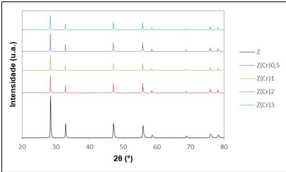
Figura 52: Difratogramas de raios-X das amostras Z, Z(Cr)0,5; Z(Cr)1, Z(Cr)2 e Z(Cr)3.
