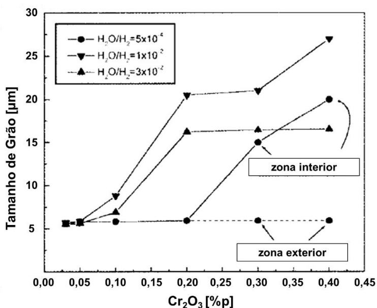
Figura 21: Relação entre tamanho de grão e teor de \text{Cr}_2\text{O}_3 para diferentes razões \text{H}_2\text{O}/\text{H}_2 na atmosfera de sinterização. Adaptado de [11].
