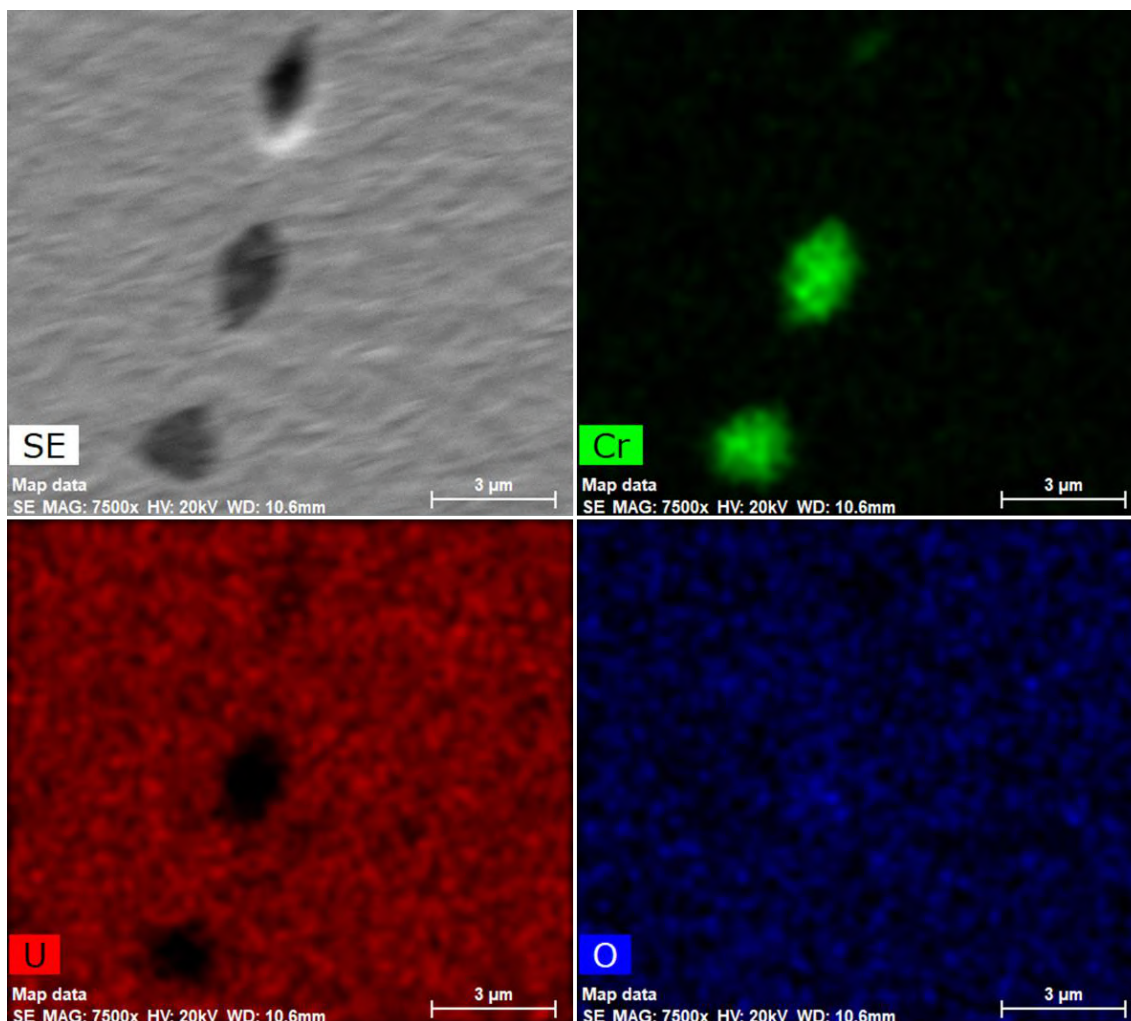
Figura 73: Micrografia da amostra Z(Cr) 3 realizada em MEV com detector de elétrons secundários, com aumento de 7500x, juntamente com as respectivas análises químicas qualitativas feitas por EDS na forma de mapeamento de Cr (verde), U (vermelho) e O (azul).
