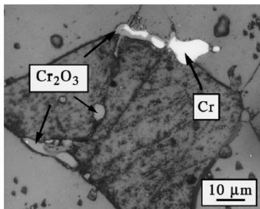
Figura 18: Morfologia da segunda fase da amostra de UO 2 inicialmente contendo 0,25 %p Cr 2 O 3 , sinterizada a 1700°C em atmosfera H 2 + 1 %v H 2 O. Adaptado de [10].
