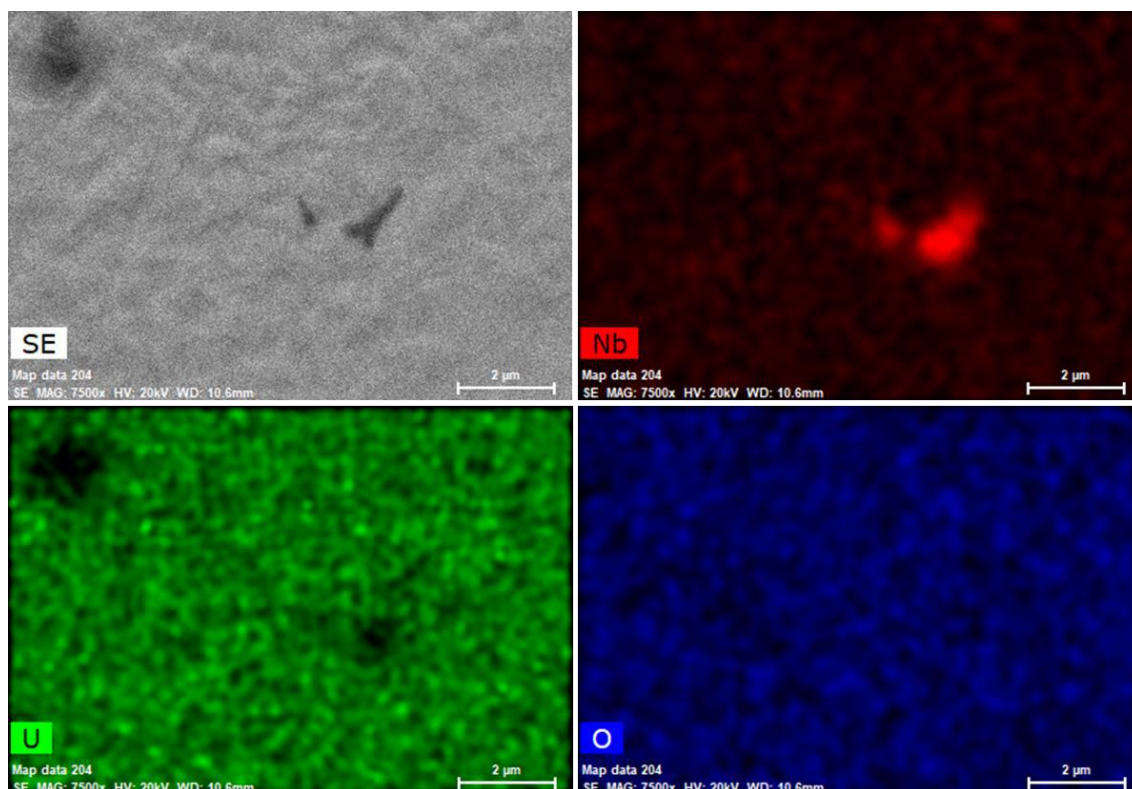
Figura 71: Micrografia da amostra \text{Z}(\text{Nb})_3 realizada em MEV com detector de elétrons secundários, com aumento de 7500x, juntamente com as respectivas análises químicas qualitativas feitas por EDS na forma de mapeamento de Nb (vermelho), U (verde) e O (azul).
