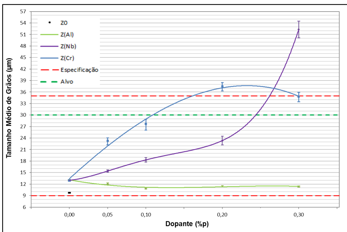
Figura 62: Influência das adições de 0,05; 0,10; 0,20 e 0,30 %p de \text{Al}_2\text{O}_3 , \text{Nb}_2\text{O}_5 e \text{Cr}_2\text{O}_3 (%p = g Metal/g U) nos tamanhos médios de grãos das pastilhas combustíveis de \text{UO}_2 .
