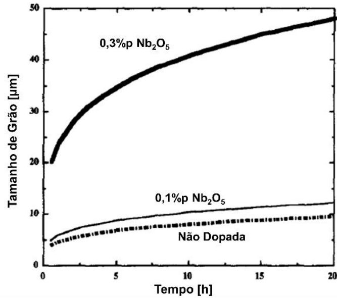
Figura 10: Crescimento de grão com o tempo das pastilhas não dopadas, dopadas com 0,1 e 0,3 %p de Nb 2 O 5 e sinterizadas em atmosfera de H 2 úmido a 1700°C. Adaptado de [26].
