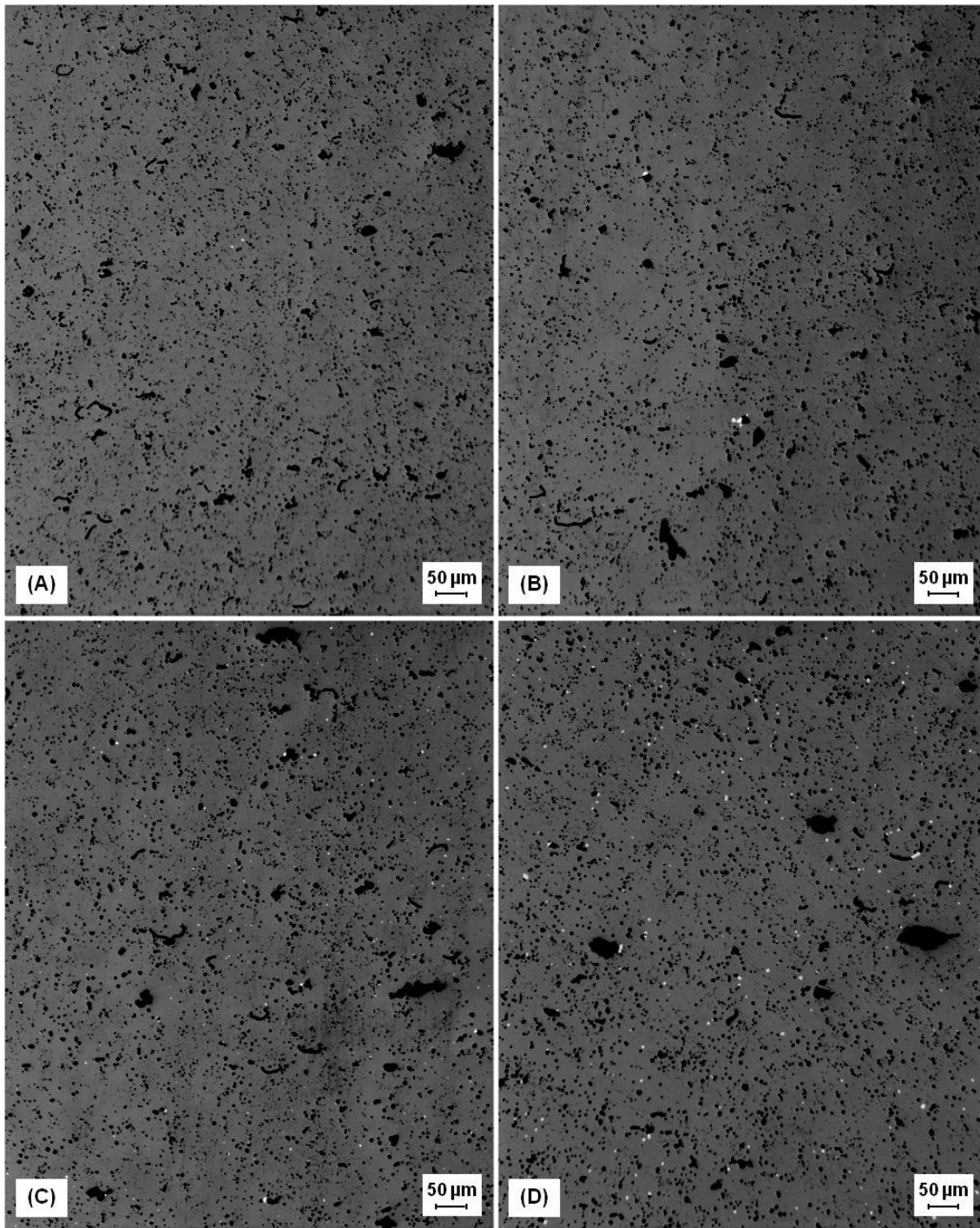
Figura 61: Estrutura de poros das pastilhas de \text{UO}_2 polidas, obtidas por microscopia óptica com aumento de 100x, das amostras (A) Z(Cr)0,5; (B) Z(Cr)1, (C) Z(Cr)2 e (D) Z(Cr)3.
