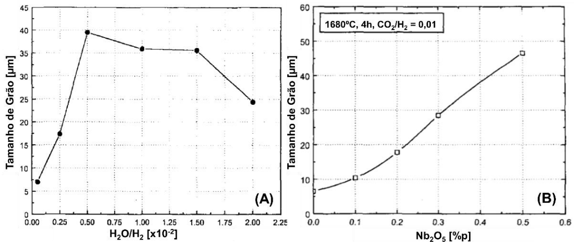
Figura 14: Dependência do tamanho de grão (A) da pastilha dopada com 0,3 %p de Nb 2 O 5 sinterizada a 1700°C em função da razão H 2 O/H 2 da atmosfera de sinterização, e (B) em função da adição de Nb 2 O 5 sinterizadas a 1680°C por 4 h (CO 2 /H 2 = 0,01). Adaptado de [28].
