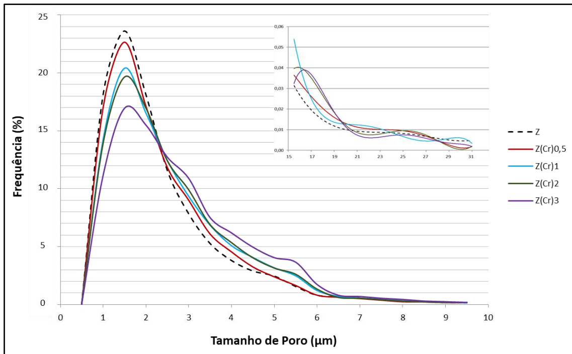
Figura 57: Distribuição dos tamanhos de poros (μm) das amostras Z, Z(Cr)0,5; Z(Cr)1, Z(Cr)2 e Z(Cr)3 para as regiões de 0 a 10 μm e de 15 a 31 μm.
