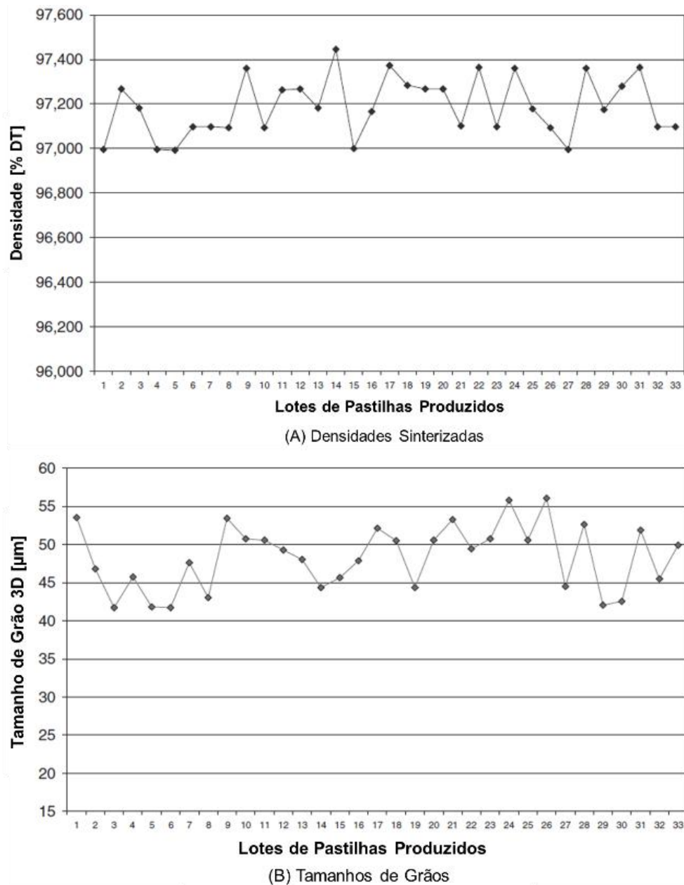
Figura 5: Estabilidade do processo produtivo das pastilhas ADOPT em relação a (A) densidades sinterizadas e (B) tamanhos de grãos. Adaptado de [2].
