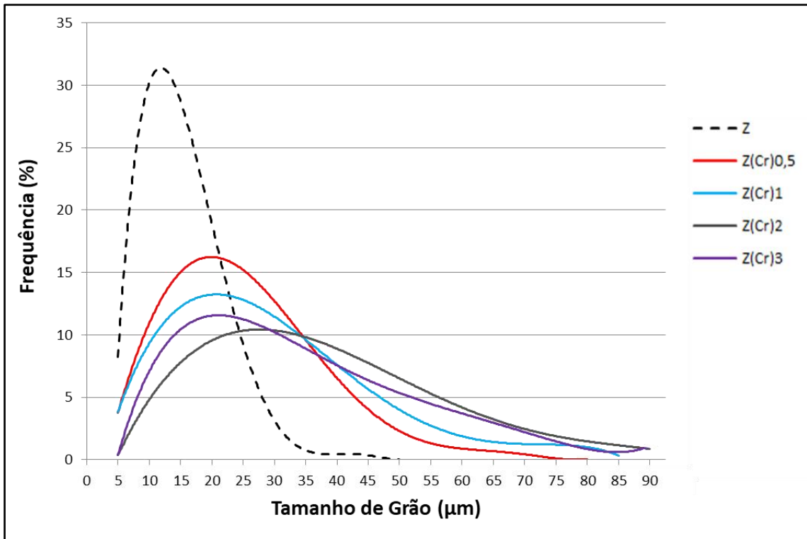
Figura 66: Influência da adição de 0,05; 0,10; 0,20 e 0,30 %p de crômio na distribuição dos tamanhos médios de grãos das pastilhas combustíveis de \text{Cr}_2\text{O}_3\text{-UO}_2 .
