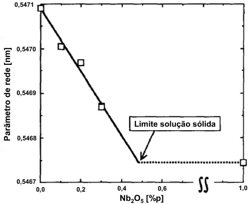
Figura 9: Relação do parâmetro de rede com a composição de Nb 2 O 5 para as pastilhas dopadas sinterizadas em atmosfera de H 2 umidificado acima de 1700°C. Adaptado de [26].
