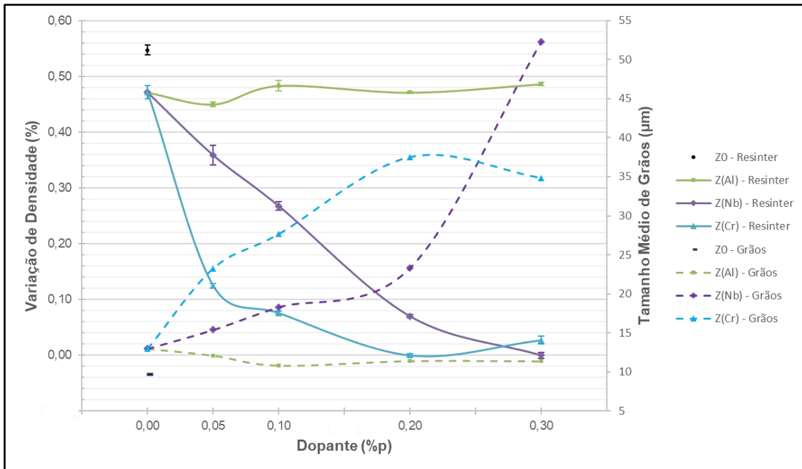
Figura 77: Relação entre a variação percentual de densidade (%) dos ensaios de resinterização com os tamanhos médios de grãos das pastilhas.
