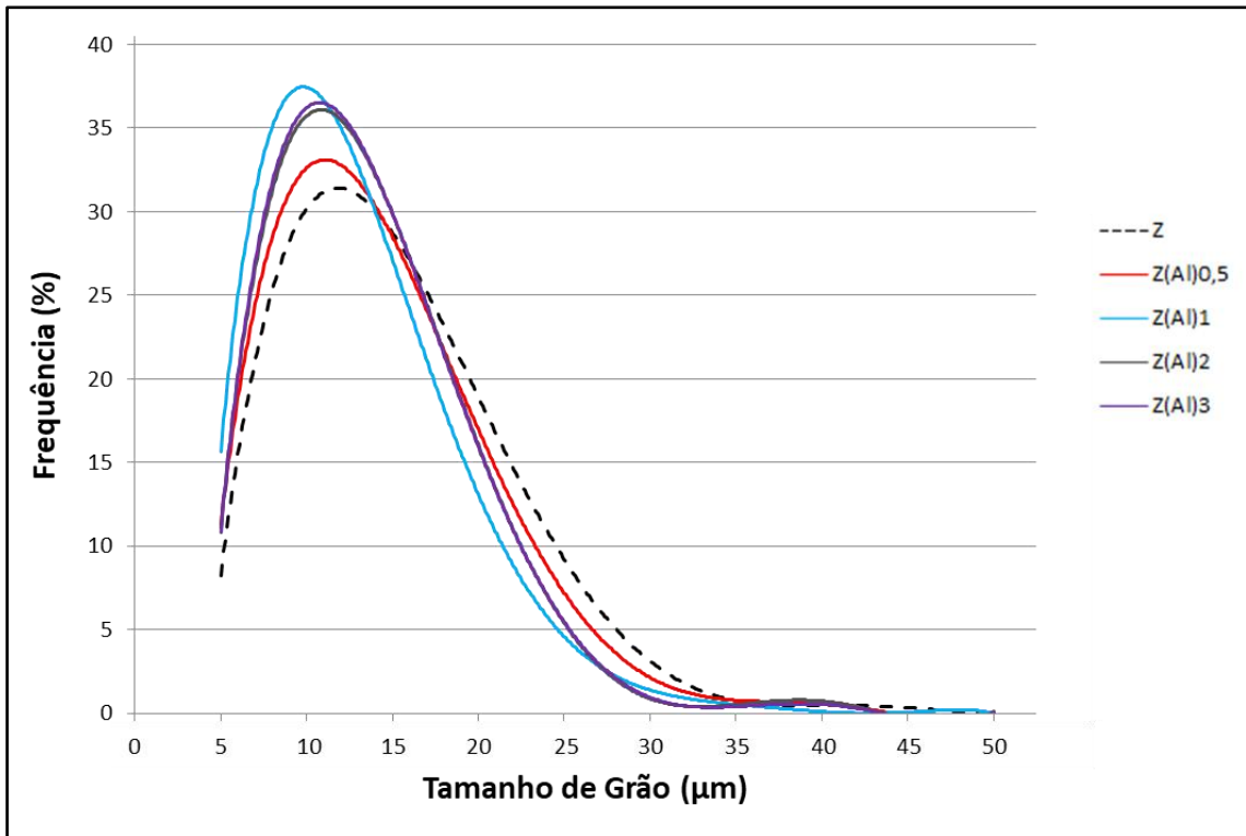
Figura 64: Influência da adição de 0,05; 0,10; 0,20 e 0,30 %p de alumina na distribuição dos tamanhos médios de grãos das pastilhas combustíveis de \text{Al}_2\text{O}_3\text{-UO}_2 .
