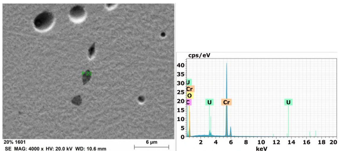
Figura 74: Micrografia da amostra \text{Z}(\text{Cr})_3 realizada em MEV com detector de elétrons secundários, com aumento de 4000x (esquerda), juntamente com as análises por EDS.
