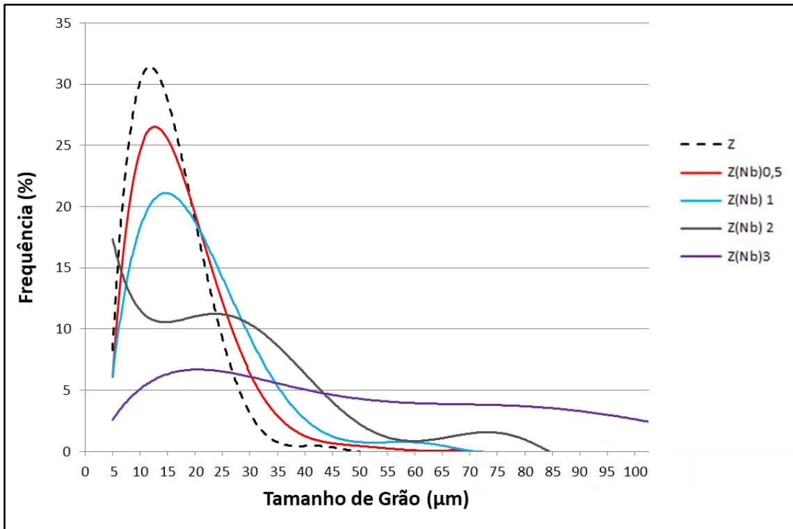
Figura 65: Influência da adição de 0,05; 0,10; 0,20 e 0,30 %p de nióbia na distribuição dos tamanhos médios de grãos das pastilhas combustíveis de Nb_2O_5-UO_2 .
