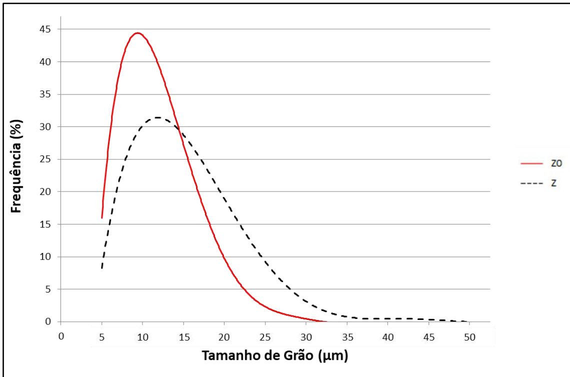
Figura 63: Influência da adição de 0,20 %p de ADS na distribuição dos tamanhos médios de grãos das pastilhas combustíveis de UO 2 .
