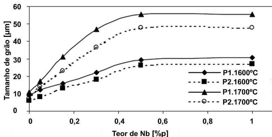
Figura 16: Tamanho de grão em função do teor de Nb. Adaptado de [5].
