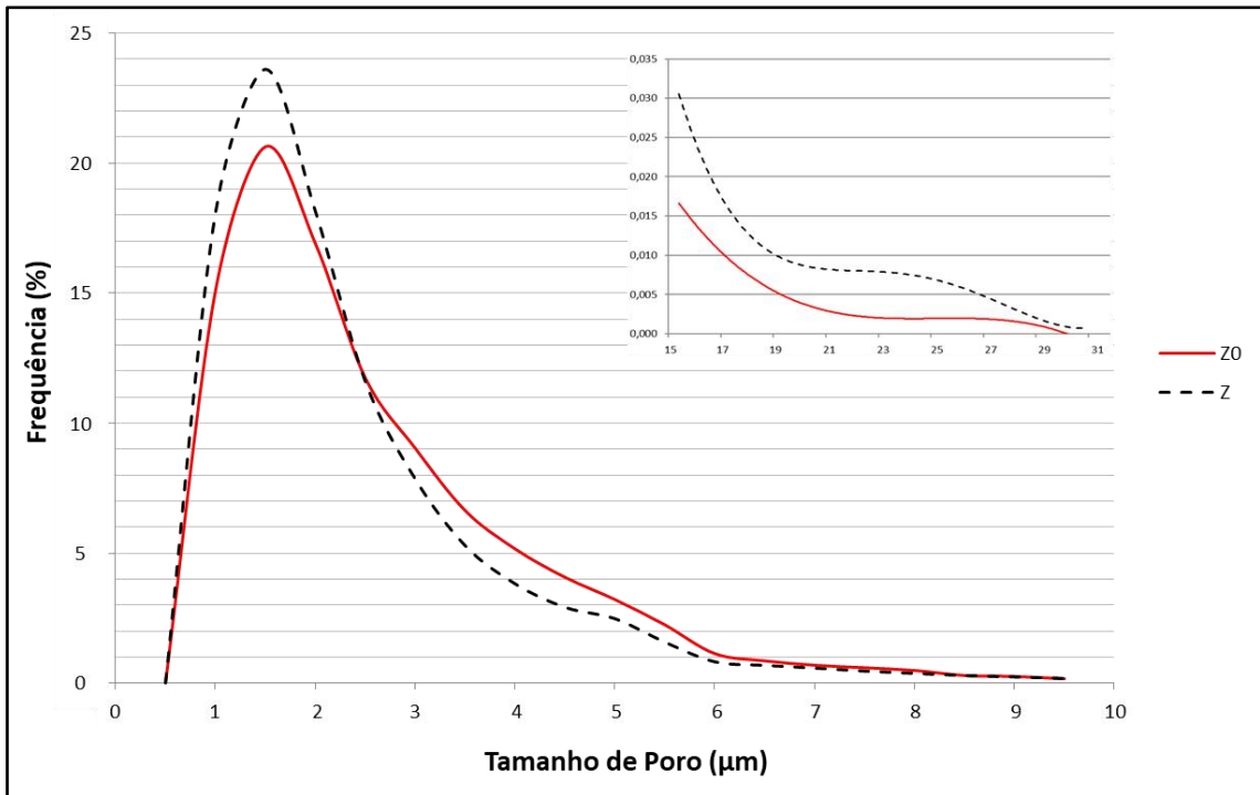
Figura 54: Distribuição dos tamanhos de poros ( \mu\text{m} ) das amostras Z0 e Z para as regiões de 0 a 10 \mu\text{m} e de 15 a 31 \mu\text{m} .
