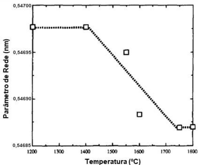
Figura 8: Variação do parâmetro de rede com a temperatura de sinterização das pastilhas dopadas com 0,3 %p de Nb_2O_5 , sinterizadas por 5 h em atmosfera de hidrogênio umidificado com ponto de orvalho entre 5 e 10°C. Adaptado de [26].
