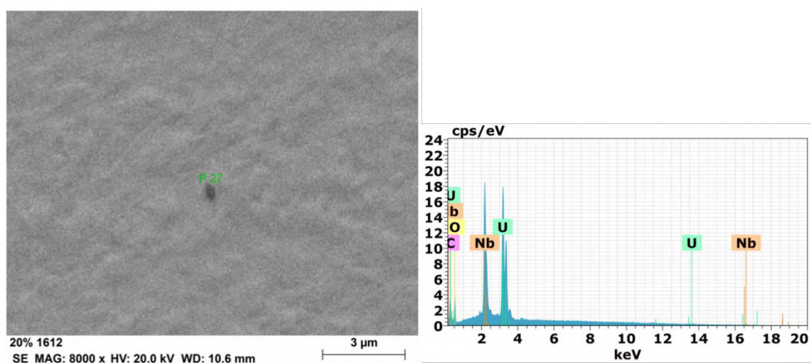
Figura 72 Micrografia da amostra Z(Nb)3 realizada em MEV com detector de elétrons secundários, com aumento de 8000x (esquerda), juntamente com as análises por EDS.
