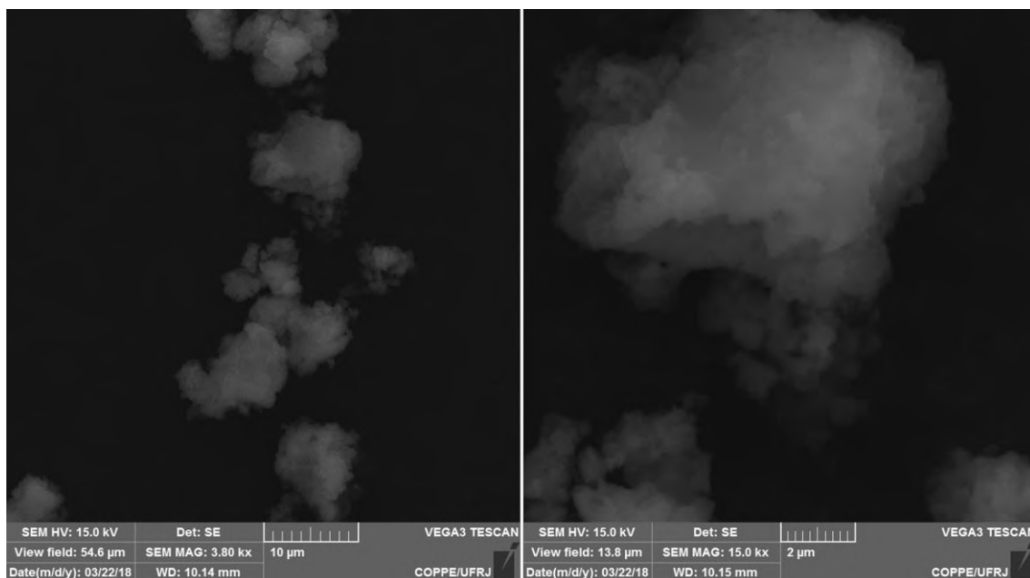
Figura 26: Micrografias do ADS realizadas em MEV com detector de elétrons secundários, com aumentos nominais de 3800x (esquerda) e 15000x (direita).
