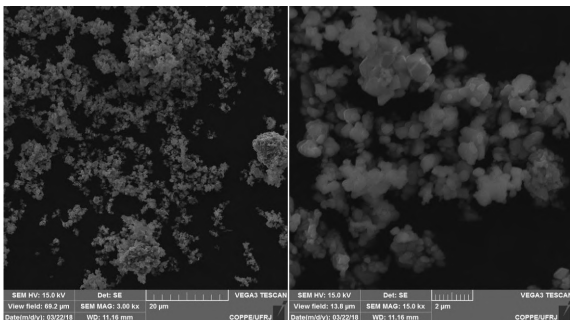
Figura 29: Micrografias da crômia realizadas em MEV com detector de elétrons secundários, com aumentos nominais de 3000x (esquerda) e 15000x (direita).
