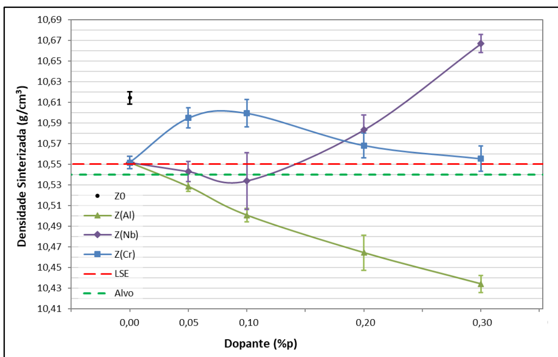
Figura 46: Variação da densidade sinterizada média com a adição de 0,05; 0,10; 0,20 e 0,30 %p de Al 2 O 3 , Nb 2 O 5 e Cr 2 O 3 (%p = g Metal/g U).
