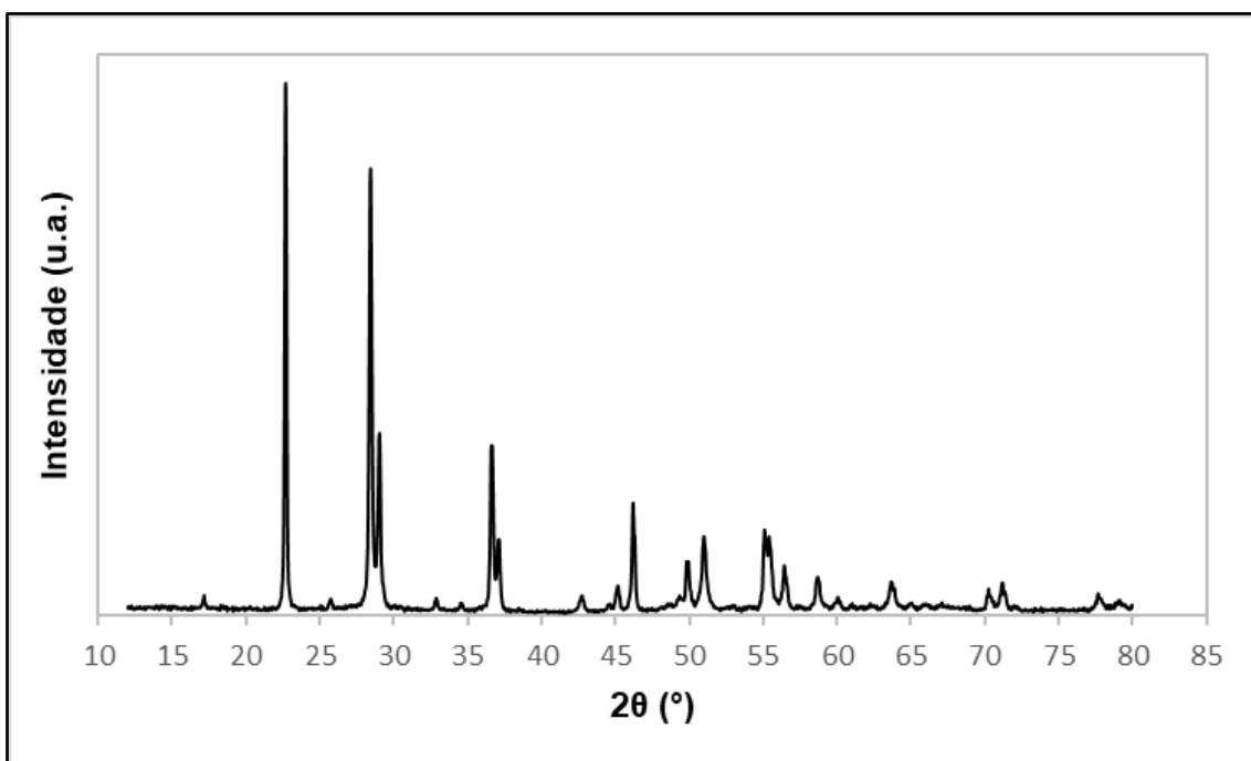
Figura 31: Difratoograma de raios-X da nióbia utilizada como dopante.
