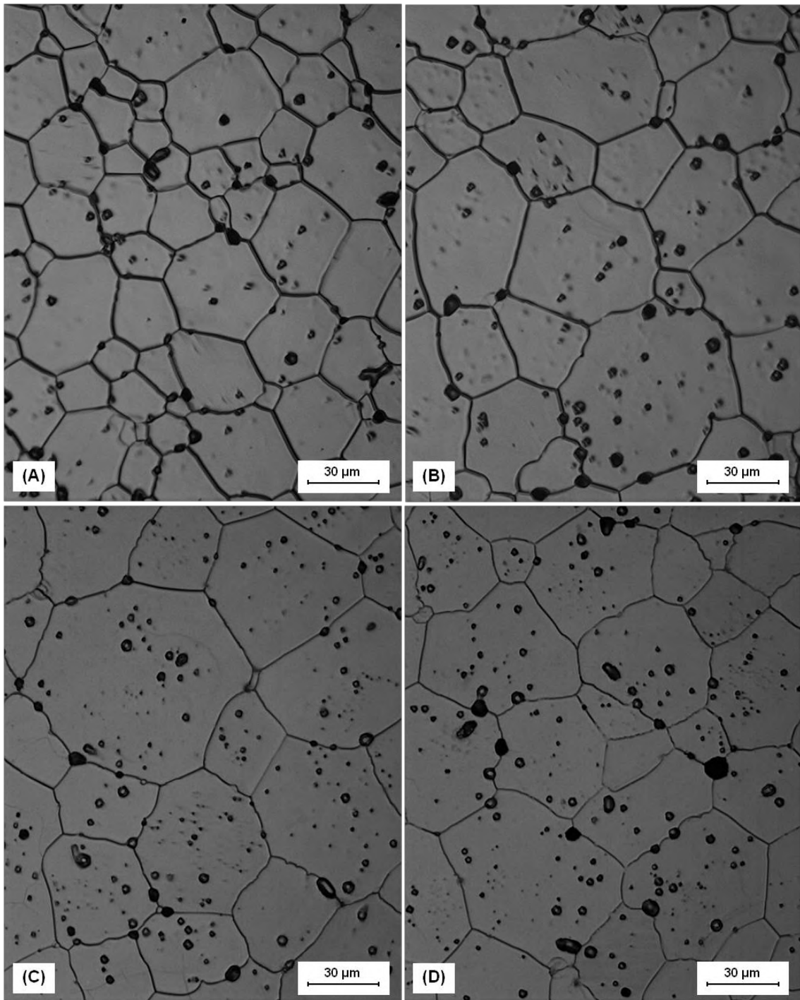
Figura 70: Microestruturas de grãos das pastilhas atacadas termicamente com \text{CO}_2 por 1 h a 1400^\circ\text{C} , obtidas por microscopia óptica com aumento de 500x, das amostras (A) Z(Cr)0,5; (B) Z(Cr)1, (C) Z(Cr)2 e (D) Z(Cr)3.
