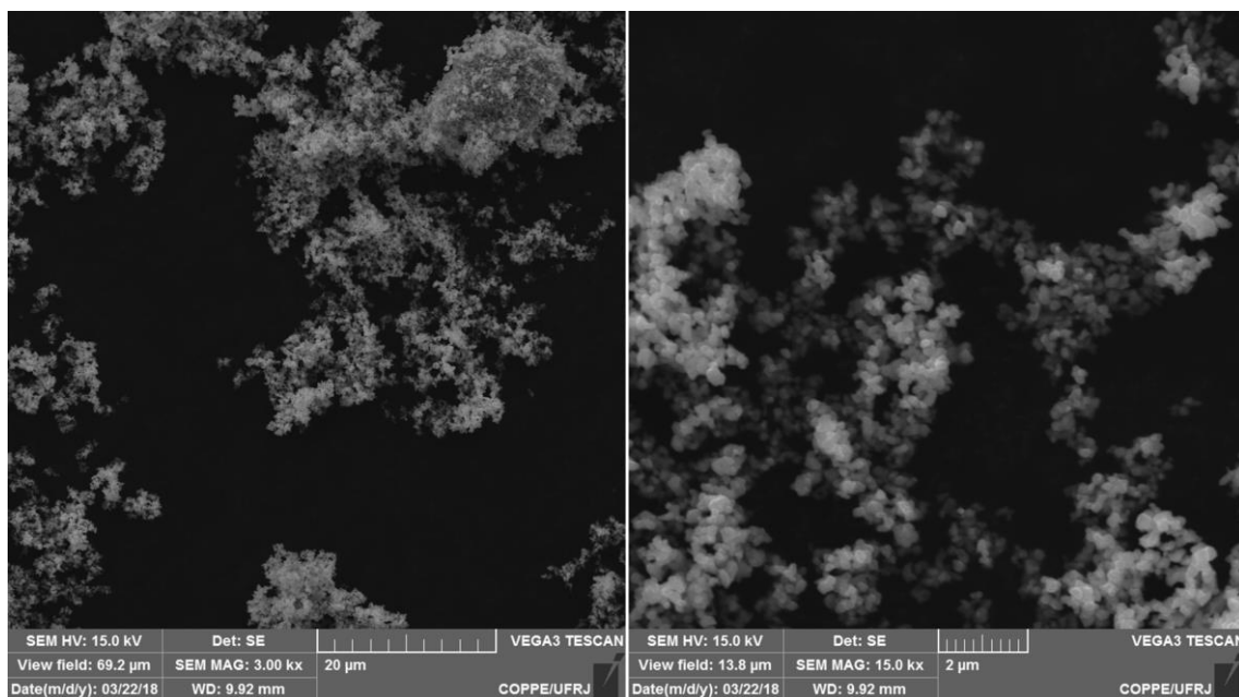
Figura 28: Micrografias da nióbia realizadas em MEV com detector de elétrons secundários, com aumentos nominais de 3000x (esquerda) e 15000x (direita).
