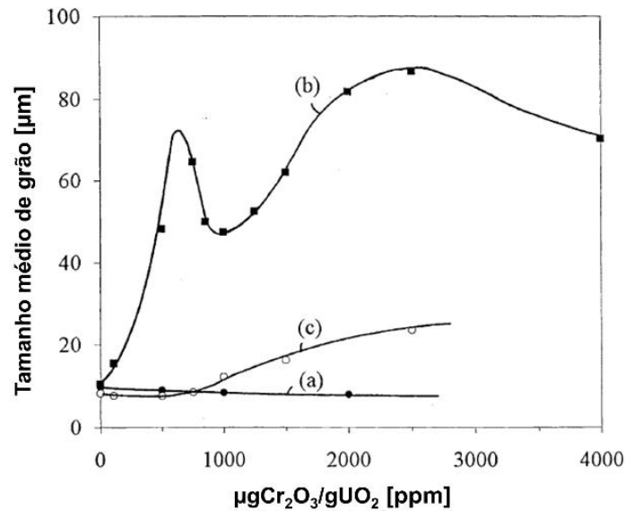
Figura 17: Relação entre o tamanho médio de grãos e a quantidade de Cr 2 O 3 em (a) H 2 + 0,05%v H 2 O, (b) H 2 + 1%v H 2 O e (c) H 2 + 5%v H 2 O. Adaptado de [10].
