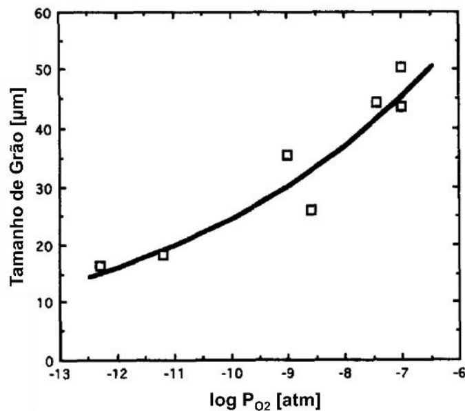
Figura 11: Crescimento de grão das pastilhas dopadas com 0,3 %p de Nb 2 O 5 em função da pressão parcial de O 2 na atmosfera de sinterização (1400°C por 5 h). Adaptado de [26].
