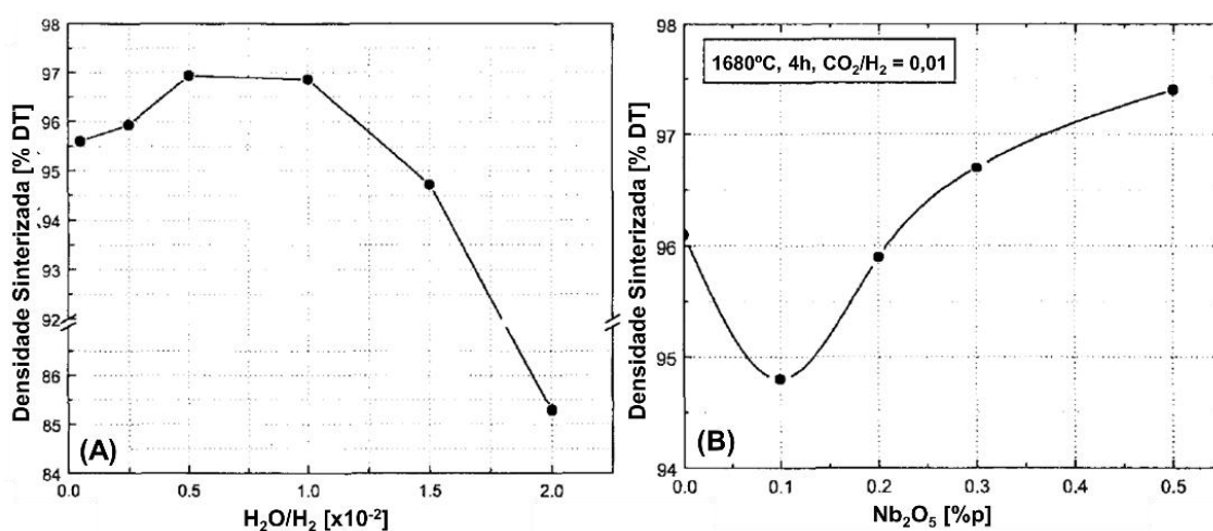
Figura 13: Variação da densidade sinterizada das (A) pastilhas dopadas com 0,3 %p de nióbia em função da razão \text{H}_2\text{O}/\text{H}_2 sinterizadas a 1700^\circ\text{C} e (B) sinterizadas a 1680^\circ\text{C} por 4 h variando a adição de nióbia em atmosfera com razão \text{CO}_2/\text{H}_2 = 0,01 . Adaptado de [28].
