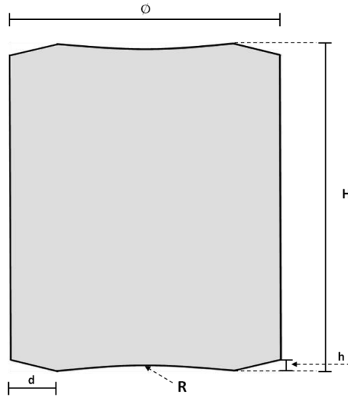
Figura 37: Perfil geométrico da pastilha de UO_2 , onde: \varnothing = diâmetro da pastilha; H = altura da pastilha; h = altura do ombro (0,12 mm); R = raio esférico (0,38 mm); e d = comprimento do ombro (1,92 mm). Todas as cotas estão em “mm” na especificação de produto da INB.
