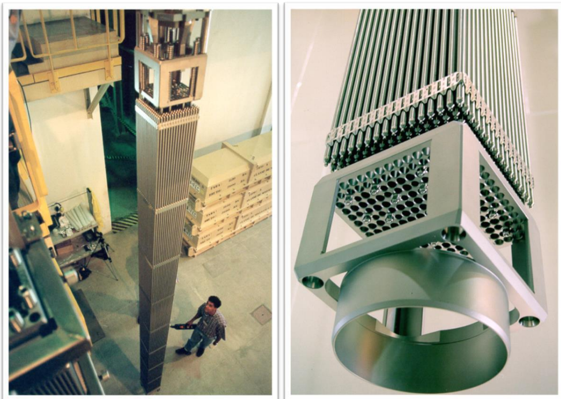
Figura 4: Elemento combustível final do projeto Angra 2 em escala real (à esquerda) e em destaque a parte inferior (à direita).
