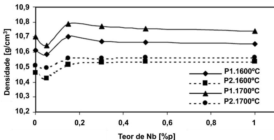
Figura 15: Densidade sinterizada das pastilhas em função do teor de Nb. Adaptado de [5].
