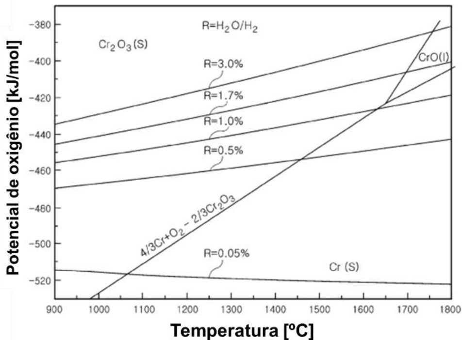
Figura 23: Fases em equilíbrio em função do potencial de oxigênio (razão R = \text{H}_2\text{O}/\text{H}_2 ) e da temperatura de sinterização. Adaptado de [36].
