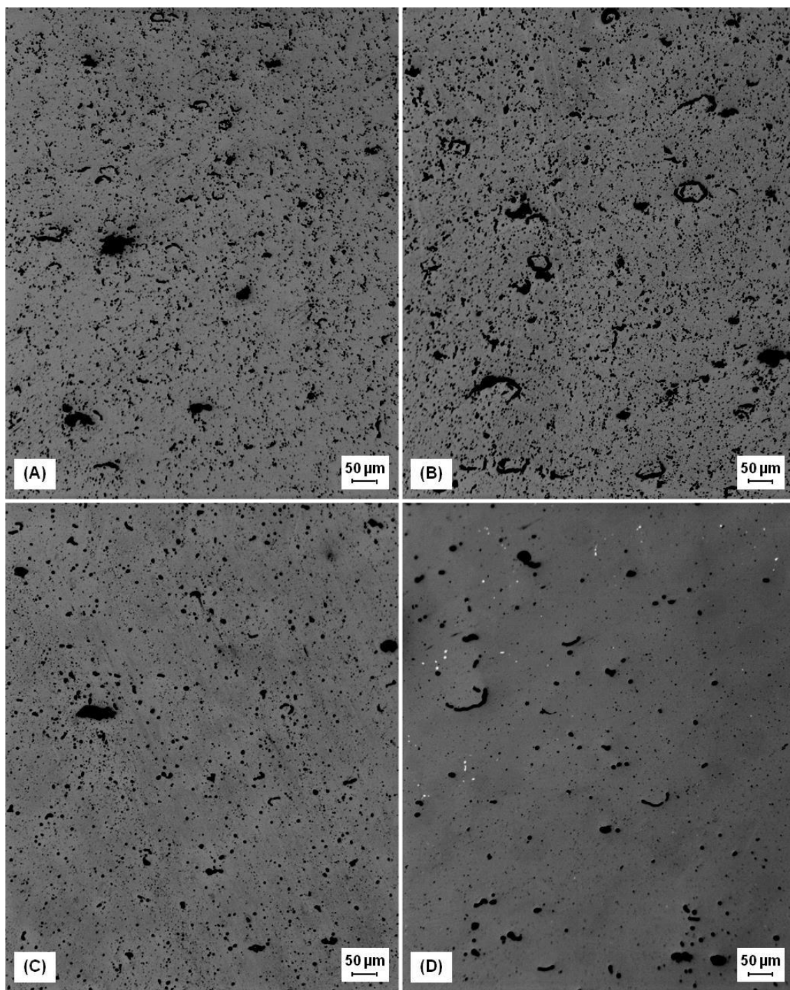
Figura 60: Estrutura de poros das pastilhas de \text{UO}_2 polidas, obtidas por microscopia óptica com aumento de 100x, das amostras (A) \text{Z(Nb)}_{0,5} ; (B) \text{Z(Nb)}_1 , (C) \text{Z(Nb)}_2 e (D) \text{Z(Nb)}_3 .
