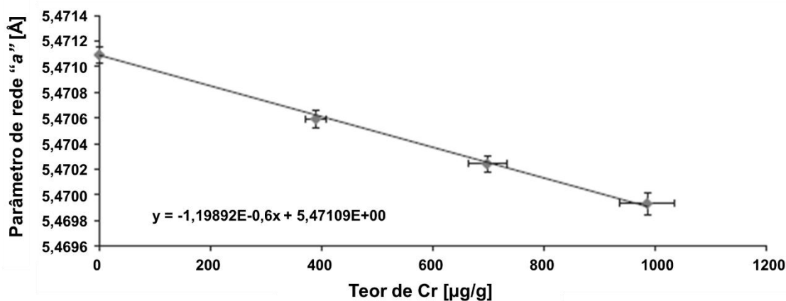
Figura 24: Parâmetro de rede a em função do teor de Cr. Adaptado de [40].
