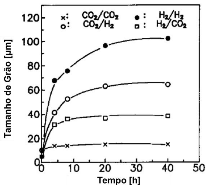
Figura 7: Tamanhos de grãos das pastilhas dopadas com nióbia em função do tempo para várias condições de sinterização. Adaptado de [13].
