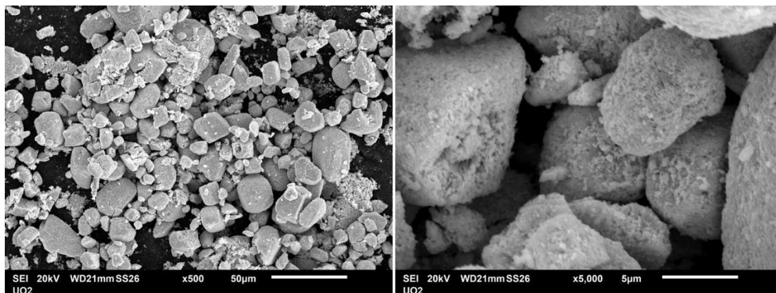
Figura 34: Micrografias em MEV com detector de elétrons secundários do pó de \text{UO}_2 padrão da INB, com aumentos nominais de 500x (esquerda) e 5000x (direita).
