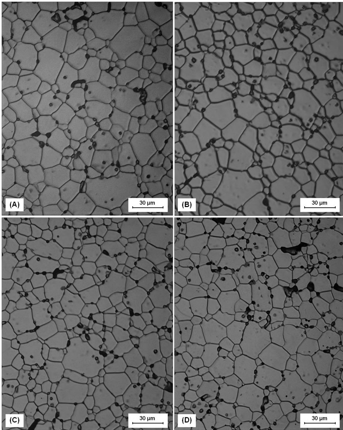
Figura 68: Microestruturas das pastilhas atacadas termicamente com \text{CO}_2 por 1 h a 1400^\circ\text{C} , obtidas por microscopia óptica com aumento de 500x, das amostras (A) \text{Z(Al)}_{0,5} ; (B) \text{Z(Al)}_1 , (C) \text{Z(Al)}_2 e (D) \text{Z(Al)}_3 .
