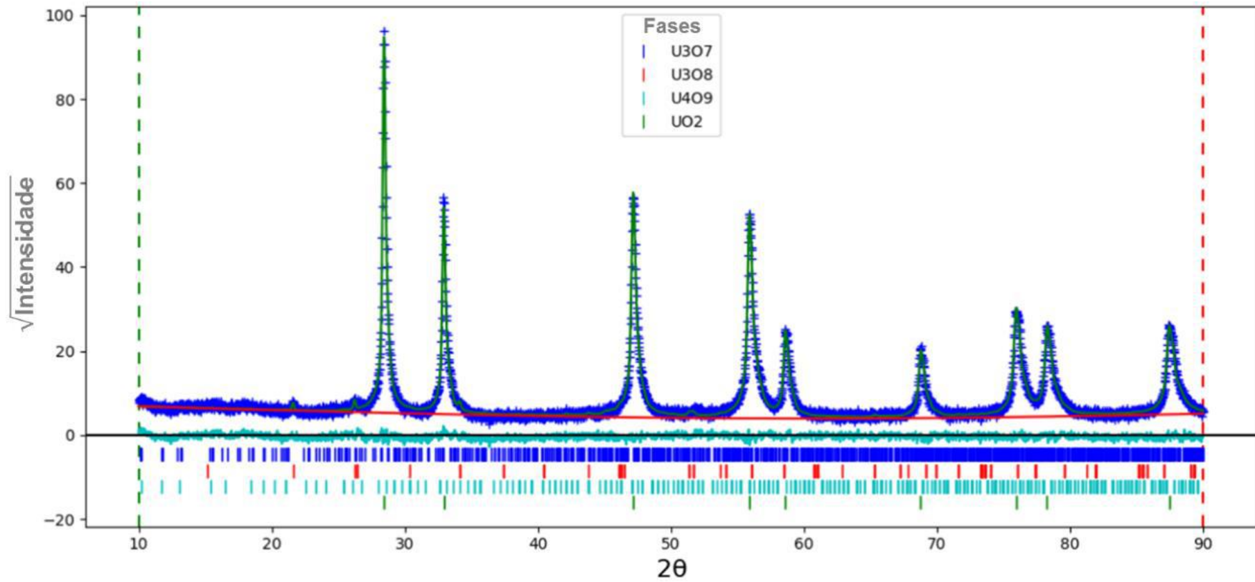
Figura 33: Difratograma do pó de \text{UO}_2 precursor das amostras.
