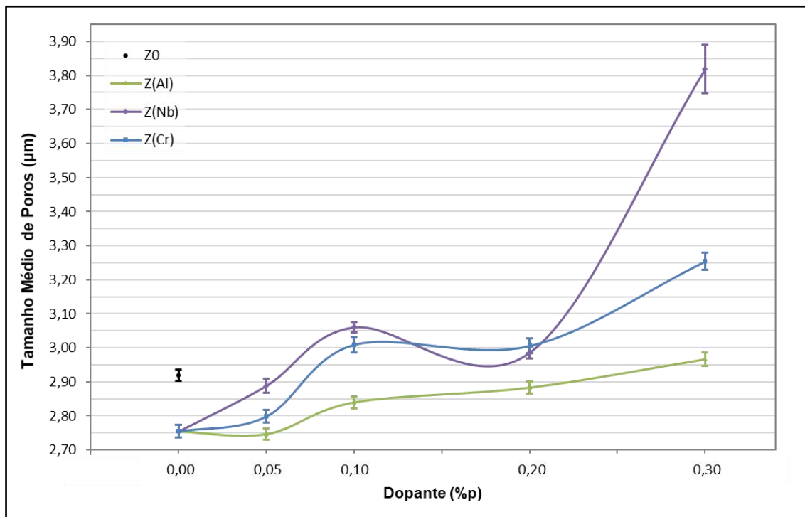
Figura 53: Variação do tamanho médio de poros em função da adição de 0,05; 0,10; 0,20 e 0,30 %p de \text{Al}_2\text{O}_3 , \text{Nb}_2\text{O}_5 e \text{Cr}_2\text{O}_3 (%p = g Metal/g U).
