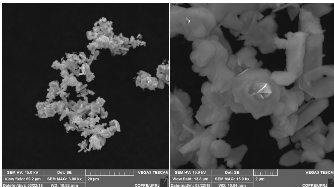
Figura 27: Micrografias da alumina realizadas em MEV com detector de elétrons secundários, com aumentos nominais de 3000x (esquerda) e 15000x (direita).
