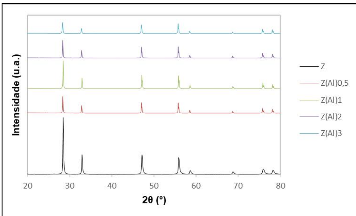
Figura 50: Difratomogramas de raios-X das amostras Z, Z(Al)0,5; Z(Al)1, Z(Al)2 e Z(Al)3.
