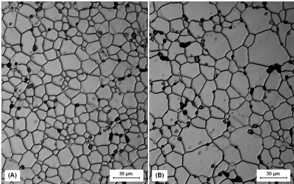
Figura 67: Microestruturas das pastilhas atacadas termicamente com \text{CO}_2 por 1 h a 1400^\circ\text{C} , obtidas por microscopia óptica com aumento de 500x, das amostras (A) Z0 e (B) Z.
