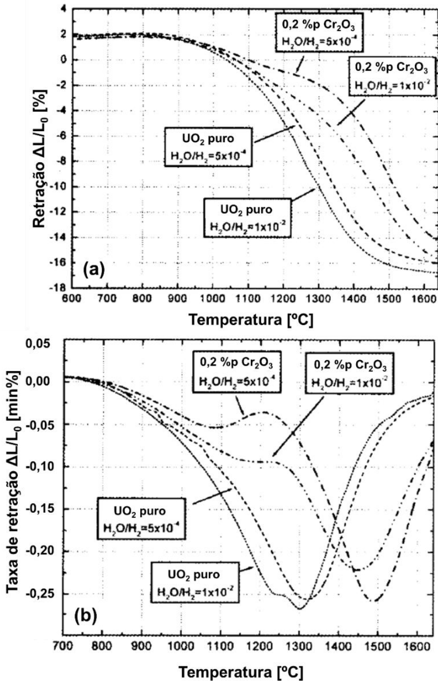
Figura 20: Curvas de densificação das pastilhas verdes com e sem adição de 0,2 %p de Cr_2O_3 nas atmosferas do tipo A ( H_2O/H_2 = 5 \times 10^{-4} ) e B ( H_2O/H_2 = 1 \times 10^{-2} ): (a) Retração; e (b) Taxa de retração. Adaptado de [11].
