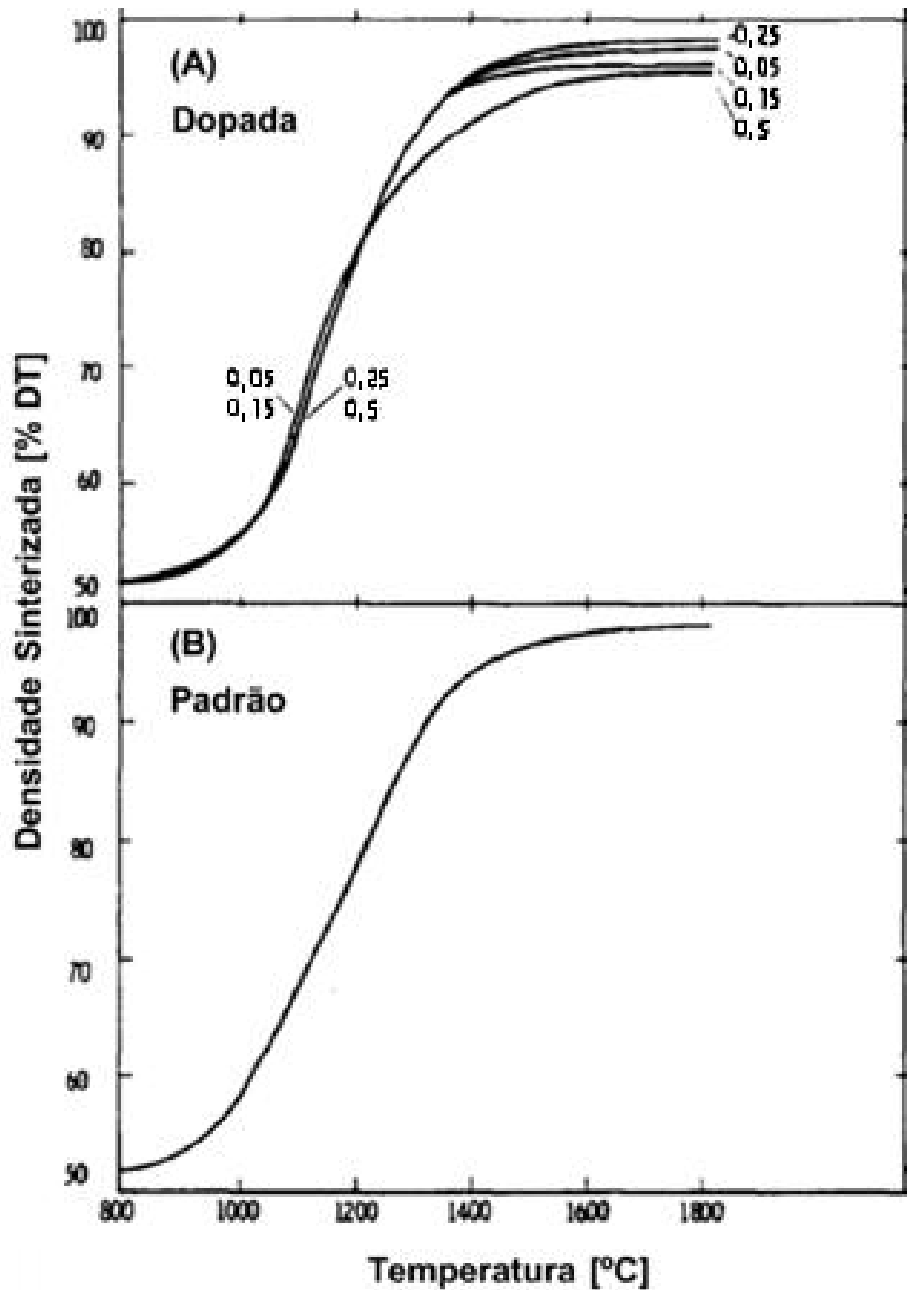
Figura 6: Cinética de sinterização das (A) pastilhas dopadas com nióbia e da (B) pastilha de UO_2 padrão. Adaptado de [24].
