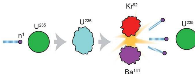
Figura 1: Exemplo de reação de fissão nuclear do isótopo físsil do urânio ^{235}\text{U} . Adaptado de [6].
