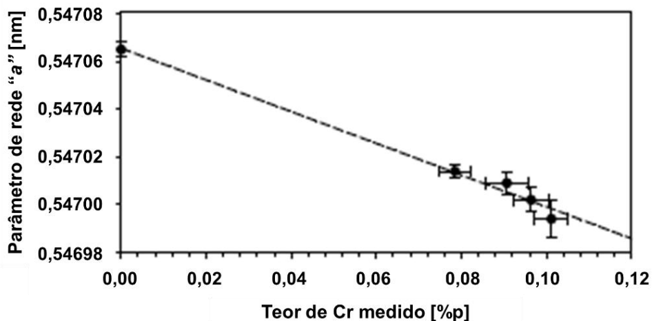
Figura 22: Parâmetro de rede "a" obtido em função do teor de Cr medido por EPMA. A linha pontilhada representa a análise de regressão linear. Adaptado de [34].
