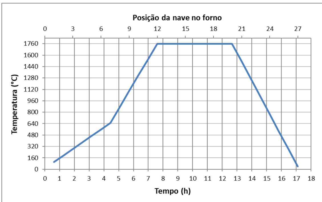
Figura 40: Perfil aproximado de temperatura do forno industrial (GWSmo 16/14/210) em função do tempo de alimentação e da posição da nave contendo as amostras (~38 min/posição).
