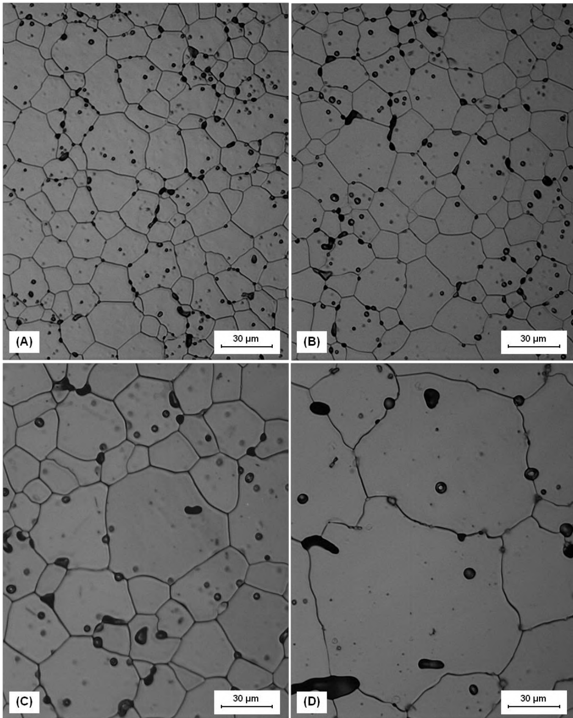
Figura 69: Microestruturas das pastilhas atacadas termicamente com \text{CO}_2 por 1 h a 1250^\circ\text{C} , obtidas por microscopia óptica com aumento de 500x, das amostras (A) \text{Z(Nb)}_{0,5} ; (B) \text{Z(Nb)}_1 , (C) \text{Z(Nb)}_2 e (D) \text{Z(Nb)}_3 .
