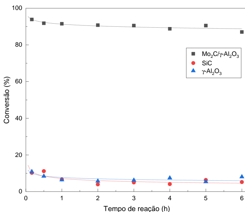
Figura D.1: Conversão do ácido oleico em função do tempo de reação empregando-se \text{Mo}_2\text{C}/\gamma\text{-Al}_2\text{O}_3 , e os testes em branco com SiC e \gamma\text{-Al}_2\text{O}_3 (WHSV = 20 \text{h}^{-1} , T = 340 °C, P_{\text{H}_2} = 30 bar; as linhas de tendência foram adicionadas apenas para facilitar a visualização).
