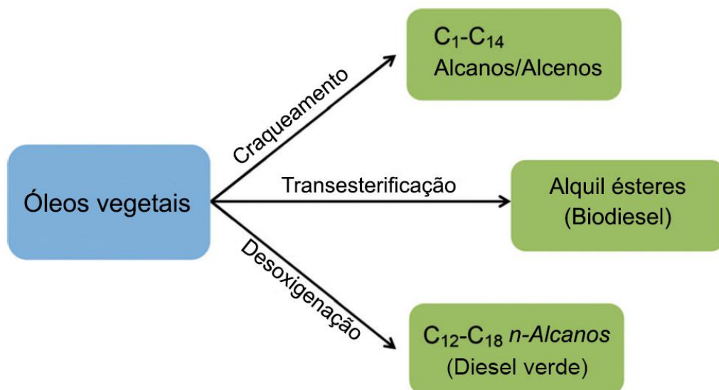
Figura 2.7: Principais processos para a produção de biocombustíveis a partir de óleos vegetais (Adaptado de GOSSELINK et al. [6]).
