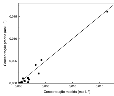
(h) Octadecano; R = 0,9852 .
