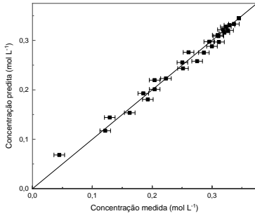
(a) Ácido oleico; R = 0,9915 .
