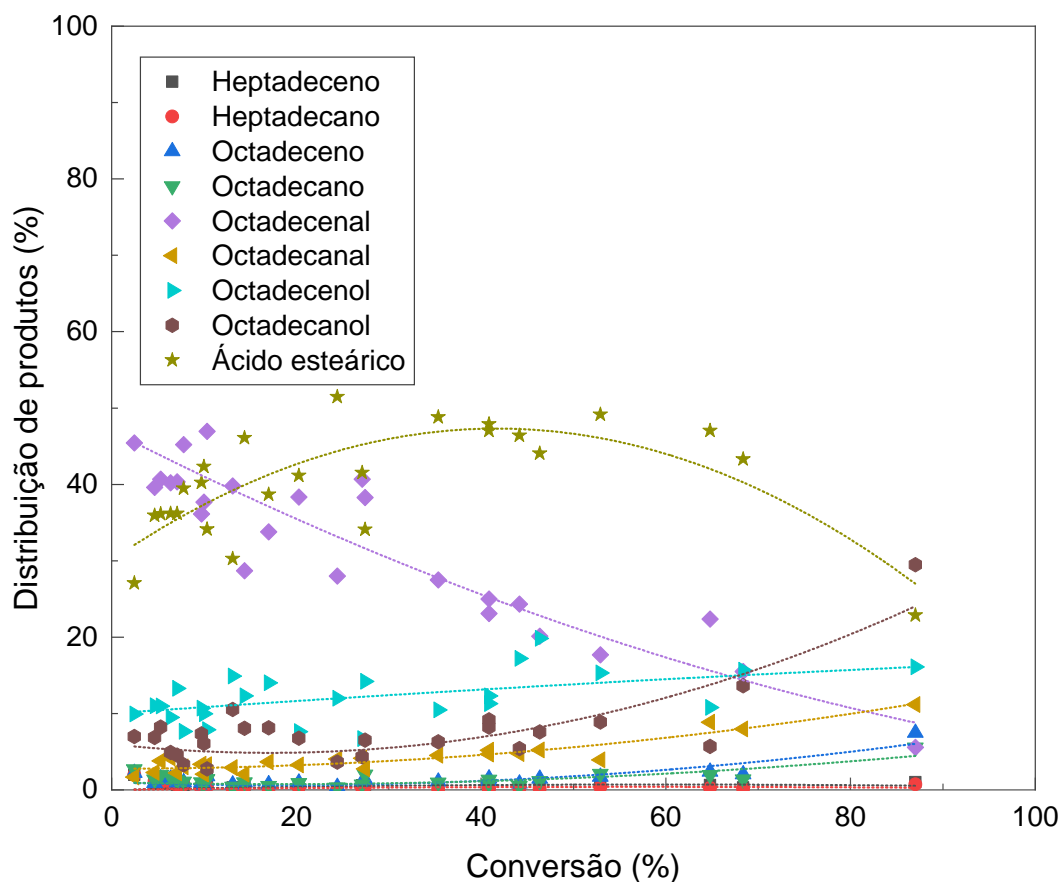
Figura 3.14: Distribuição de produtos líquidos em função da conversão na reação de hidroxidação do ácido oleico empregando Mo_2C/\gamma-Al_2O_3 ( T = 260-340\text{ }^{\circ}C ; WHSV = 20-60\text{ h}^{-1} ; P_{H_2} = 30\text{ bar} ; as linhas de tendência foram adicionadas apenas para facilitar a visualização).
