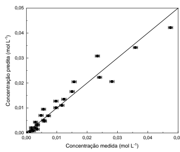
(e) Octadecenol; R = 0,9600 .
