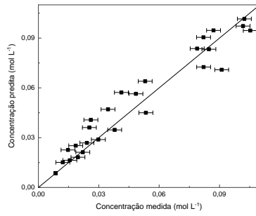
(b) Ác. esteárico; R = 0,9648 .
