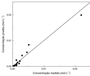
(g) Octadeceno; R = 0,9780 .
