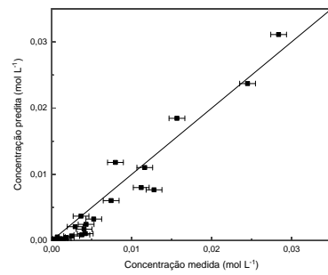
(f) Octadecanol; R = 0,9204 .
