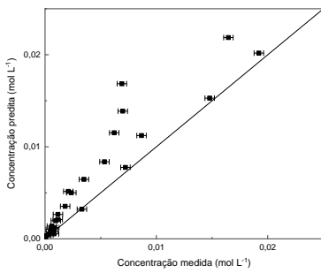
(d) Octadecanal; R = 0,8737 .
