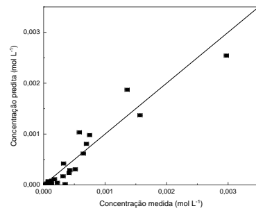
(i) Heptadeceno; R = 0,9528 .
