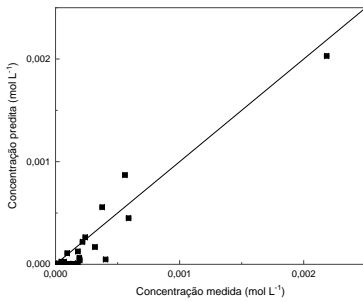
(j) Heptadecano; R = 0,9572 .
