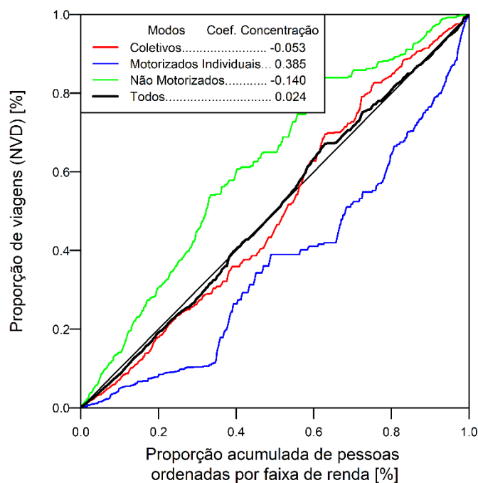
Figura 4: Exemplo de curvas de concentração Fonte: Carneiro et al. (2018) elaborado a partir do PDTU (2015)
