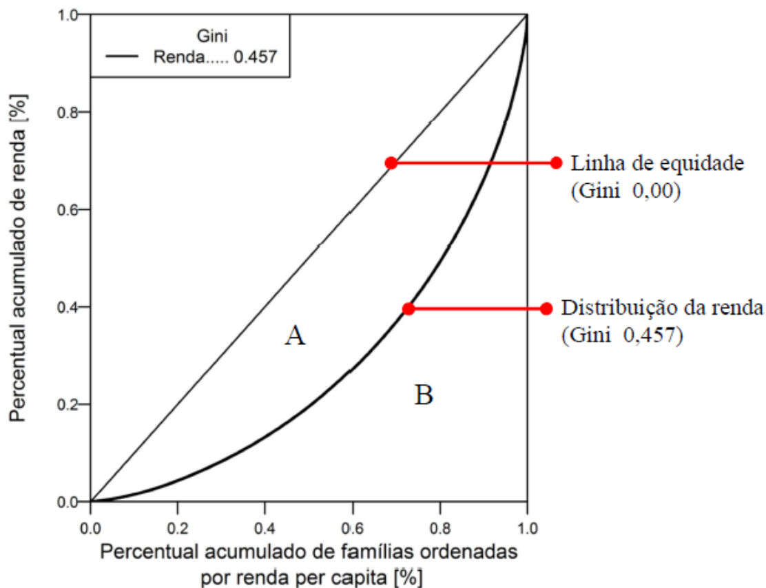
Figura 3: Exemplo de curva de Lorenz Fonte: Falavigna (2015)
