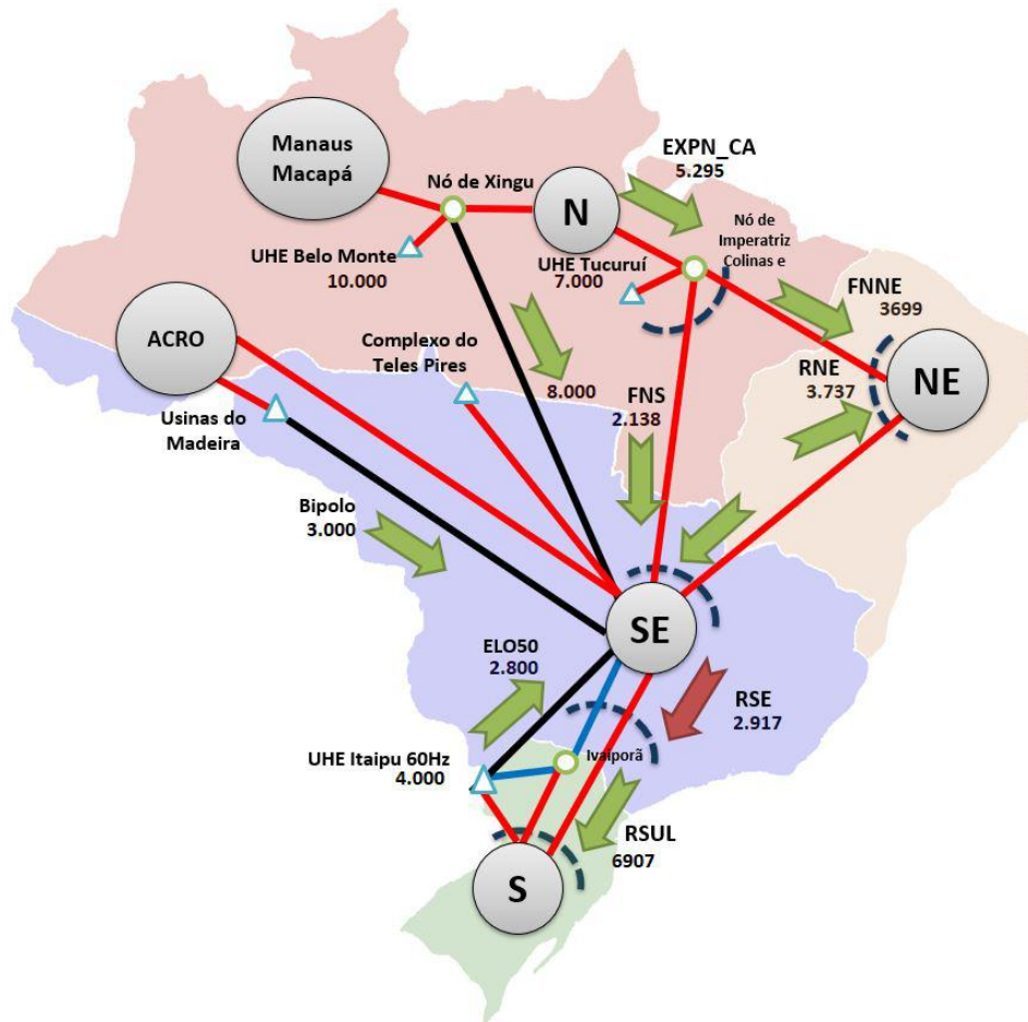
Figura 6.2: Principais fluxos sistêmicos no caso base do SIN.
