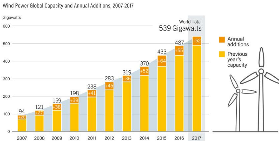
Figura 1.3: Evolução da capacidade mundial instalada de geração eólica de 2007 a 2017. Fonte: [2].
