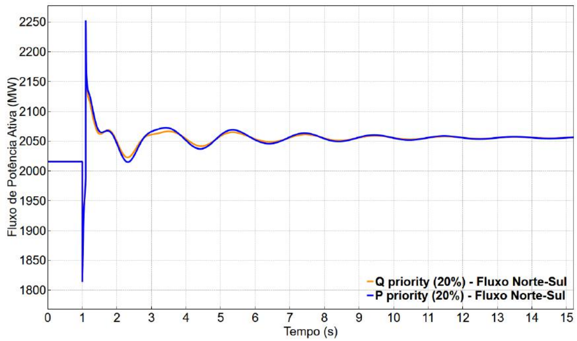
(c) Fluxo de ativo na Interligação Norte-Sul (20% penetração).
