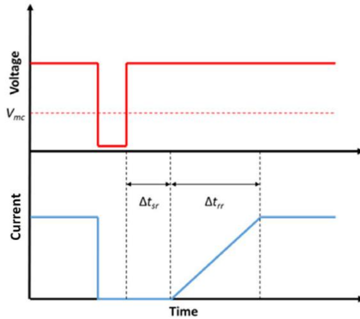
Figura 3.5: Voltage ride through com bloqueio temporário da corrente do inversor. Ao detectar grande variação de tensão o inversor bloqueia a injeção de corrente. Após a recuperação da tensão, o inversor aguarda um intervalo de tempo \Delta t_{sr} para voltar a injetar corrente na rede. Em seguida, durante \Delta t_{rr} , a corrente recupera-se em rampa até os valores pré falta. Fonte: [17].
