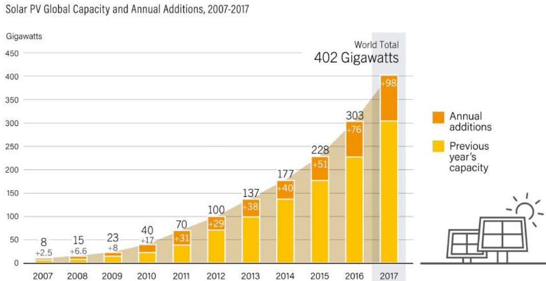
Figura 1.2: Evolução da capacidade mundial instalada de geração solar fotovoltaica de 2007 a 2017. Fonte: [2].
