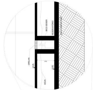
3 IMPLANTAÇÃO ESCALA 1:10
