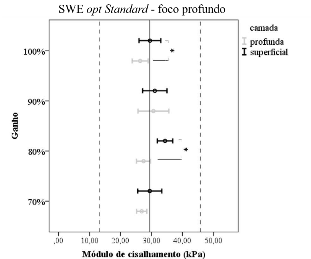
Figura 31: O gráfico de barras de erros mostra as médias de módulo de cisalhamento em cada ganho, separando as camadas superficial e profunda na carne. A linha central representa a média geral de todos os ganhos com a configuração SWE opt standard – foco profundo. As linhas tracejadas representam a variância das medidas obtidas com a configuração (* p < 0,05 ).
