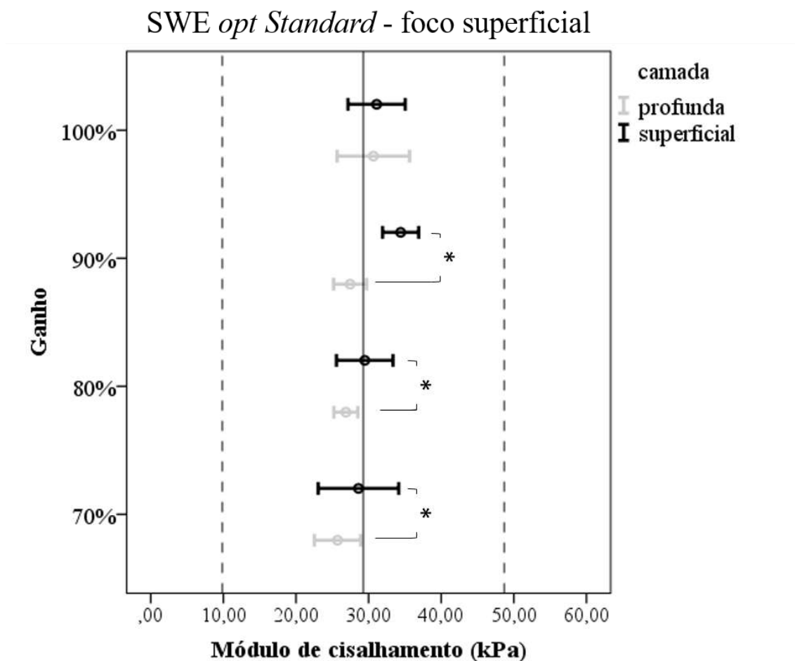
Figura 30: O gráfico de barras de erros mostra as médias de módulo de cisalhamento em cada ganho, separando as camadas superficial e profunda na carne. A linha central representa a média geral de todos os ganhos com a configuração SWE opt standard – foco superficial. As linhas tracejadas representam a variância das medidas obtidas com a configuração (* p < 0,05 ).
