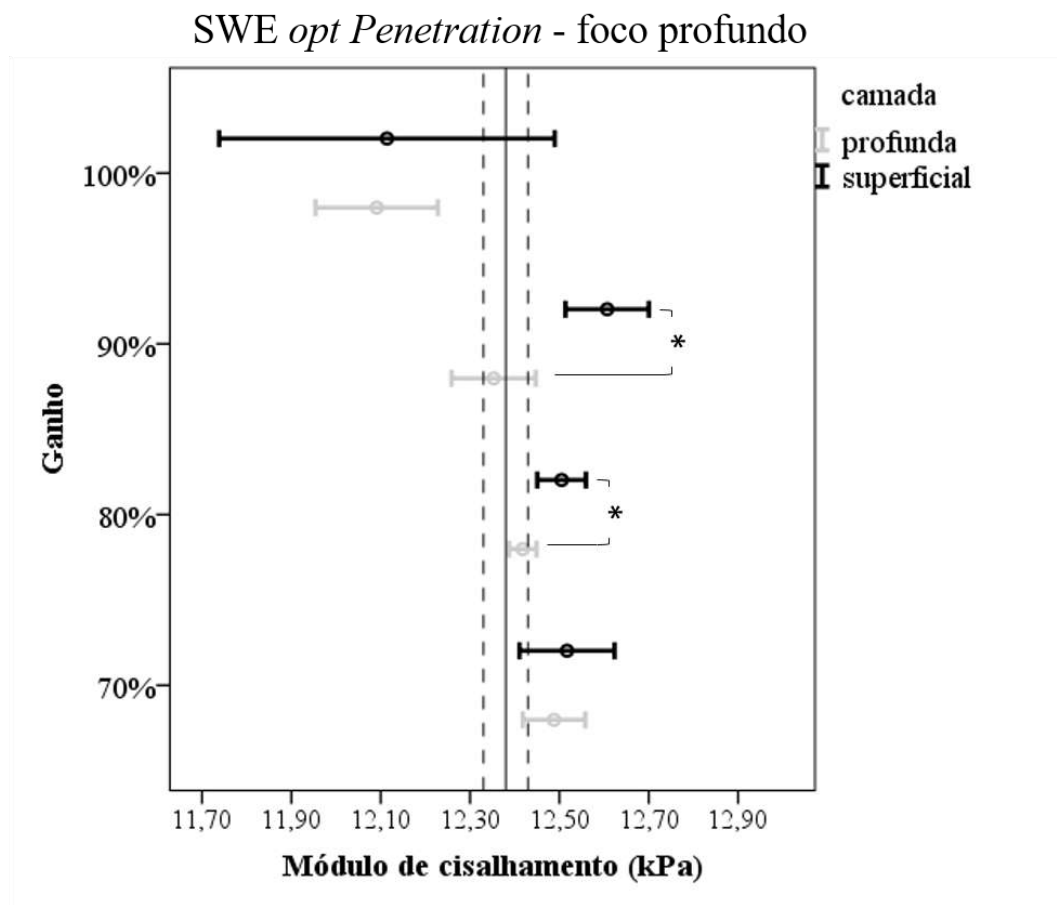
Figura 29: O gráfico de barras de erros mostra as médias de módulo de cisalhamento em cada ganho, separando as camadas superficial e profunda na gelatina. A linha central representa a média geral de todos os ganhos com a configuração SWE opt penetration – foco profundo. As linhas tracejadas representam a variância das medidas obtidas com a configuração (* p < 0,05 ).
