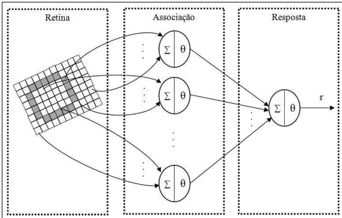
Figura 62: Representação da topologia de um perceptron simples com uma única saída.
