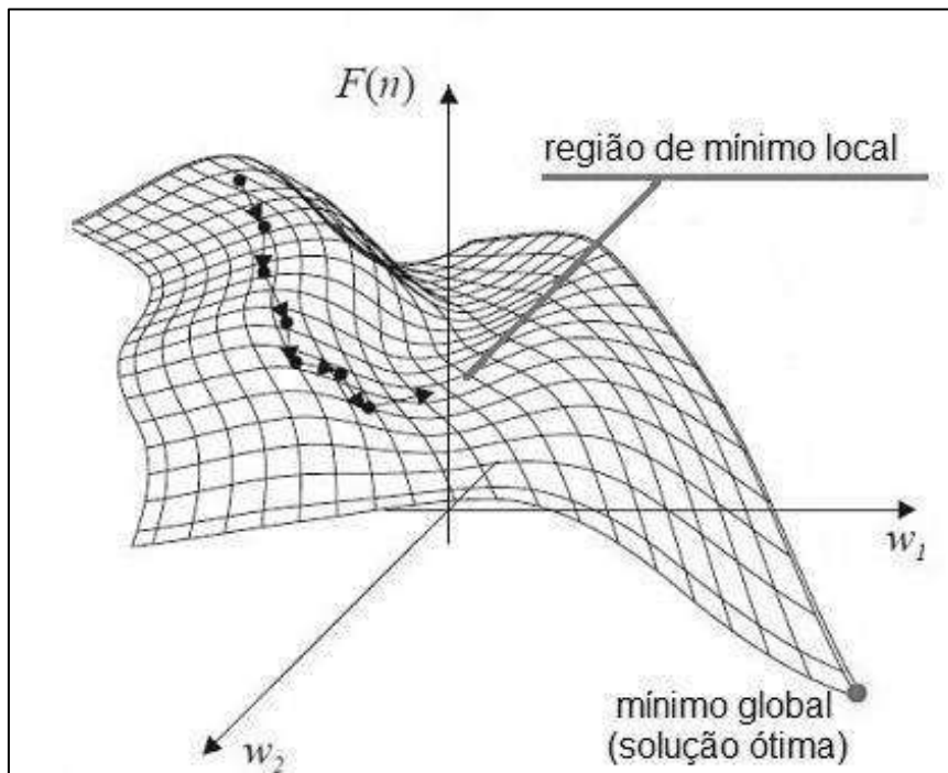
Figura 67: Exemplo de superfície de erro.
