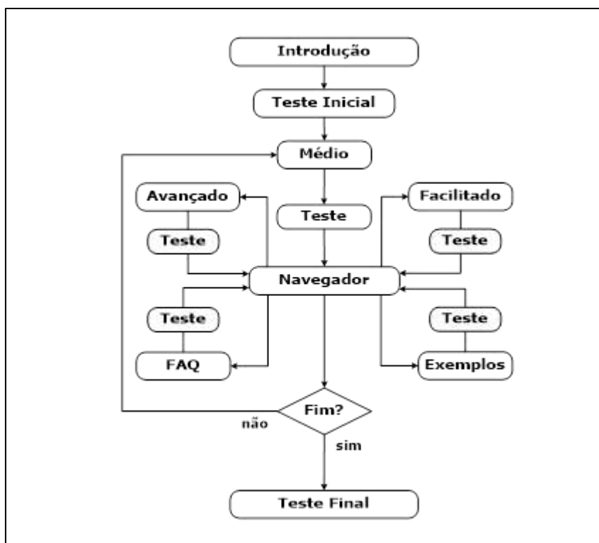
Figura 77: A estrutura do STI de Carvalho (CARVALHO, 2002)
