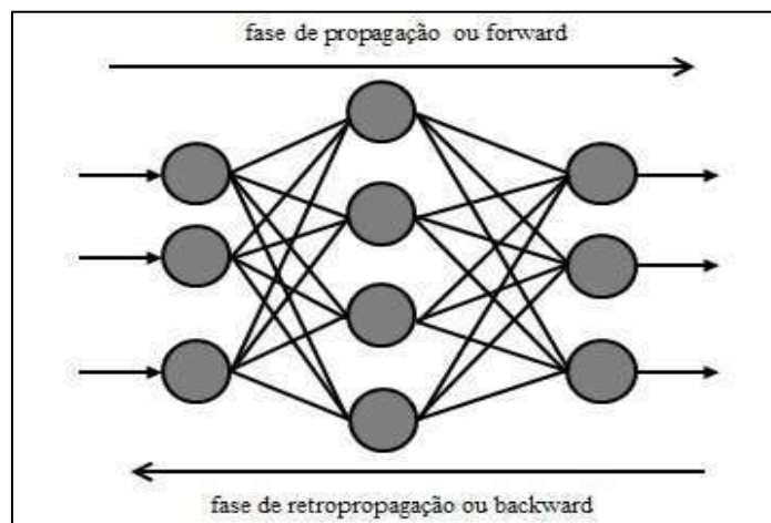
Figura 64: Fases do treinamento da Rede MLP, utilizando algoritmo backpropagation .
