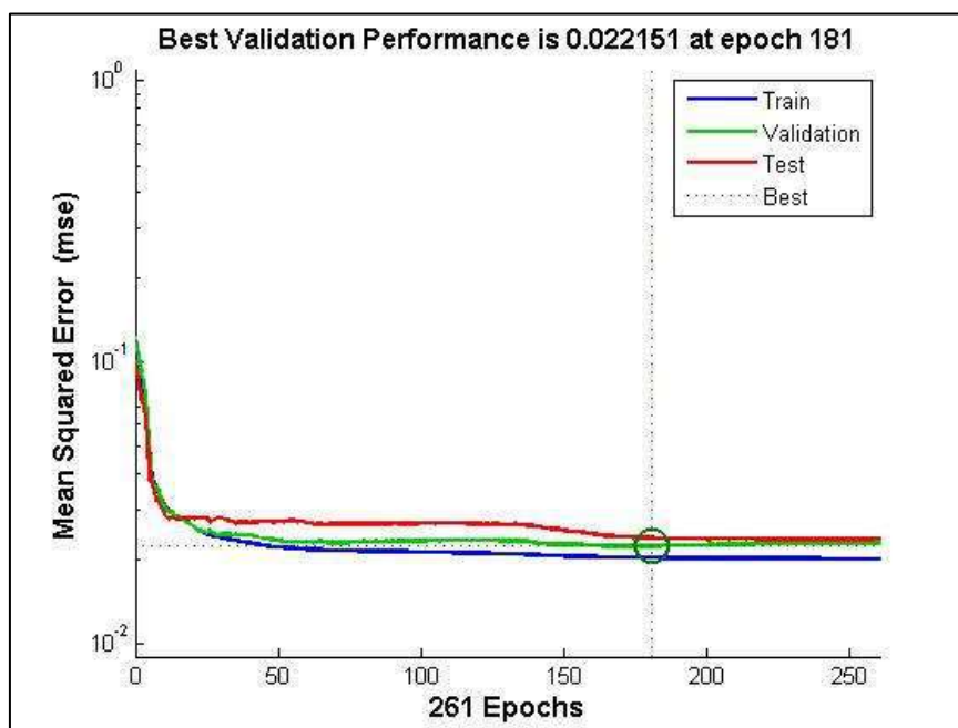
Figura 163: Gráfico de treinamento da rede neural do navegador de conteúdo
