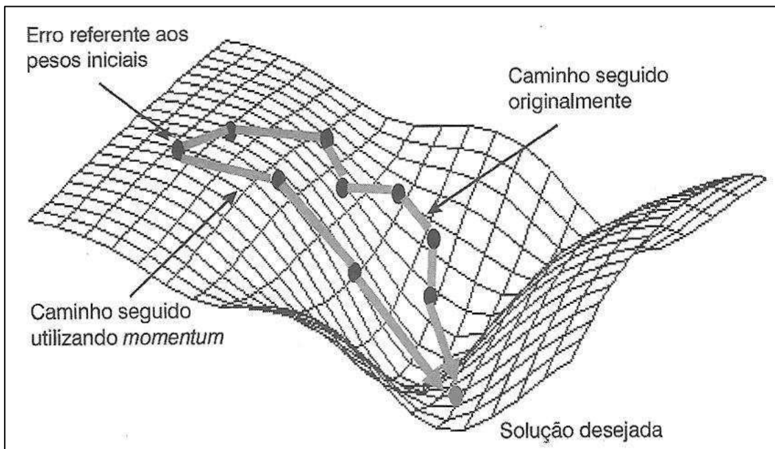
Figura 68: Influência do termo momentum (BRAGA, 2007).
