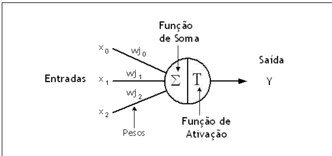
Figura 60: Estrutura do neurônio artificial MCP de McCulloch e Pitts
