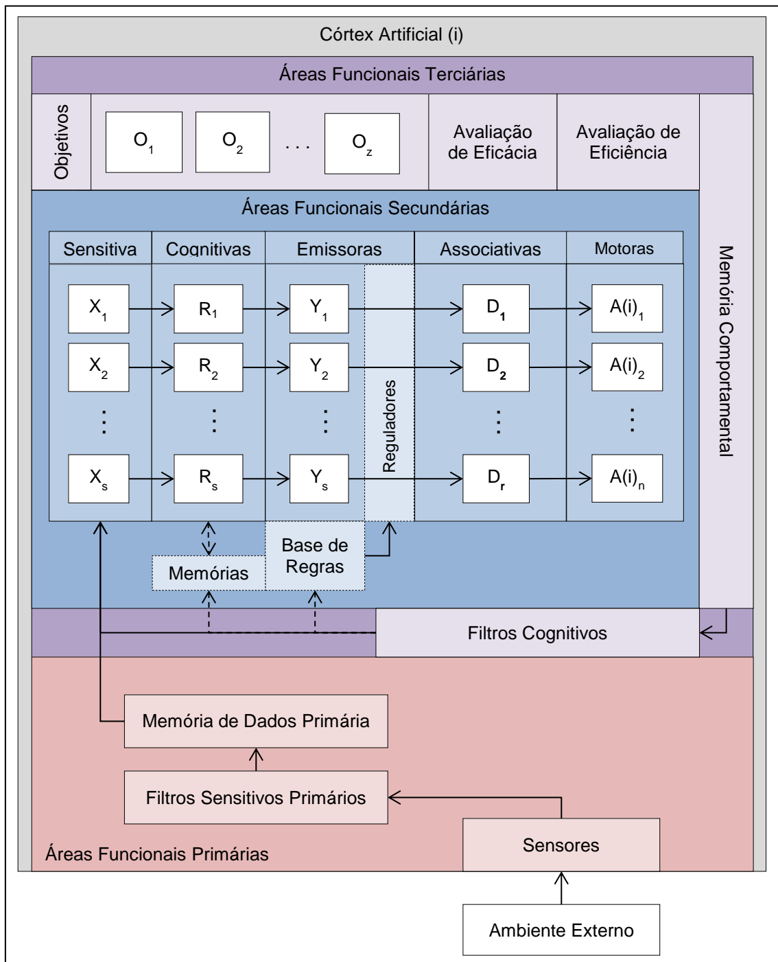
Figura 94: Estrutura do modelo conceitual de aprendizagem de máquina proposto, "Córtex Artificial".
