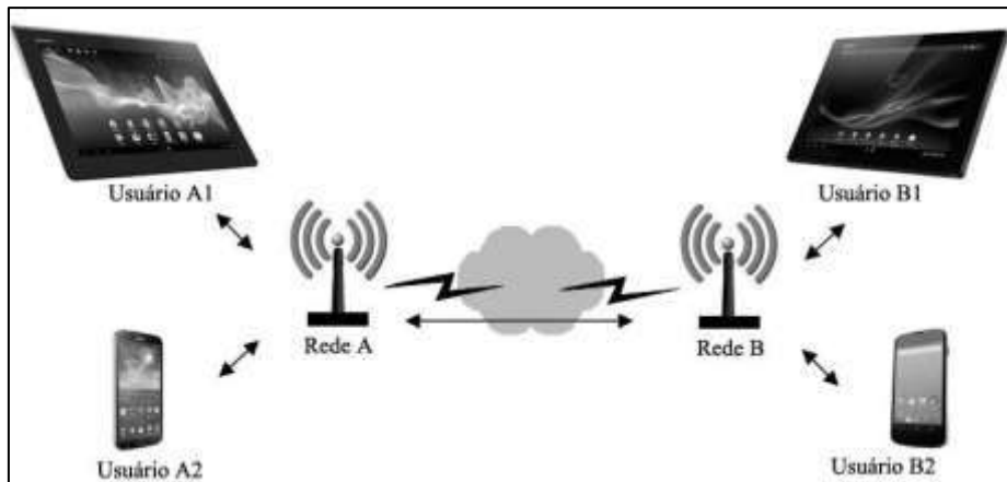
Figura 41: Comunicação Síncrona
