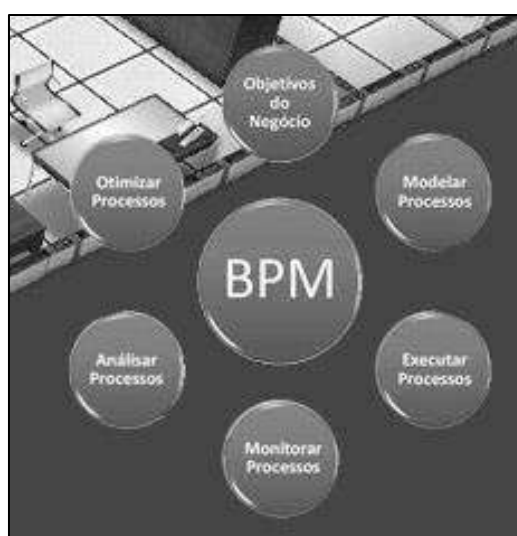
Figura 117: Objeto BPM.
