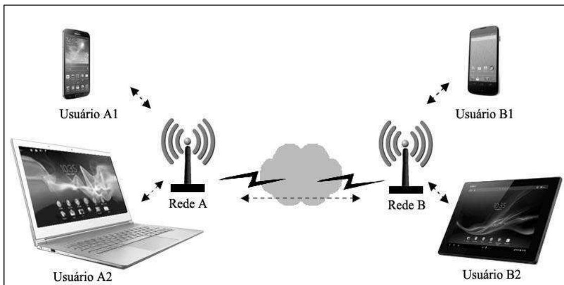
Figura 42: Interação Assíncrona
