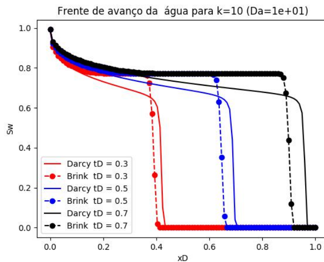
Figura 12: Solução de Brinkman diferente de Darcy ( Da alto).
