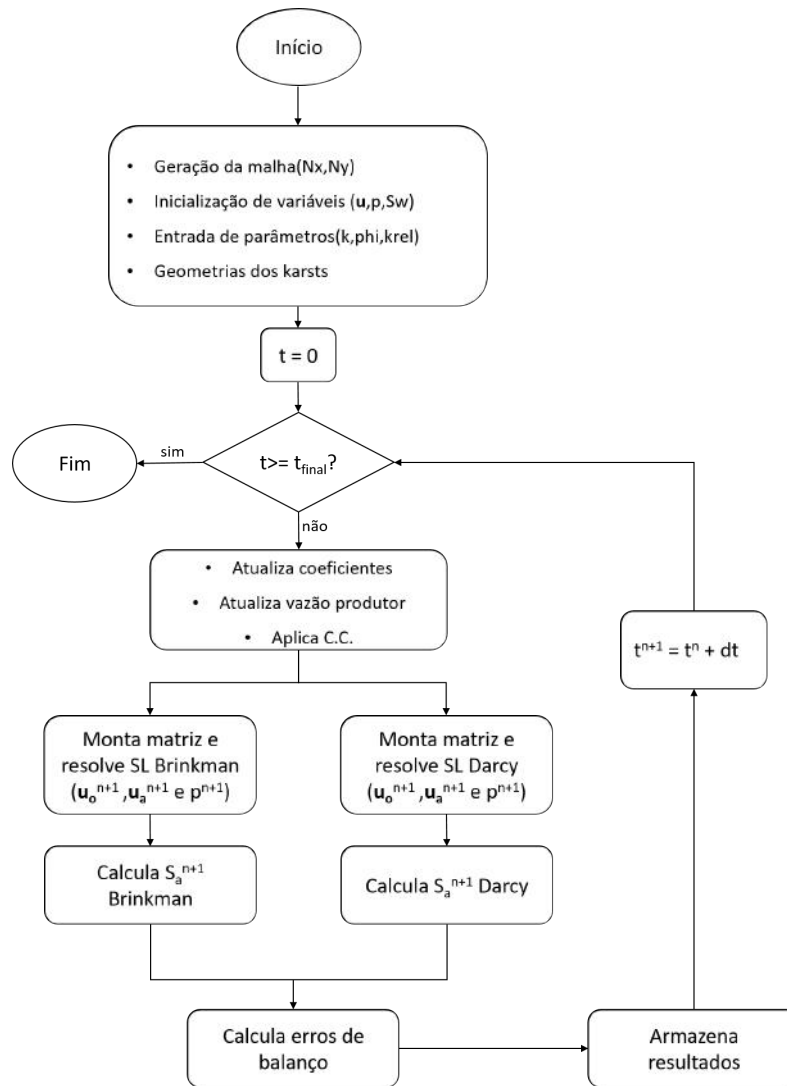
Figura 3: Estrutura resumida do programa
