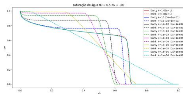
Figura 16: Análise de sensibilidade na permeabilidade absoluta ( N_x = 100 )
