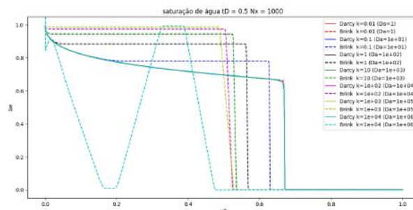
Figura 17: Análise de sensibilidade na permeabilidade absoluta com maior refinamento ( N_x = 1000 )
