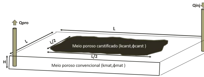
Figura 4: Esquema ilustrando modelo de reservatório
