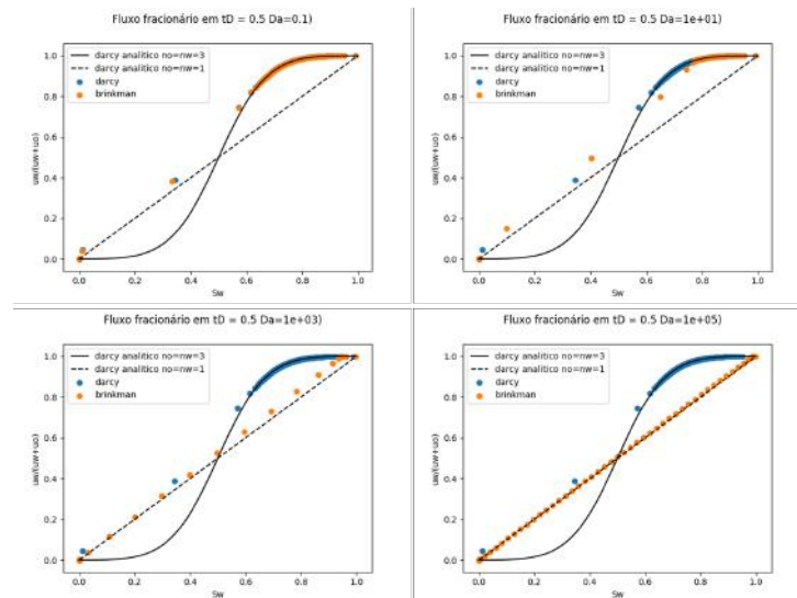
Figura 14: Análise do fluxo fracionário (a) Da = 0.1 (b) Da = 10 (c) Da = 10^3 (d) Da = 10^5
