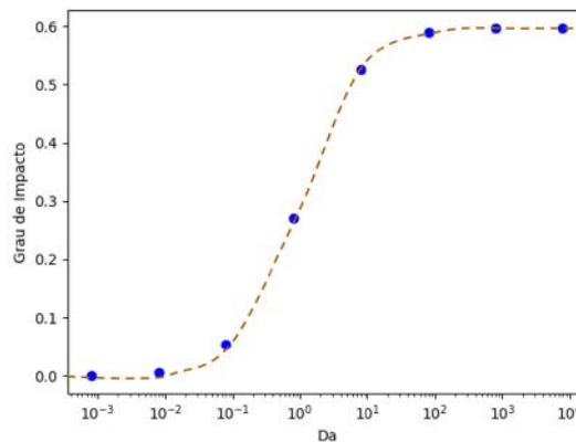
Figura 10: Grau de impacto da formulação de Brinkman
