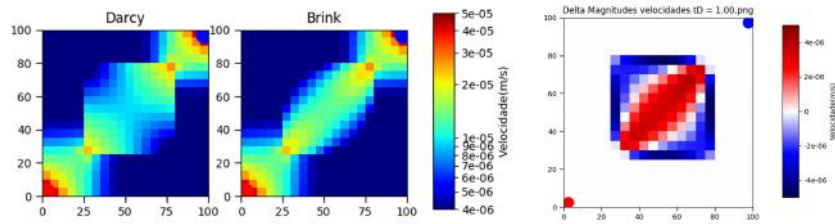
Figura 7: Magnitude velocidades (a)Darcy (b)Brinkman (c)Brinkman - Darcy
