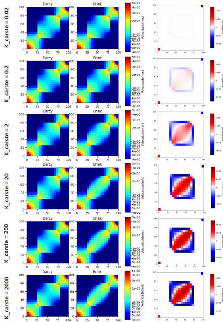
Figura 9: Sensibilidade da permeabilidade na região Carstificada
