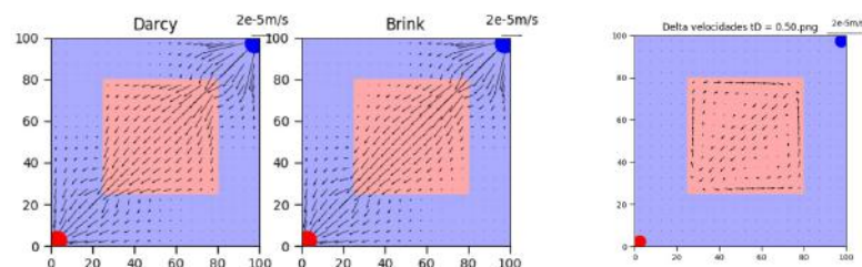
Figura 6: Campos de velocidades (a)Darcy (b)Brinkman (c)Brinkman - Darcy
