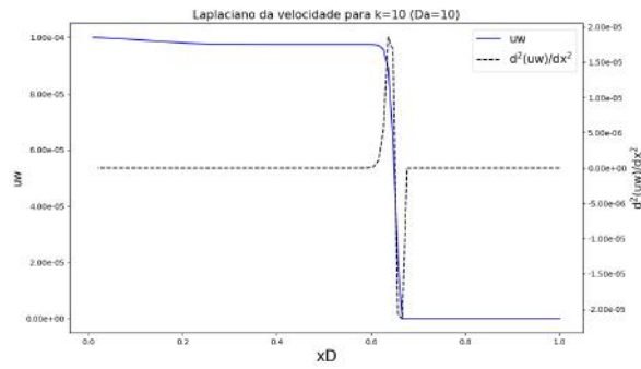
Figura 13: Análise do \nabla^2 u na frente de avanço
