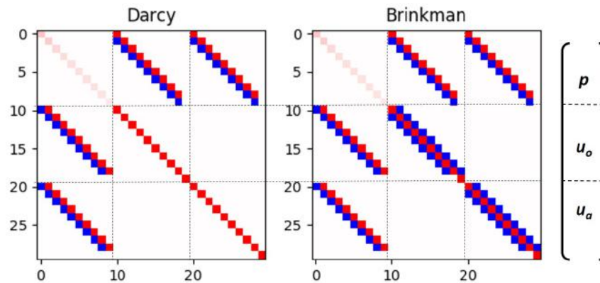
Figura 2: Matrizes bifásico 1D Nx = 10
