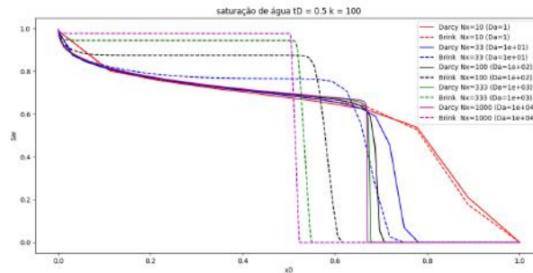
Figura 15: Análise de sensibilidade no refinamento
