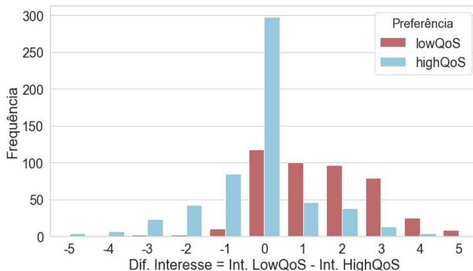
Figura 3 – Preferência pelos vídeos em função dos interesses e QoS: quando a diferença de interesse pelos vídeos é menor ou igual a 2, usuários estão dispostos a consumir conteúdo menos interessante com maior QoS.
