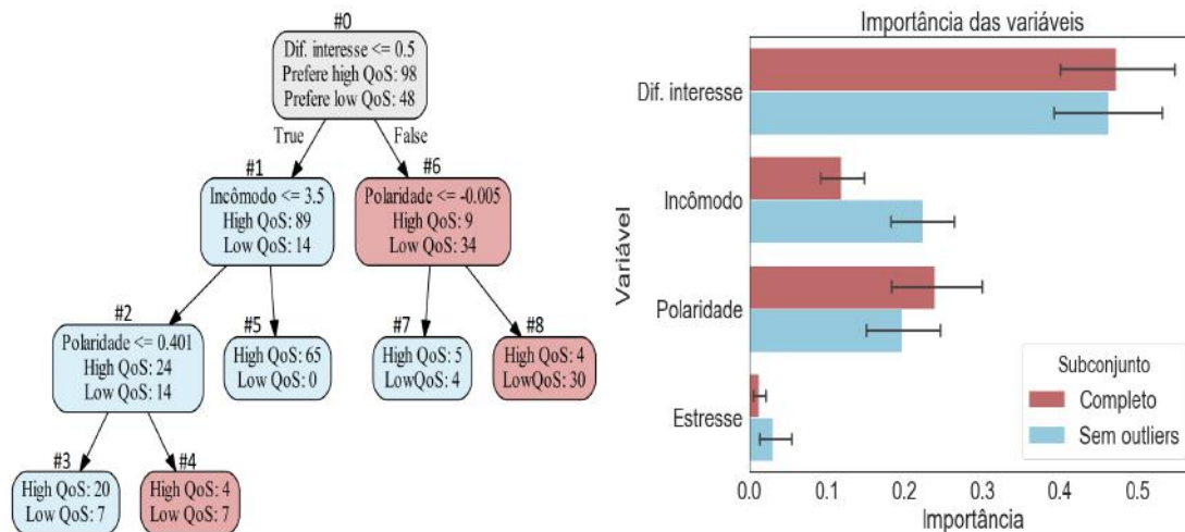
(a) Categoria música: muito sensível a QoS (b) Importância dos atributos
