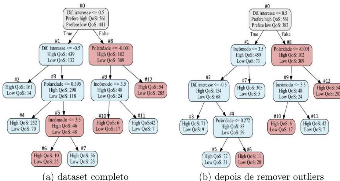
Figura 5 – Árvores de decisão que permitem interpretar as escolhas dos usuários
