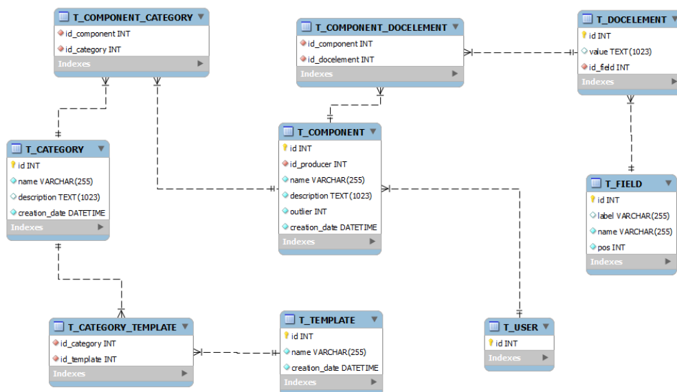
Figura 7 - Modelo Entidade-Relacionamento
