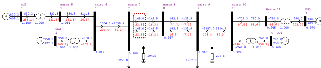
Figura 91 – G1 e G2 sobrecarregados: intercâmbio 290 MW
