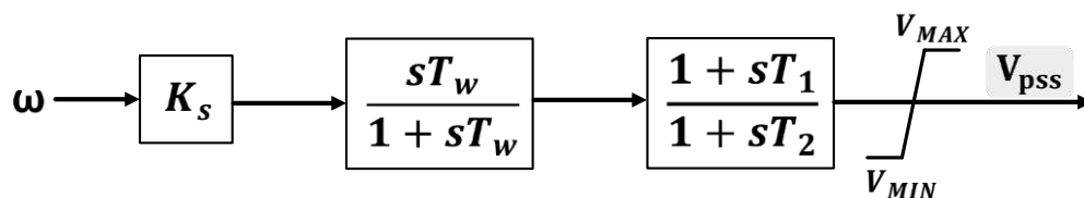
Figura 16 – Estabilizador de sistemas de potência (PSS)
