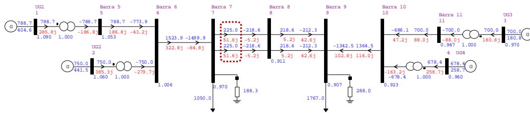
Figura 90 – G1 e G2 sobrecarregados: intercâmbio 450 MW
