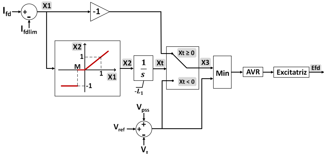
Figura 13 – Limitador de sobrecarga do tipo sobreposição ESS
