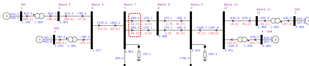
Figura 92 – G1 e G2 sobrecarregados: intercâmbio 560 MW
