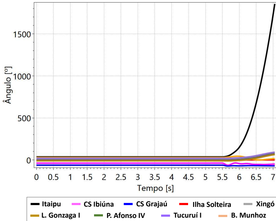
Figura 78 – Avaliação da estabilidade transitória: OEL temporizado – 5 segundos
