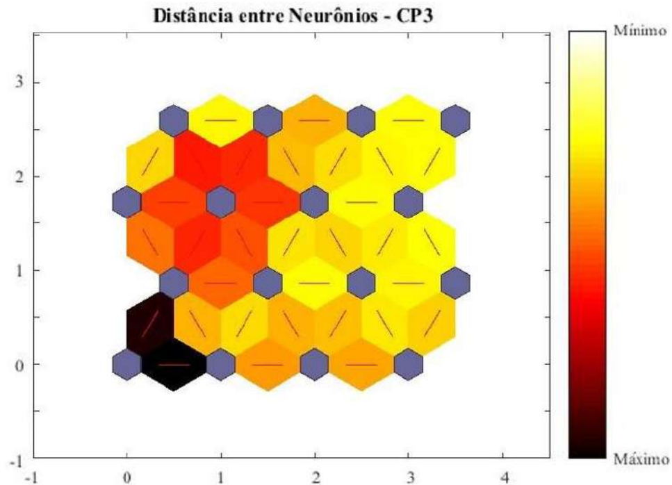
Figura 27 – Mapa de Distâncias dos Neurônios para o Ensaio CP3.
