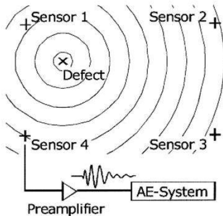
Figura 1 – Propagação de uma Emissão Acústica (MIX, 2005).
