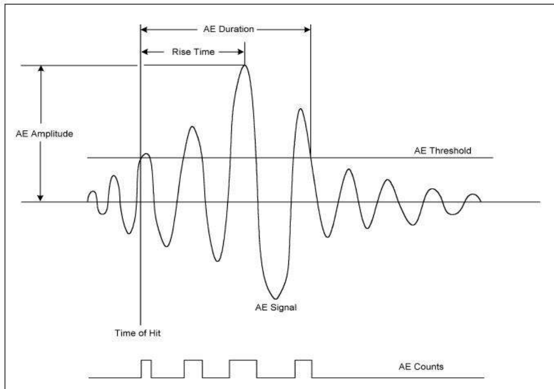
Figura 3 – Parâmetros Extraídos dos Eventos de Emissão Acústica (Physical Acoustics Corporation, 2011).
