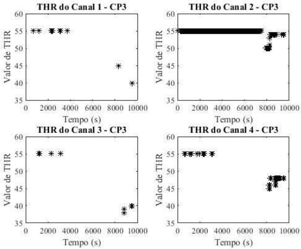
Figura 17 – Valor do Threshold (THR) ao Longo do Tempo para o Ensaio CP3.
