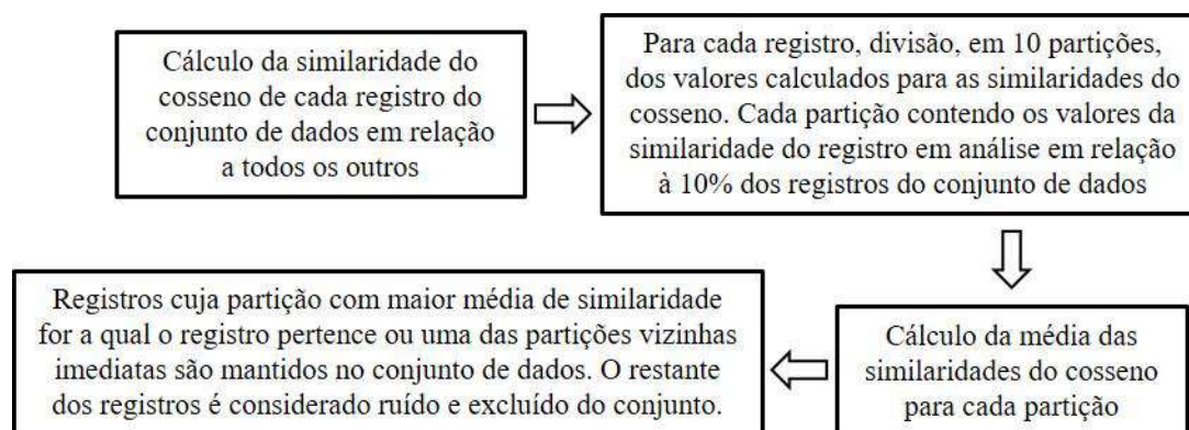
Figura 12 – Fluxograma do Passo a Passo da Limpeza através da similaridade do Cosseno.
