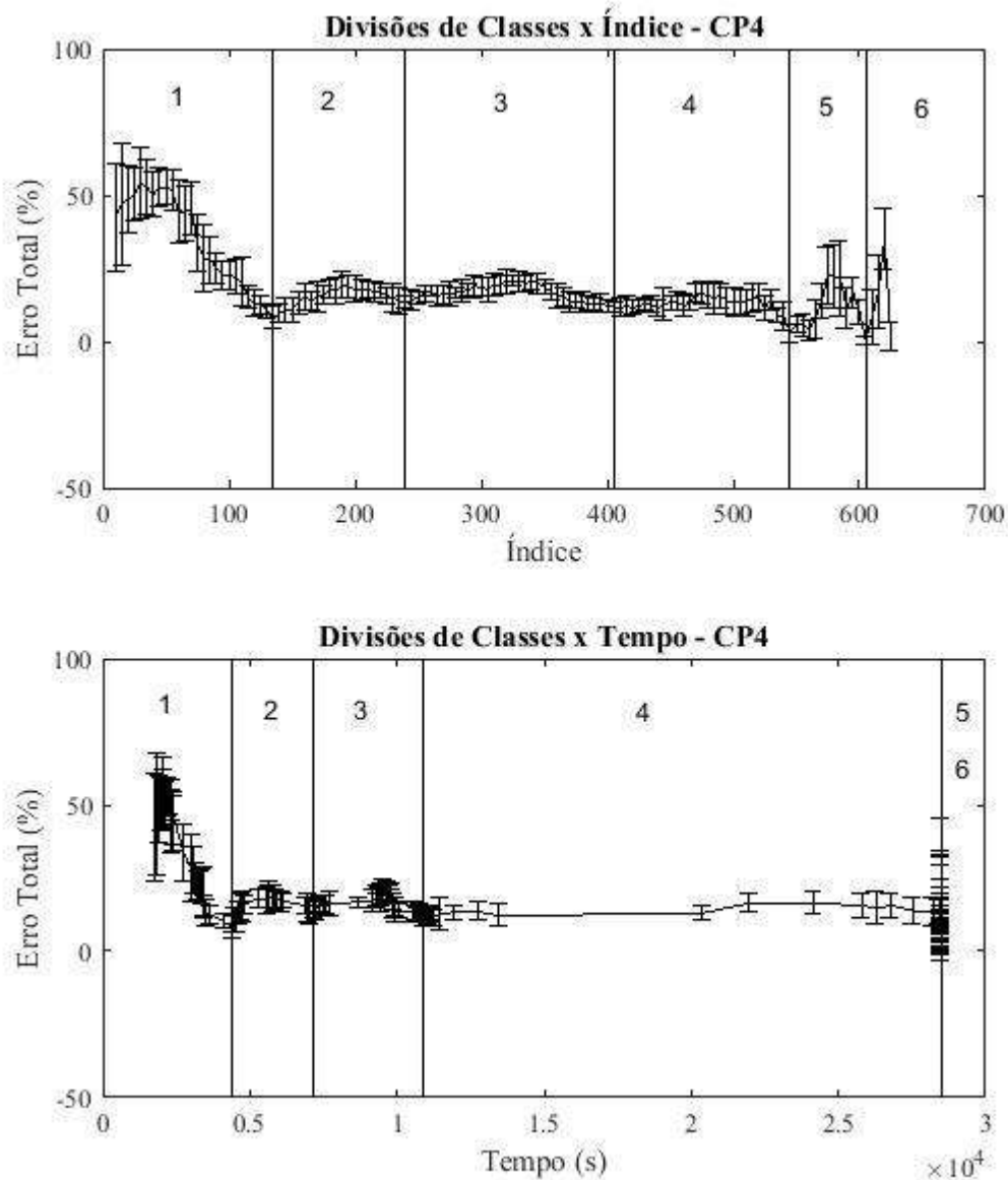
Figura 26 – Erro de Classificação por Ponto de Corte Testado para o Ensaio CP4.
