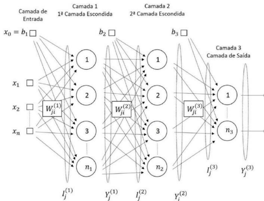
Figura 7 – Notação dos Elementos do Algoritmo Backpropagation .
