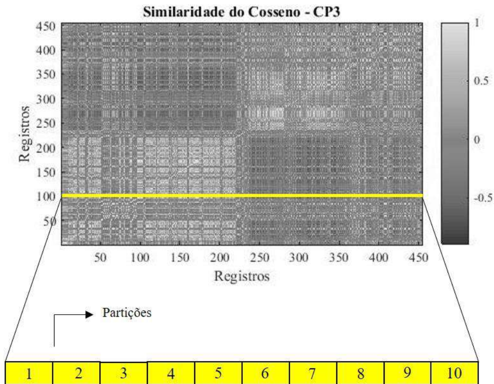
Figura 13 – Exemplo de processo de limpeza dos registros utilizando similaridade do cosseno.
