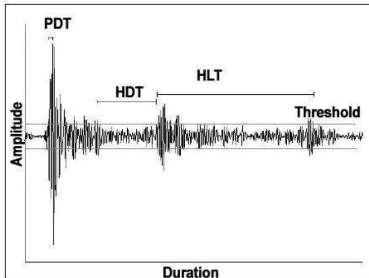
Figura 2 – Parâmetros de Tempo para a Detecção de Eventos de Emissão Acústica (Jacques, 2009).
