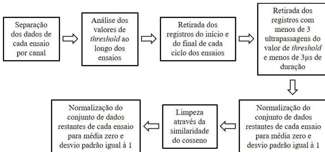
Figura 11 – Fluxograma do Passo a Passo do Pré-Processamento dos Dados de Cada Ensaio.
