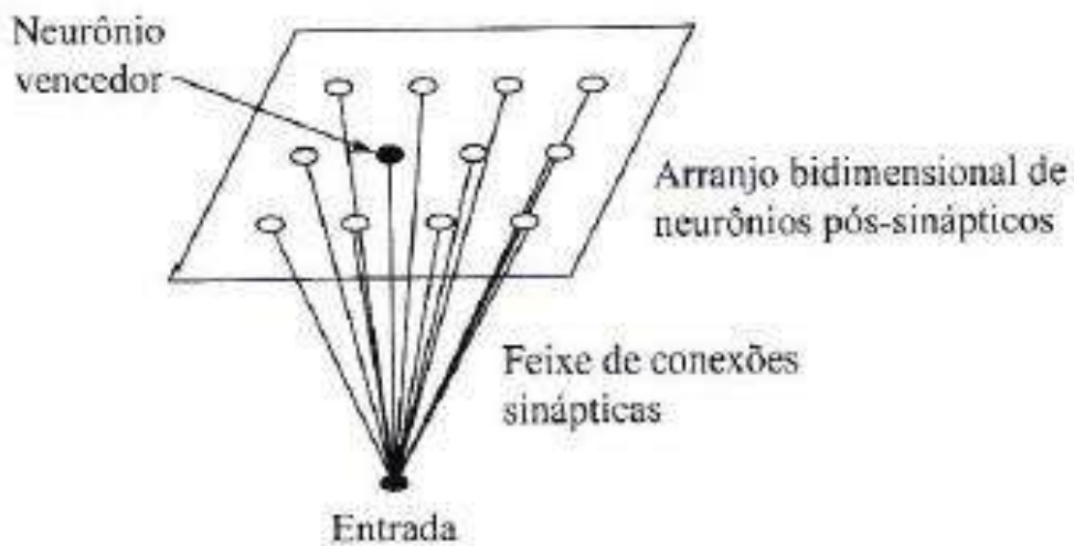
Figura 8 – Mapa Auto-Organizável de Kohonen (HAYKIN, 2001).
