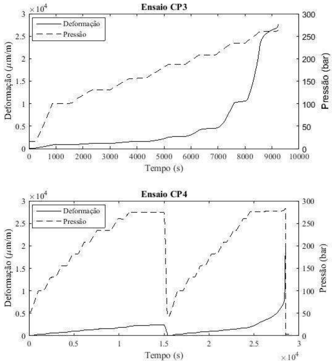
Figura 9 – Gráficos da Pressão e da Deformação ao Longo do Tempo dos Testes
