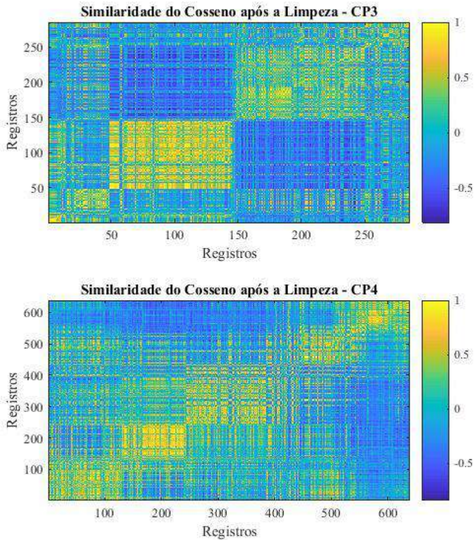
Figura 24 – Data Image da Similaridade do Cosseno dos Dados de CP3 e CP4 após Limpeza.
