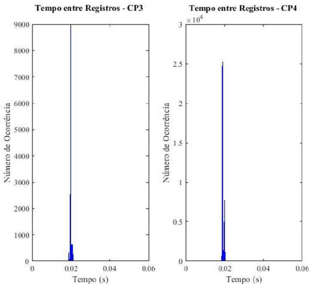
Figura 19 – Histograma de Intervalo de Tempo entre Sinais Consecutivos Captados.
