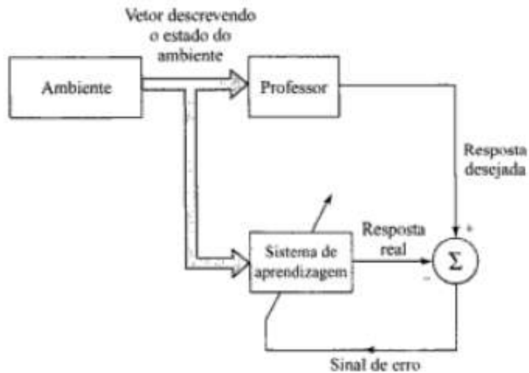
Figura 4 – Representação da Aprendizagem Supervisionada (HAYKIN, 2001).
