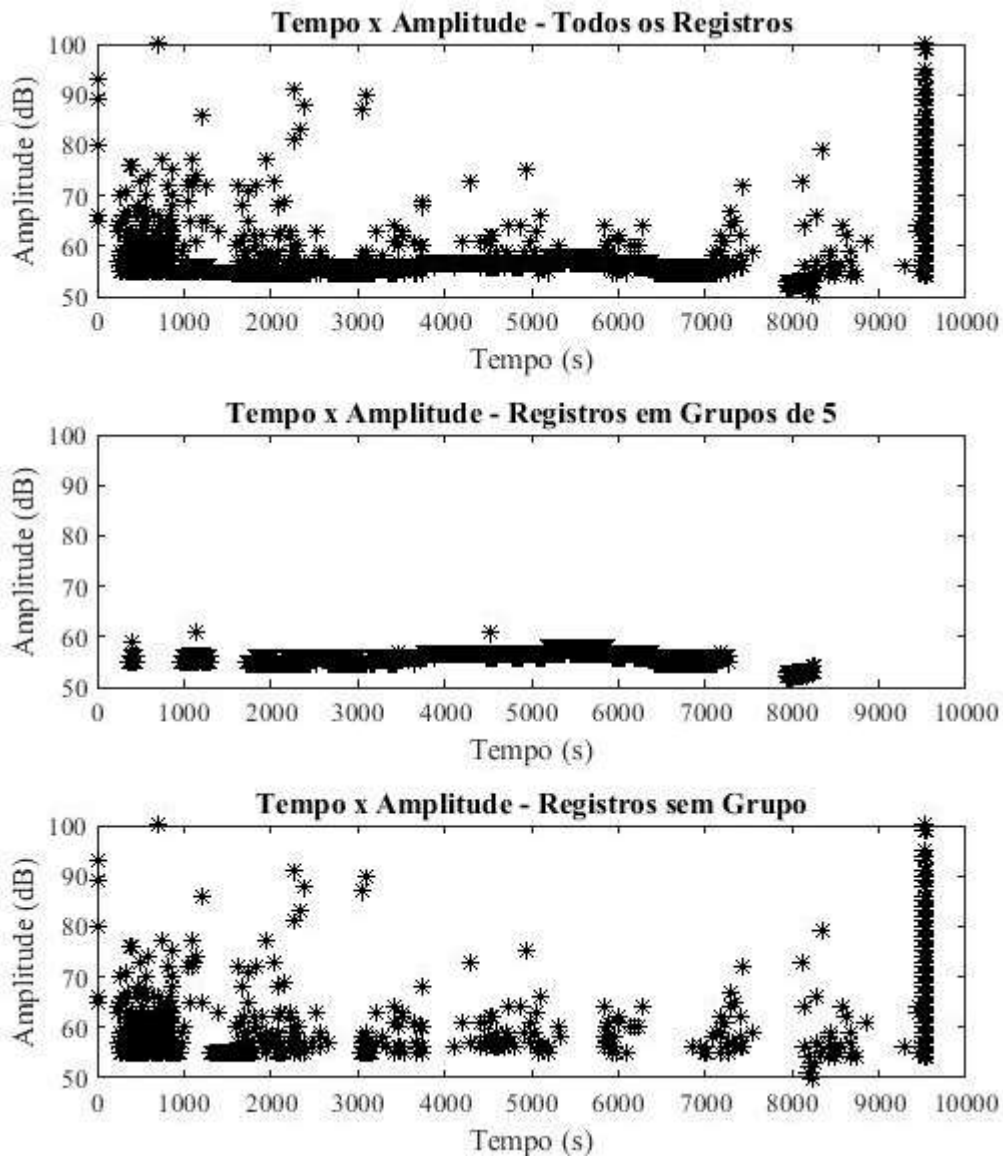
Figura 21 – Amplitudes dos Registros do Ensaio CP3 - Canal 2.
