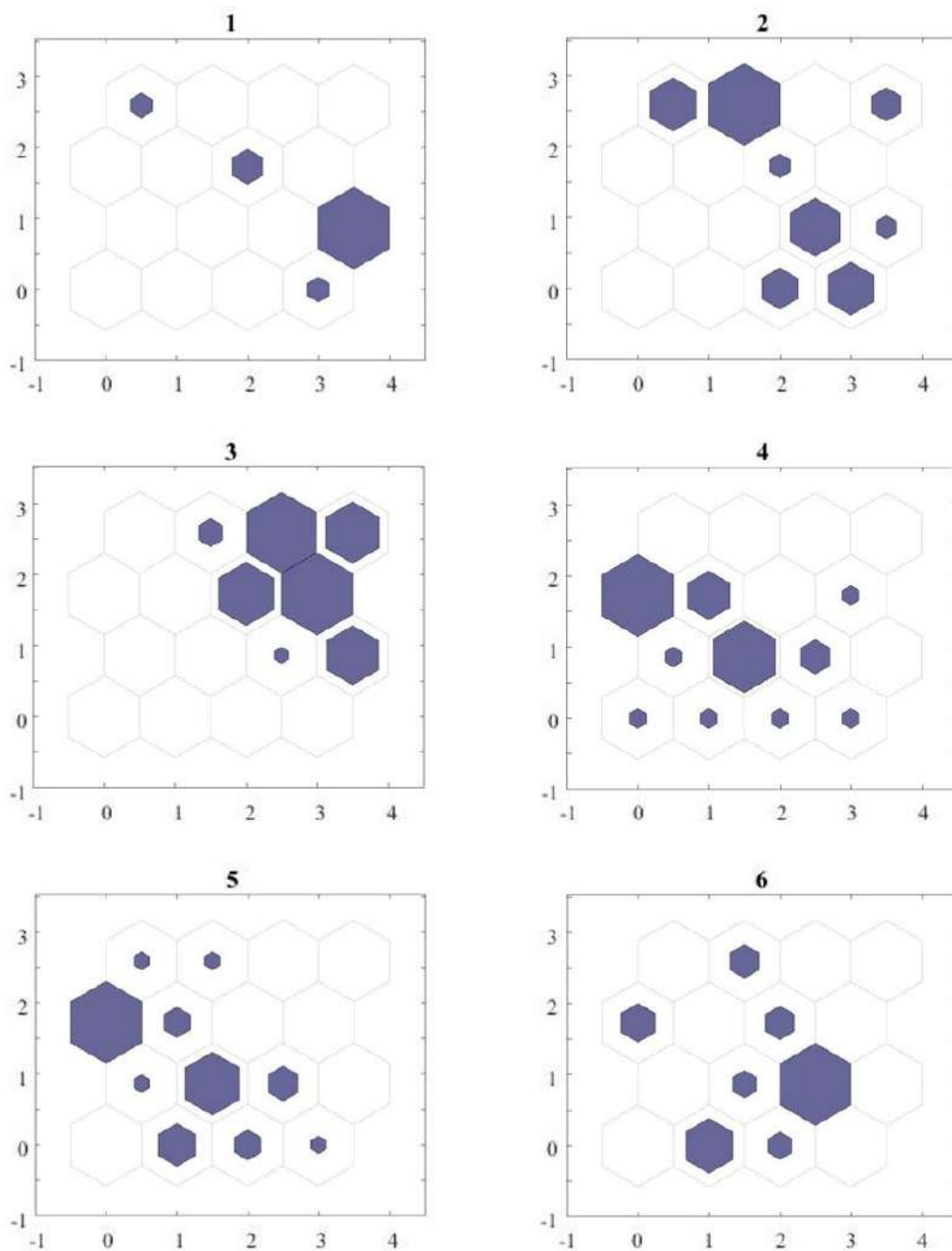
Figura 28 – Mapa de Ativação dos Neurônios para o Ensaio CP3.
