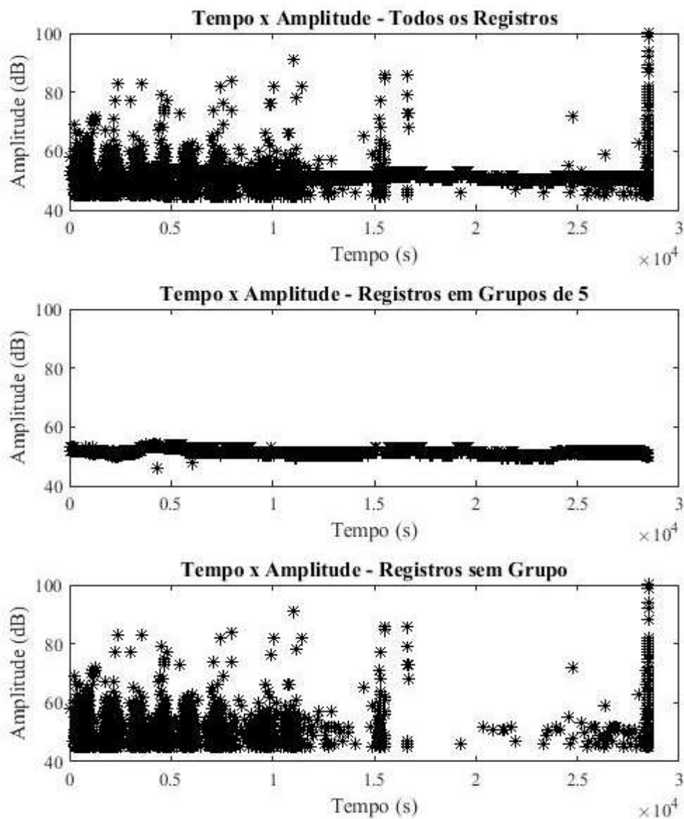
Figura 22 – Amplitudes dos Registros do Ensaio CP4 - Canal 2.
