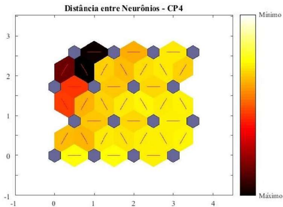
Figura 29 – Mapa de Distâncias dos Neurônios para o Ensaio CP4.
