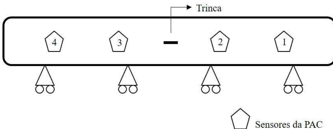
Figura 10 – Posicionamento dos sensores ao longo do duto.
