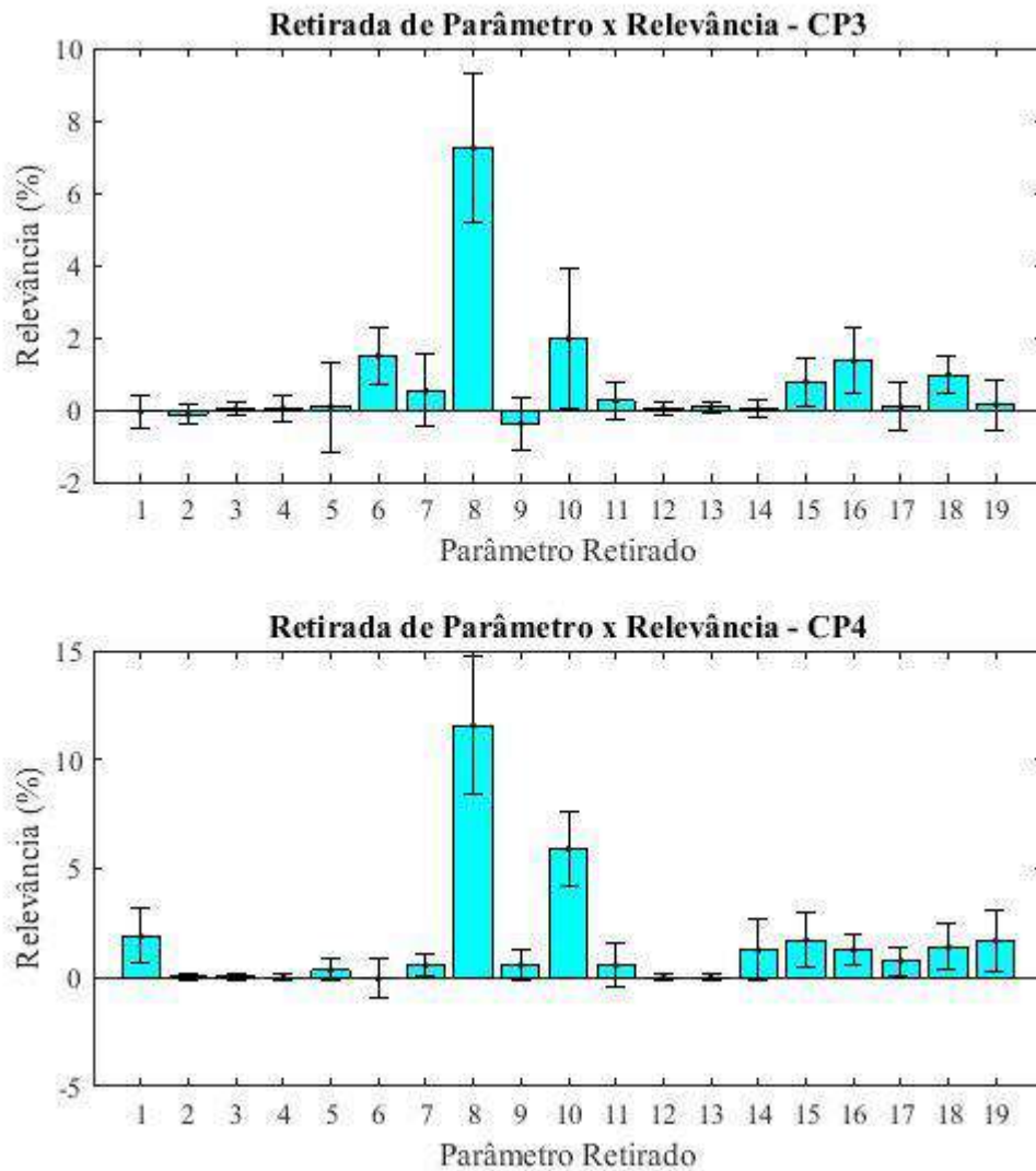
Figura 31 – Relevância dos Parâmetros para as Redes Treinadas.
