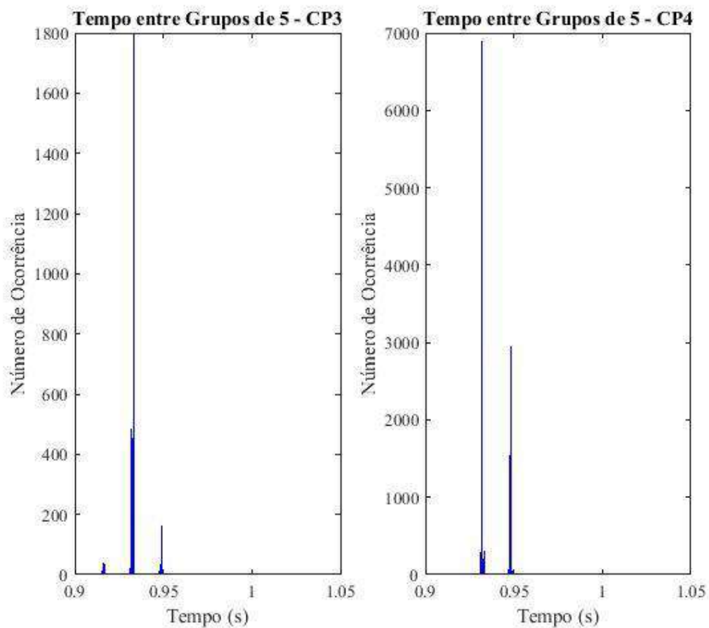
Figura 20 – Histograma do Intervalo de Tempo entre os Grupos de 5 Sinais.
