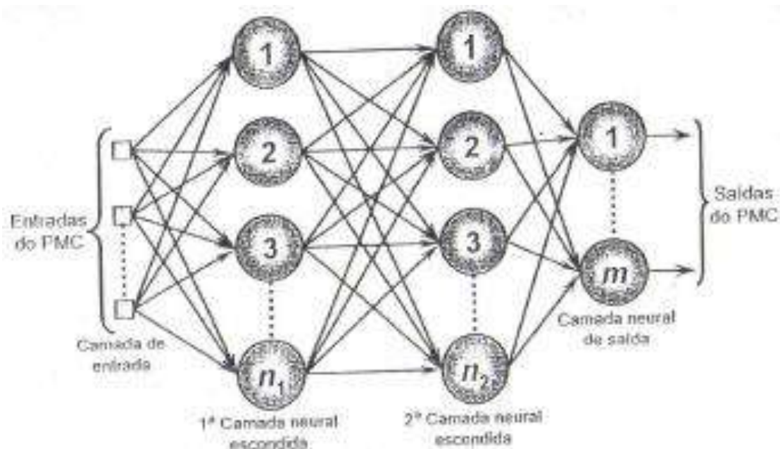
Figura 6 – Representação da Rede Perceptron Multicamadas (Da SILVA et al. , 2010).
