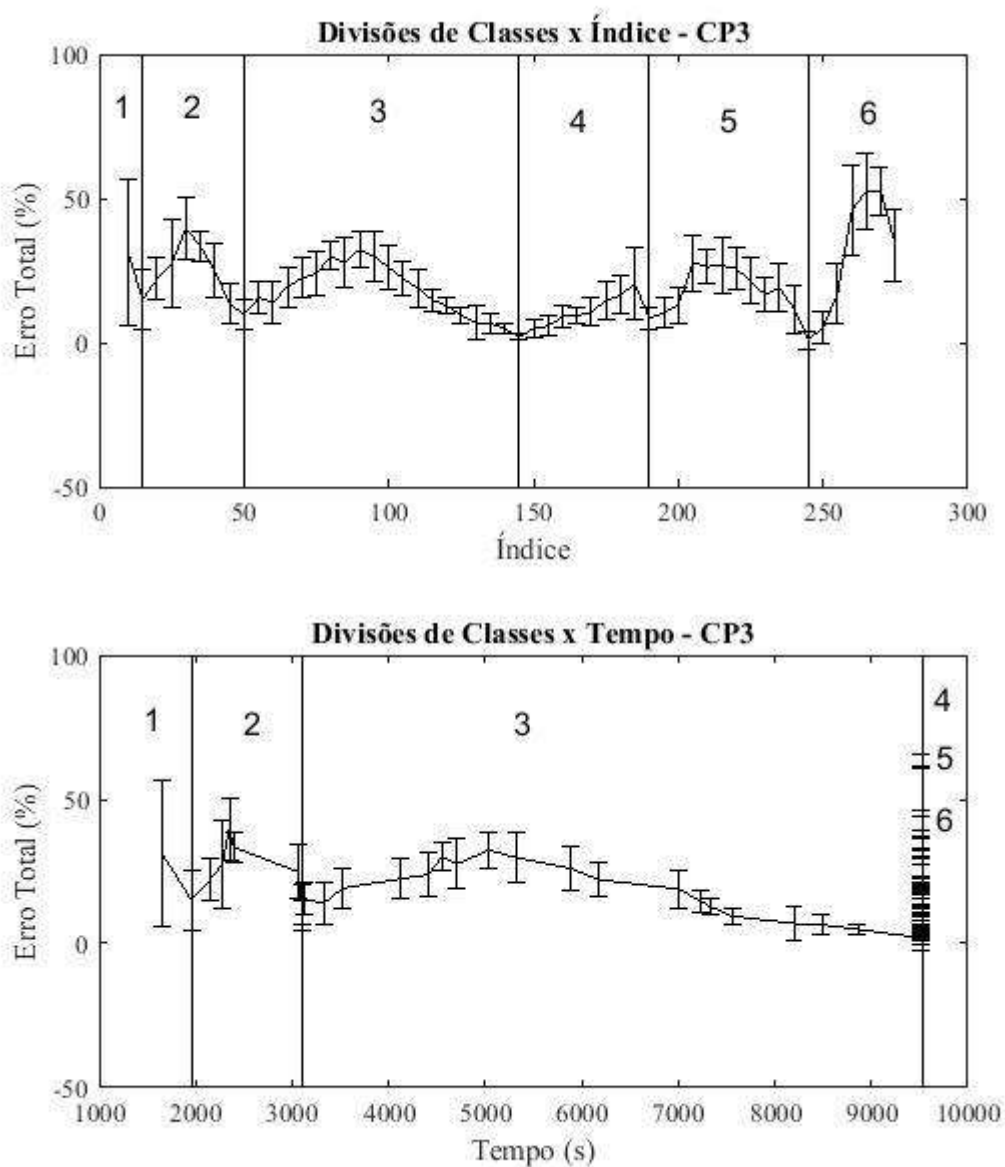
Figura 25 – Erro de Classificação por Ponto de Corte Testado para o Ensaio CP3.
