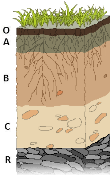
Figura 2.8 Horizontes típicos de um solo bem desenvolvido
