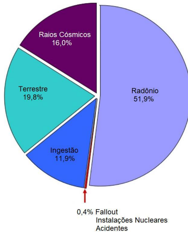
Figura 1.1 Contribui33o da dose de radia33o natural em seres humanos de acordo com a sua origem (adaptado de UNSCEAR, 2008)
