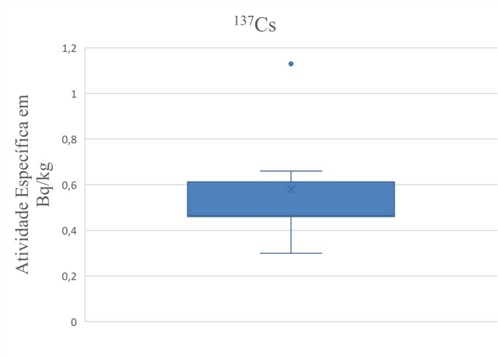
Figura 4.4 O diagrama boxplot com a variação de concentração de ^{137}\text{Cs}
