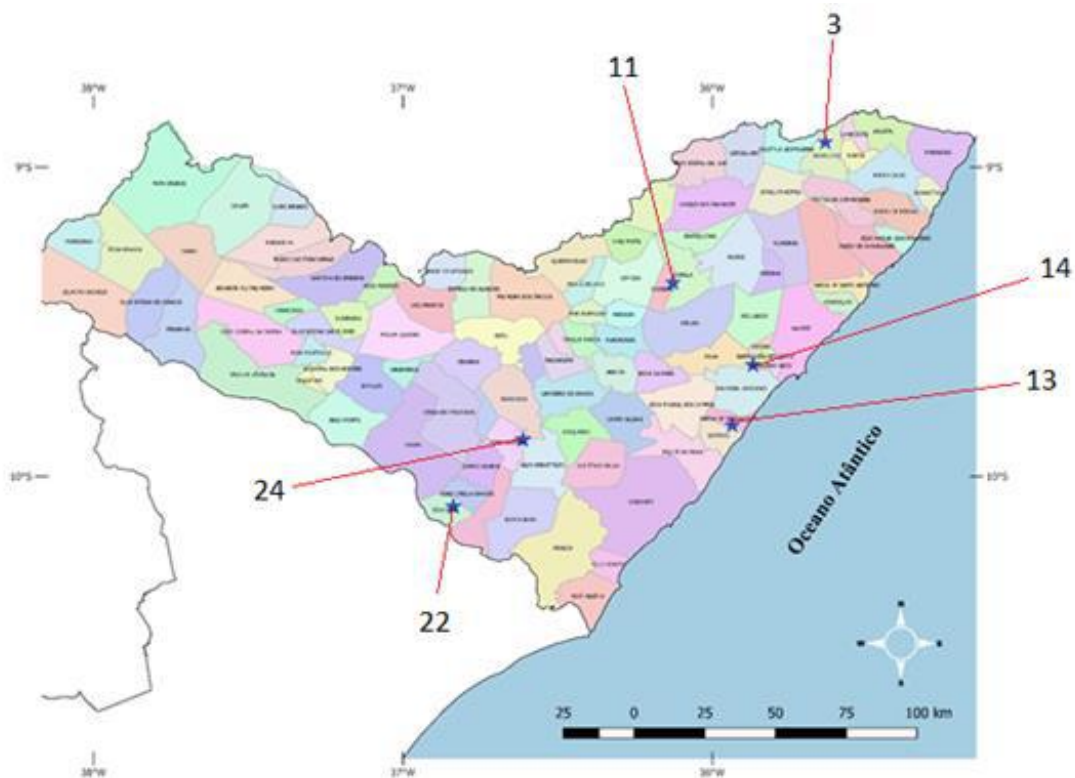
Figura 4.19 Localização das amostras de ^{137}\text{Cs} com concentração acima da AMD
