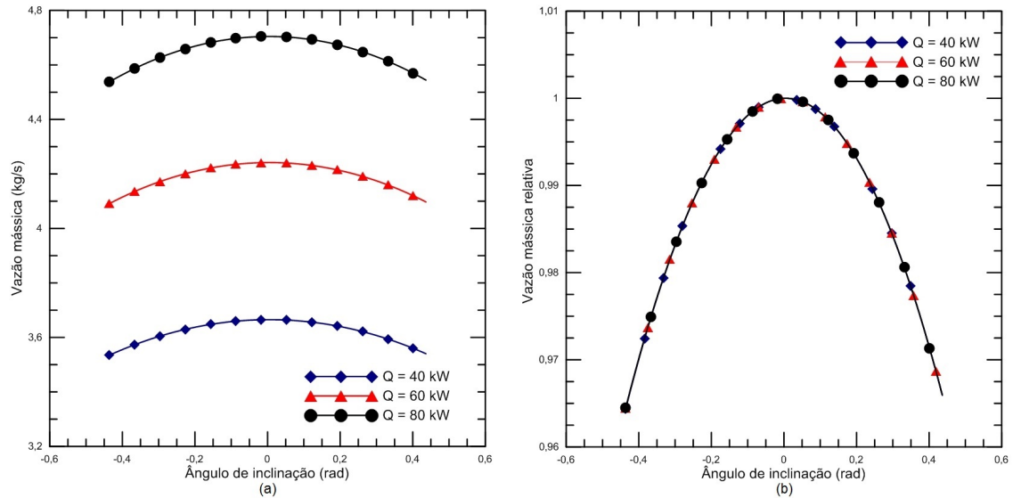
Figura 4.1: (a) Vazão mássica em função do ângulo de inclinação quando a potência é igual a 40 kW, 60 kW ou 80 kW; (b) Vazão mássica relativa à vazão mássica inicial em função do ângulo de inclinação quando a potência é igual a 40 kW, 60 kW ou 80 kW.
