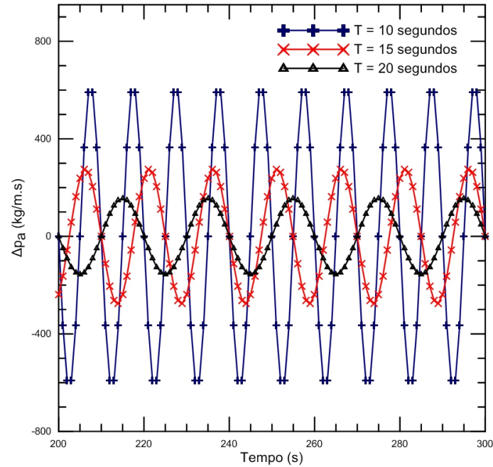
Figura 4.15: Queda de pressão total devido às acelerações adicionais em função do tempo quando a amplitude do movimento de balanço é igual a 10^\circ .
