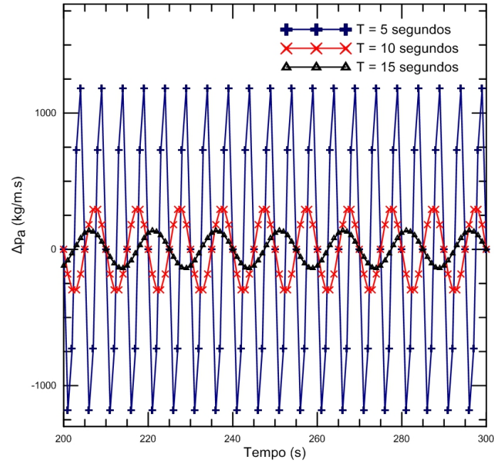
Figura 4.14: Queda de pressão total devido às acelerações adicionais em função do tempo quando a amplitude do movimento de balanço é igual a 5^\circ .
