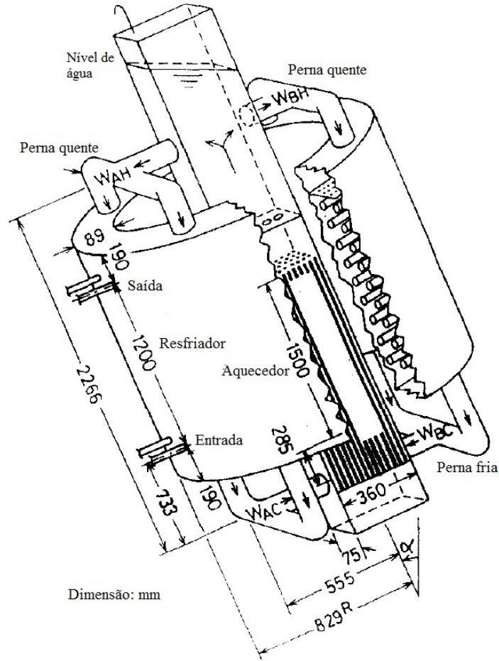
Figura 2.1: Aparato experimental utilizado por IYORI et al. [21].
