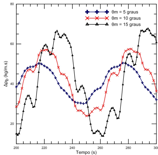
Figura 4.13: Queda de pressão total devido ao empuxo em função do tempo quando o período é igual a 12 segundos.
