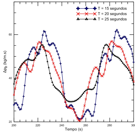
Figura 4.12: Queda de pressão total devido ao empuxo em função do tempo quando a amplitude do movimento de balanço é igual a 15^\circ .
