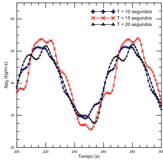
Figura 4.11: Queda de pressão total devido ao empuxo em função do tempo quando a amplitude do movimento de balanço é igual a 10^\circ .
