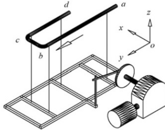
Figura 2.6: Aparato experimental utilizado por ZHANG et al. [32].
