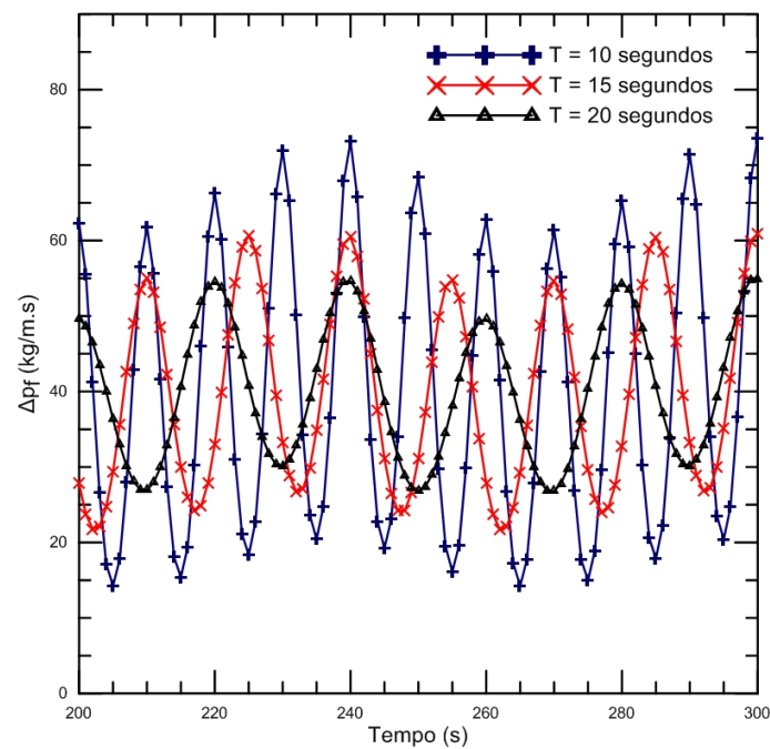
Figura 4.19: Queda de pressão total devido ao atrito em função do tempo quando a amplitude do movimento de balanço é igual a 10^\circ .
