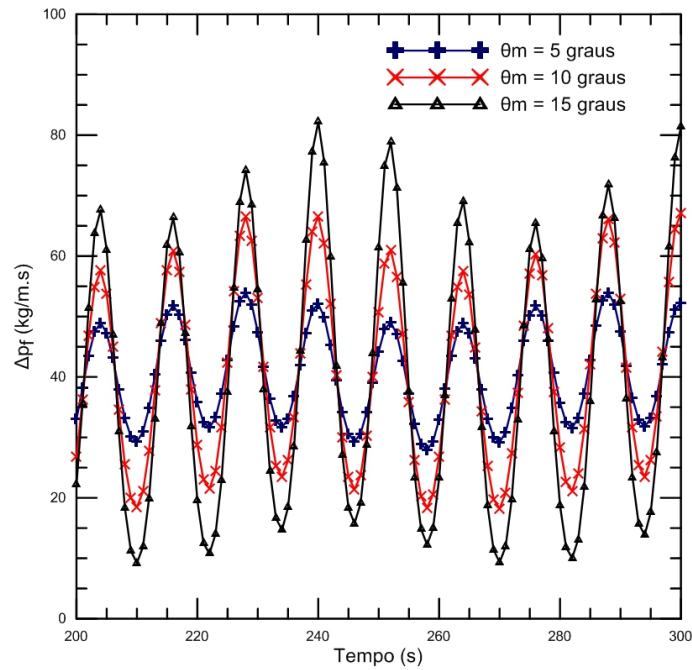
Figura 4.21: Queda de pressão total devido ao atrito em função do tempo quando o período do movimento de balanço é igual a 12 segundos.
