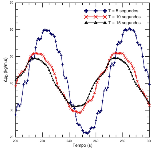
Figura 4.10: Queda de pressão total devido ao empuxo em função do tempo quando a amplitude do movimento de balanço é igual a 5^\circ .
