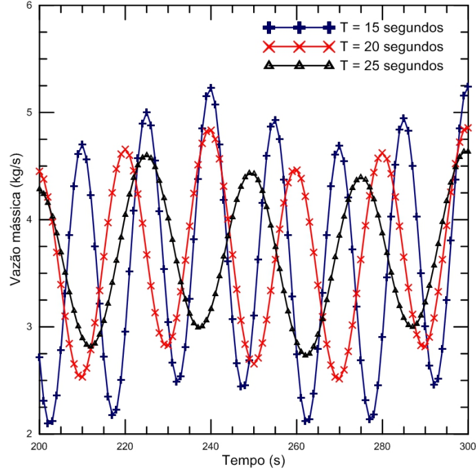
Figura 4.6: Vazão mássica em função do tempo quando a amplitude do movimento de balanço é igual a 15^\circ .
