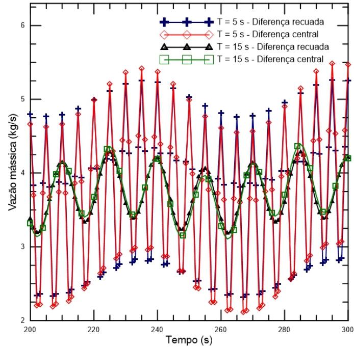
Figura 4.8: Vazão mássica em função do tempo quando a amplitude do movimento de balanço é igual a 5^\circ , utilizando diferença finita recuada e central.
