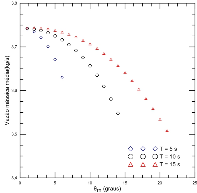
Figura 4.22: Vazão mássica média em função da amplitude.
