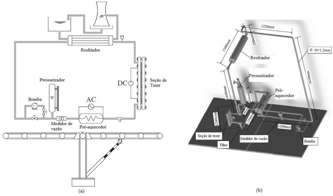
Figura 2.5: (a)Plataforma experimental; (b) Aparato experimental utilizado por TIAN et al. [31].
