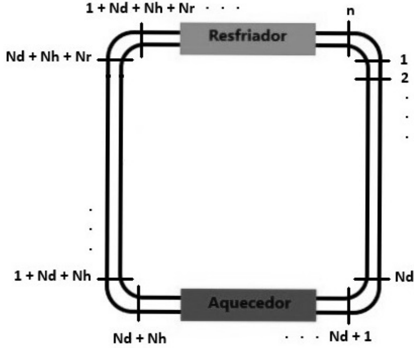
Figura 3.3: Discretização espacial ao longo do circuito.
