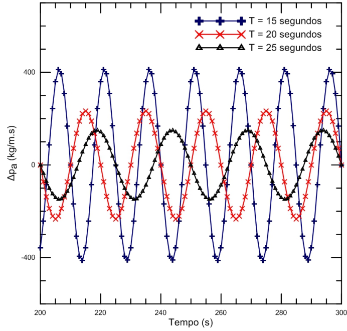
Figura 4.16: Queda de pressão total devido às acelerações adicionais em função do tempo quando a amplitude do movimento de balanço é igual a 15^\circ .
