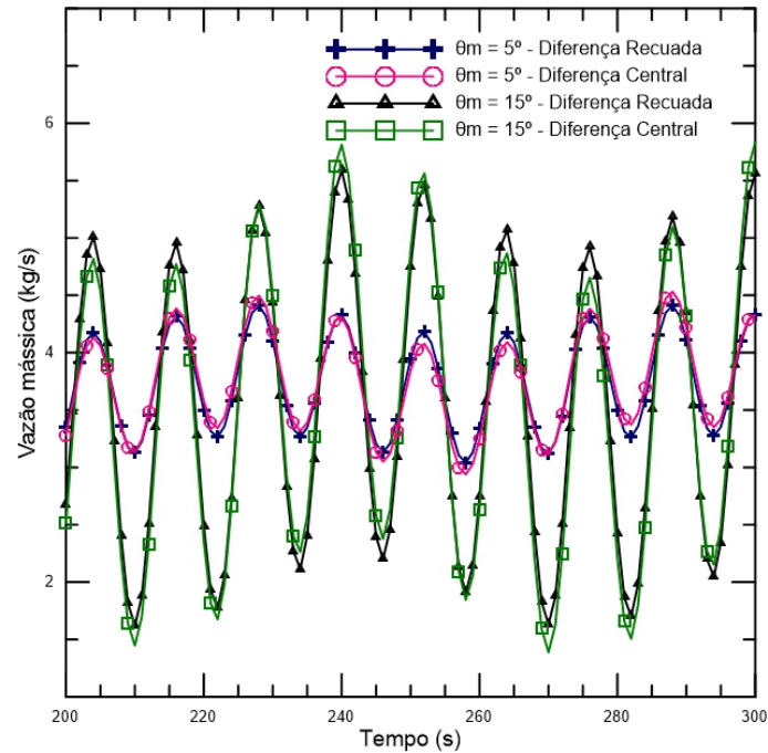
Figura 4.9: Vazão mássica em função do tempo quando o período do movimento de balanço é igual a 12 segundos, utilizando diferença finita recuada e central.
