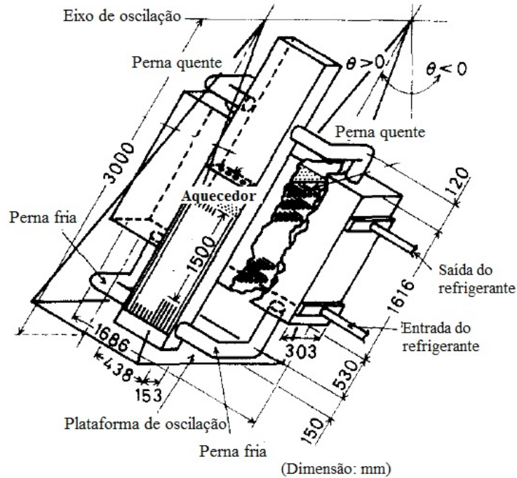
Figura 2.3: Aparato experimental utilizado por MURATA et al. [25].
