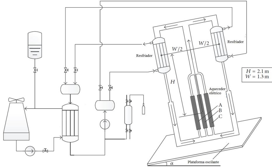
Figura 2.2: Aparato experimental utilizado por ZHU et al. [22] e YANG et al. [23].
