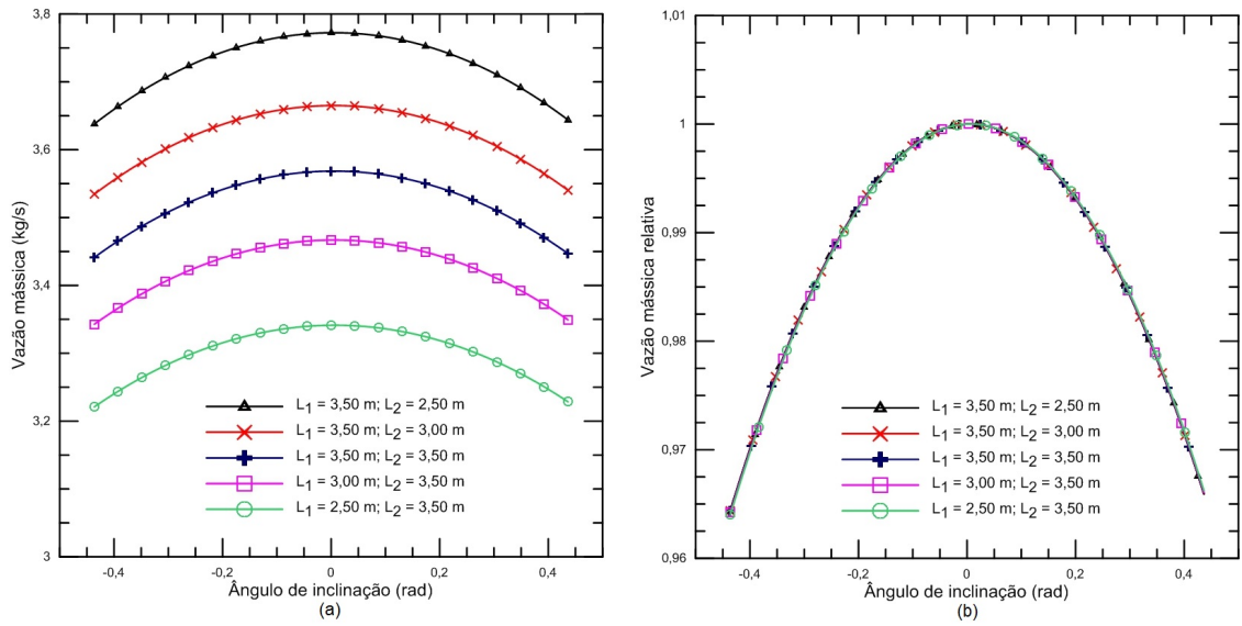
Figura 4.3: (a)Vazão mássica em função do ângulo de inclinação para diversos tamanhos do circuito; (b)Vazão mássica relativa à vazão mássica inicial em função do ângulo de inclinação para diversos tamanhos do circuito.
