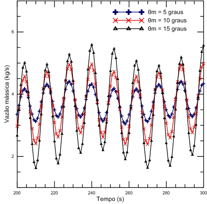
Figura 4.7: Vazão mássica em função do tempo quando o período do movimento de balanço é igual a 12 segundos.
