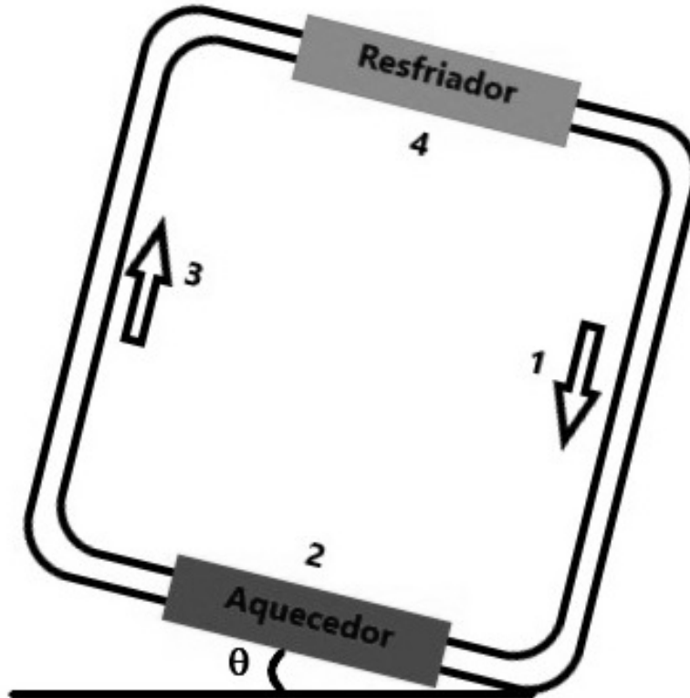
Figura 3.1: Circuito retangular de circulação natural.
