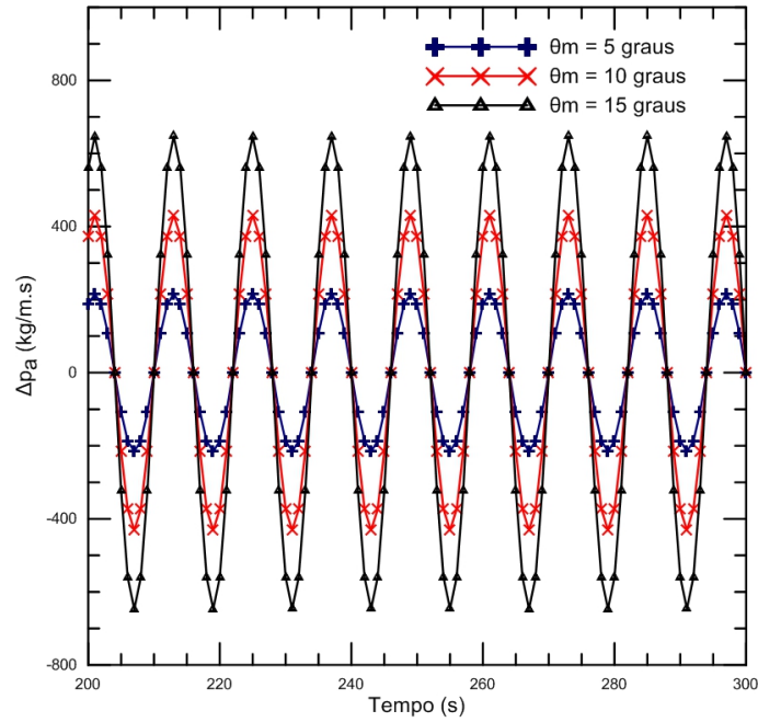
Figura 4.17: Queda de pressão total devido às acelerações adicionais em função do tempo quando o período do movimento de balanço é igual a 12 segundos.
