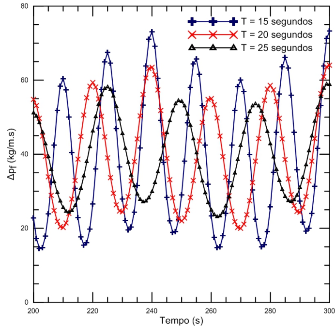
Figura 4.20: Queda de pressão total devido ao atrito em função do tempo quando a amplitude do movimento de balanço é igual a 15^\circ .
