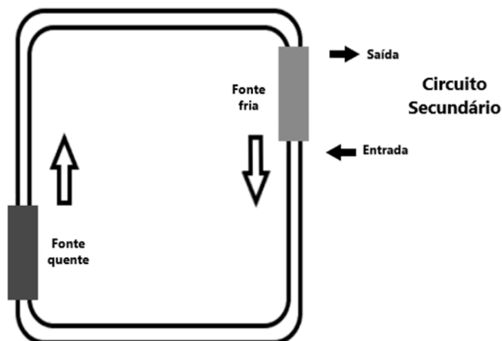
Figura 1.2: Circuito de Circulação Natural.
