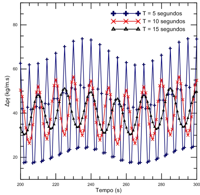
Figura 4.18: Queda de pressão total devido ao atrito em função do tempo quando a amplitude do movimento de balanço é igual a 5^\circ .
