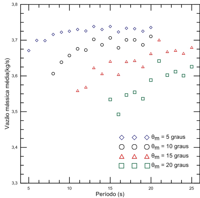
Figura 4.23: Vazão mássica média em função do período.
