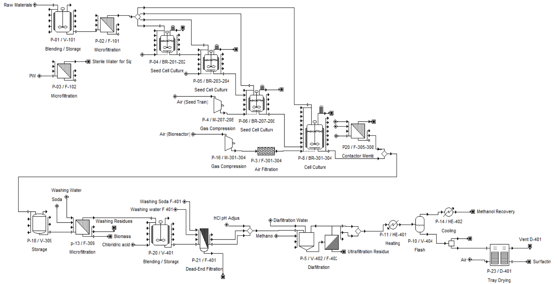
Figura 30: Layout do processo do cenário 4 e principais equipamentos simulado no SPD
