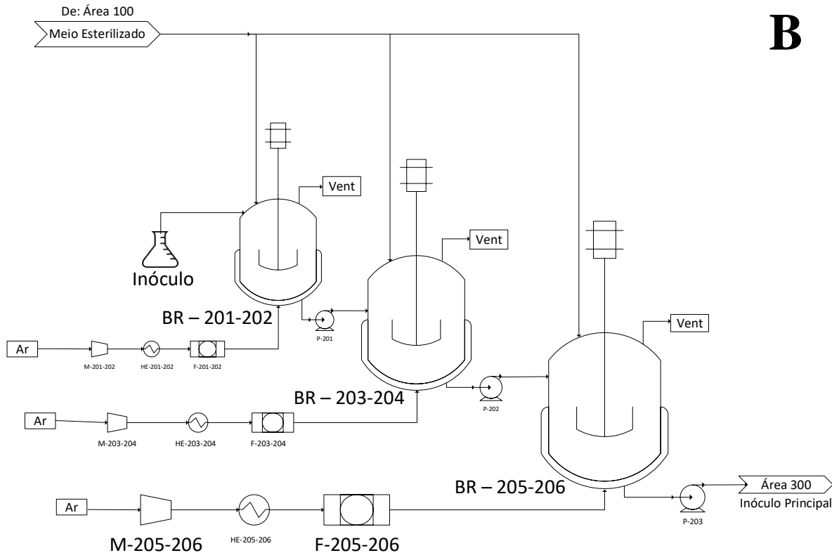
Figura 8: Fluxogramas de processos: áreas 100 (A) e 200 (B)
