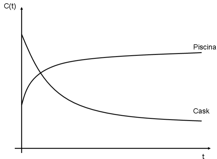
Figura 14 - Esboço do comportamento das duas parcelas do custo que são função do tempo de armazenamento inicial
