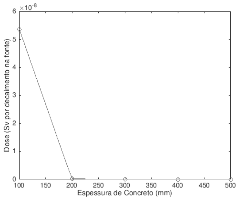
Figura 27 - Dose medida no detector por decaimento na fonte em função da espessura de concreto do cask
