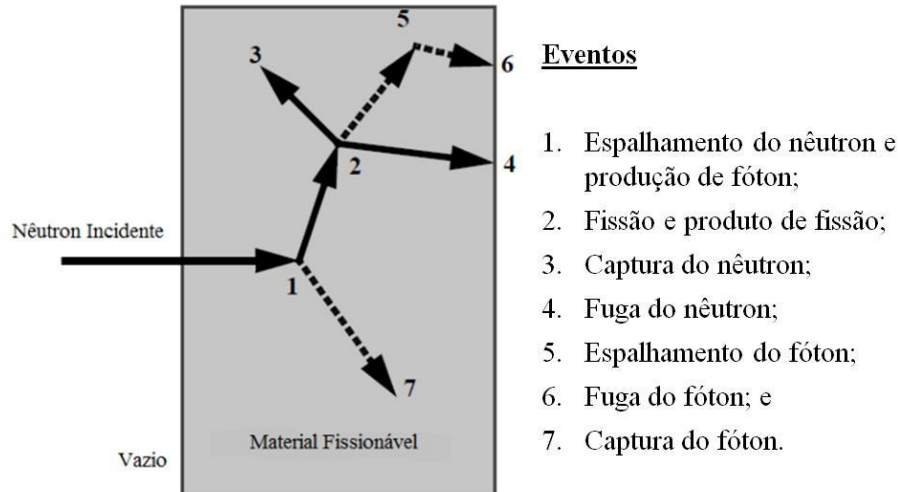
Figura 8 - História no MCNP de um nêutron incidente em um material (adaptado de X-5 MONTE CARLO TEAM, 2003)
