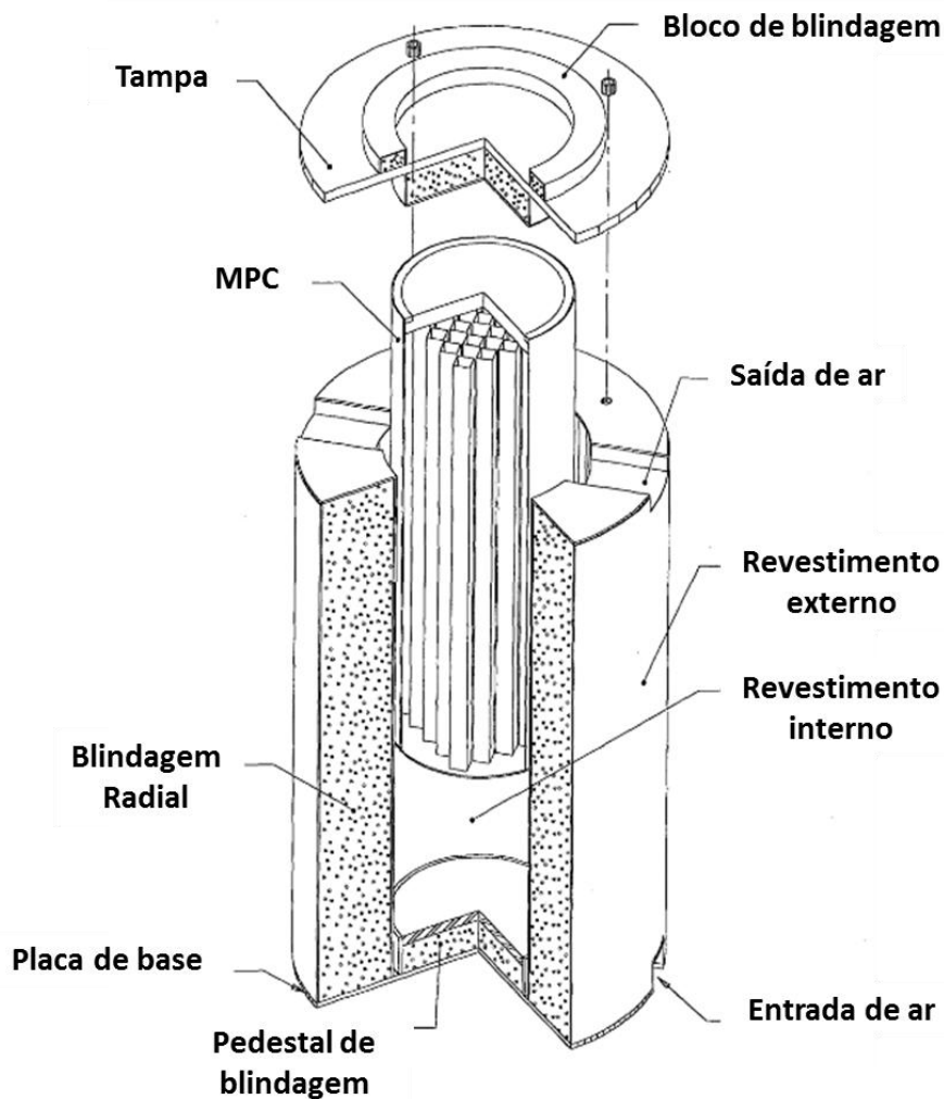
Figura 17 - Overpack do sistema HI-STORM 100 com o MPC parcialmente inserido (adaptado de HOLTEC, 2010a)
