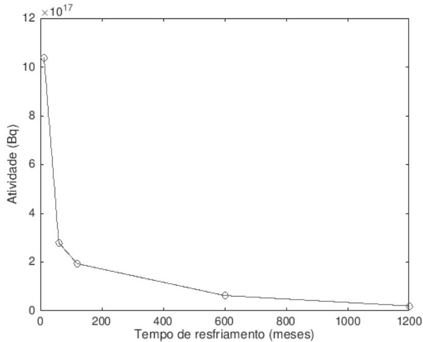
Figura 29 - Valores linearmente interpolados para a atividade da fonte adaptada em função do tempo de resfriamento inicial
