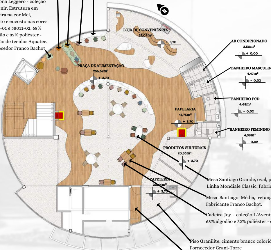
1 Layout Praça de Alimentação Escala 1:25
