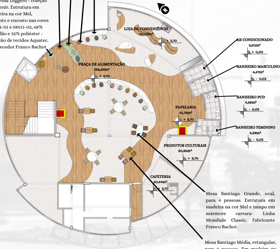
1 Layout Praça de Alimentação Escala 1:25
