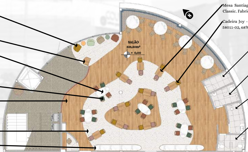
1 Layout Salão do Restaurante Escala 1:25
