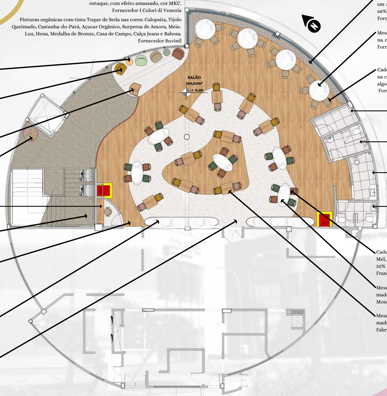
1 Layout Salão Restaurante Escala 1:50
