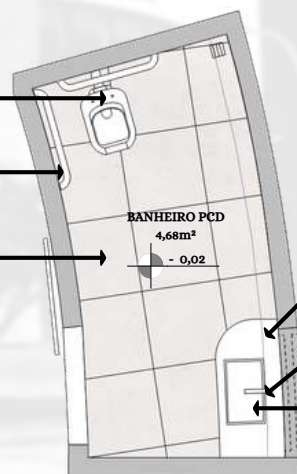
1 Banheiro PCD Escala 1:25
