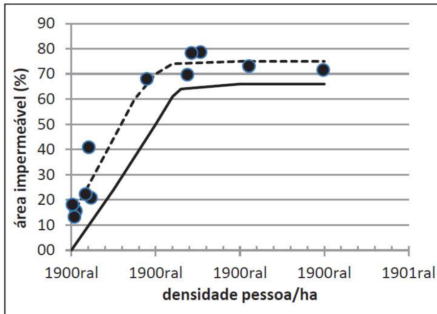
Figura 30. Área impermeável (%) X densidade populacional (pessoas/ha). A curva tracejada reflete a atualização da relação para a cidade de Porto Alegre. Fonte: MENEZES FILHO e TUCCI (2012)
