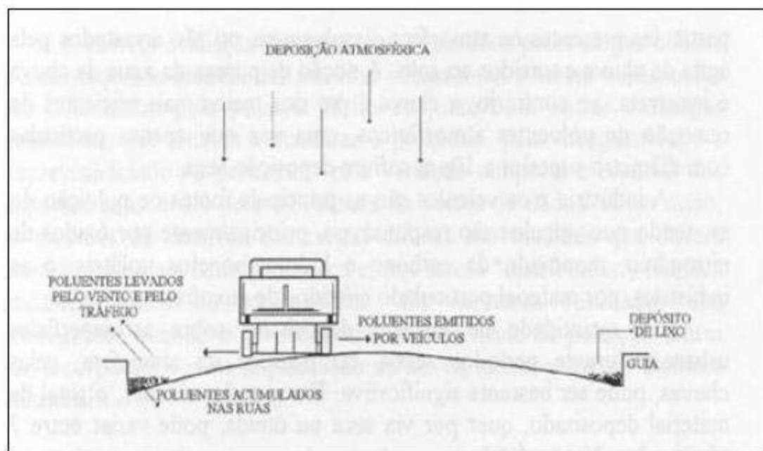
Figura 7. Principais processos responsáveis pelo acúmulo de poluentes nas ruas.
