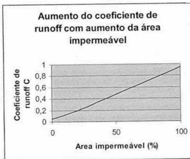
Figura 3. Relação entre área impermeável e o coeficiente de runoff Fonte: TOMAZ (2006)
