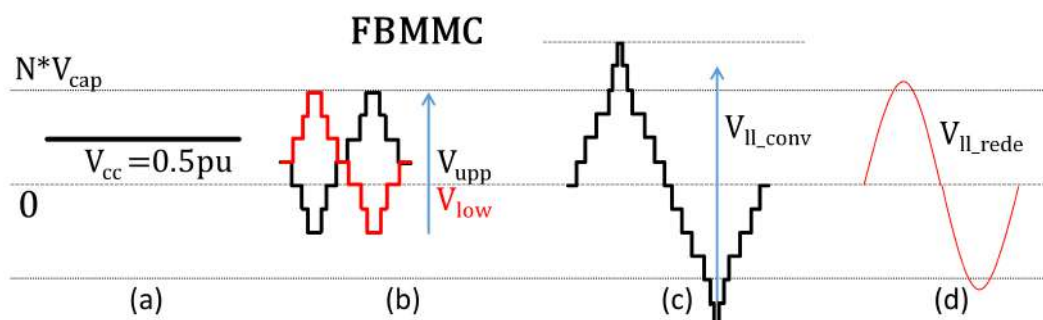
Figura 2.3: Modo de operação para FBMMC com tensão CC reduzida e sobremodulação CA. (a) Tensão CC. (b) Tensões no braço superior ( V_{upp} ) e inferior ( V_{low} ). (c) Tensão entre fases do conversor. (d) Tensão da rede.
