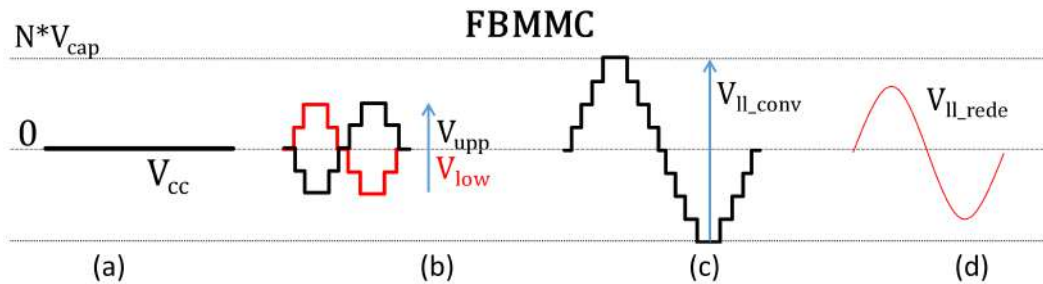
Figura 2.2: Modo de operação para FBMMC com tensão CC igual a zero. (a) Tensão CC. (b) Tensões no braço superior ( V_{upp} ) e inferior ( V_{low} ). (c) Tensão entre fases do conversor. (d) Tensão da rede.
