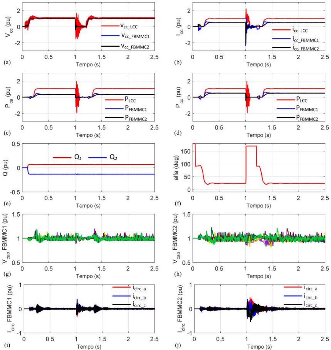
Figura 4.8: Comportamento do HVDC híbrido multiterminal frente à ocorrência de um curto-circuito CC polo-terra próximo ao FBMNC 1 - Curto CC 2 da Figura 4.4: (a) tensões cc; (b) correntes cc; (c) potência ativa nas barras ca; (d) potência ativa nos terminais cc; (e) potência reativa em p1 e p2; (f) ordem de ângulo de disparo \alpha ; (g) tensões nos capacitores do FBMNC1 - fase a; (h) tensões nos capacitores do FBMNC2 - fase a; (i) correntes circulantes no FBMNC1; (j) correntes circulantes no FBMNC2.
