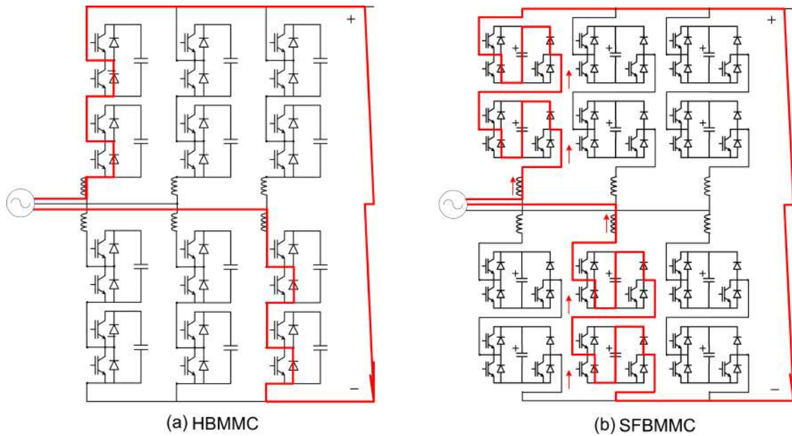
Figura 1.2: Caminho da corrente de curto-circuito do lado CA para o lado CC com chaves bloqueadas. (a) HBMMC. (b) SFBMMC.
