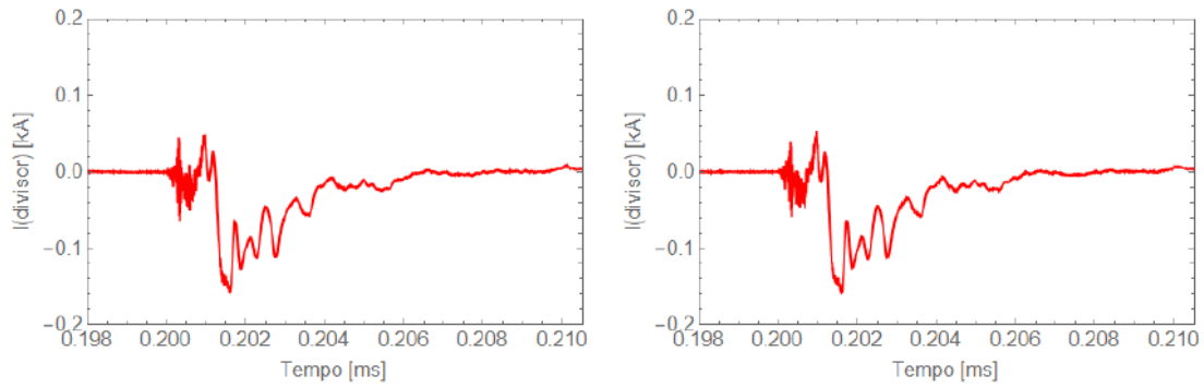
Corrente - TC 20 kA - 2000 kV
