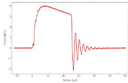
Oscilograma 12
