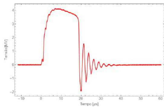
Oscilograma 16
