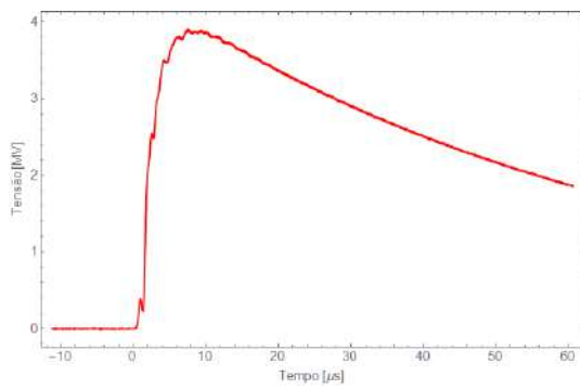
Oscilograma 17
