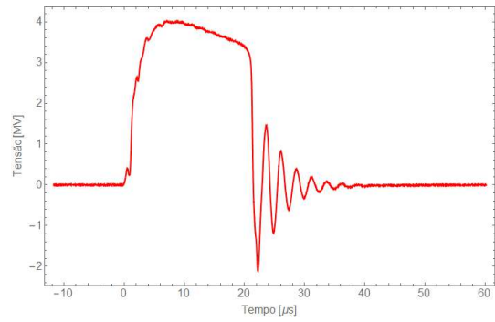
Oscilograma 26
