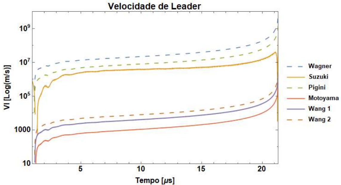
Figura 4.9: Gráficos das velocidades do leader obtidos a partir das equações de WAGNER [1], SUZUKI [3], MOTOYAMA [4], PIGNI [5] e WANG [6].
