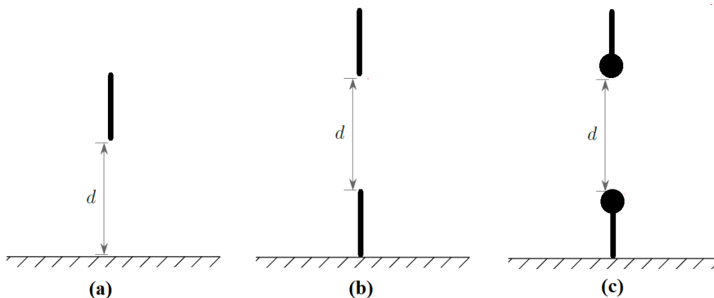
Figura 2.10: Tipos de configurações de gaps : (a) - Ponta-plano, (b) - ponta-ponta e (c) - esfera-esfera.
