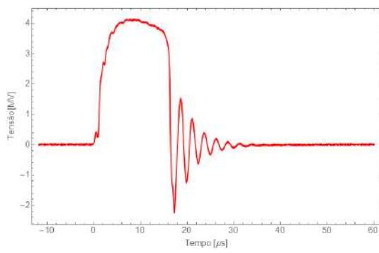
Oscilograma 21
