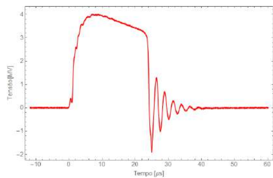
Oscilograma 14
