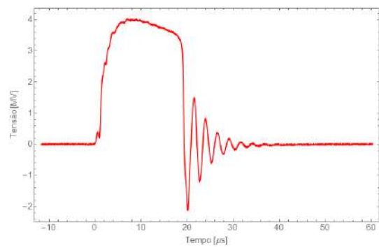
Oscilograma 22
