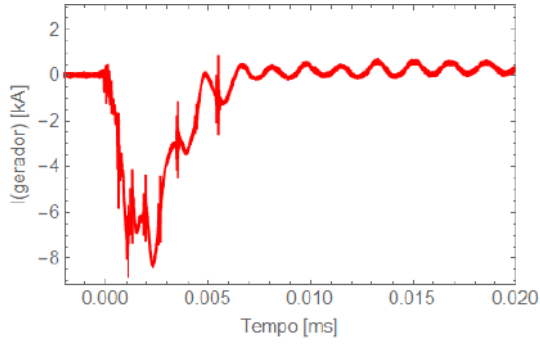
Corrente - TC 50 kA - 2000 kV 9
