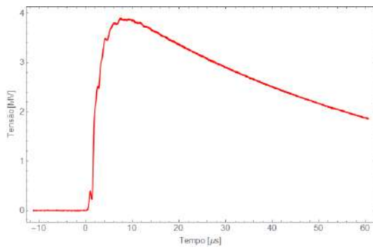
Oscilograma 27
