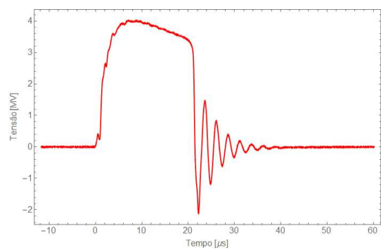
Oscilograma 28
