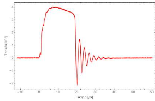
Oscilograma 10
