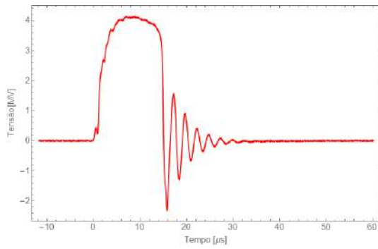
Oscilograma 25
