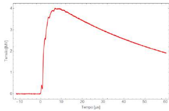
Oscilograma 18
