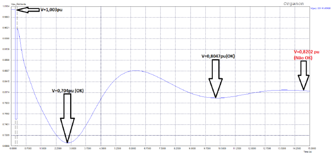
Figura 4.6: Simulação dinâmica da variação de tensão no barramento 231 R. VERDE-230
