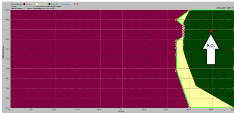
Figura 4.8: Nomograma G_1XG_2 da região de segurança obtida com a simulação do redespatcho termelétrico 1
