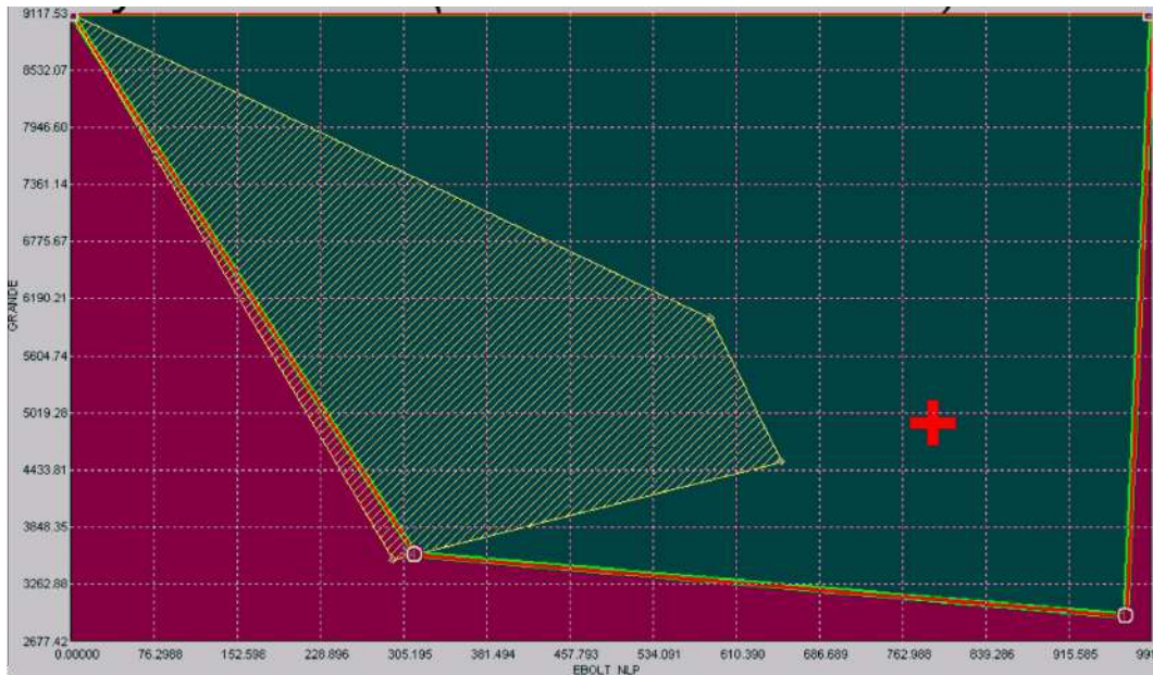
Figura 4.36: Despacho Termelétrico para evitar possível atuação do EEP-GRAJAU
