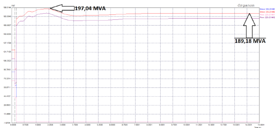
Figura 4.27: Rede alterada 1: sobrecarga em ITUMBIRA-R.VERDE230#2 eliminada pelo redespacho termelétrico e elevação de geração nas outras usinas do Grupo 1
