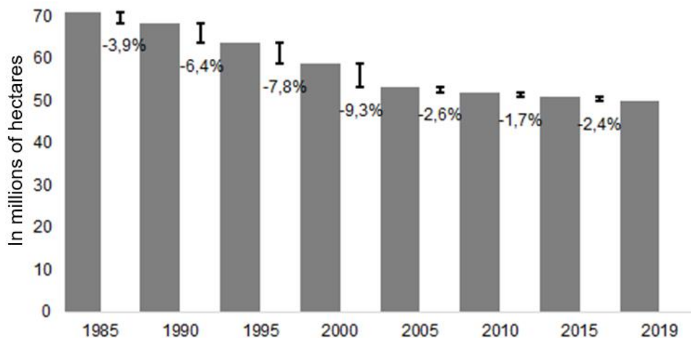
Figure 6. Variation of forest cover (in hectares) from 1985 to 2019 in Mato Grosso. Figura 2. Variação da cobertura florestal (em hectares) de 1985 a 2019 em Mato Grosso. Source: Own elaboration.from Projeto MapBiomias.
