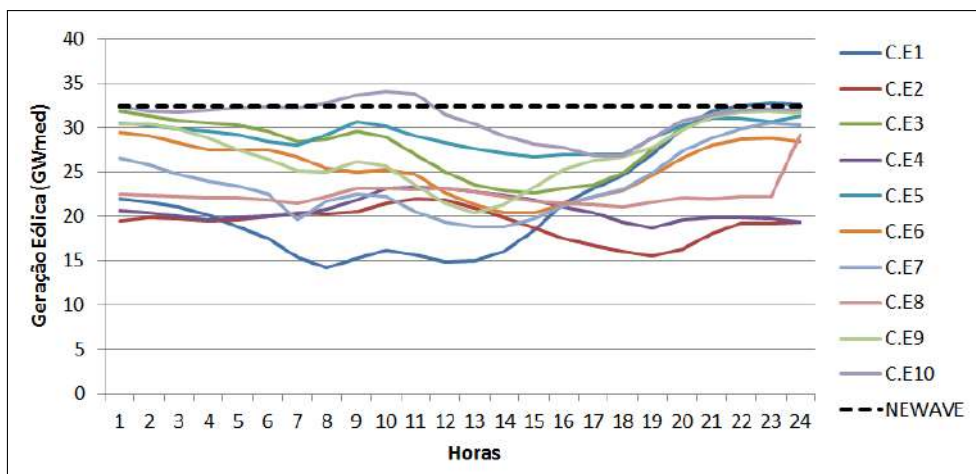
Figura 5.22: Geração horária de usinas eólicas do terceiro dia de agosto de 2031.
