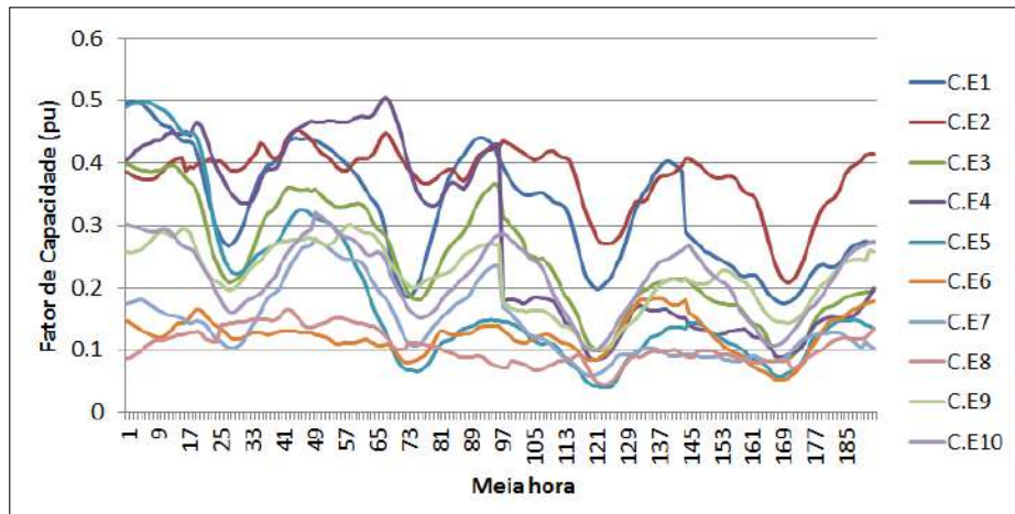
Figura 4.7: Fator de capacidade horário das séries de vento utilizadas em fevereiro.
