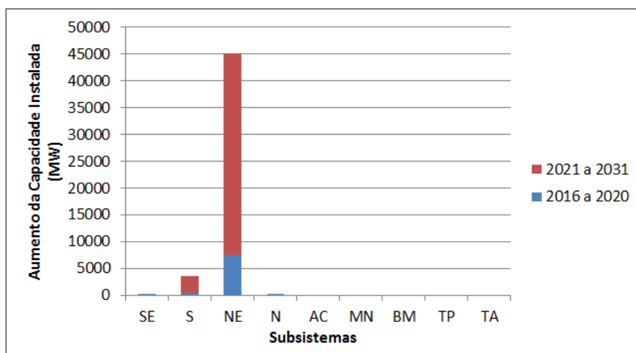
Figura 5.5: Aumento da capacidade instalada de usinas eólicas por subsistema.
