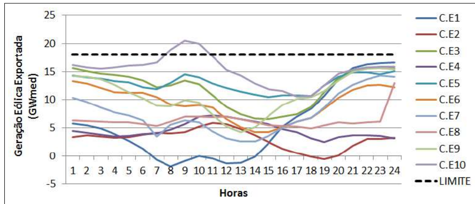
Figura 5.39: Explotação de geração eólica do Nordeste no terceiro dia de agosto de 2031.
