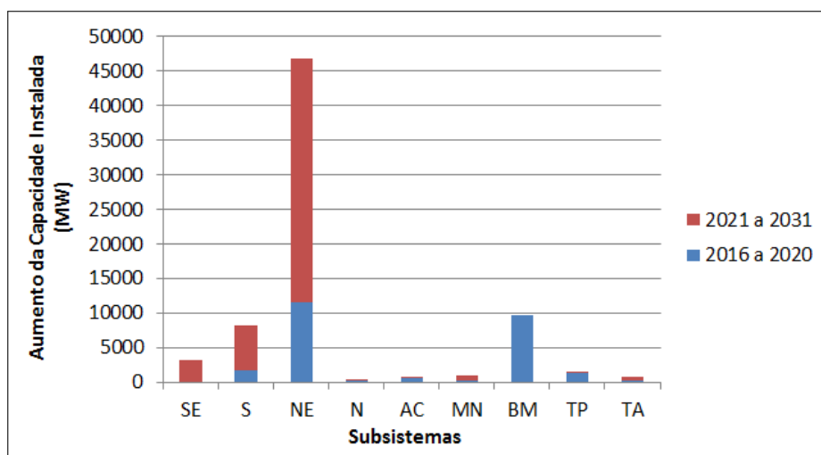
Figura 5.3: Aumento da capacidade instalada total por subsistema.
