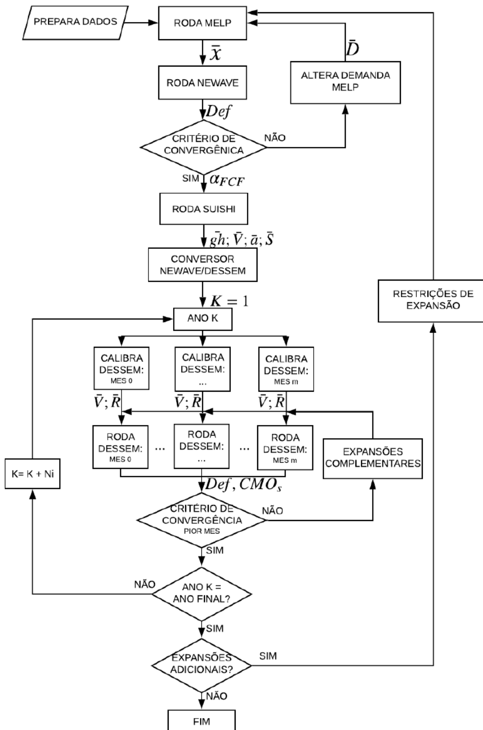
Figura 3.6: Fluxograma da proposta metodológica com modelos descritos.
