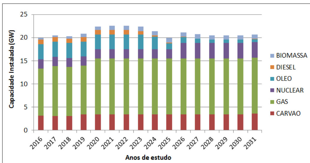
Figura 5.2: Evolução da capacidade instalada das usinas térmicas.
