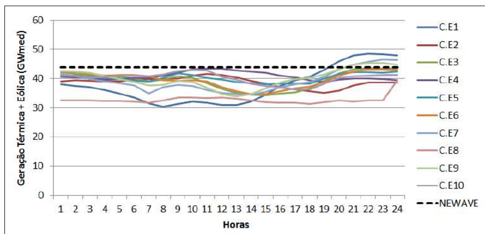
Figura 5.24: Soma da geração térmica e geração eólica horária total do terceiro dia de agosto de 2031.
