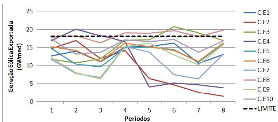
Figura 5.38: Exportação de geração eólica do Nordeste nos dois primeiros dias de agosto de 2031.
