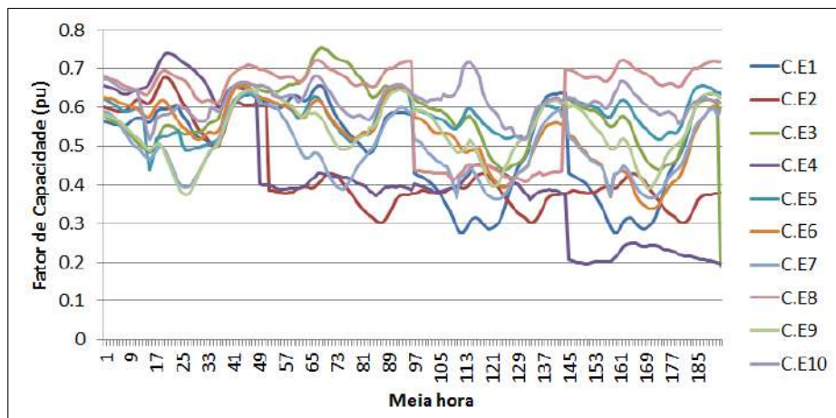
Figura 4.8: Fator de capacidade horário das séries de vento utilizadas em agosto.
