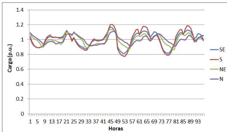
Figura 4.4: Perfil de demanda horário de fevereiro.
