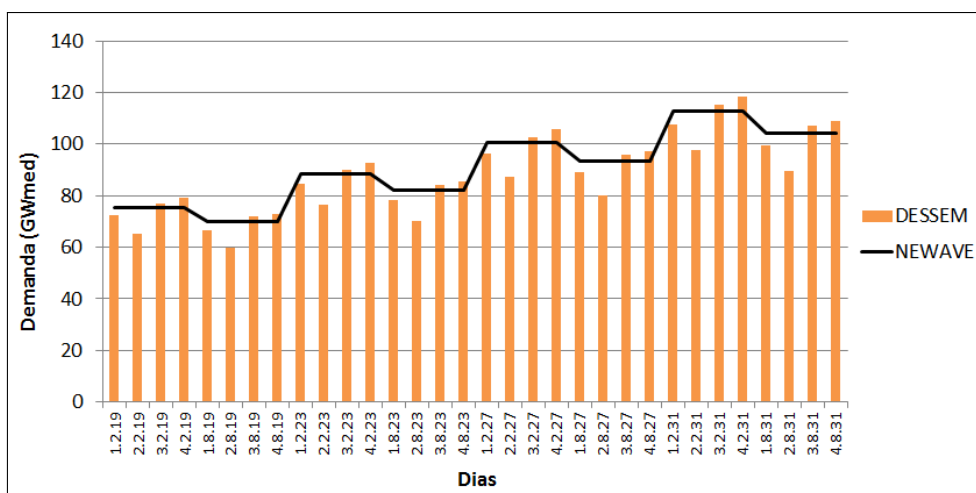
Figura 5.19: Média da demanda total de energia para cada dia dos meses simulados.
