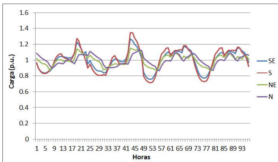
Figura 4.5: Perfil de demanda horário de agosto.
