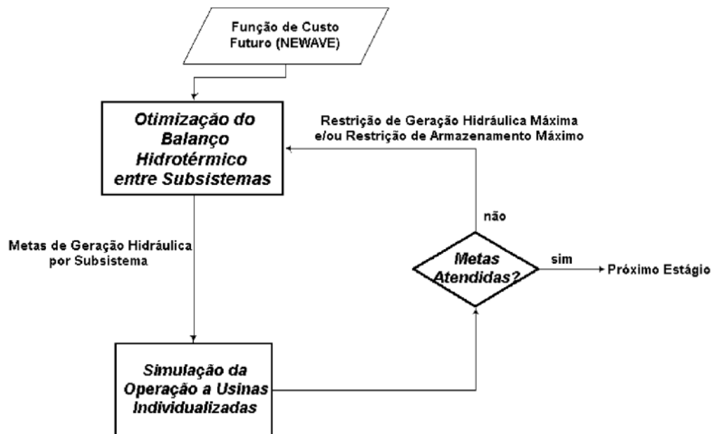
Figura 3.3: Processo iterativo realizado na simulação hidrotérmica. (Fonte: CEPEL, 2013, p. 4 [93])
