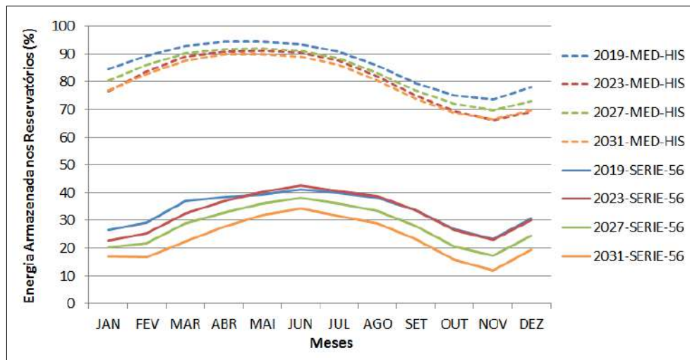
Figura 5.17: Energia armazenada nos reservatórios da série histórica de 1956 e da média das séries históricas.
