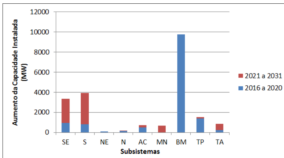
Figura 5.4: Aumento da capacidade instalada de UHE por subsistema.
