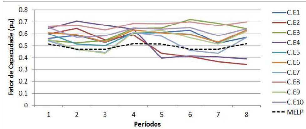
Figura 5.41: Curvas de geração eólica em agosto para os dois primeiros dias de simulação do DESSEM.
