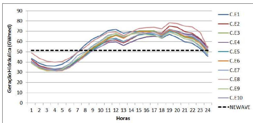
Figura 5.25: Geração hidráulica horária total do terceiro dia de agosto de 2031.
