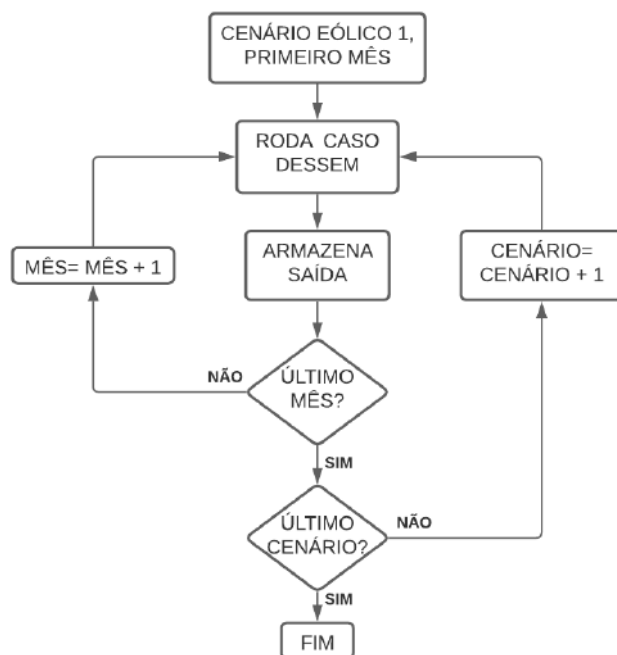
Figura 3.5: Fluxograma representativo da rotina que administra as execuções do DESSEM.
