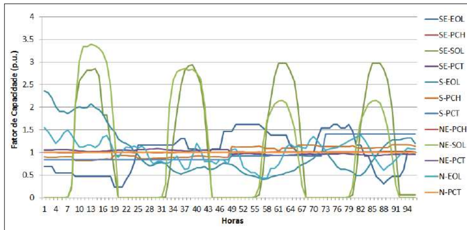
Figura 4.9: Perfis horários de geração das usinas não despachadas centralizadamente, exceto eólica, em fevereiro.
