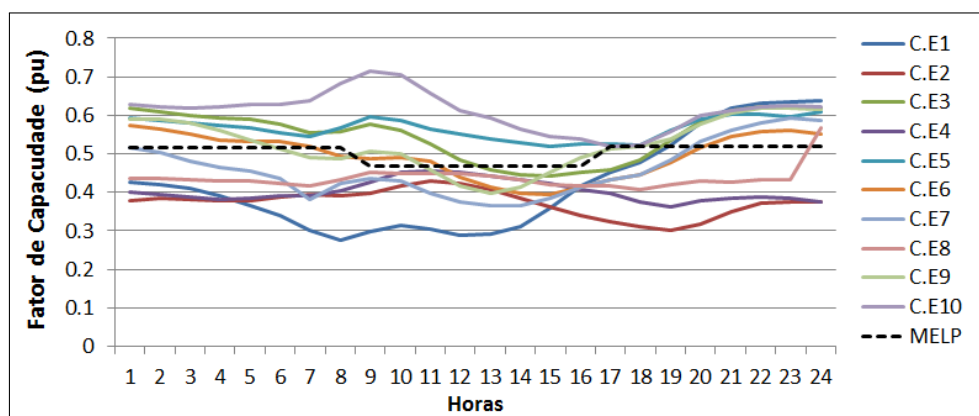
Figura 5.42: Curvas horárias de geração eólica em agosto para o terceiro dia de simulação do DESSEM.
