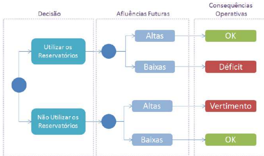
Figura 2.2: Consequências operativas de um sistema hidrotérmico.
