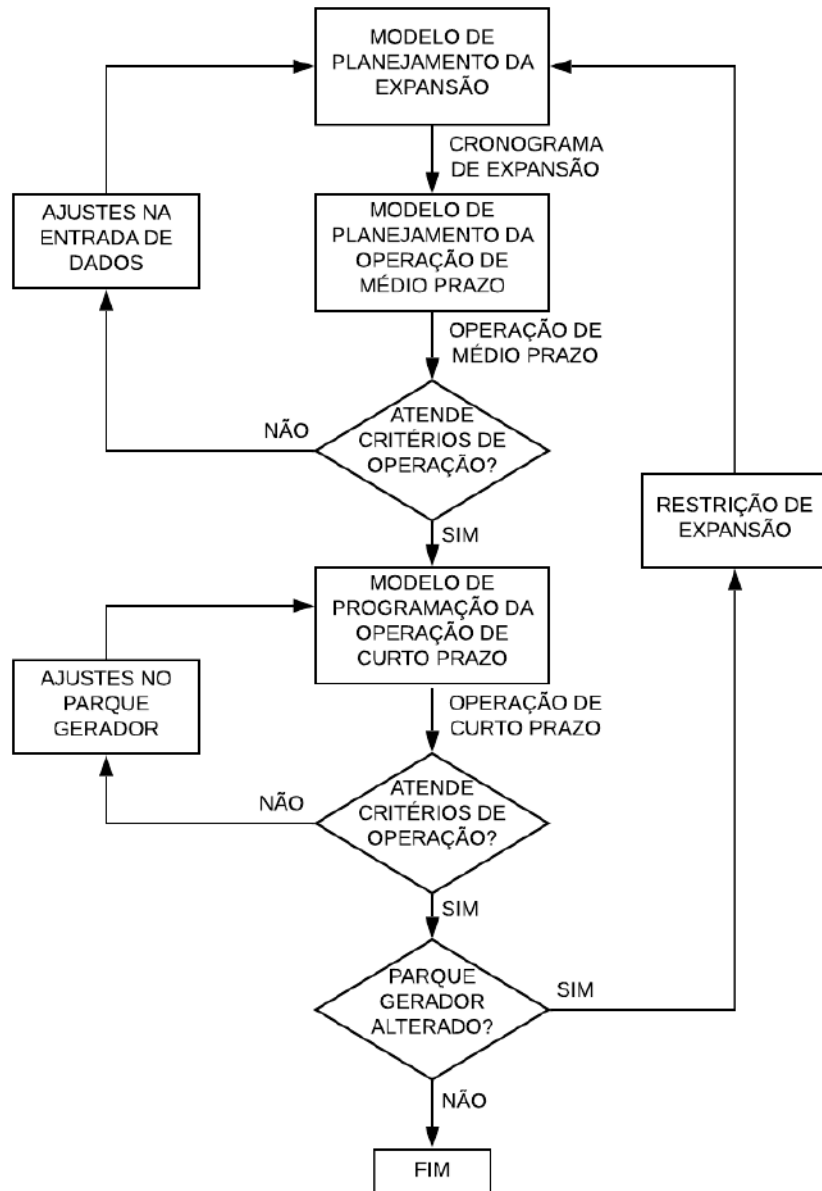
Figura 3.1: Fluxograma representativo da metodologia proposta.
