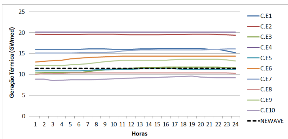
Figura 5.23: Geração térmica horária total do terceiro dia de agosto de 2031.
