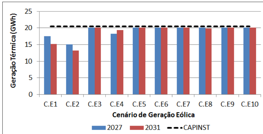
Figura 5.31: Geração térmica as 15h do terceiro dia de fevereiro de 2027 e 2031.
