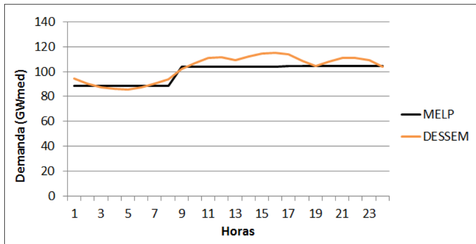
Figura 5.32: Curvas horárias de demanda do terceiro dia de fevereiro de 2027.
