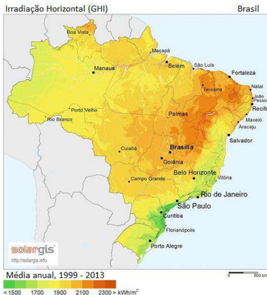
Figura 1 - Índices de irradiância global horizontal no Brasil
