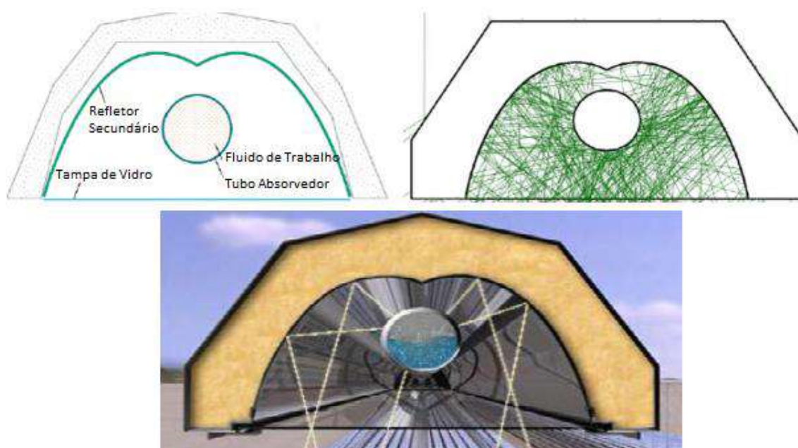
Figura 12 - Receptor de Cilindro único de Fresnel
