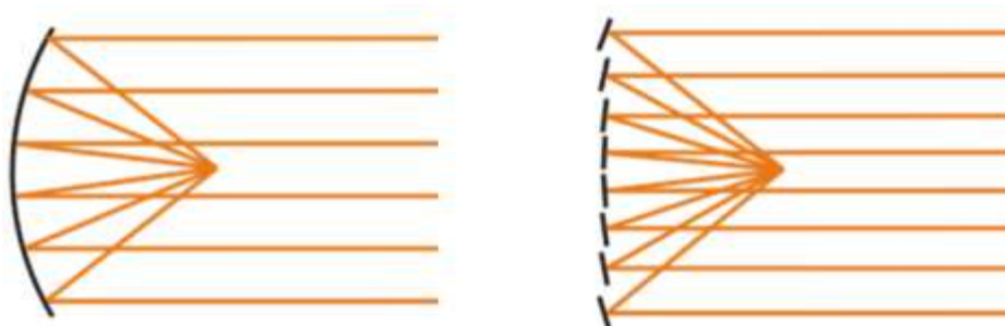
Figura 11 - Exemplo do posicionamento dos espelhos do concentrador Fresnel
