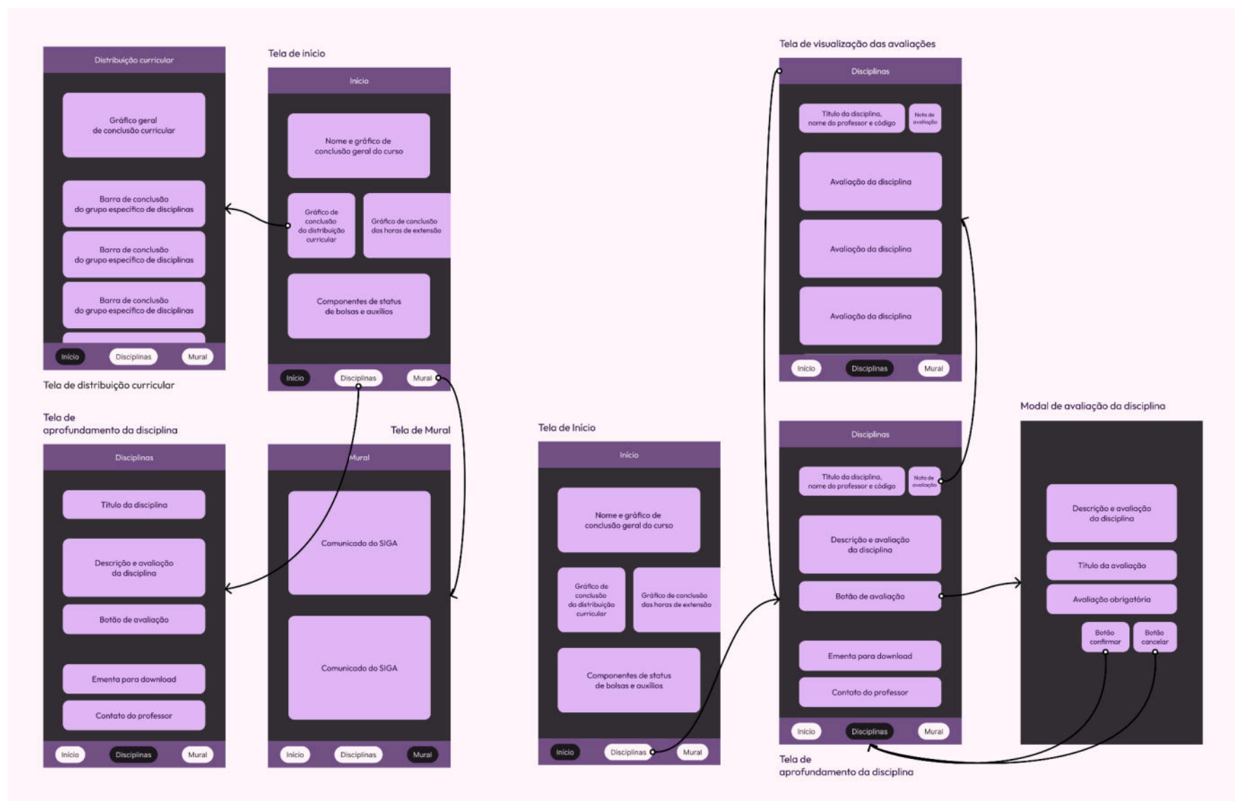
Figura 29 - Wireframes do Prometheus: componentes e navegação. Fonte: O Autor.
