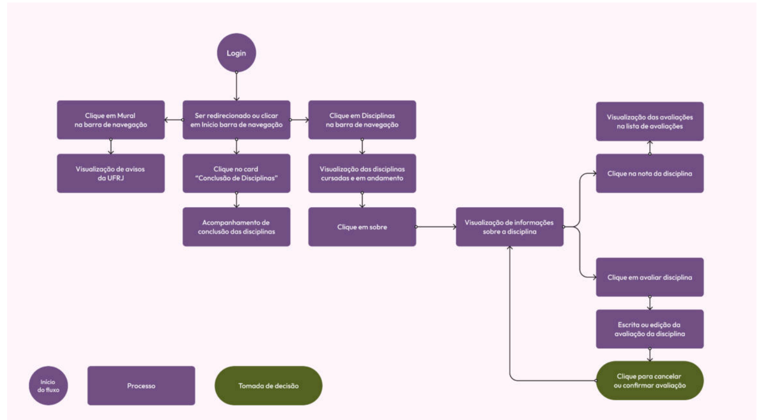
Figura 19 - Fluxo de navegação dos usuários no aplicativo. Fonte: O Autor.
