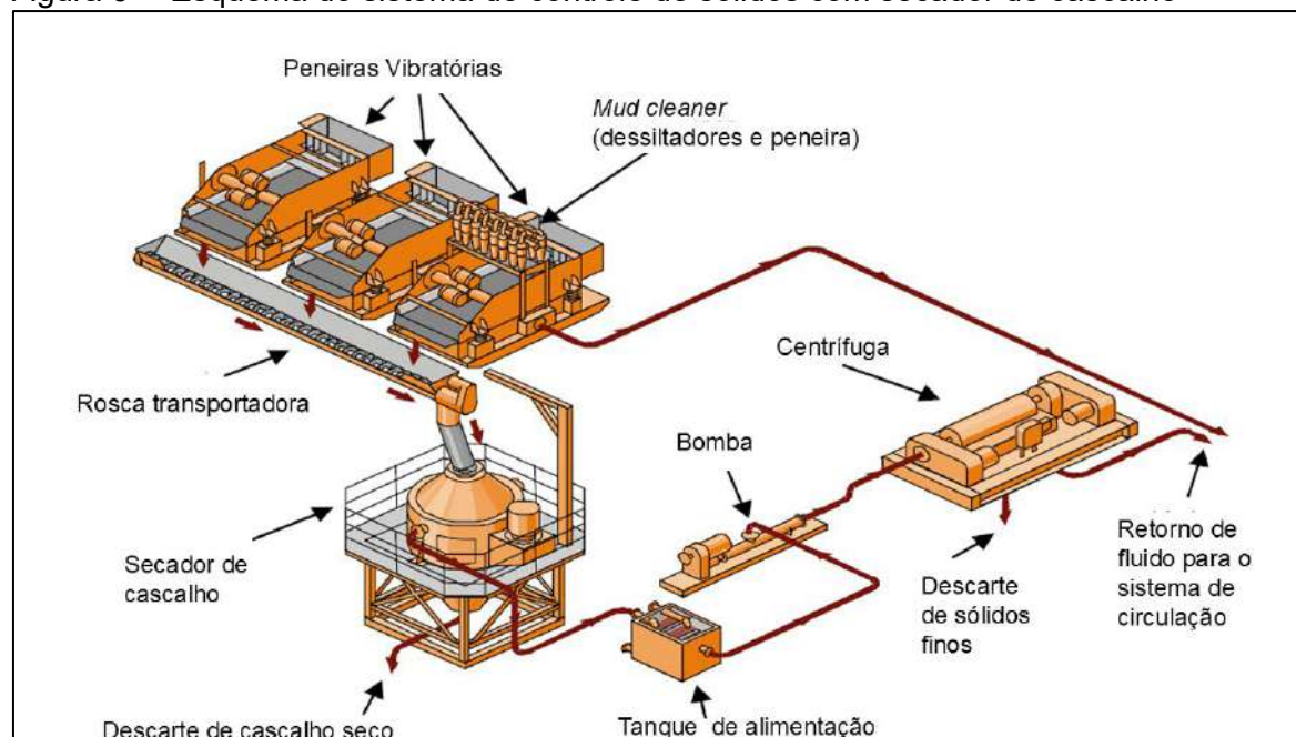
Figura 6 — Esquema do sistema de controle de sólidos com secador de cascalho
