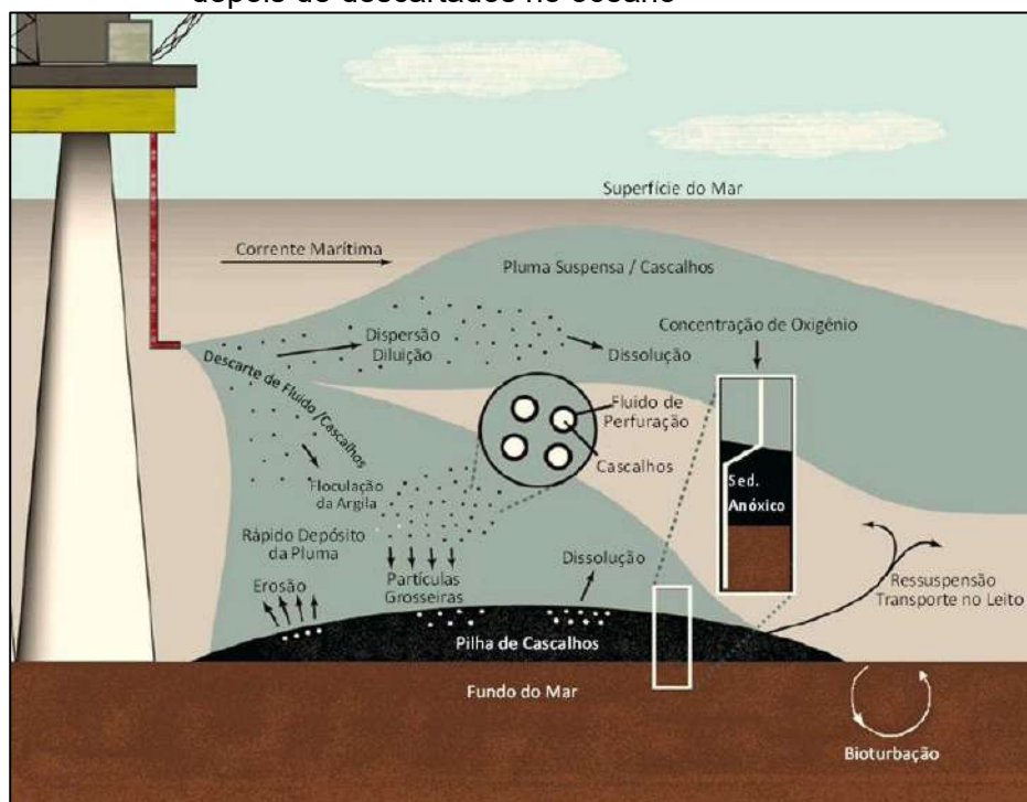
Figura 8 — Dispersão e destino do fluido de perfuração aquoso e cascalho depois de descartados no oceano
