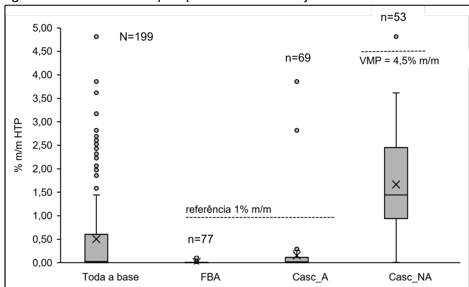
Figura 22 – Gráfico Box plot para as concentrações de HTP
