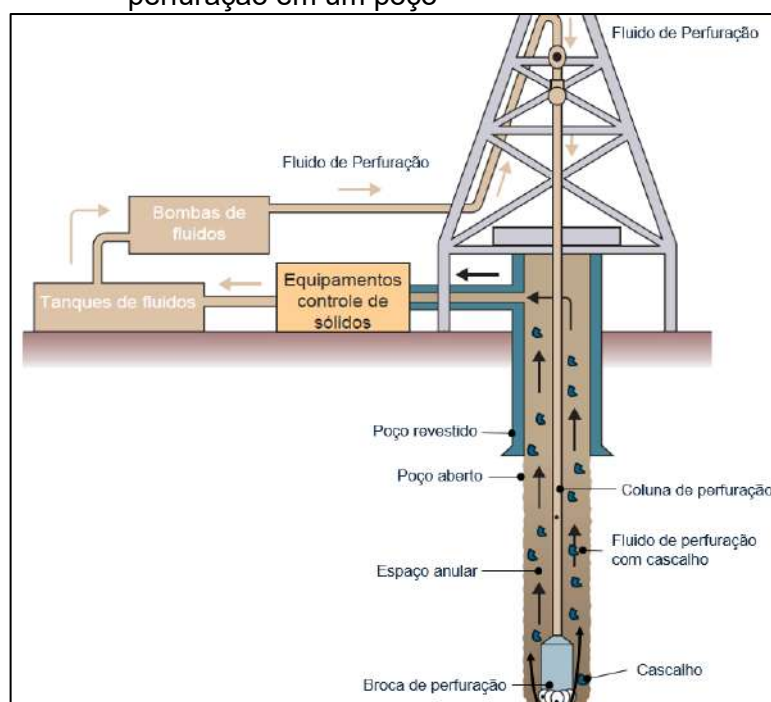
Figura 4 – Esquema simplificado da circulação do fluido de perfuração em um poço
