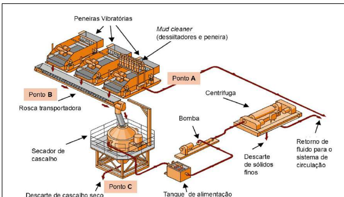
Figura 13 — Pontos de coleta de fluido e cascalho na superfície
