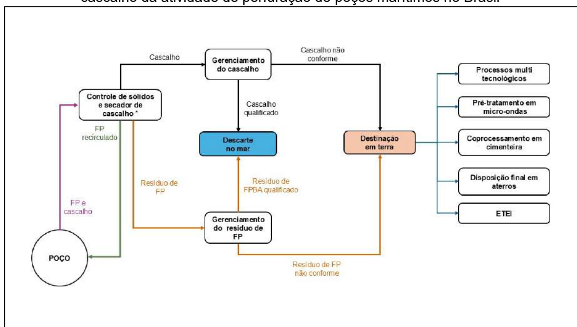
Figura 5 — Visão integrada das alternativas do gerenciamento de resíduos de fluidos e cascalho da atividade de perfuração de poços marítimos no Brasil
