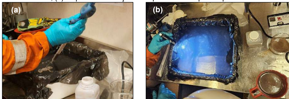
Figura 15 – Ensaio de iridescência estática. (a) etapa de adição do fluido aquoso no recipiente teste; (b) etapa de observação da superfície do corpo receptor teste
