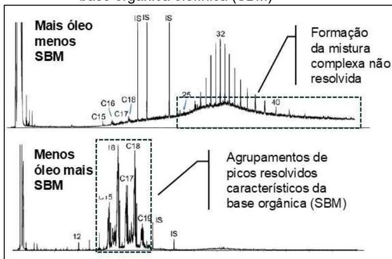
Figura 9 — Exemplos de cromatogramas de análise de HTP em amostras de sedimento marinho com óleo e base orgânica olefínica (SBM)
