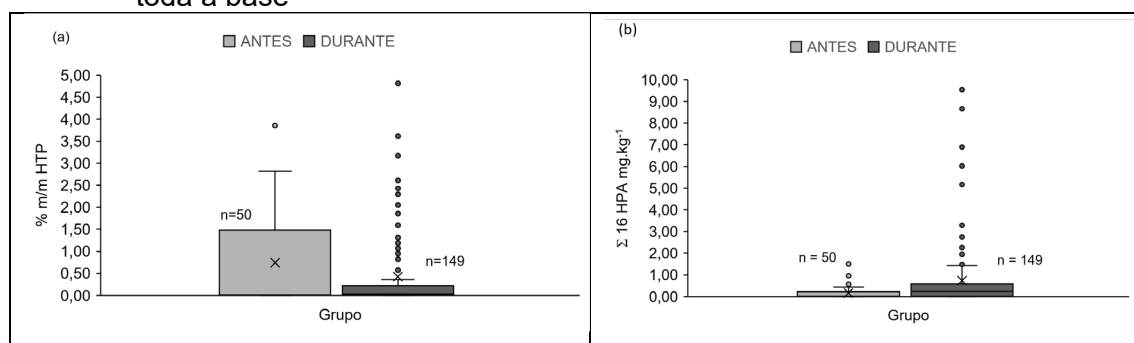
Figura 35 – Box plot para as concentrações de (a) HTP e (b) \Sigma 16\text{HPAs} considerando toda a base
