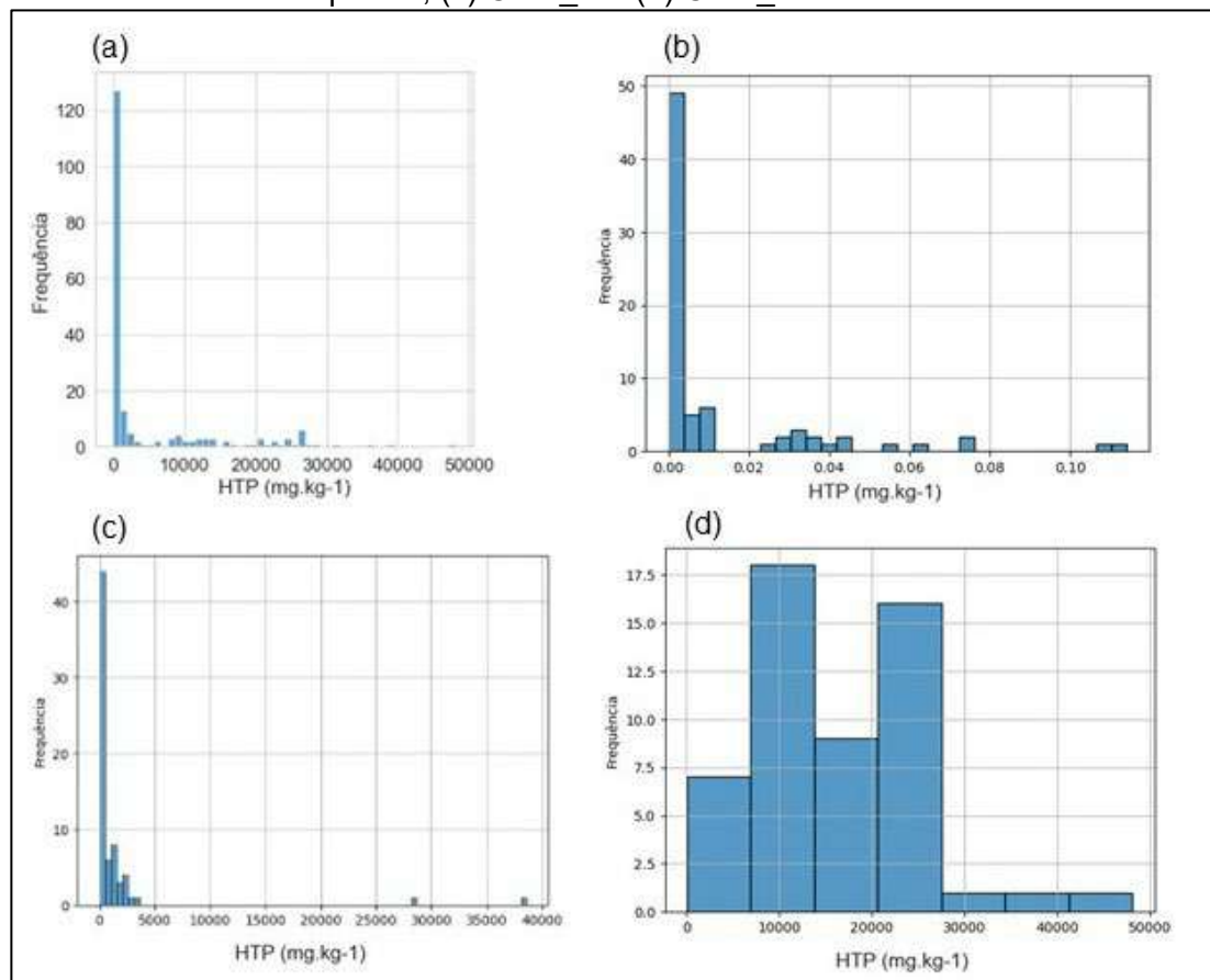
Figura 21 – Gráficos de frequência da concentração de HTP para: (a) toda a base; (b) fluidos aquosos; (c) Casc_A e (d) Casc_NA.
