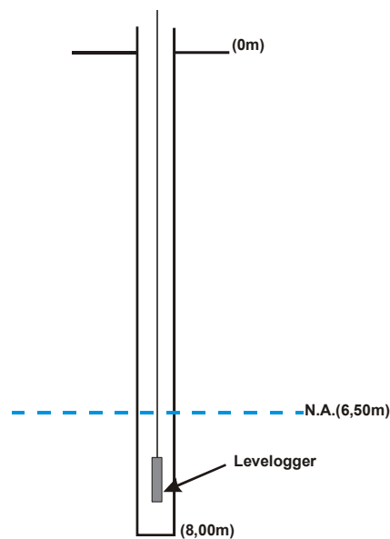
Figura 5 - Esquema do poço onde foi instalado o Levellogger .
