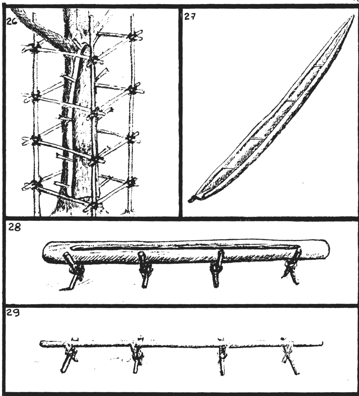
FIG.26-EXTRAÇÃO DA CASCA-DO-JATOBA PARA FAZER CANOA- APUD. PEDRO E. DELIMA 1950.- ESC. 1:100
