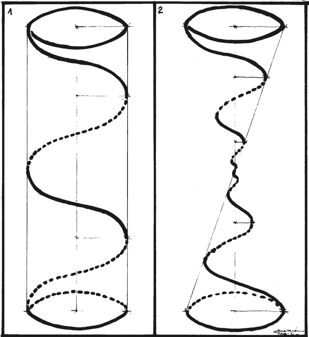
FIG.1 HELICOIDE DE REVOLUÇÃO
