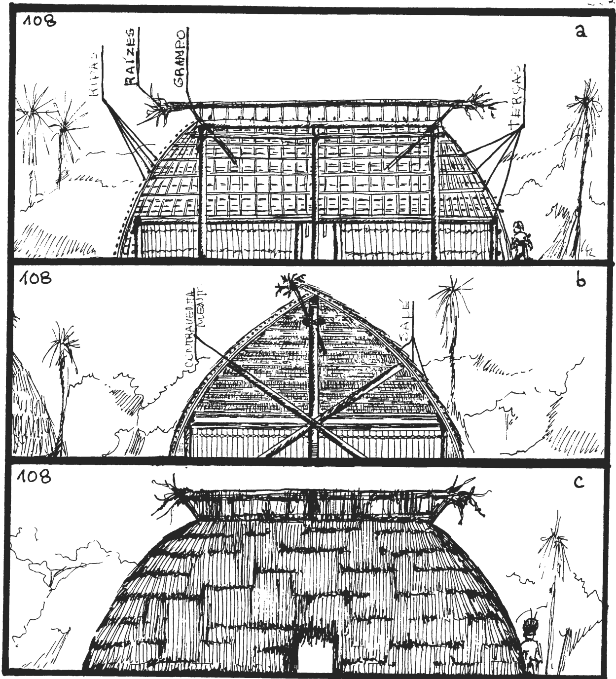
FIG.108-a- CORTE LONGITUDINAL -b- CORTE TRANSVERSAL -c- TACHADA -DE-DENTRO ESCALA 1:250
