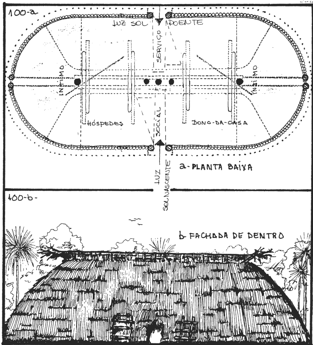
FIG.100- INSOLAÇÃO DA CASA-VERDADEIRA : a- PLANTA-BAIXA; b- FACHADA-DE-DENTRO - ESC. 1:200
