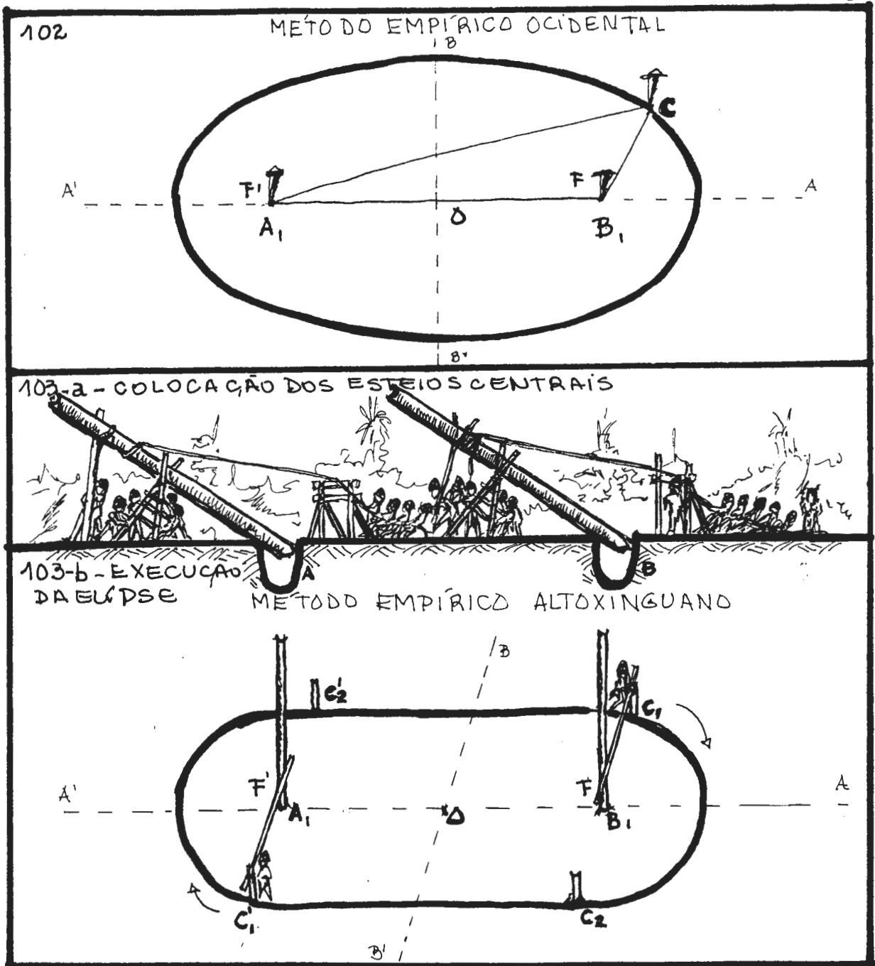
FIG.102- MÉTODO EMPÍRICO OCIDENTAL DE CONSTRUÇÃO DE UMA ELÍPSE E DEMARCAÇÃO DE SEU PERÍMETRO NO SOLO: "A" E "B" — ESTACAS FÍXAS "C" — ESTACA MÓVEL A, B, C — CORDA
