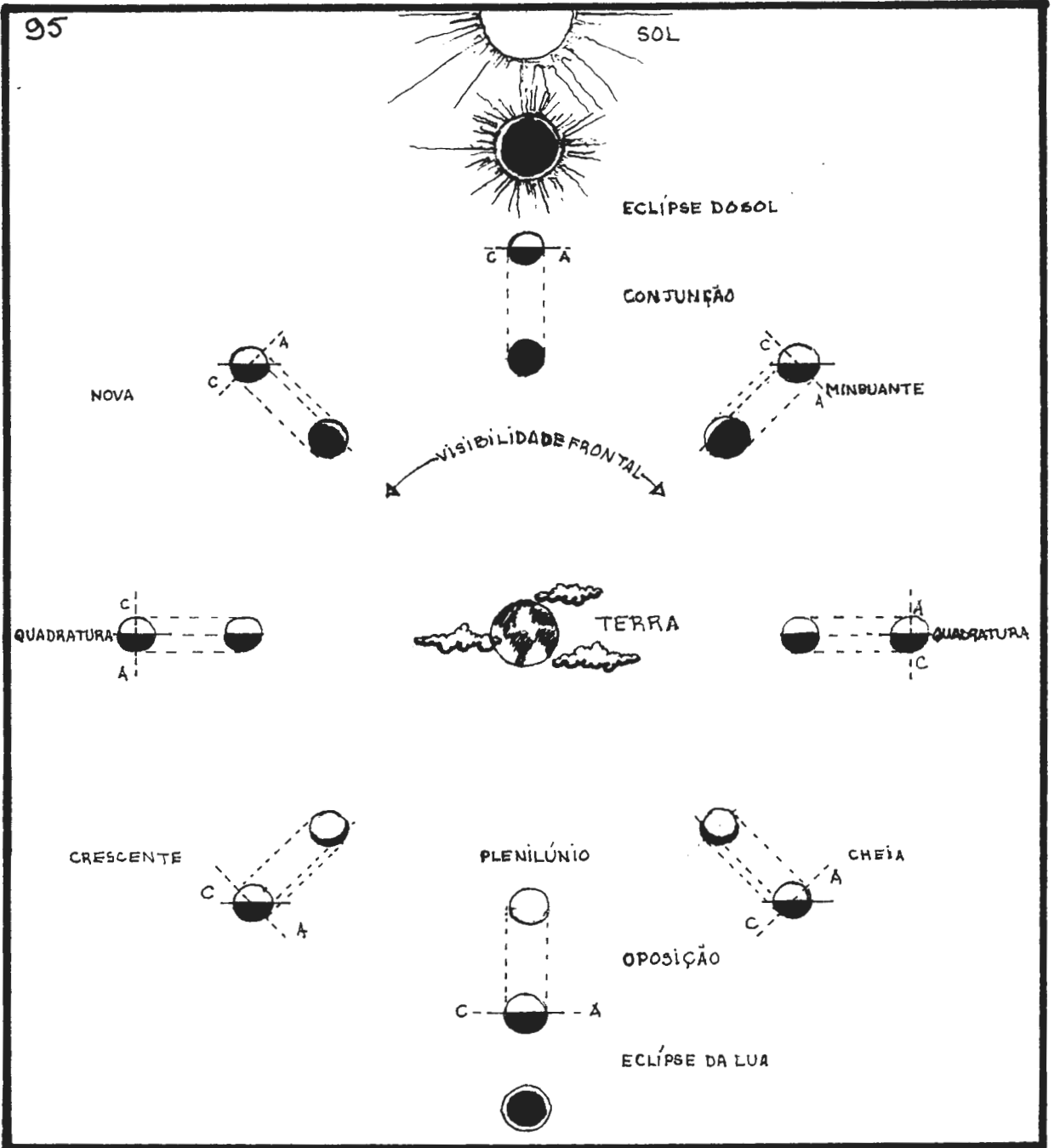
FIG. 95- FASES DA LUA; LUNACÕES; ECLÍPSES DA LUA E DO SOL - CA - CONTORNO APARENTE: LIMITA A VISIBILIDADE DO HEMISFÉRIO LUNAR EXPOSTO À TERRA - FORA DE ESCALA
