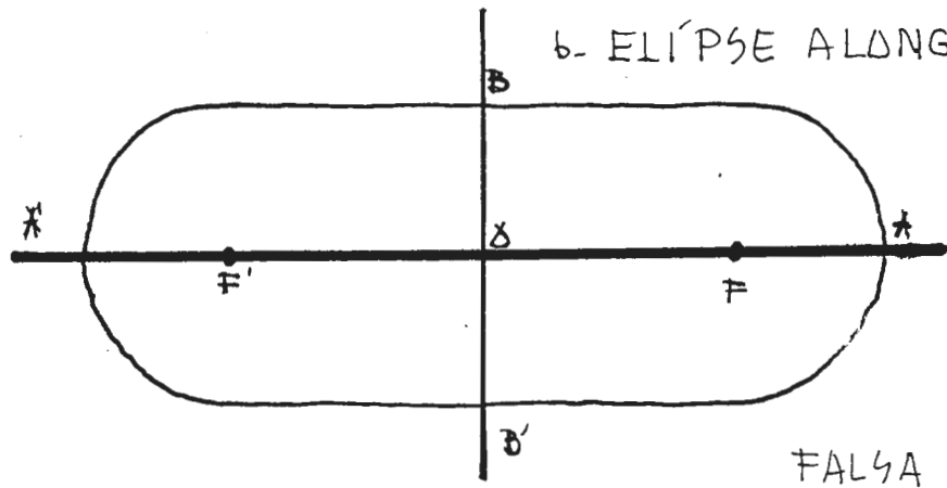
FIG.101- ELÍPSES : a- REGULAR; VERDADEIRA - b- ALONGADA; FALSA
