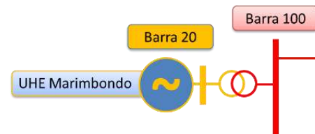
Figura 128 Diagrama esquemático da conexão da UHE Marimbondo
