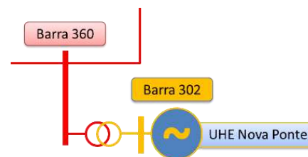
Figura 130 Diagrama esquemático da conexão da UHE Nova Ponte
