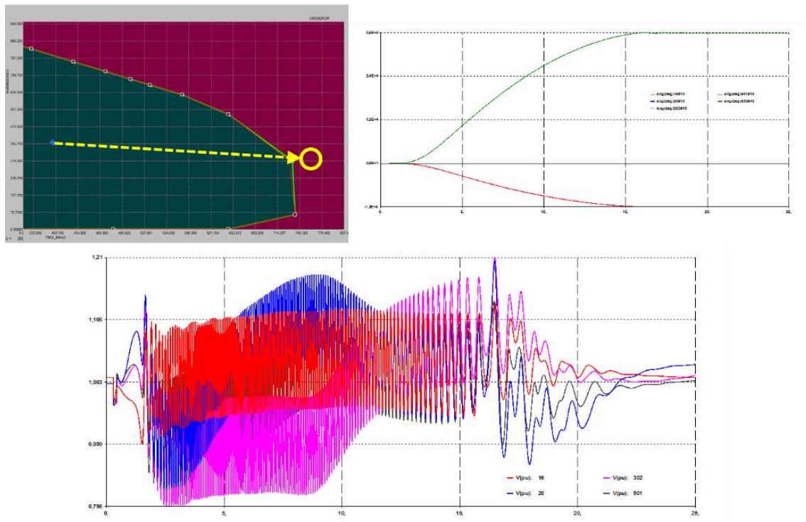
Figura 7 - Mosaico com a exploração de uma contingência em um ponto inseguro
