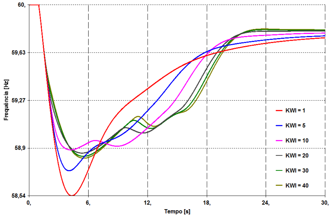
Figura 5.5: Freqüência – Ajuste do Ganho do Controlador
