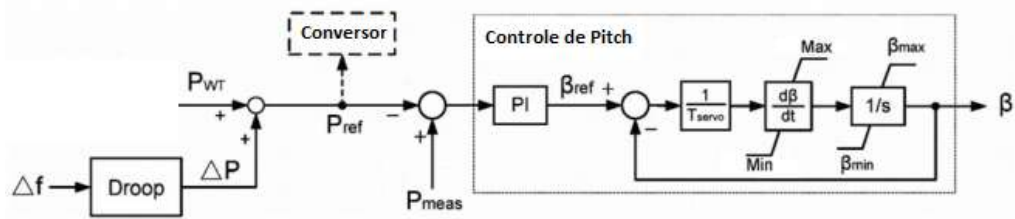
Figura 3.9: Modelo Modificado de Controle de Pitch
