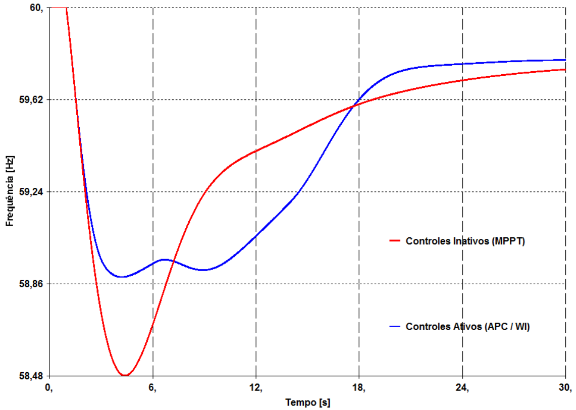
Figura 5.6: Frequência – Aumento de Carga
