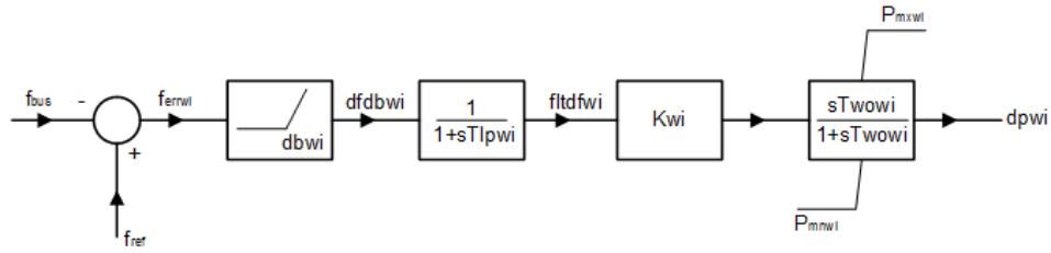
Figura 4.17: Representação Detalhada do Controle de Inércia Sintética
