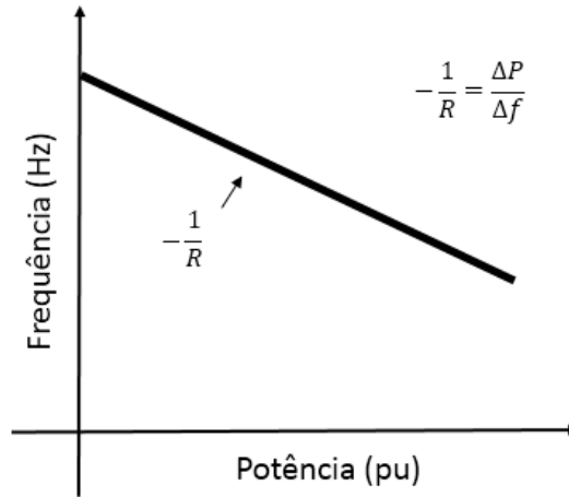
Figura 3.5: Curva Característica de Regulação ( Droop )
