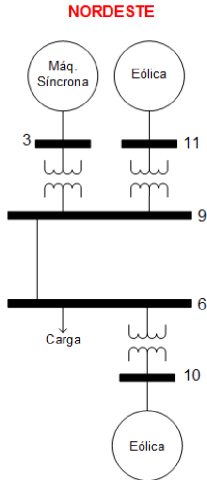
Figura 5.34: Sistema Nordeste Ilhado
