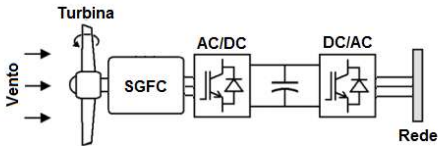
Figura 2.6: Gerador de Velocidade Variável - SGFC
