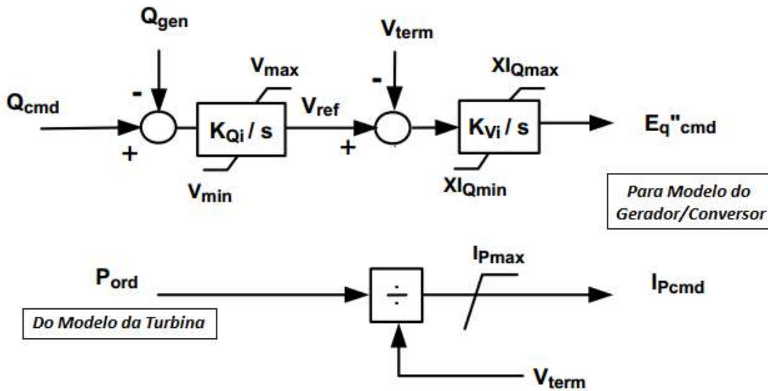
Figura 4.10: Representação do Modelo de Controles Elétricos
