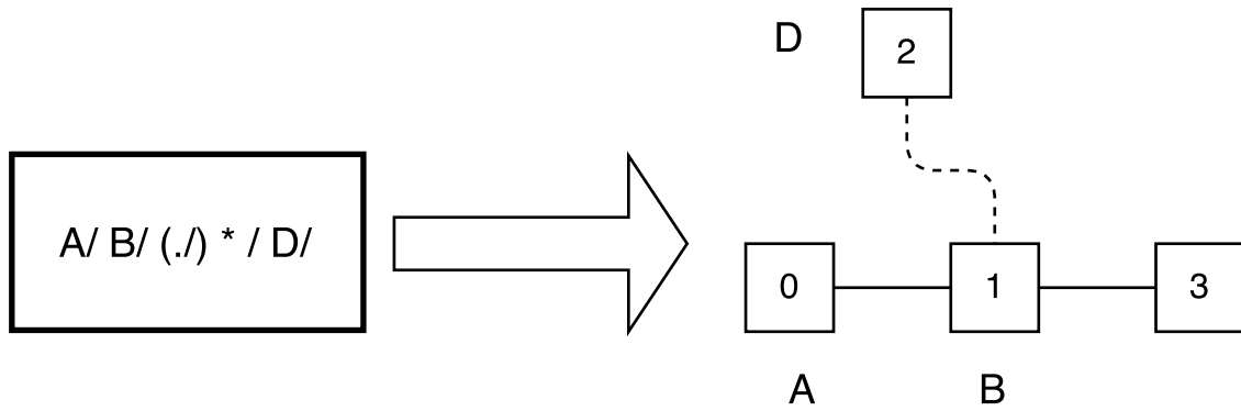
Figura 2.8: grafos
