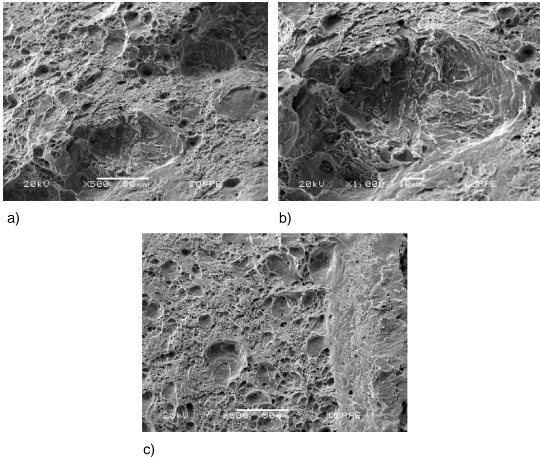
Figura 51 - Fractografias do material hidrogenado com aplicação de -1100 mV/ECS, a) aumento de 500 x – centro da superfície de fratura, b) aumento de 1000 x – centro da superfície de fratura, c) aumento de 500 x – borda da superfície de fratura .
