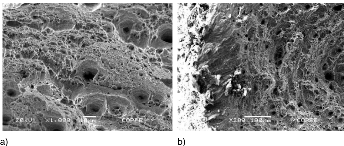
Figura 49 – Fractografias do material como recebido, a) aumento de 1000 x – centro da superfície de fratura, b) aumento de 200 x – borda da superfície de fratura.
