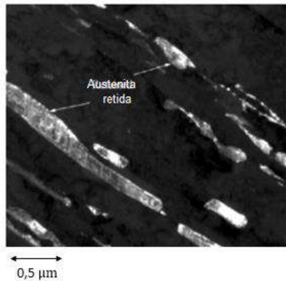
Figura 5 - Microestrutura de um AISM revenido, mostrando a austenita retida (Adaptado de [13]).
