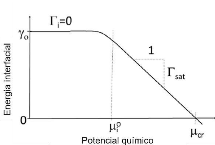
Figura 15 – Energia interfacial em função do potencial químico do hidrogênio (Adaptado de [4]).
