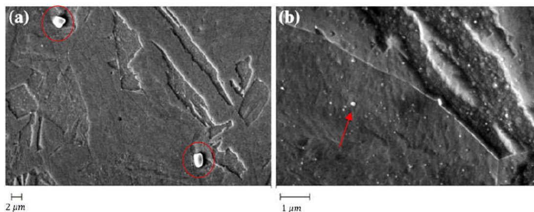
Figura 8 - Microestrutura de um AISM temperado, mostrando as partículas poliédricas de nitreto de titânio em (a) e carbeto de titânio (pontos brancos dispersos) em (b) (Adaptado de [5]).
