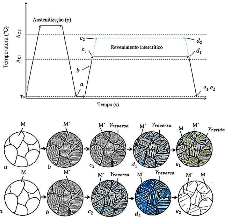
Figura 2 – Diagrama esquemático dos tratamentos térmicos e formação das fases (Adaptado de [23]).
