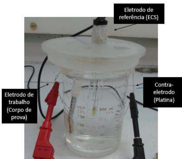
Figura 27 - Célula de hidrogenação.
