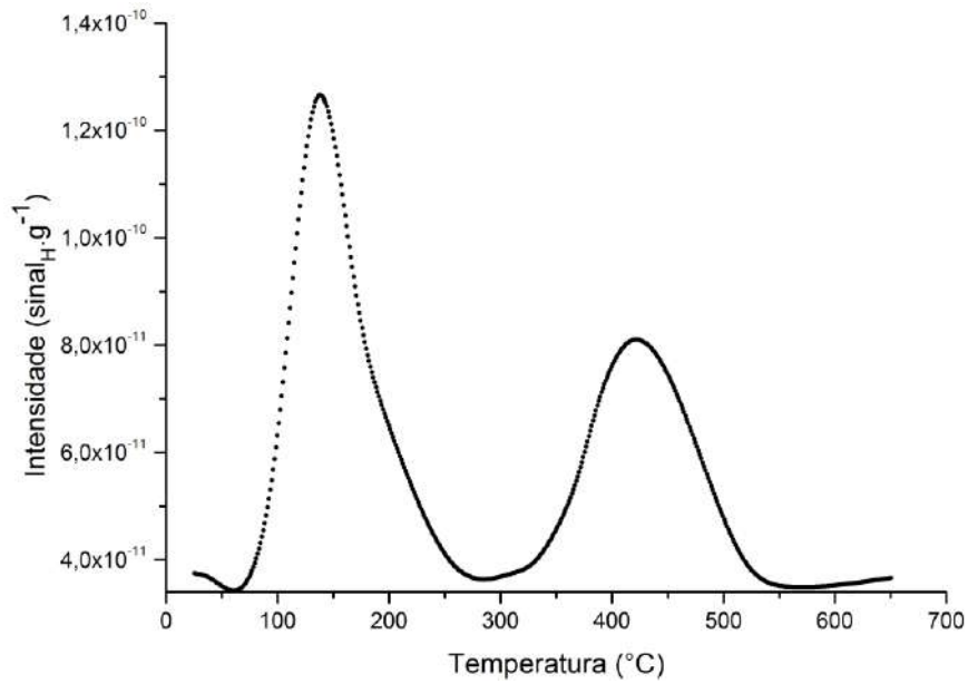
Figura 43 - Espectro de desorção para a amostra hidrogenada com aplicação de -1100mV/ECS.
