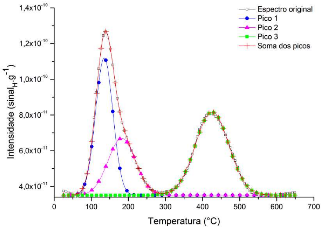
Figura 44 – Espectro de desorção com a deconvolução dos picos.
