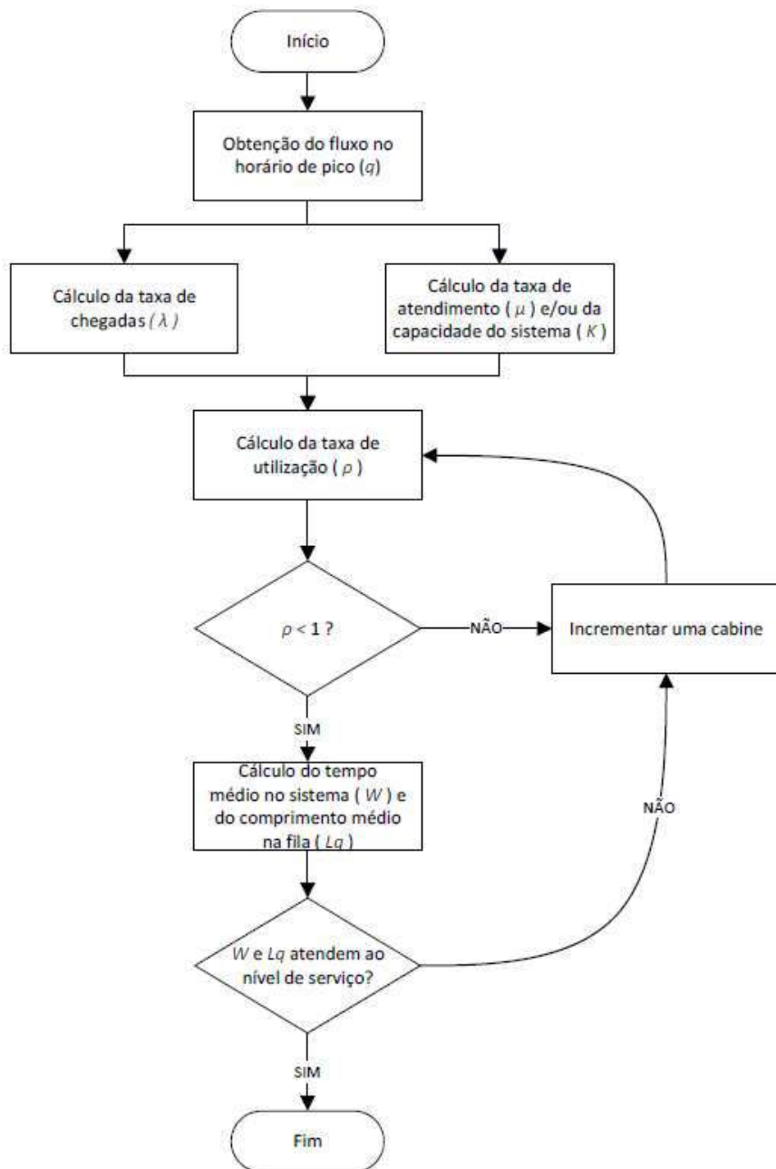
Figura 2.6: Dimensionamento do número de cabines
