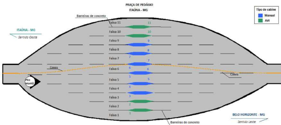
Figura 5.9: Configuração da praça de pedágio de Itaúna/MG no pico da manhã
