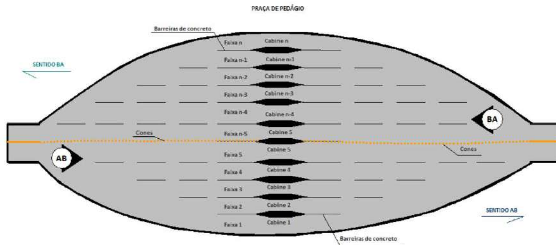
Figura 4.2: Exemplo de estrutura de praça de pedágio
