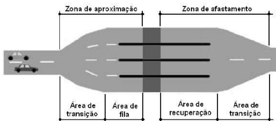
Figura 2.5: Elementos de projeto do layout de uma praça de pedágio
