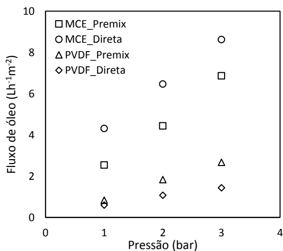
Figura 4.25 Fluxo de óleo ao longo dos testes de EM variando-se a pressão aplicada à membrana.
