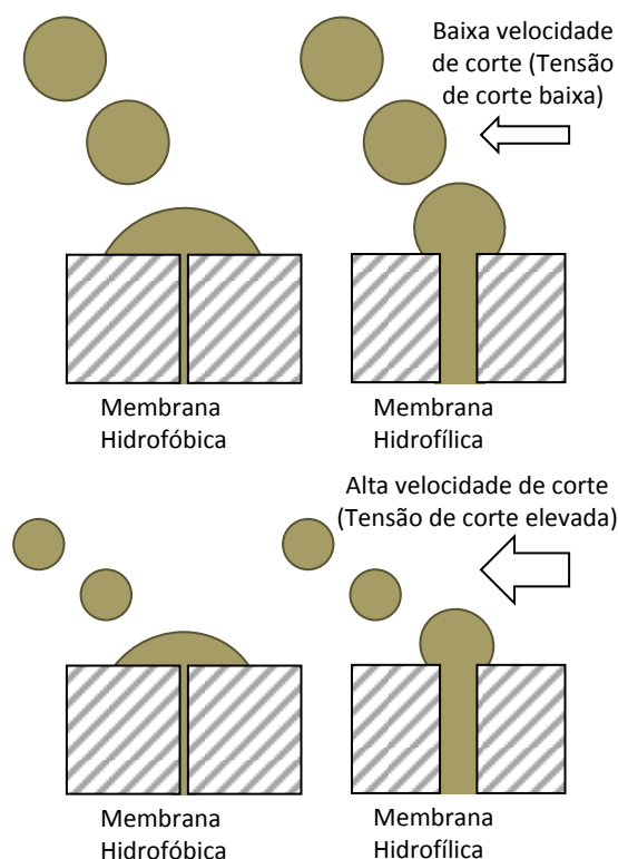
Figura 4.19 Representação esquemática da formação de gotículas de óleo e desprendimento sob alta e baixa velocidade corte na EM utilizando membranas hidrofóbicas e hidrofílicas.
