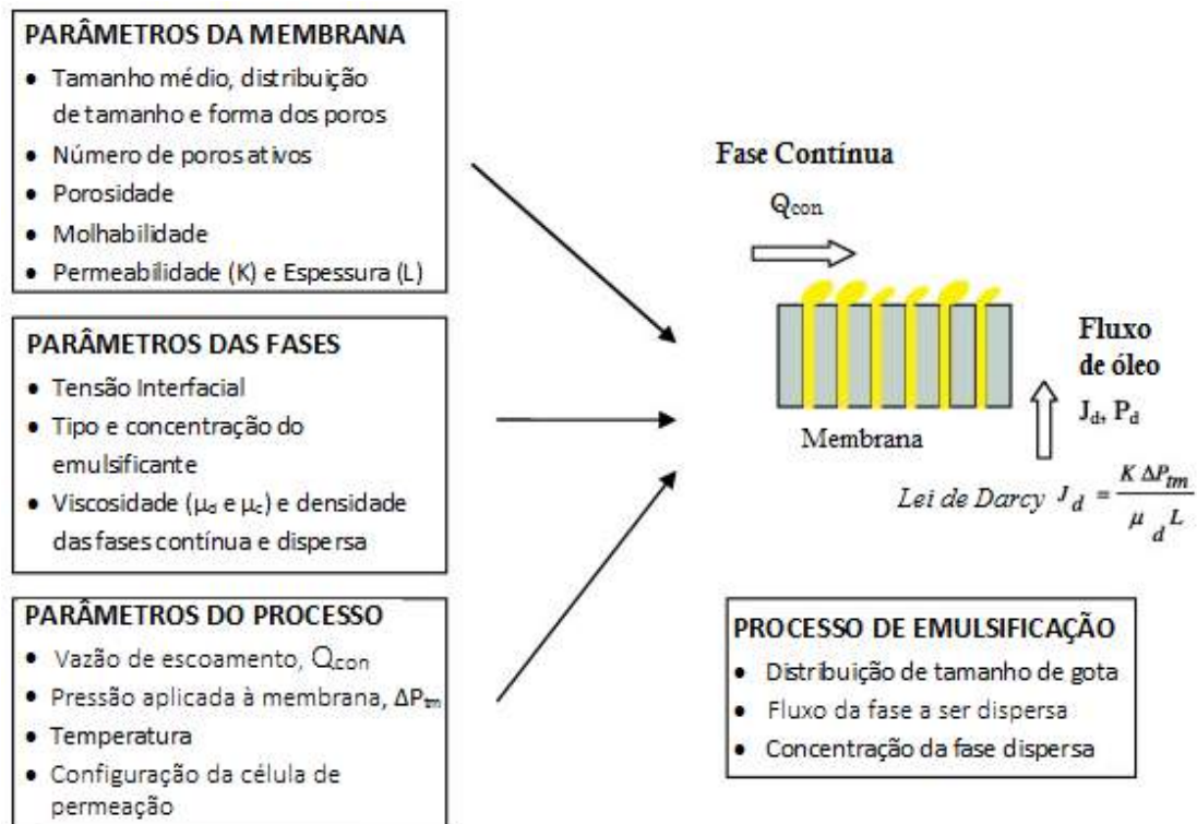
Figura 2.7 Os principais parâmetros que influenciam a emulsificação por membranas (Adaptado de CHARCOSSET, 2009).
