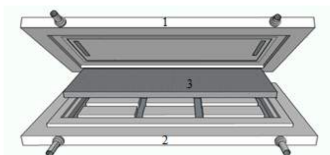
Figura 3.1 Representação esquemática da célula de permeação
