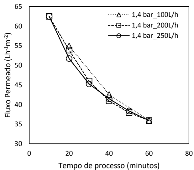
Figura 6. Fluxo permeado ao longo do processo de ME premix operando a 1,4 bar, utilizando a membrana de PVDF e variando-se a vazão de escoamento da fase contínua.
