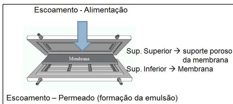
Figura 1. Esquema da montagem da membrana na célula.
