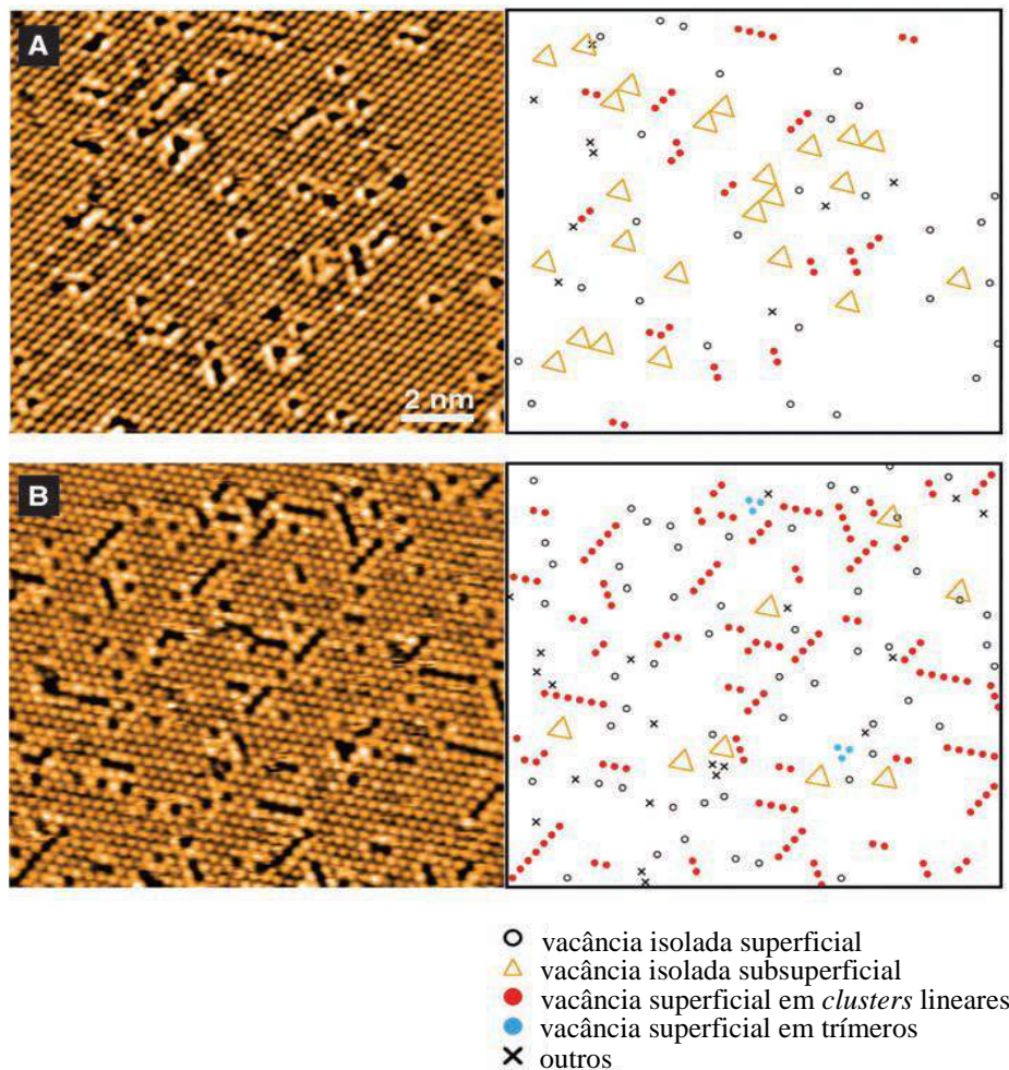
Figura 2.4 - Imagens de STM da superfície CeO 2 (111) obtida após ciclos de sputtering e calcinação a 900 °C por (a) 1 min, (b) 5 min, com as representações correspondentes dos defeitos observados. Condições de análise: -3 V (amostra em relação à ponta), 0,3 nA, 300 °C. Adaptado de ESCH et al. (2005).
