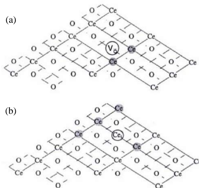
Figura 2.5 - Representação esquemática de: (a) uma vacância de oxigênio (V o ), (b) Ce +4 intersticial (Ce i ) em uma superfície de CeO 2 . Os átomos de Ce circundados representam as posições em que os cátions Ce +4 foram substituídos por espécies M +3 . Fonte: TROVARELLI (2002).
