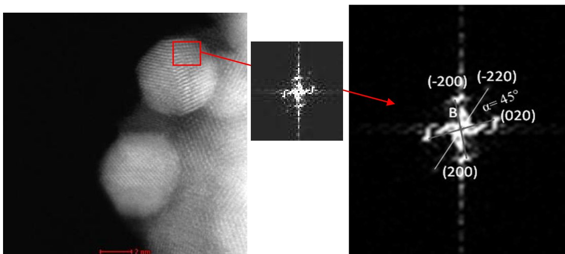
Figura 4.18 – Imagem de campo escuro de alto ângulo (HAADF) para o catalisador \text{Au/Ce}_{0,8}\text{Fe}_{0,2}\text{O}_{2-\delta} e a transformada de Fourier (FFT) de uma região da nanopartícula de ouro com a indicação dos planos difratados. Eixo de zona [001].
