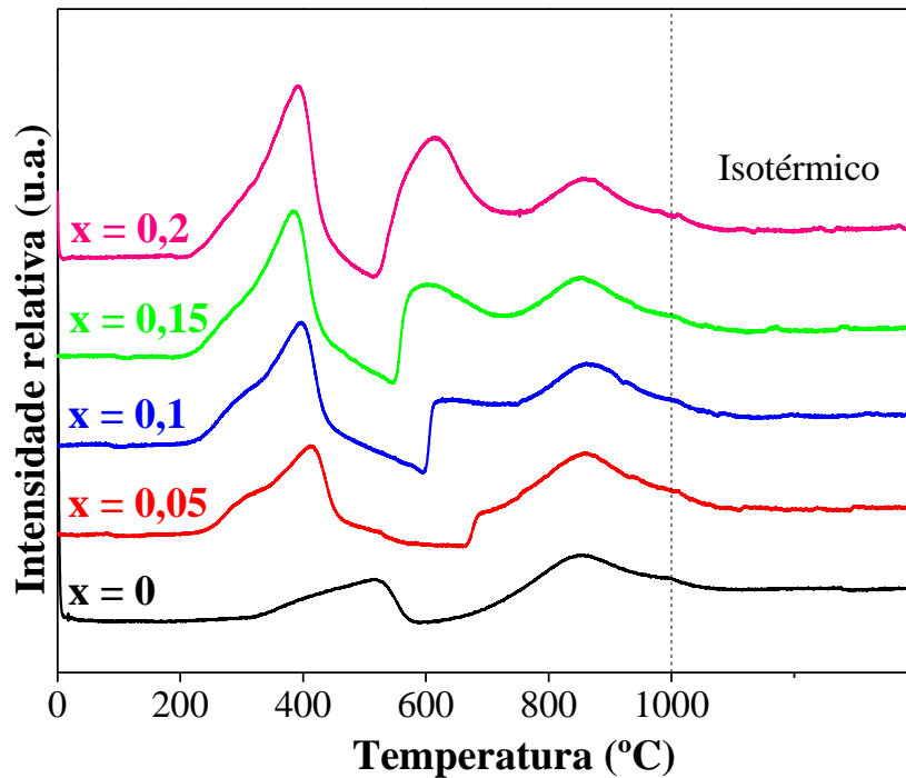
Figura 4.34 – Perfis de TPR do CeO 2 e dos óxidos mistos Ce 1-x Fe x O 2-δ sintetizados pelo método de Pechini e calcinados a 300 °C por 30 minutos e a 500 °C por 5 horas. Condições de redução: T final = 1000 °C, taxa de aquecimento = 10 °C/min, massa de catalisador = 150 mg, vazão da mistura 10% H 2 /He = 30 mL/min.
