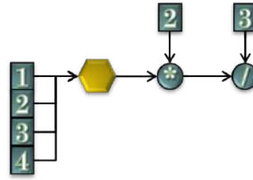
(b) Grafo dataflow stream processando objeto iterável.
