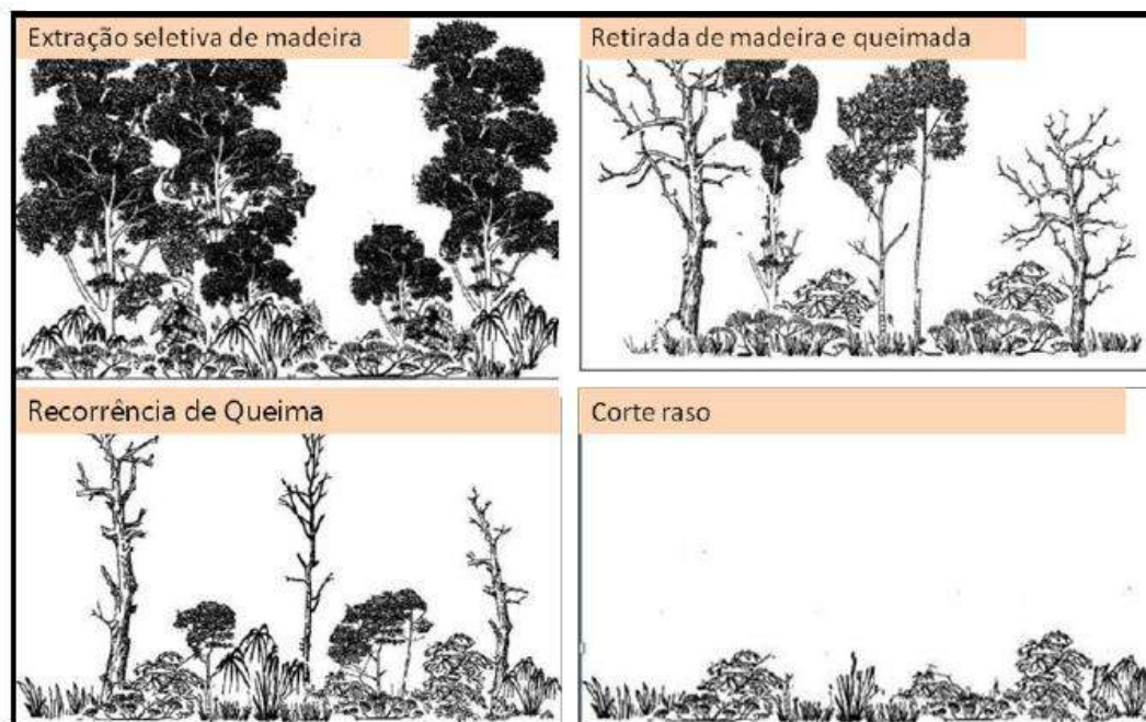
Figura 9 - Etapas do processo de desmatamento
