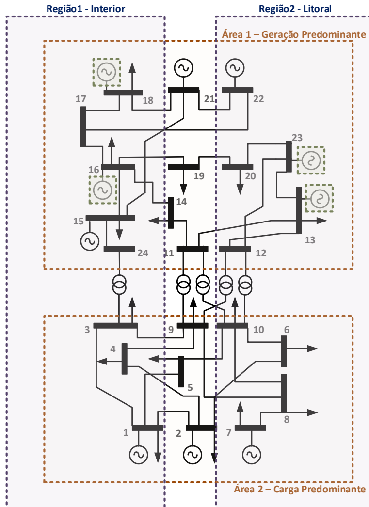
Figura 64 – Divisão do sistema em duas regiões
