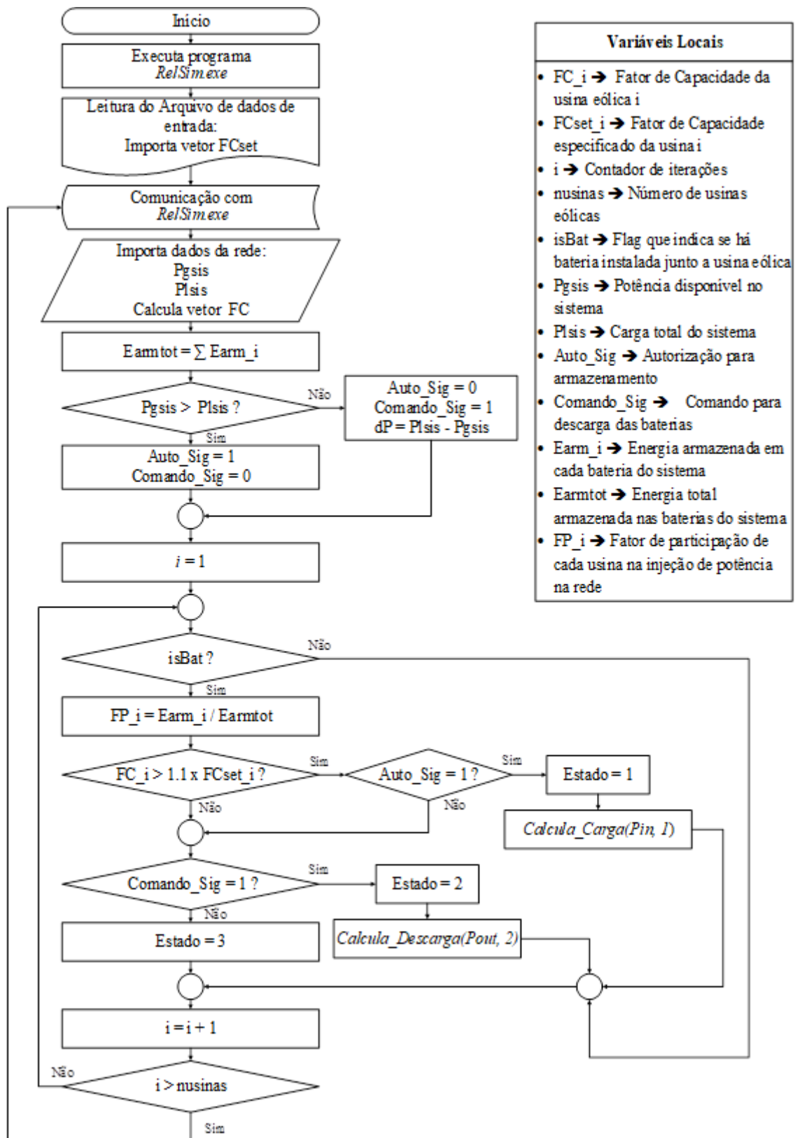
Figura 32 - Fluxograma da Estratégia Operativa das baterias – Objetivo 3
