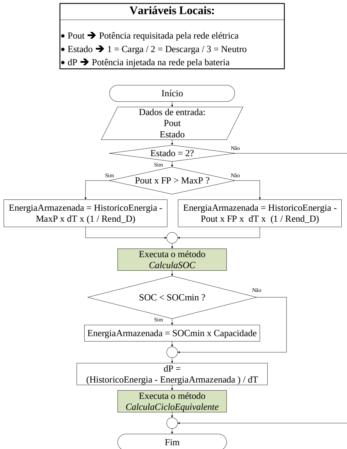
Figura 23 - Fluxograma da Modelagem do processo de descarga da bateria
