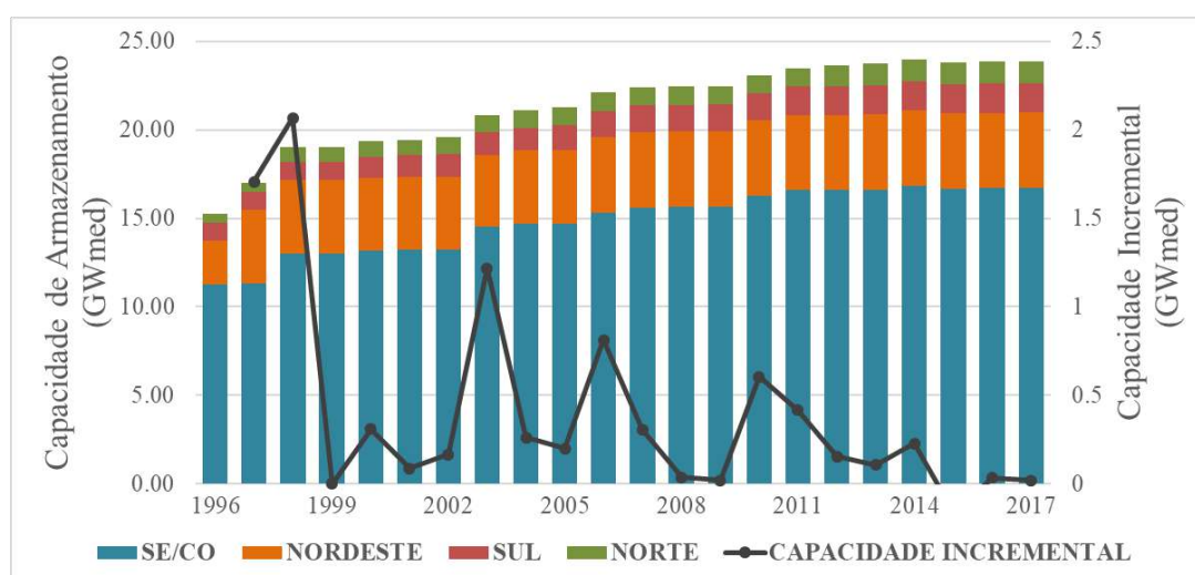
Figura 4 – Evolução da Capacidade de Armazenamento do SIN
