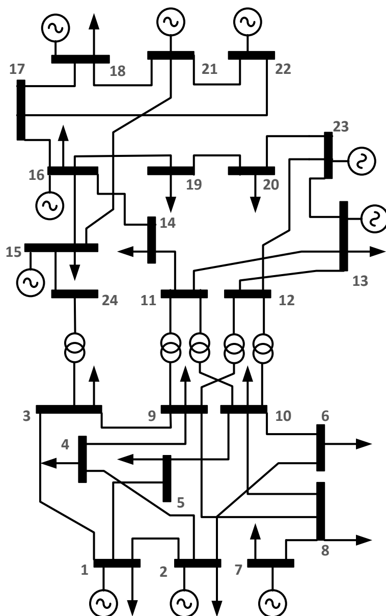
Figura 77 – Sistema RTS
