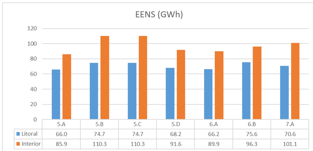
Figura 63 – Valor esperado de energia não suprida nos sistemas 5, 6 e 7
