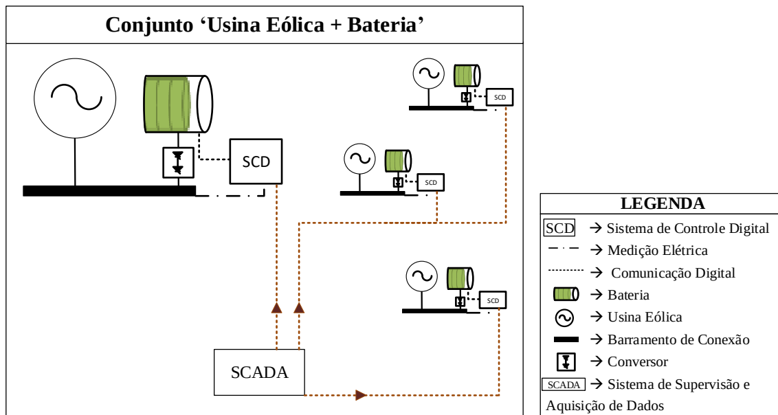
Figura 30 - Esquema simplificado do sistema 'Usina Eólica + Bateria' - Estratégia Operativa 2
