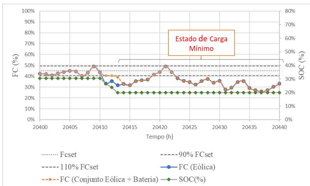
Figura 37 – Sistema 1A: Estado de Carga Mínimo
