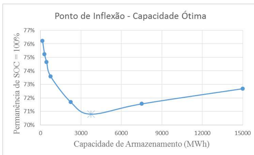
Figura 51 – Permanência da bateria em estado de carga máxima
