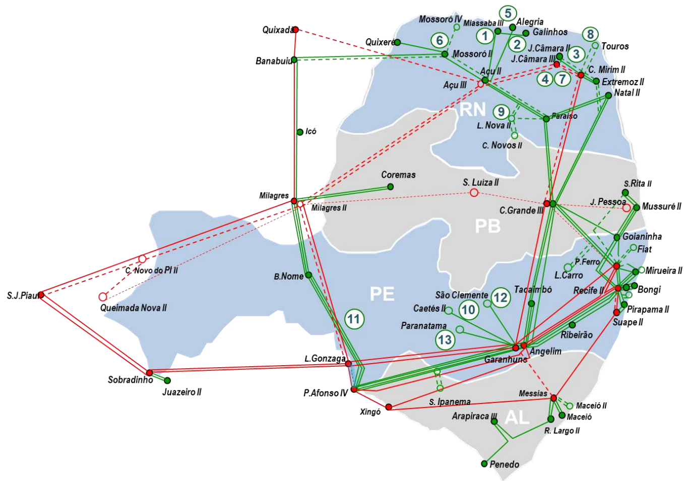
Figura 72 – Área leste do sistema Nordeste
