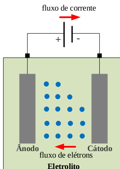
Figura 19 – Carga da bateria
