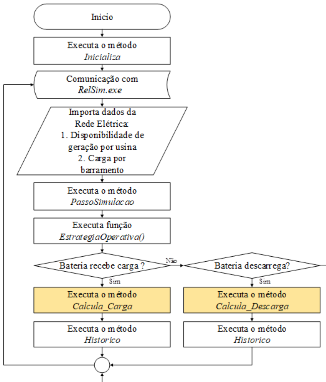
Figura 20 – Fluxograma simplificado de uso da biblioteca Armazenamento.dll
