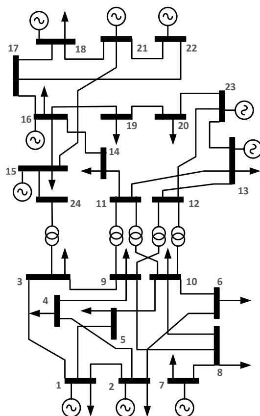
Figura 55 – Sistema RTS – 24 Barras
