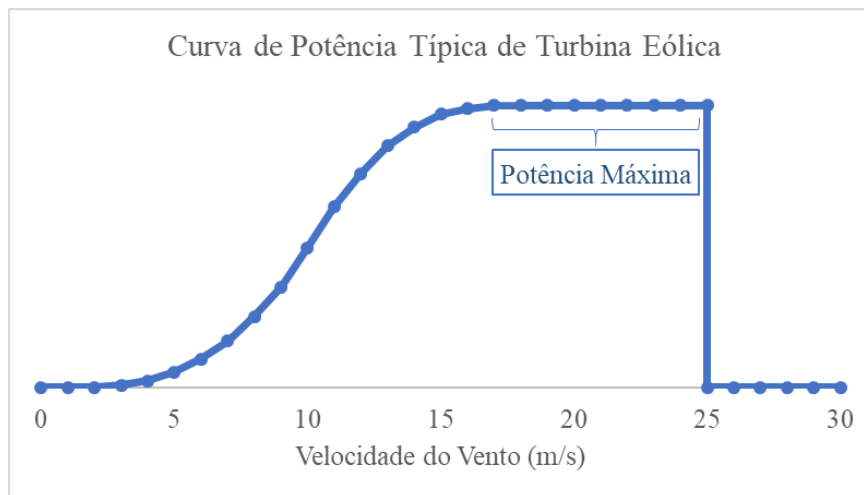
Figura 7 – Curva típica de potência de turbina eólica
