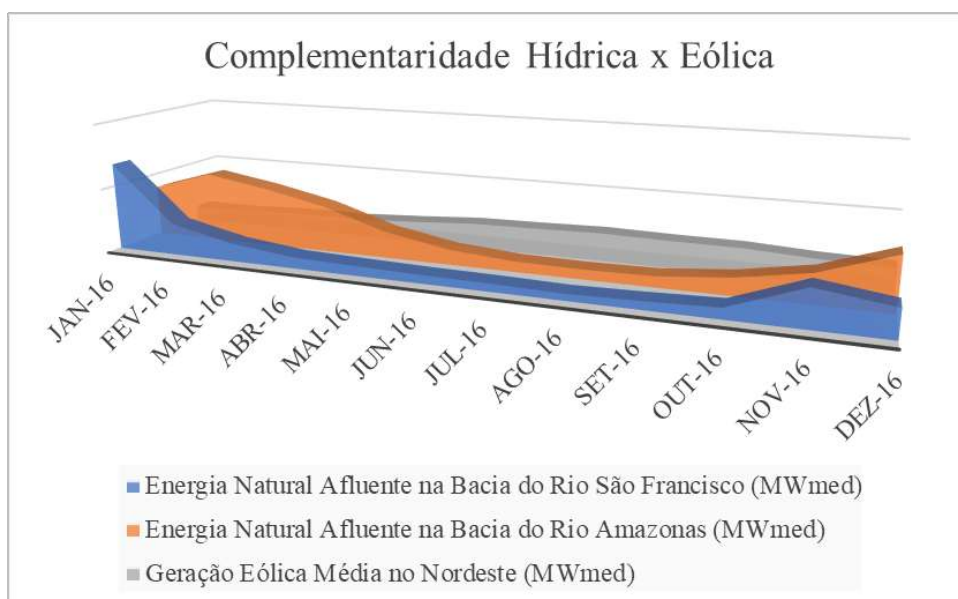
Figura 12 – Curvas de geração eólica no Nordeste e energia natural afluente no subsistema N/NE
