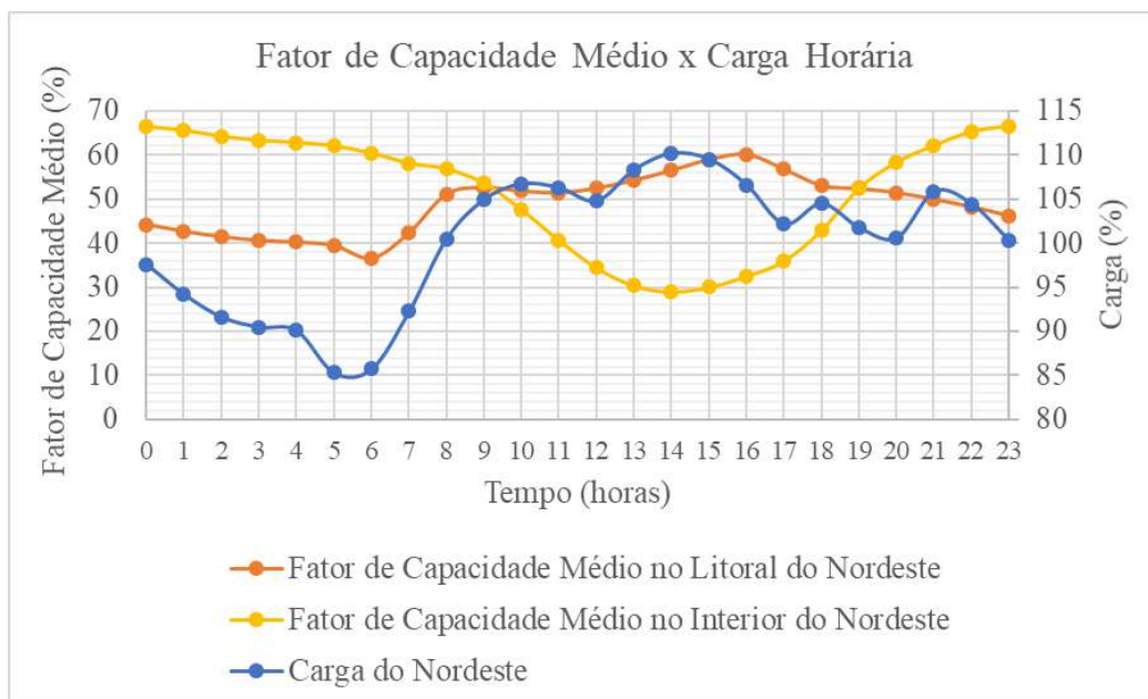
Figura 10 – Perfil diário de Carga x Geração Eólica no Nordeste
