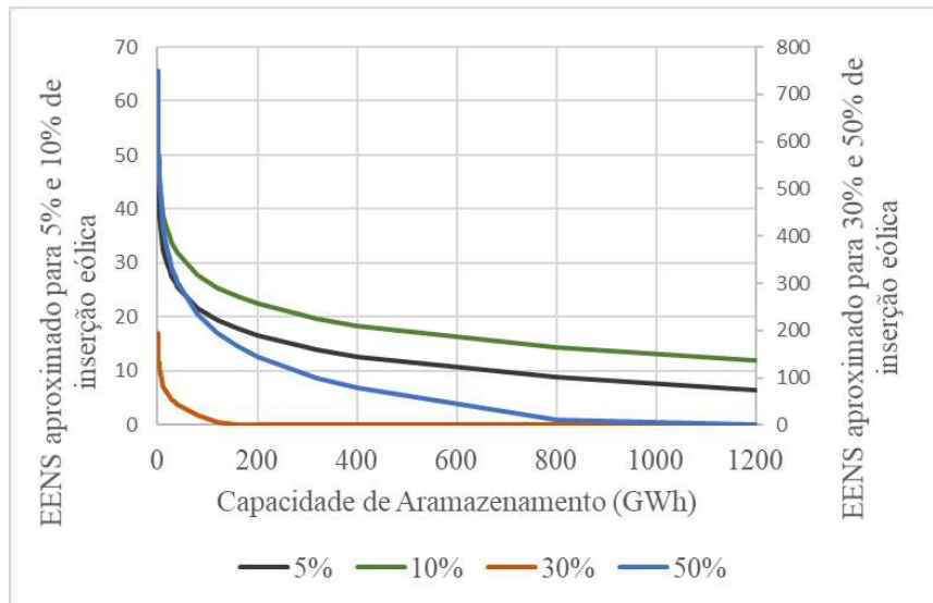
Figura 59 – Extrapolação do resultado dos testes a partir das curvas de tendência
