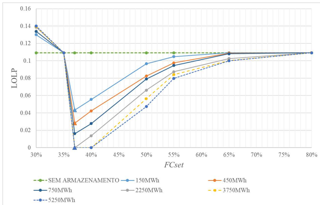
Figura 47 – Variação do FCset e Capacidade de Armazenamento no Sistema 2A
