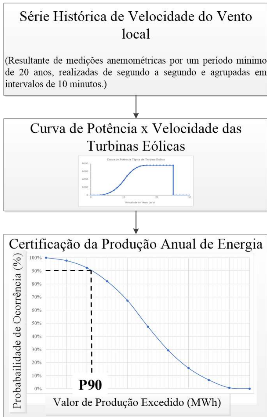
Figura 15 – Fluxograma simplificado para cálculo da Garantia Física de usinas Eólicas
