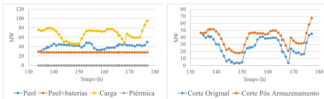
Figura 48 – Redução da Confiabilidade do sistema utilizando a Estratégia Operativa 1
