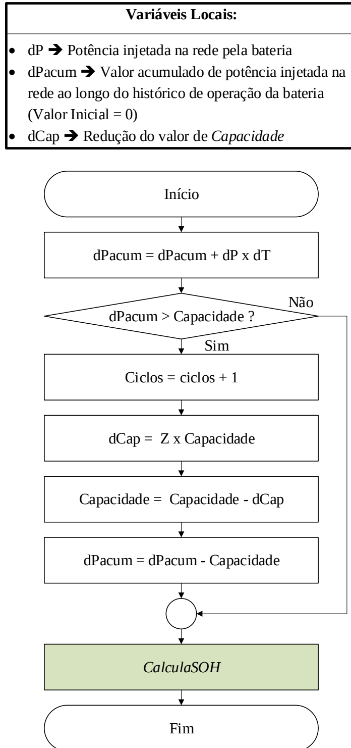
Figura 25 – Fluxograma da modelagem do sistema de gerenciamento e proteção (Parte 2 / 3)
