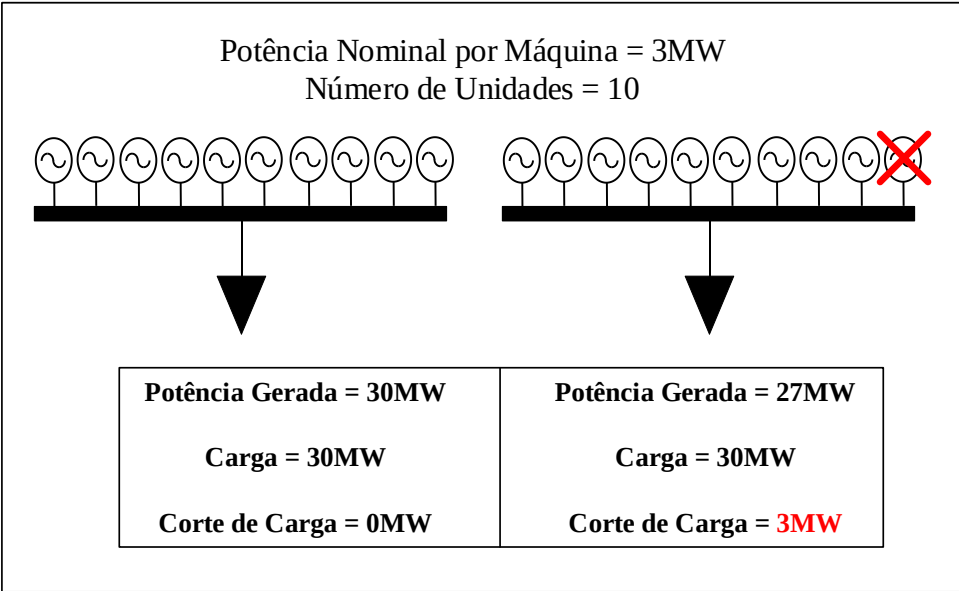
Figura 9 - Confiabilidade no suprimento à demanda: Sistema fictício 2
