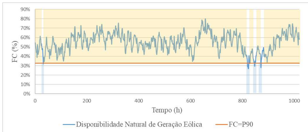
Figura 44 - Distribuição de Fator de Capacidade em torno de P90
