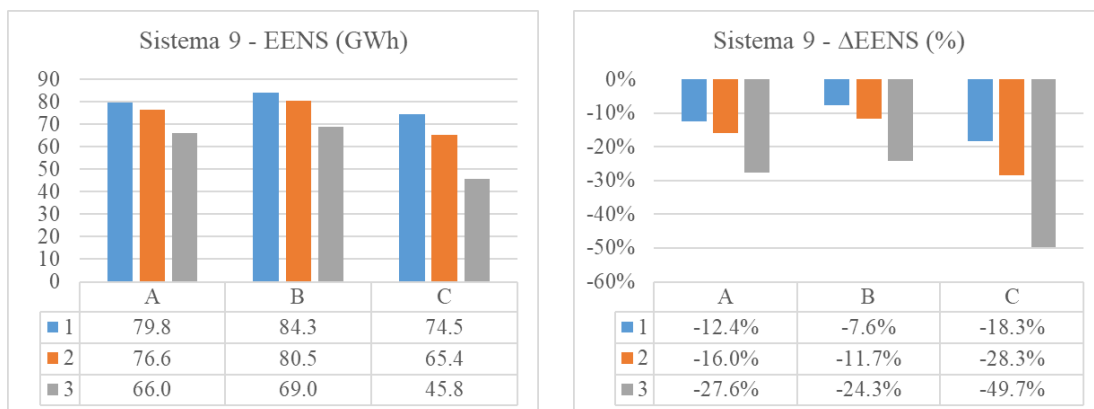
Figura 67 – Resultados de testes com o Sistema 9
