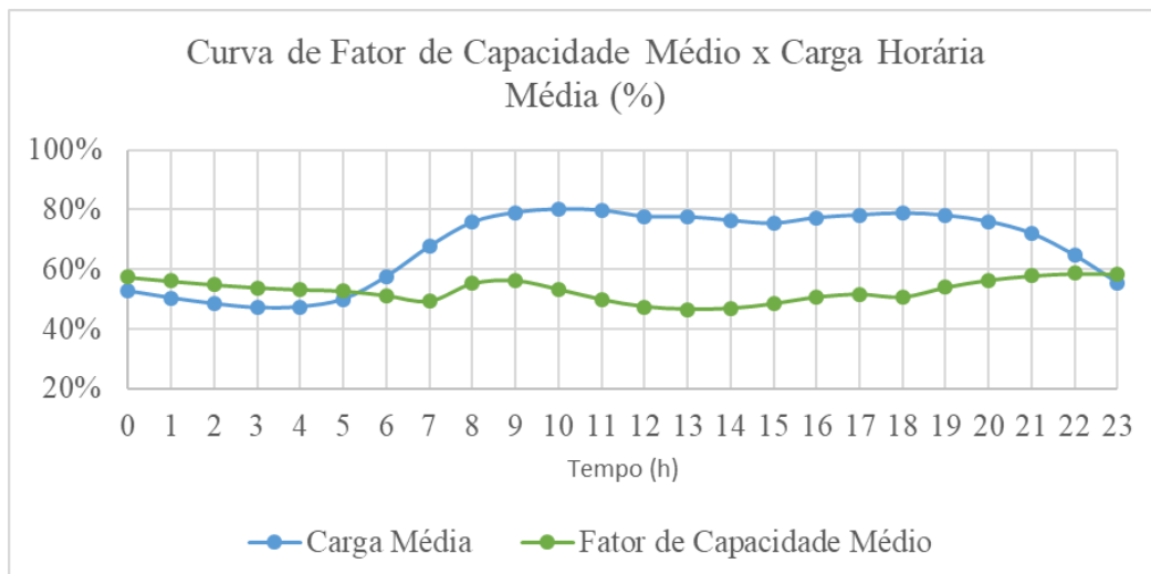
Figura 34 – Curva de carga média e fator de capacidade médio utilizados no Sistema 1A
