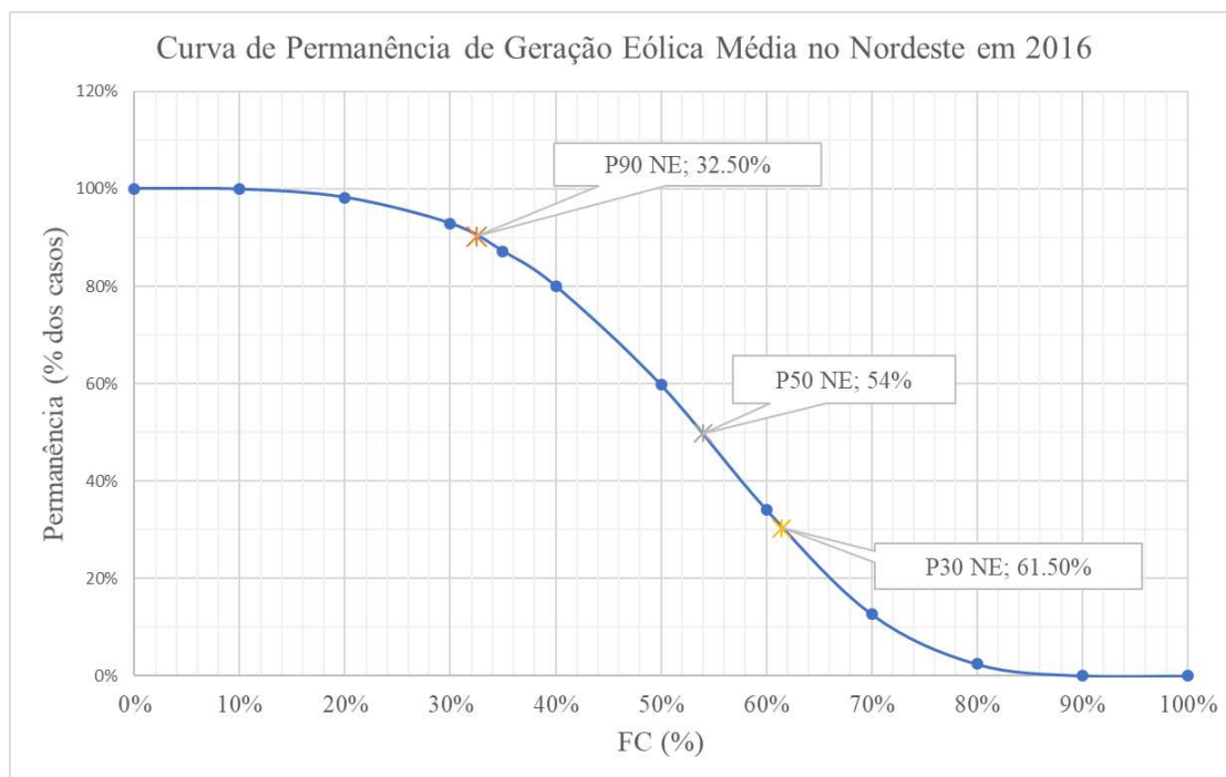
Figura 41 – Curva de permanência da geração eólica média no Nordeste em 2016
