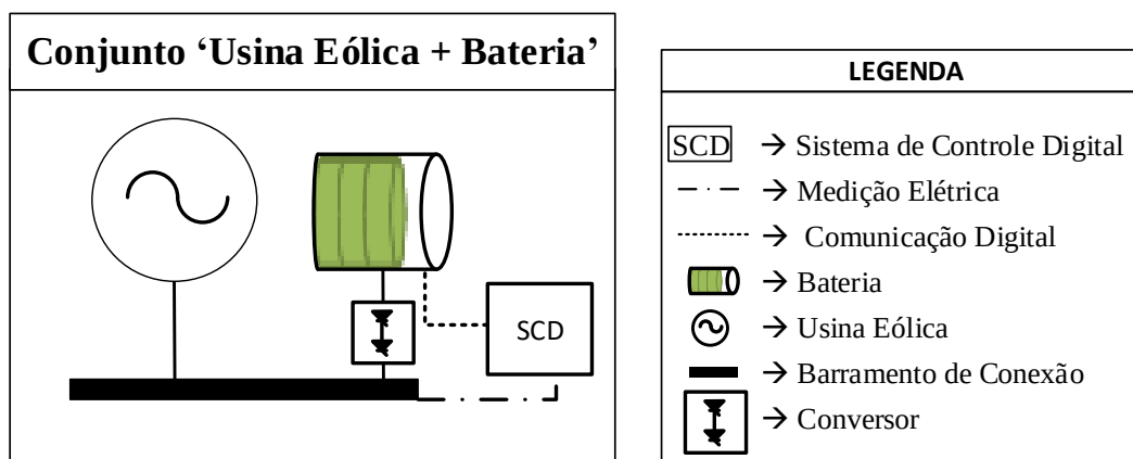
Figura 28 – Esquema simplificado do sistema ‘Usina Eólica + Bateria’ – Estratégia Operativa 1
