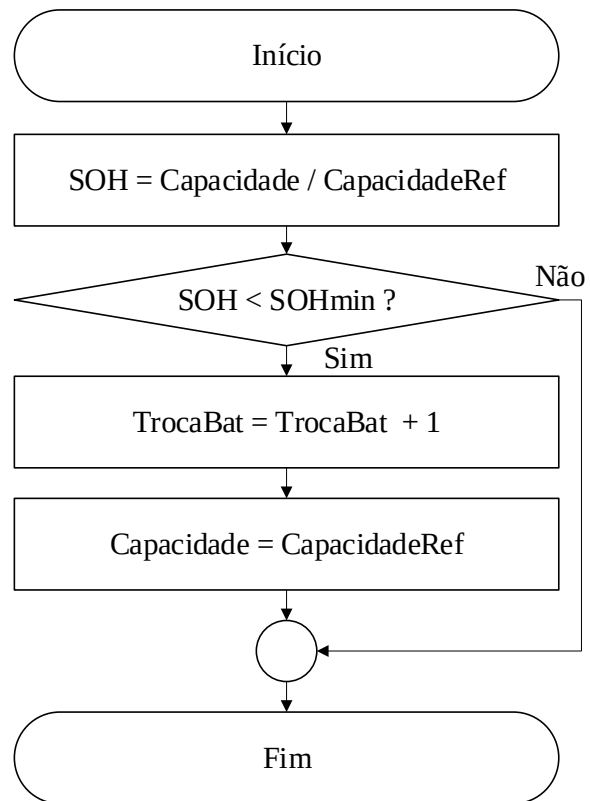
Figura 26 - Fluxograma da modelagem do sistema de gerenciamento e proteção (Parte 3 / 3)
