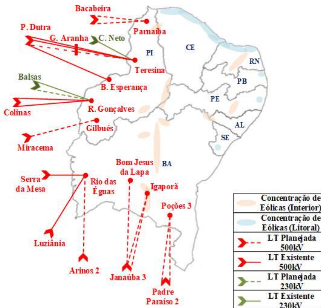
Figura 69 – Detalhamento do sistema de transmissão planejado para 2026
