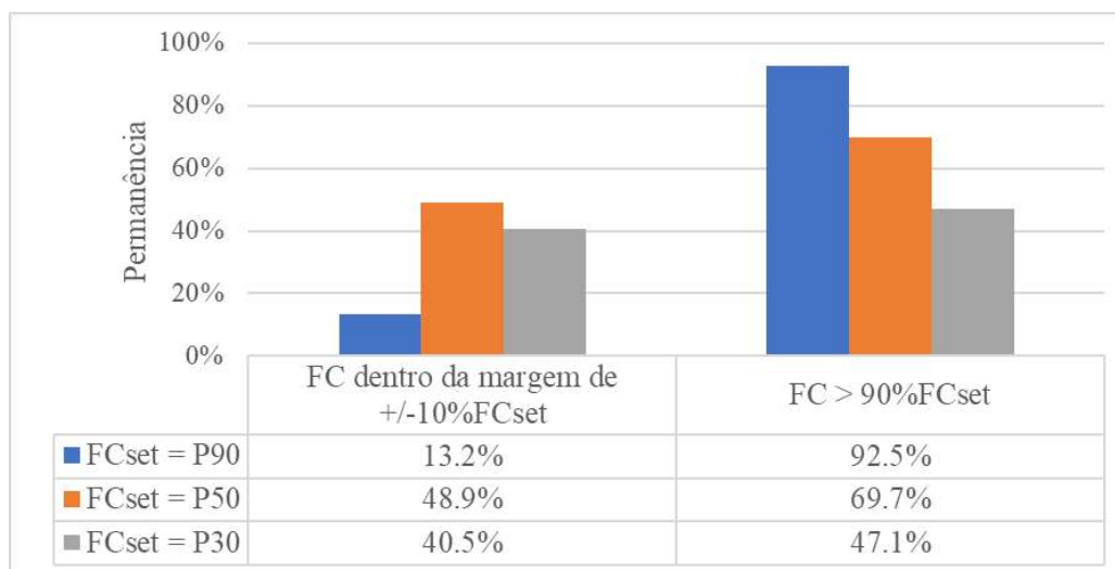
Figura 42 – Sistemas 1B, 1C e 1D – Permanência do Fator de Capacidade
