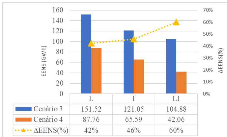
Figura 75 – Valor esperado de energia não suprida
