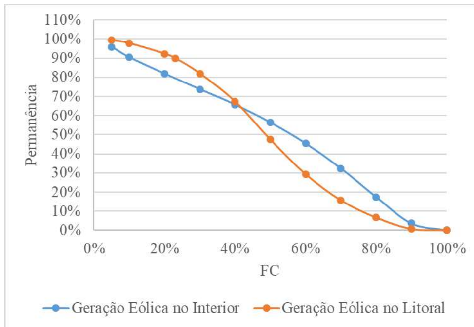
Figura 53 – Curva de permanência dos ventos de cada região ao longo de um ano de medição
