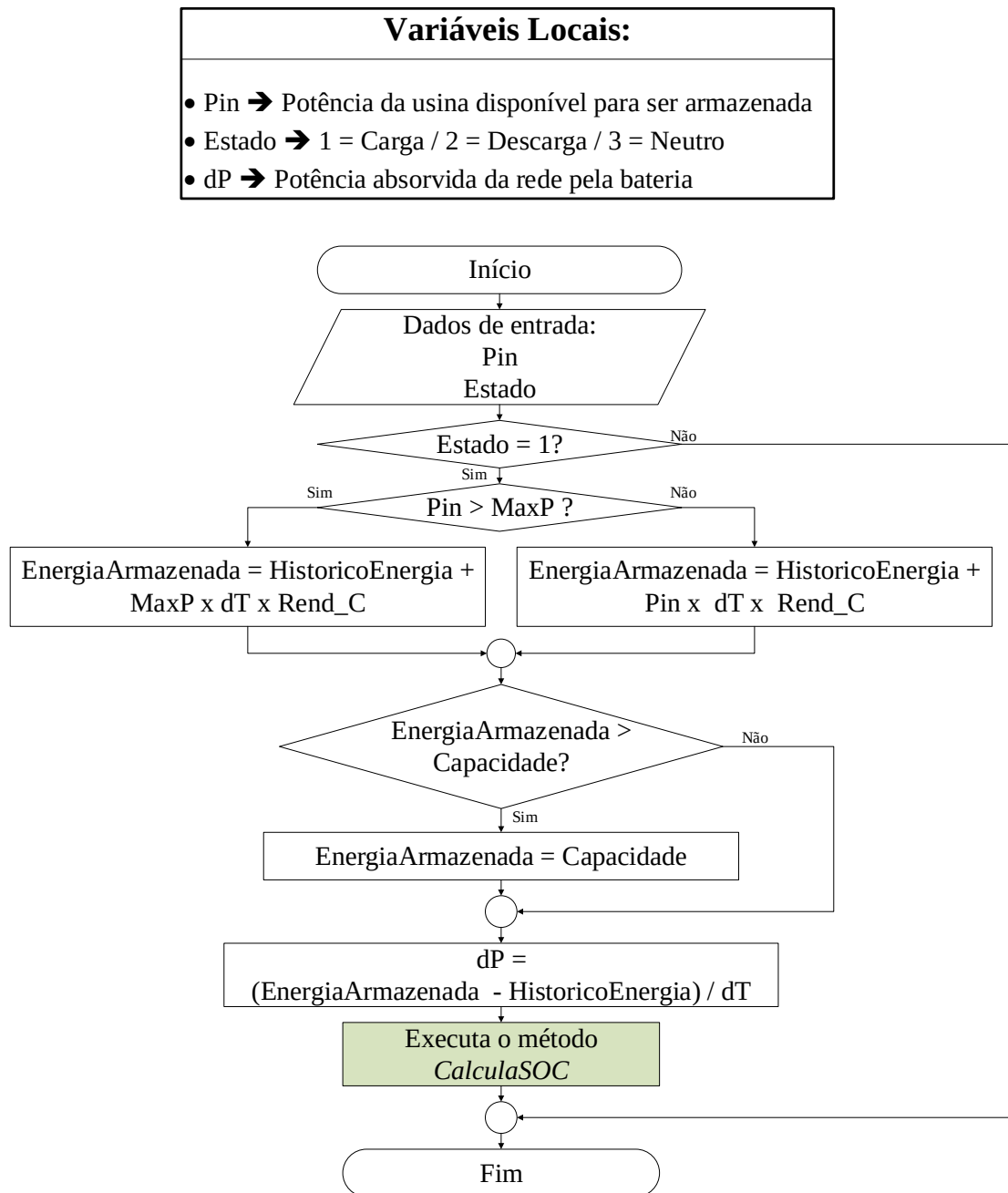
Figura 22 – Fluxograma da Modelagem do processo de carga da bateria
