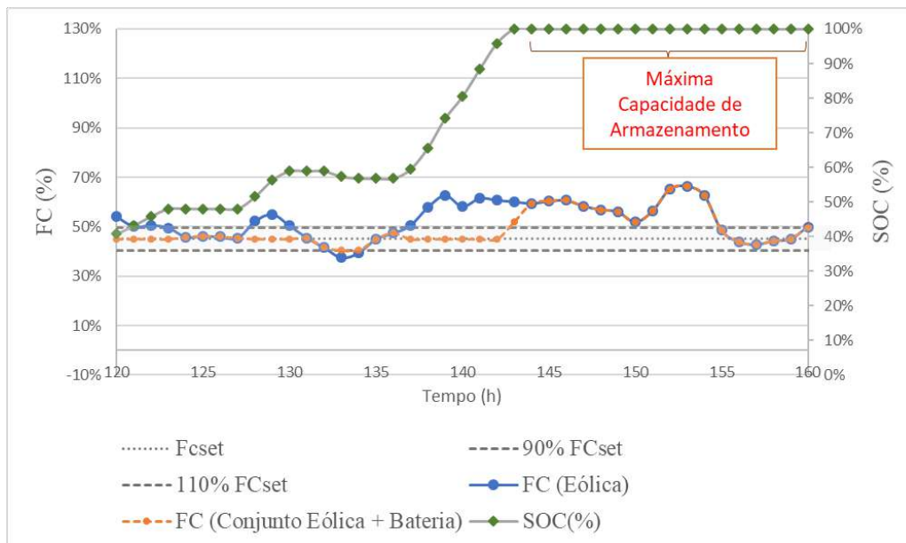
Figura 36 – Sistema 1A: Limite da Capacidade de Armazenamento
