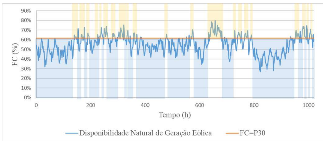
Figura 45 - Distribuição de Fator de Capacidade em torno de P30
