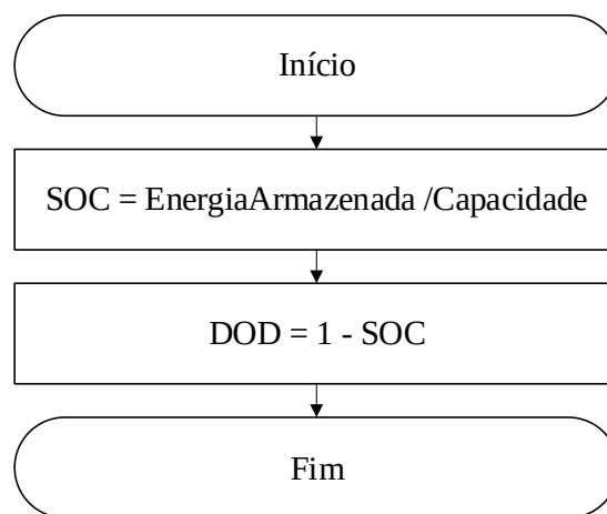
Figura 24 – Fluxograma da modelagem do sistema de gerenciamento e proteção (Parte 1 / 3)
