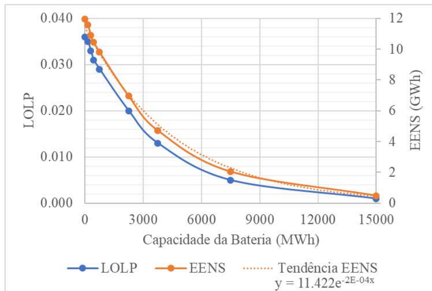
Figura 54 – Tendência exponencial de redução dos índices com o aumento da capacidade de armazenamento
