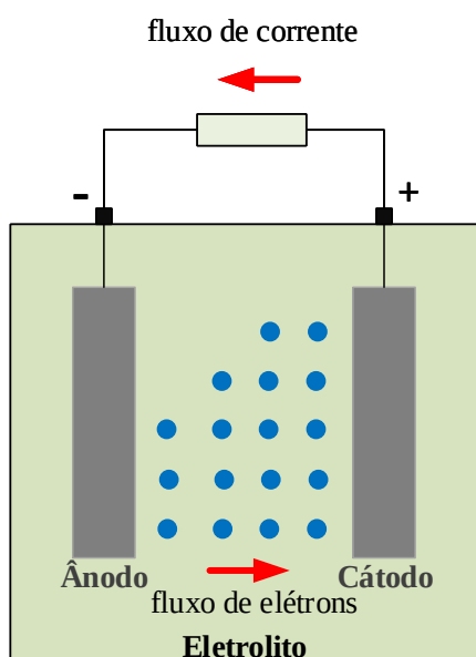
Figura 18 – Descarga da Bateria
