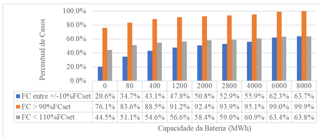
Figura 40 – Avaliação do aumento da capacidade de baterias
