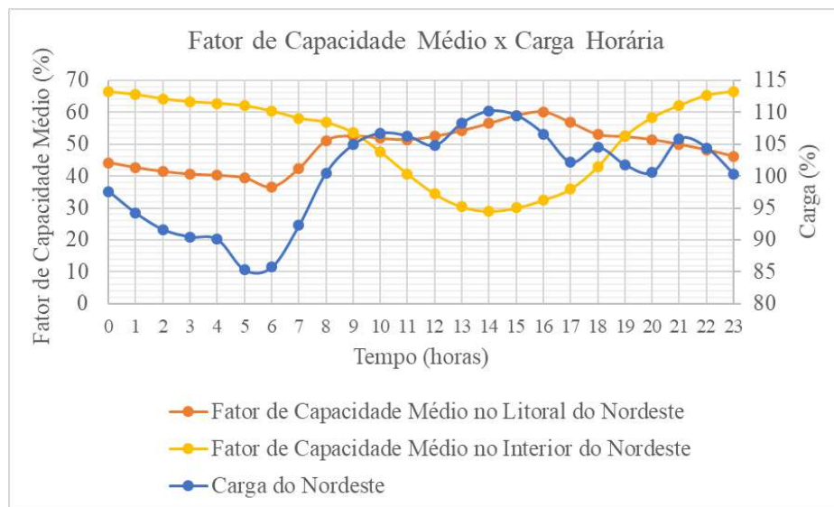
Figura 74 – Fator de Capacidade no Litoral e no Interior e Curva de Carga Horária Média
