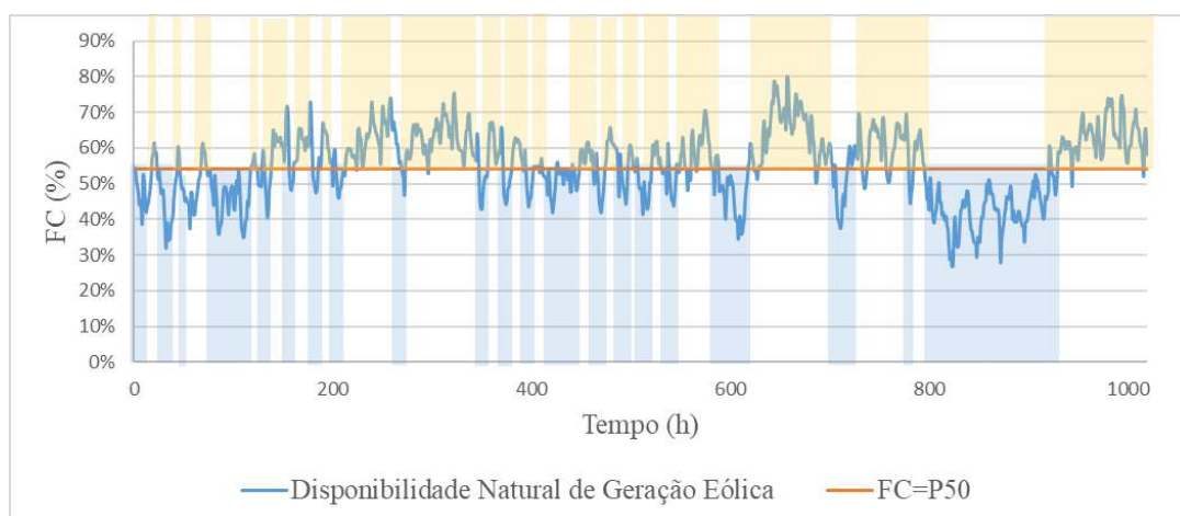
Figura 43 – Distribuição de Fator de Capacidade em torno de P50
