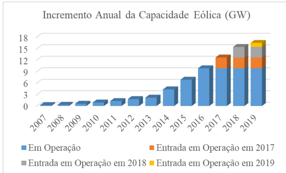
Figura 3 – Projeção da Capacidade Instalada de Geração Eólica até 2019
