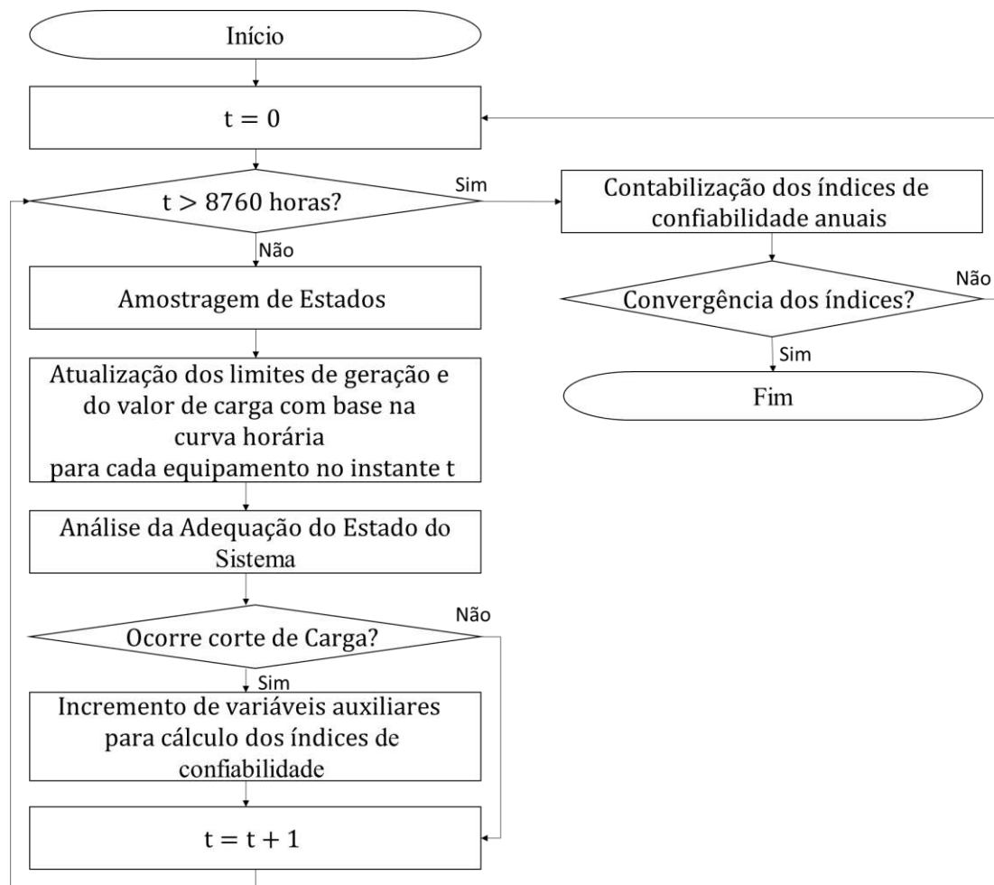
Figura 14 – Fluxograma simplificado da SMC
