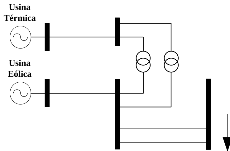
Figura 46 – Sistema 5 barras
