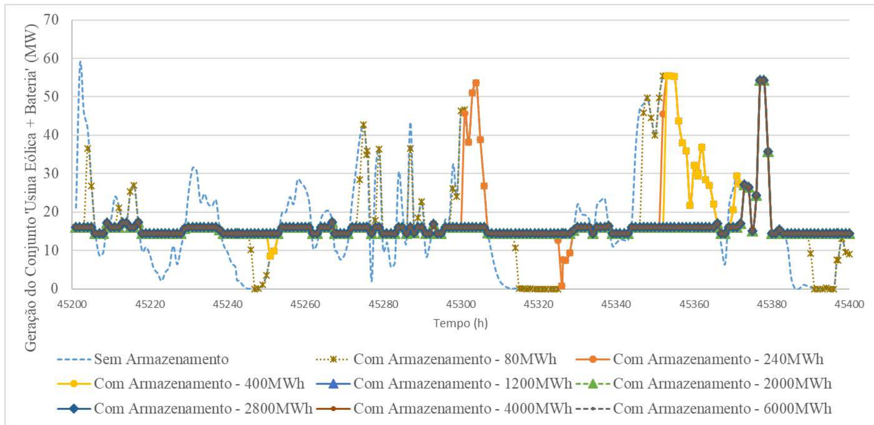
Figura 39 – Sistema 1A: Geração do Conjunto 'Usina Eólica + Baterias' a medida que se aumenta a capacidade de armazenamento
