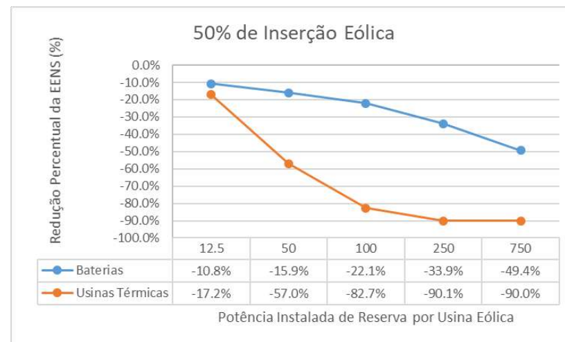
Figura 60 – Comparação do uso de Baterias x Usinas Térmicas para composição da reserva
