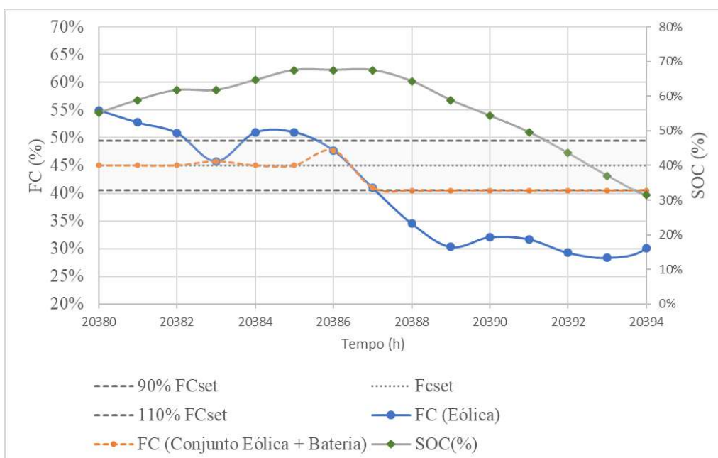
Figura 35 – Sistema 1A: Redução da intermitência da geração eólica
