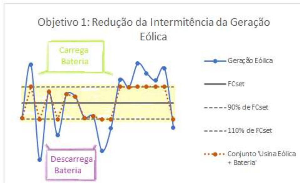
Figura 27 – Estratégia Operativa das baterias – Objetivo 1
