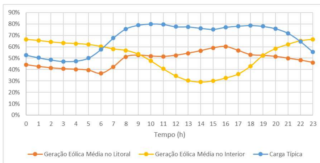
Figura 52 – Curva de carga e curvas de disponibilidade eólica média por região no Nordeste ao longo de um ano de medição
