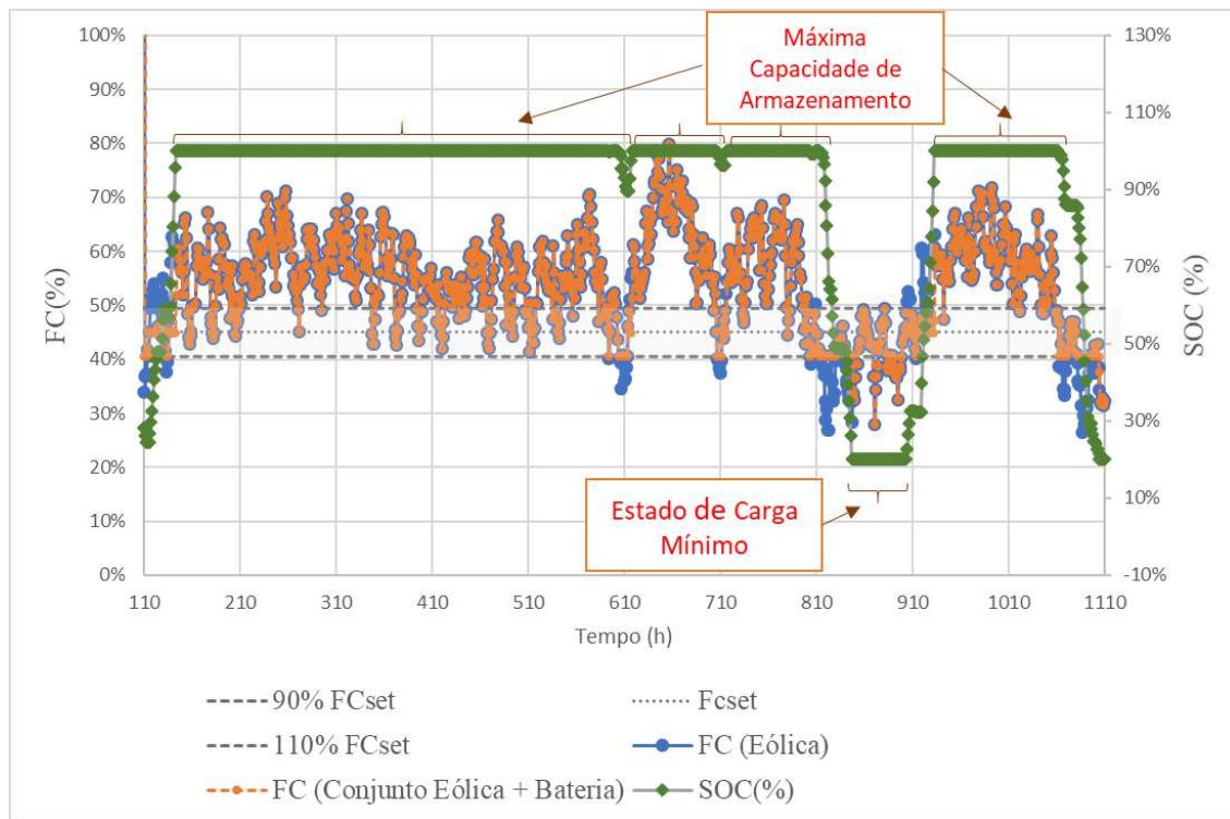
Figura 38 – Sistema 1A: Baixa Capacidade de Modulação da Bateria
