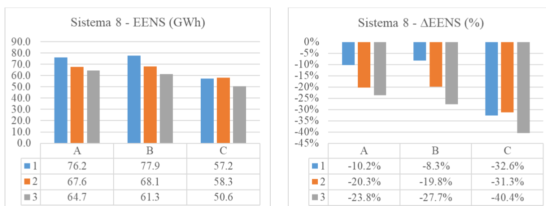
Figura 66 – Resultados de testes com o Sistema 8
