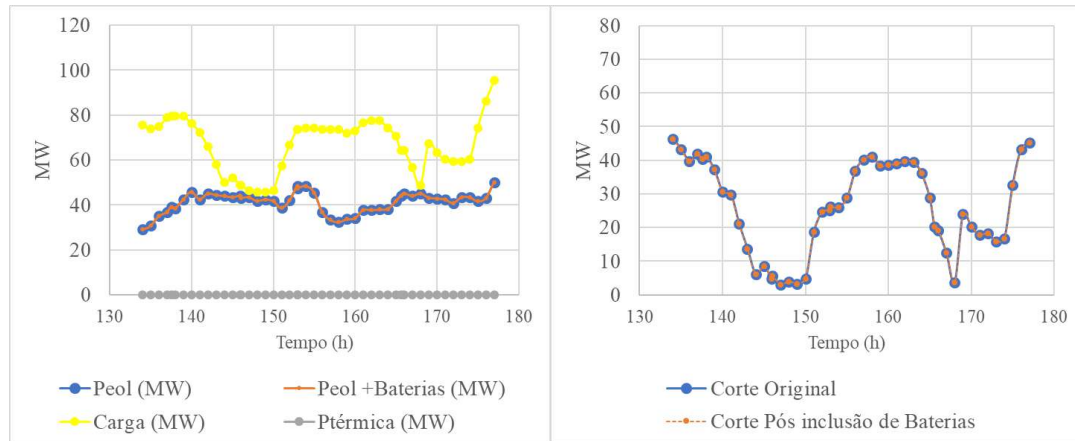
Figura 50 – Eliminação do problema de redução da confiabilidade na Estratégia Operativa 2
