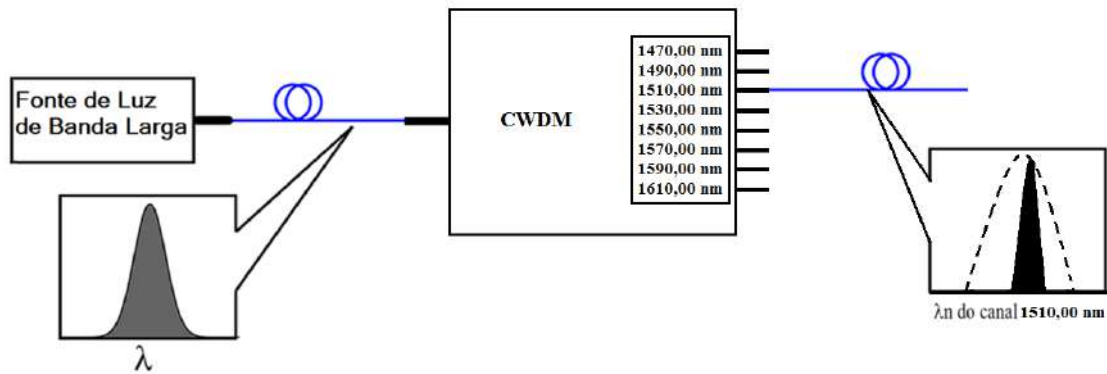
Figura 2.2.2 – Diagrama do sistema CWDM.
