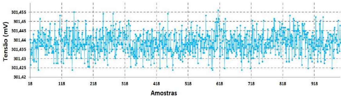
Figura 4.6.2 – Gráfico de ruído com canais A/D curto circuitados do microcontrolador, dados retirados do software desenvolvido.
