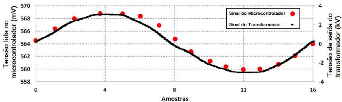
Figura 4.11.8 – Gráfico da relação do sinal de aquisição pelo interrogador e osciloscópio.
