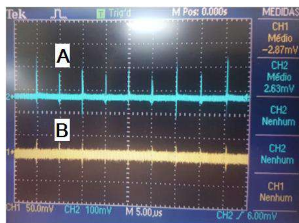
Figura 4.4.10 – Análise DC, saída (A) A0+ = 2,63 \text{ mV} (escala de 100 mV) e saída (B) A0- = -2,87 \text{ mV} (escala de 50 mV).
