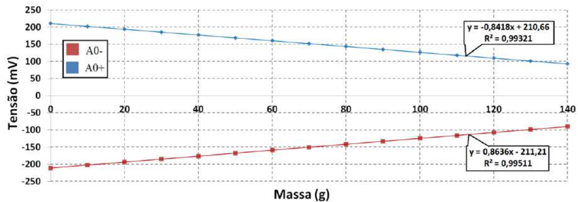
Figura 4.5.2 – Gráfico de calibração por deformação mecânica utilizando fotodetector projetado.
