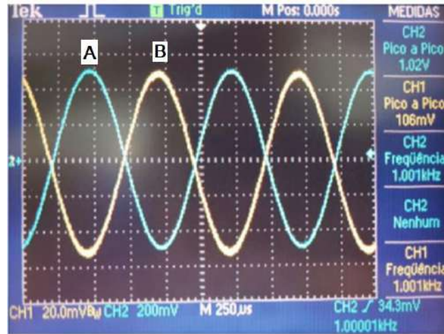
Figura 4.4.2 – Sinal amplificado (A) com frequência de 1 kHz do canal A0+ e sinal do gerador de sinais (B) (Escala do sinal B 20 mV e do sinal A 200 mV).
