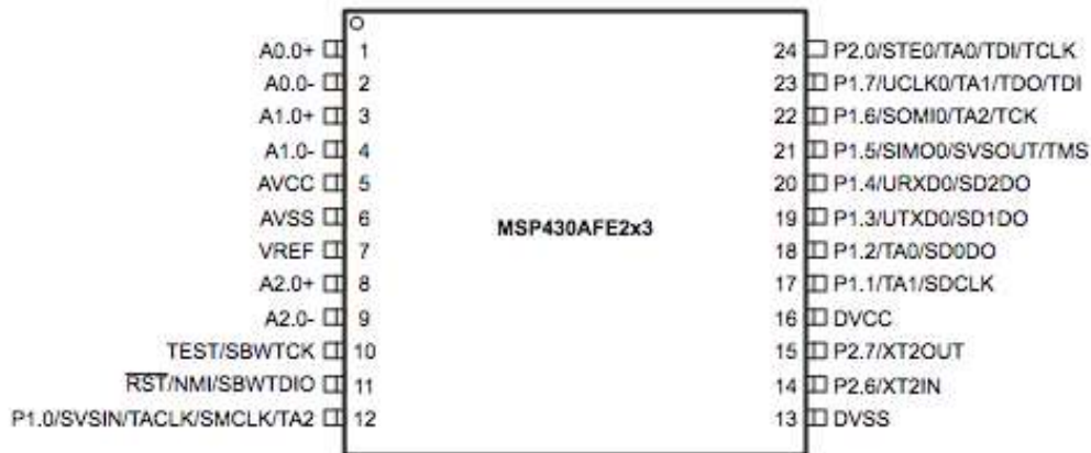
Figura 3.4.1 – Microcontrolador MSP430AFE253.
