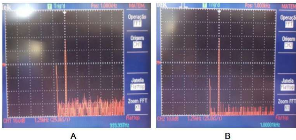
Figura 4.4.5 – FFT do sinal sem capacitor imagem A e com capacitor imagem B com frequência de 1 kHz do canal A0- (Escala 10 dB).
