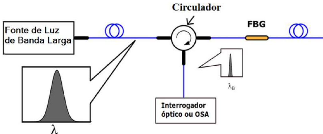
Figura 2.1.4 – Diagrama do circuito óptico para caracterização de uma FBG.
