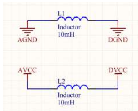
Figura 3.2.2 – Circuito de acoplamento.
