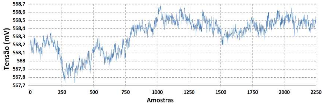
Figura 4.8.1 – Curva de ruído de aquisição de sinal óptico.
