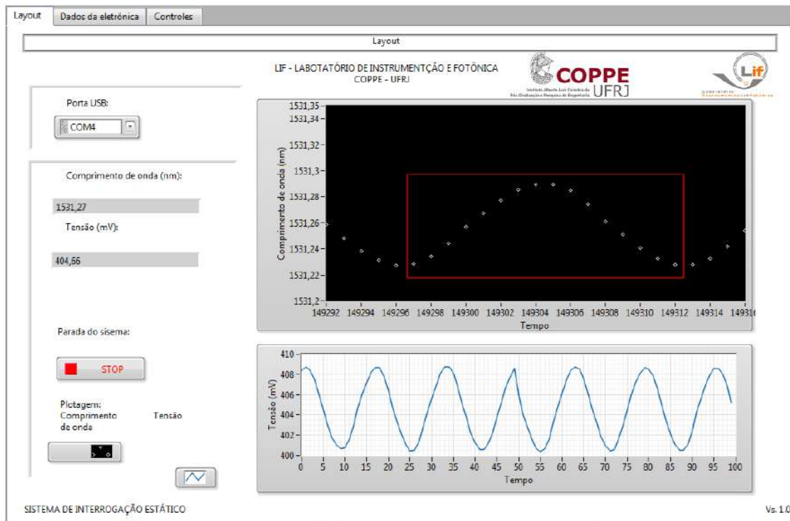
Figura 4.11.7 – Layout da interface LabVIEW®, operando testes com tensão ac 2,12 kVrms.
