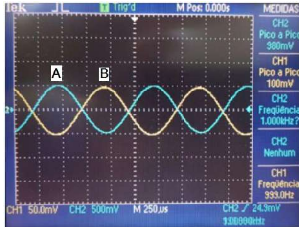
Figura 4.4.4 – Sinal amplificado (A) com frequência de 1 kHz do canal A0- e sinal do gerador de sinais (B) (Escala do sinal B 50 mV e do sinal A 500 mV).
