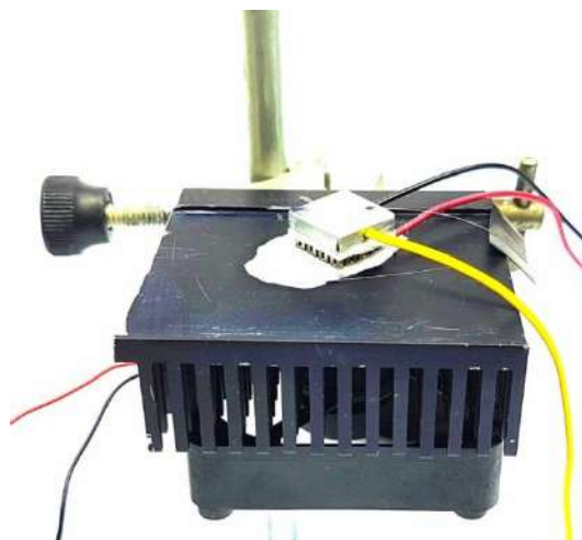
Figura 4.11.3 – Arranjo utilizado para realizar a calibração por temperatura via peltier.
