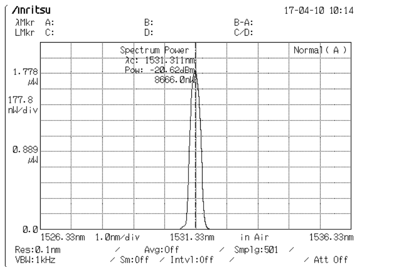
Figura 2.3.1 – Espectro de reflexão da FBG pelo OSA MS9710C.
