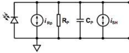
Figura 4.2.1 – Modelo do fotodiodo.
