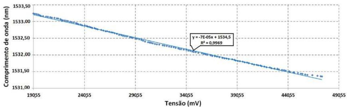
Figura 4.11.2 – Gráfico de calibração por deformação mecânica - \lambda_B x tensão.
