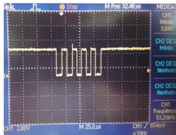
Figura 4.9.2 – Aquisição do carácter “U” (tabela ASCII) pelo osciloscópio.
