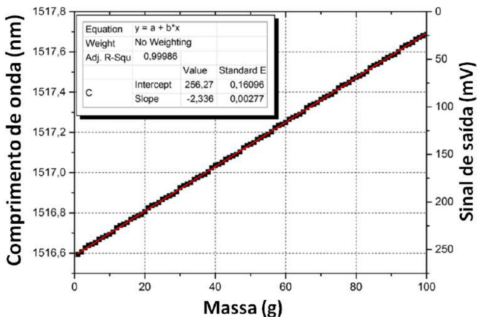
Figura 4.12.6 – Curva de calibração para a FBG centrada em 1516,6 nm, modulada pelo filtro de borda CWDM.
