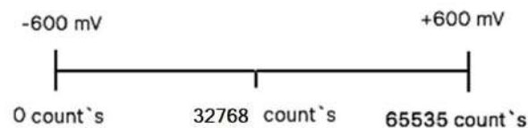
Figura 3.4.2 – Escala de conversão tensão x counts .
