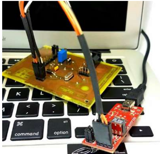
Figura 4.9.1 - Interface isolada RS-485/USB de comunicação com o computador em configuração operante.
