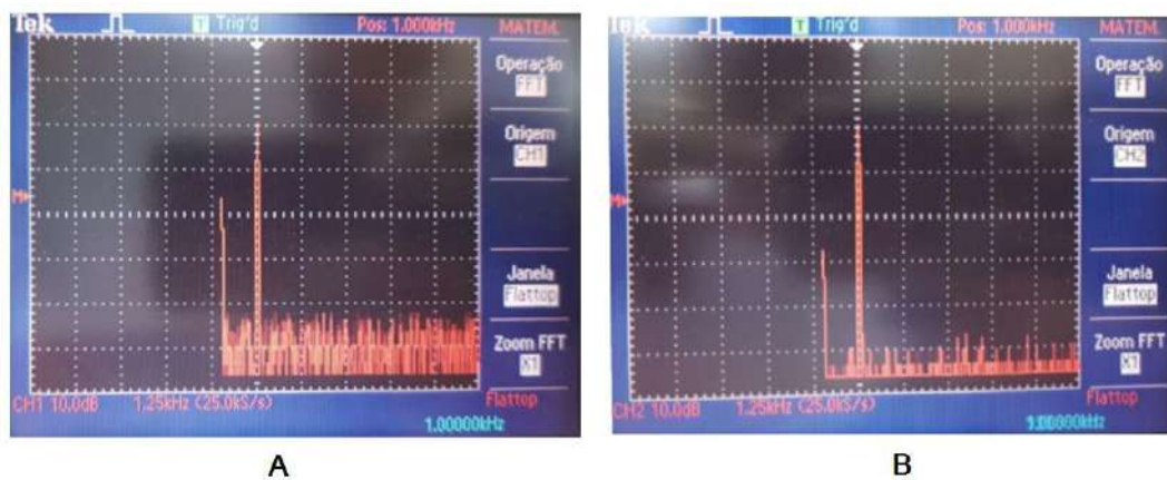
Figura 4.4.3 – A transformada rápida de Fourier FFT do sinal sem capacitor imagem A e com capacitor imagem B com frequência de 1 kHz do canal A0+ (Escala 10 dB).
