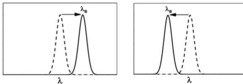
Figura 2.1.3 – Efeito da deformação mecânica longitudinal e/ou variação de temperatura no \lambda_B de uma FBG [8].
