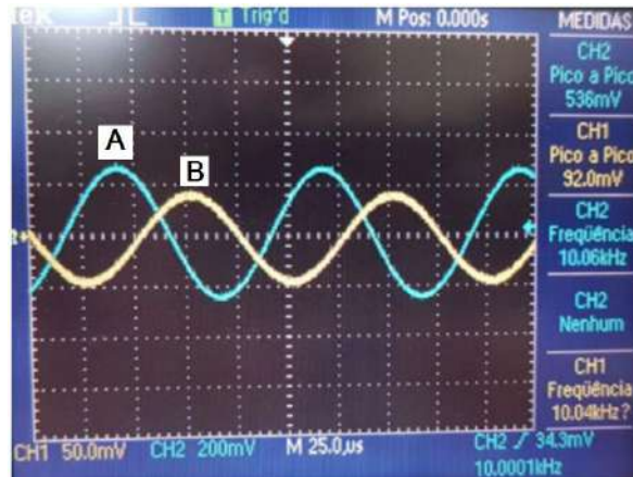
Figura 4.4.8 – Sinal A0- (A), defasado e atenuado em relação ao sinal de entrada (B) do circuito e atenuado em relação ao obtido com menor frequência (Escala do sinal de entrada 50 mV e do sinal de saída 200 mV).
