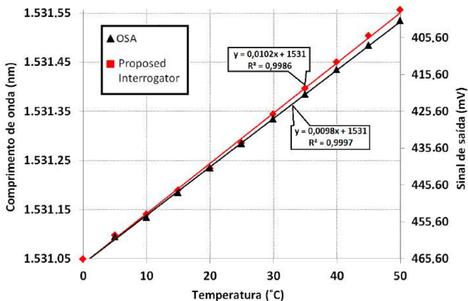
Figura 4.11.5 – Gráfico do experimento no OSA e no sistema de interrogação desenvolvido.
