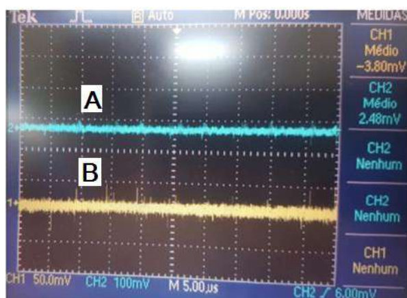
Figura 4.4.11 – Análise DC, saída (A) A0+ = 2,48 \text{ mV} (escala de 100 mV) e saída (B) A0- = -3,8 \text{ mV} (escala 50 mV) com capacitor de 100 nF implementado nas saídas diferenciais.
