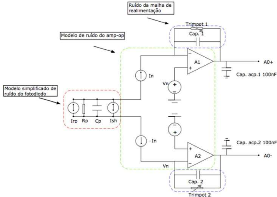
Figura 4.4.1 – Diagrama para análise de ruído do amplificador de transimpedância.
