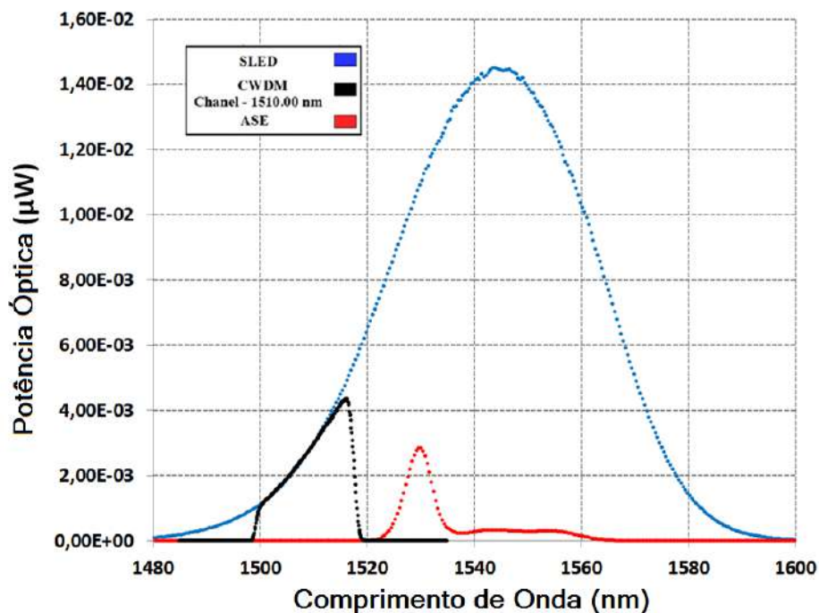
Figura 4.12.5 – Comparação entre os espectros de transmissão da fonte de luz de espectro largo e SLED, mostrando o uso do filtro de borda CWDM, utilizado em conjunto com SLED.
