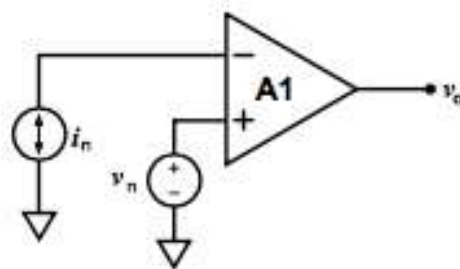
Figura 4.3.1 – Modelo do amplificador para análise de ruído.
