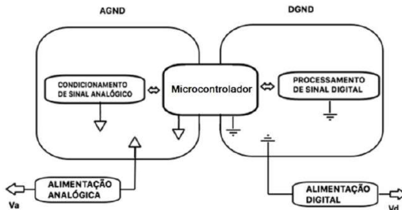
Figura 3.2.1 – Terra de sinais mistos em uma placa de circuito impresso.
