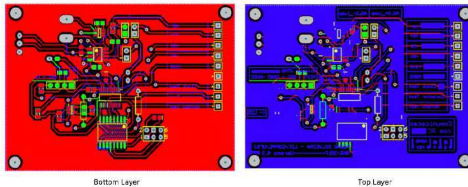
Figura 3.5.1 – Layout desenvolvido no software Altium Designer®.
