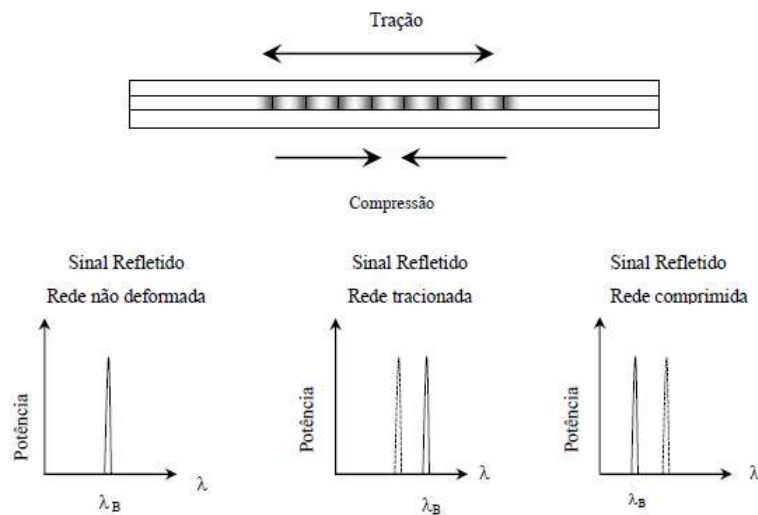
Figura 2.1.2 – Esquema do deslocamento espectral de uma FBG submetida à tração e compressão.
