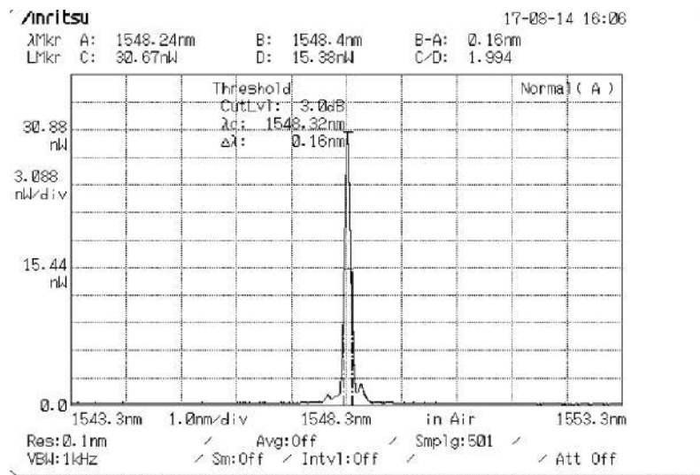
Figura 4.12.3 – Espectro de convolução entre CWDM e a FBG fabricada com \lambda_B = 1548,32 nm pelo laser de pulso de argônio Nd: YAG.
