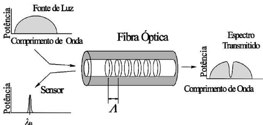
Figura 2.1.1 – Rede de Bragg
