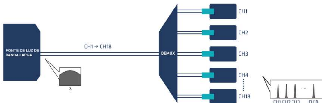
Figura 2.2.1 – Diagrama óptico do dispositivo CWDM.
