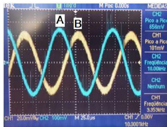
Figura 4.4.9 – Sinal A0+ (A), defasado e atenuado em relação ao sinal de entrada (B) do circuito e atenuado em relação ao obtido com menor frequência (Escala do sinal de entrada 20 mV e do sinal de saída 100 mV).
