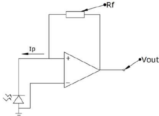
Figura 3.3.1 – Circuito amplificador de transimpedância.
