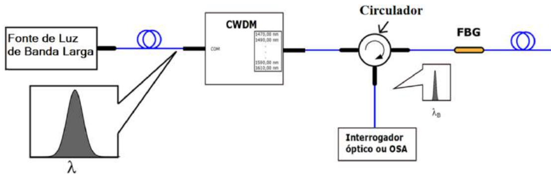
Figura 2.3.2 – Diagrama óptico utilizado para obter o sinal refletido pela FBG.
