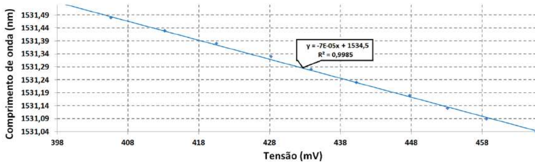
Figura 4.11.4 – Gráfico de calibração por temperatura – tensão x \lambda_B .
