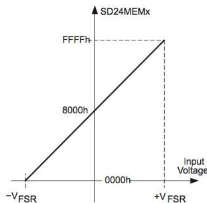
Figura 3.4.3 – Gráfico para o modo “ Bipolar Offset Binary ”.
