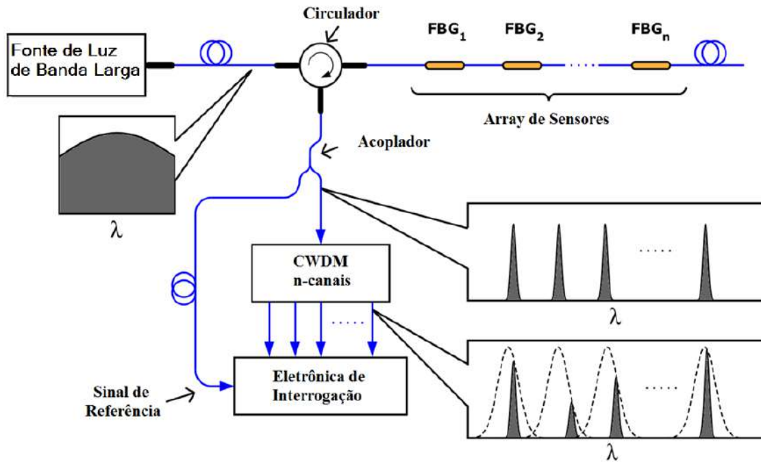
Figura 4.12.1 – Diagrama de blocos do arranjo montado para realizar os testes com CWDM.
