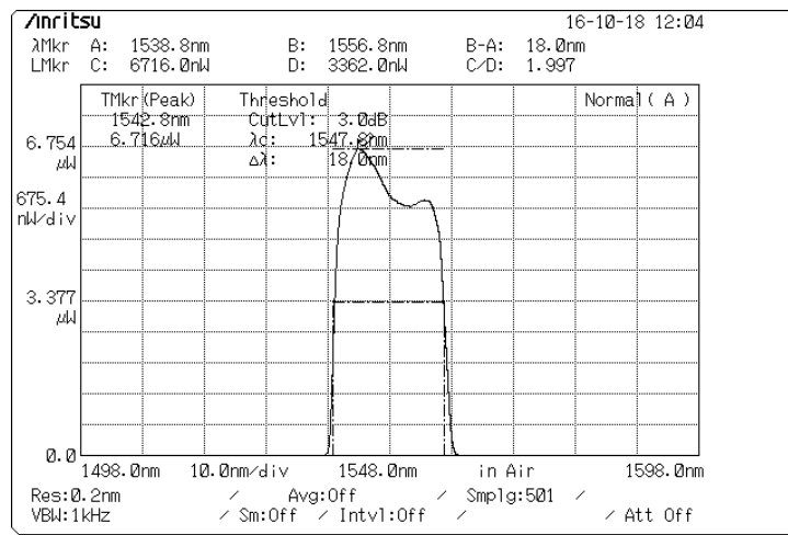
Figura 2.2.3 – Filtro CWDM com canal de saída centrado em 1550 nm.
