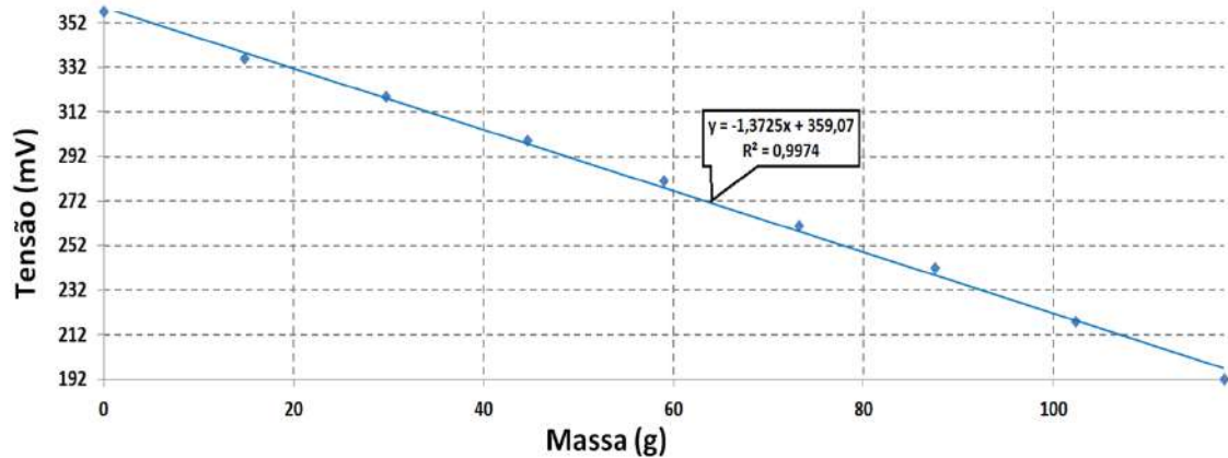
Figura 4.5.1 – Gráfico de calibração por deformação mecânica utilizando fotodetector da fabricante ThorLabs.
