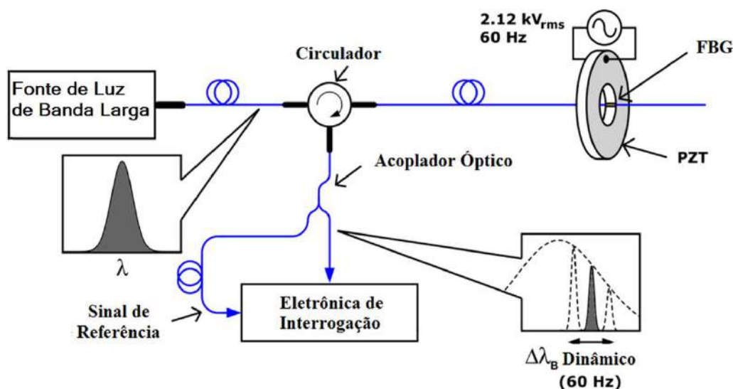
Figura 4.11.6 – Layout experimental para medições de \Delta\lambda_B induzido por deformação dinâmica de um protótipo de sensor de alta tensão.
