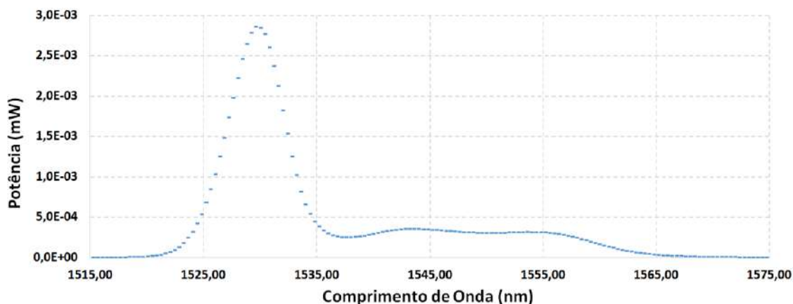
Figura 2.2.4 – Espectro da fonte de luz de banda larga da fabricante OptoLink.
