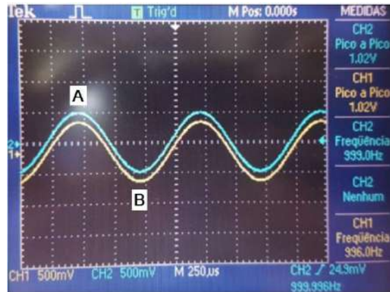
Figura 4.4.6 – Saídas de saída A0+ (A) e A0- (B) amplificadas com frequência de 1 kHz e mesmo sinal de entrada (Escala 500 mV).
