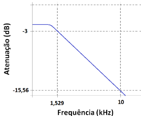
Figura 4.4.8 – Gráfico filtro RC de primeira ordem.
