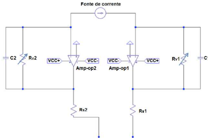
Figura 3.3.2 – Esquemático do sistema de amplificação de transimpedância desenvolvido no software LTspice© IV5.
