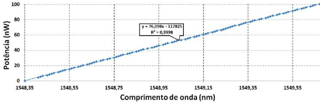
Figura 4.12.4 – Curva de calibração para a FBG centrada em 1548,35 nm, modulada pelo filtro de borda CWDM.
