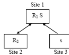
Figura 6 - Modelo de Replicação Parcial com dois objetos R e S [Vidal, Pacitti, Valduriez 2007].
