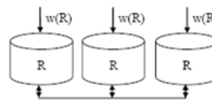
Figura 2 - Replicação de Múltiplos Mestres [Vidal, Pacitti, Valduriez 2007]; R é a cópia primária do mesmo objeto
