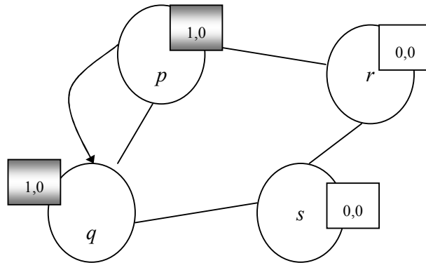
Figura 11 - Exemplo de rede onde a função de replicação é aplicada
