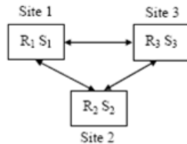
Figura 5 - Modelo de Replicação Total com dois objetos R e S [Vidal, Pacitti, Valduriez 2007].
