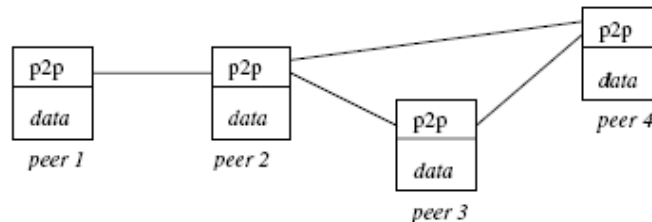
Figura 7 – Rede ponto-a-ponto não estruturada. [Valduriez, Pacitti 2004]
