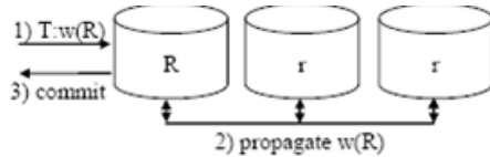
Figura 3 - Princípio de Propagação Síncrona [Vidal, Pacitti, Valduriez 2007].
