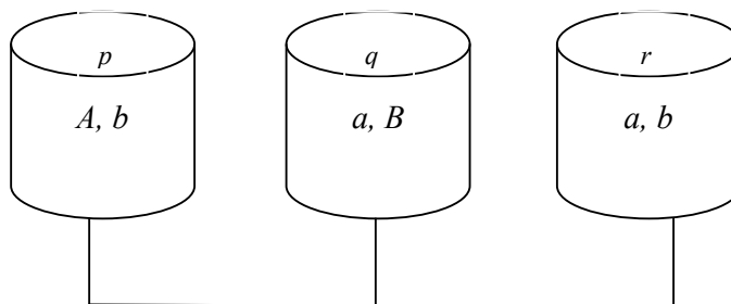
Figura 8 - Representação do modelo múltiplos únicos mestres; p , q e r são nós que armazenam objetos a e b , onde A é cópia principal, a é réplica e B é cópia principal enquanto b é a réplica.
