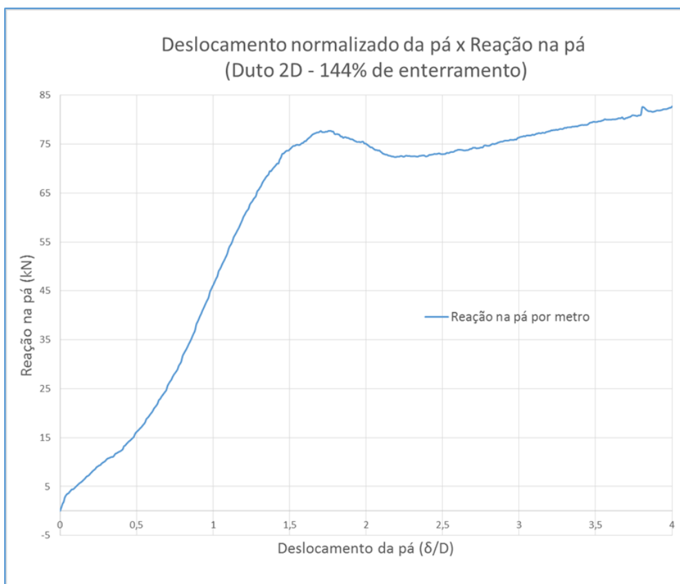
Figura 4-12 - Reação na pá por metro - Ensaio com duto 2D e 144% de enterramento
