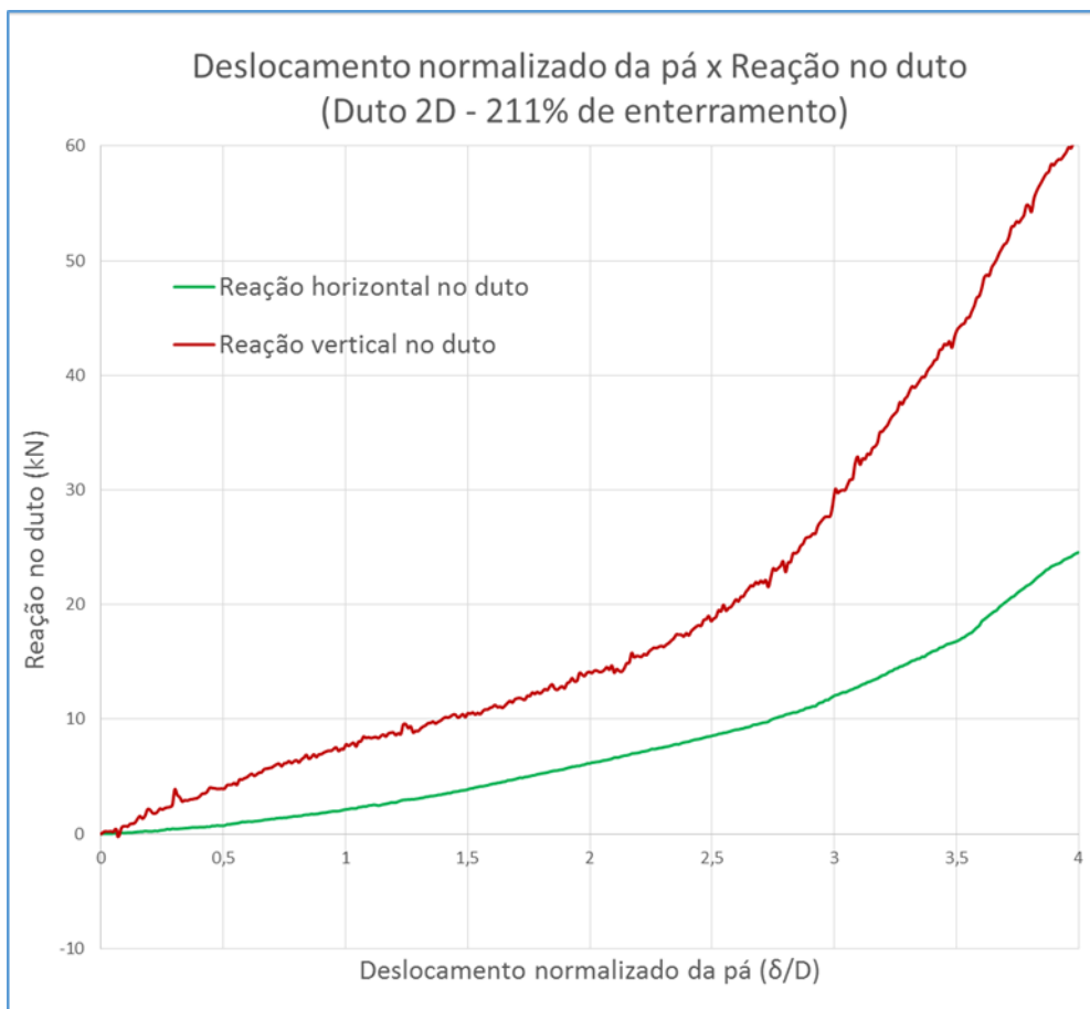
Figura 4-11 - Reação total no duto - Ensaio com duto 2D e 211% de enterramento
