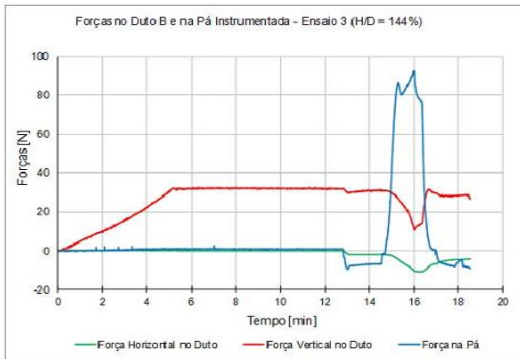
Figura 4-5 - Forças no Duto 2D e na Pá com enterramento de 144% (PEQUENO, 2013)
