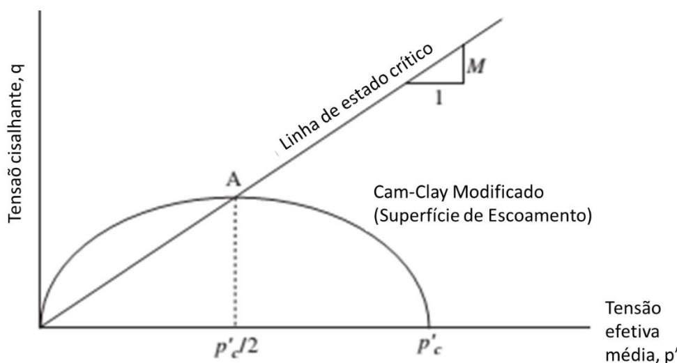
Figura 2-12 – Superfície de escoamento do modelo cam-clay no plano p' \times q (adaptado de HELWANY, 2007)
