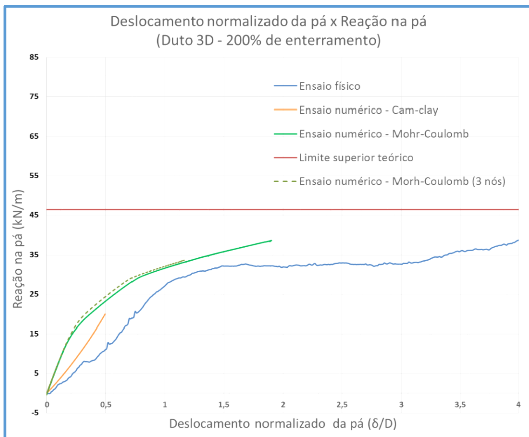
Figura 5-59 - Gráfico deslocamento versus reação na pá com Duto 3D e 200% de enterramento
