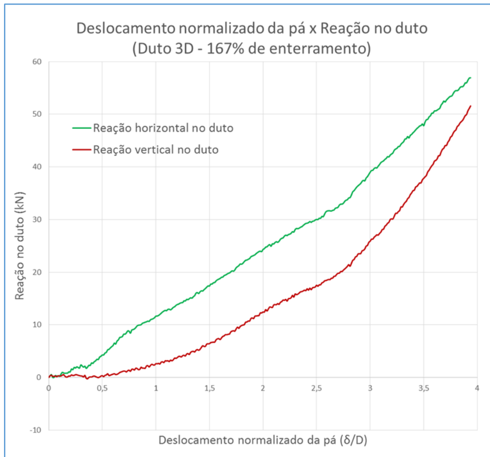
Figura 4-9 - Reação total no duto - Ensaio com duto 3D e 167% de enterramento
