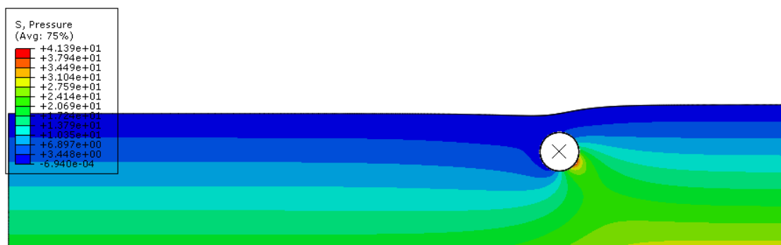
Figura 5-29 - Distribuição de tensões na massa de solo após deslocamento de 0,299m da pá contra Duto 2D com 144% de enterramento – Solo Cam-clay – Modo implícito
