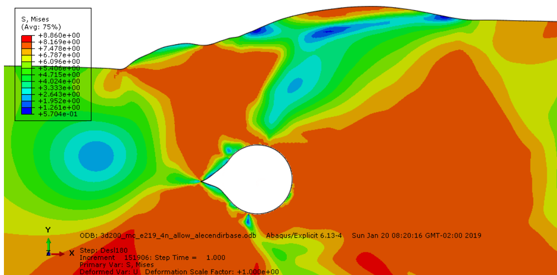
Figura 5-42 - Tensões de von Mises junto ao Duto 3D com 200% de enterramento após deslocamento de 0,869m da pá (Mohr-Coulomb - modo explícito)
