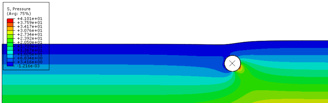
Figura 5-21 - Distribuição de tensões na massa de solo após deslocamento de 0,248m da pá contra Duto 3D com 167% de enterramento – Solo Cam-clay – Modo implícito
