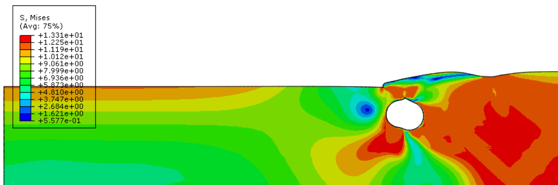
Figura 5-56 - Tensões de von Mises na massa de solo após deslocamento de 0,569m da pá contra Duto 2D com 144% de enterramento (Mohr-Coulomb - modo explícito)
