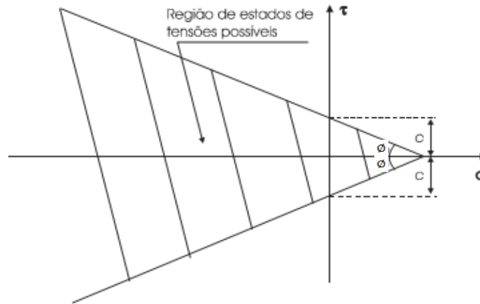
Figura 2-5 - Representação da região de estados possíveis de tensões para o critério de Mohr-Coulomb no plano \tau \times \sigma (CARDOSO, 2005)
