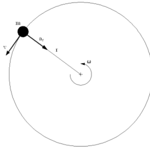
Figura 2-1 - Desenho esquemático de um modelo sujeito à aceleração em centrífuga. (PEQUENO, 2013)
