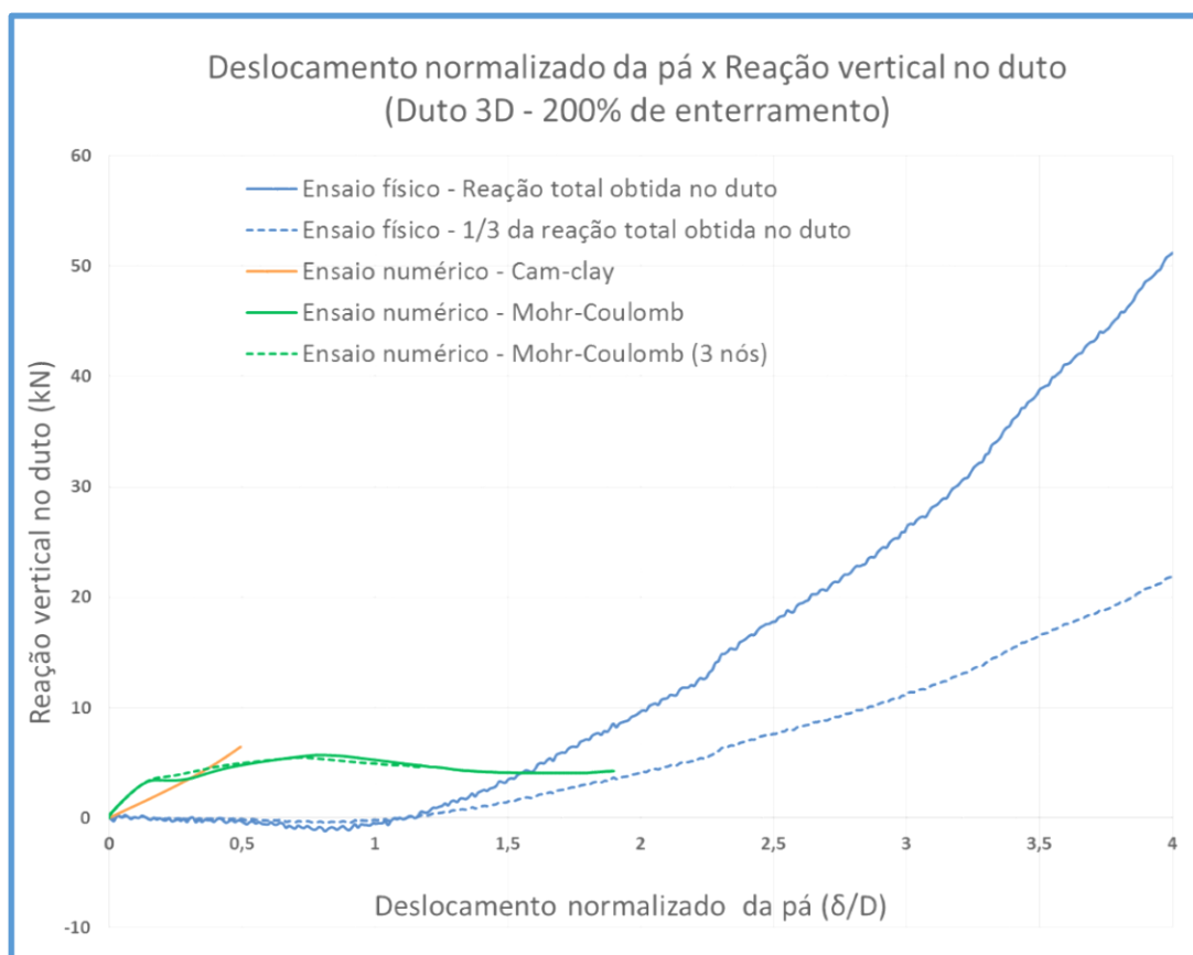
Figura 5-68 - Gráfico deslocamento versus reação vertical no duto com Duto 3D e 200% de enterramento
