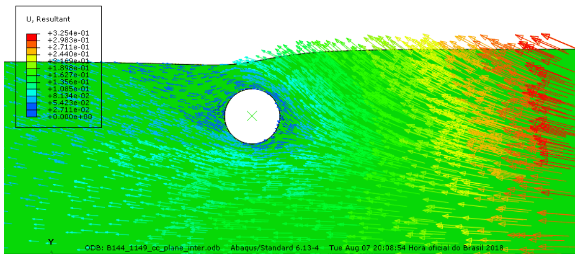
Figura 5-16 - Deslocamento total ampliado para Duto 2D com 144% de enterramento – Solo Cam-clay – Modo implícito
