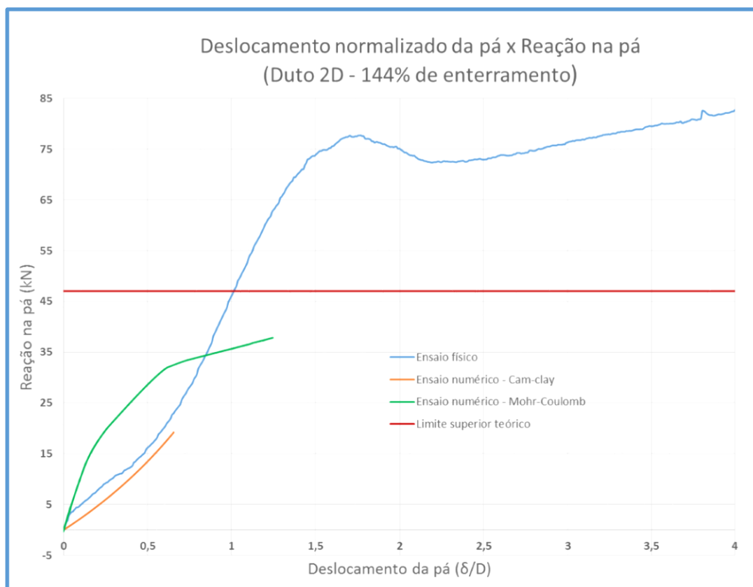
Figura 5-62 - Gráfico deslocamento versus reação na pá com Duto 2D e 144% de enterramento
