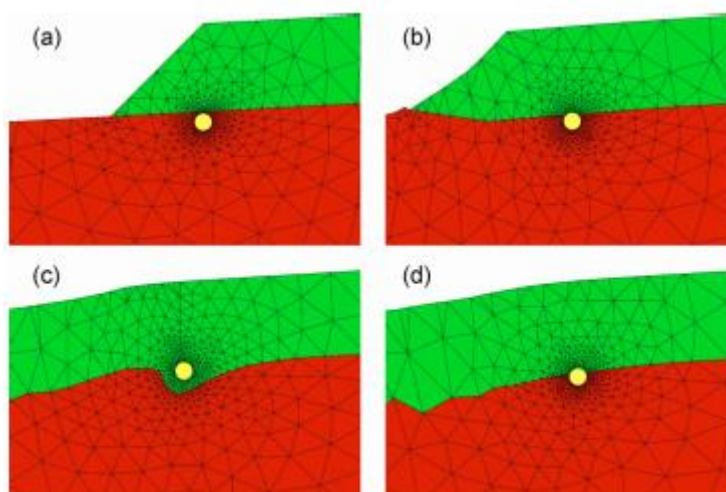
Figura 2-13 - Simulação numérica de deslizamento sobre duto enterrado (ZHU, 2010)
