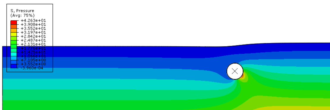
Figura 5-17 - Distribuição de tensões na massa de solo após deslocamento de 0,226m da pá contra Duto 3D com 200% de enterramento – Solo Cam-clay – Modo implícito
