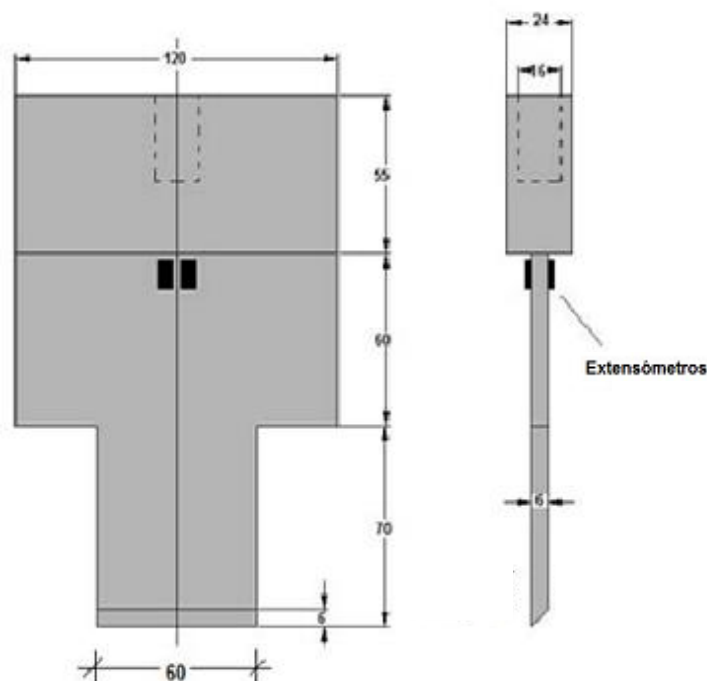
Figura 3-8 - Projeto da pá instrumentada com dimensões em mm (PEQUENO, 2013)
