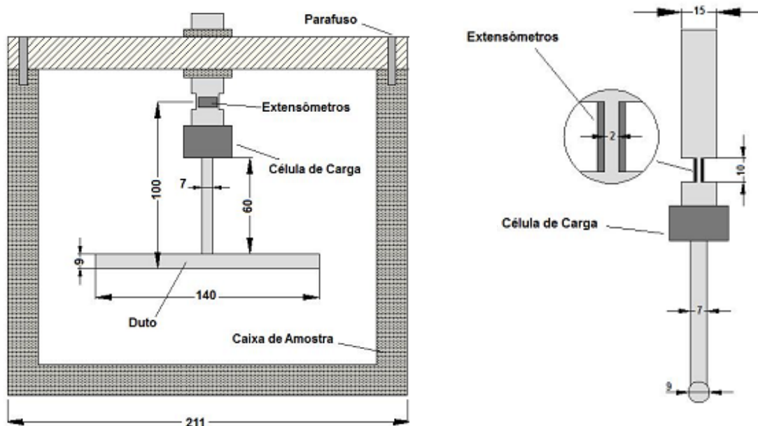
Figura 3-7 - Projeto do Duto 2D com dimensões em mm (PEQUENO, 2013)
