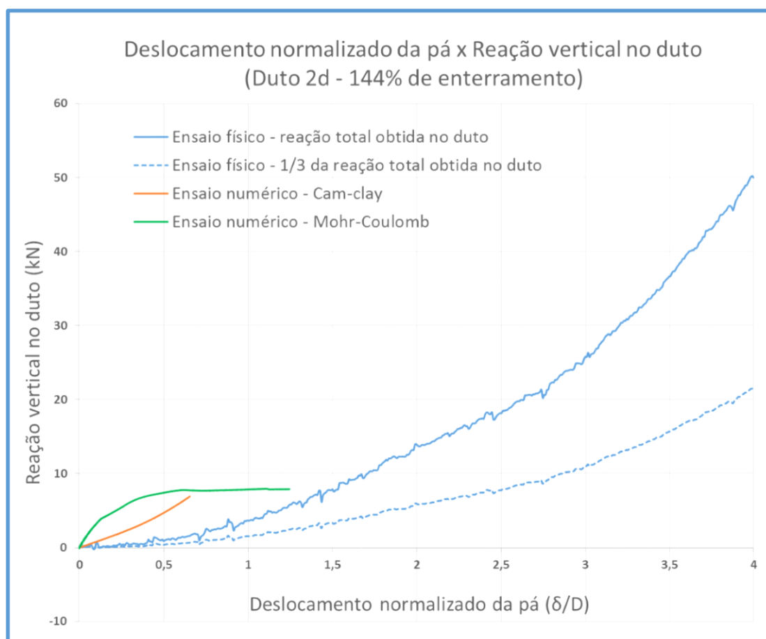
Figura 5-71 - Gráfico deslocamento versus reação vertical no duto com Duto 2D e 144% de enterramento
