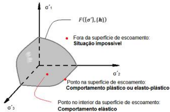
Figura 2-4 - Superfície de escoamento e domínios elástico, plástico e elastoplástico. (adaptada de DEOTTI, 2015)
