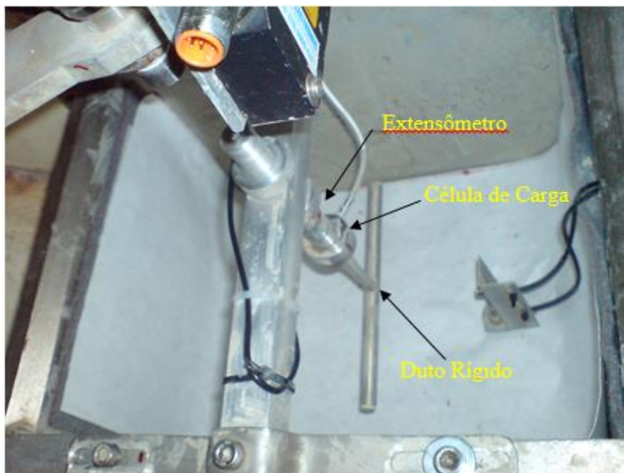
Figura 3-3 - Sistema Duto B posicionado na caixa de ensaio (PEQUENO, 2013)
