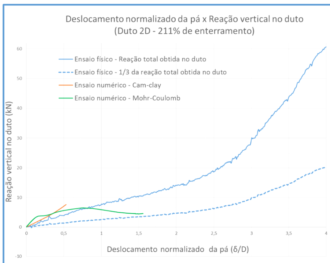
Figura 5-70 - Gráfico deslocamento versus reação vertical no duto com Duto 2D e 211% de enterramento
