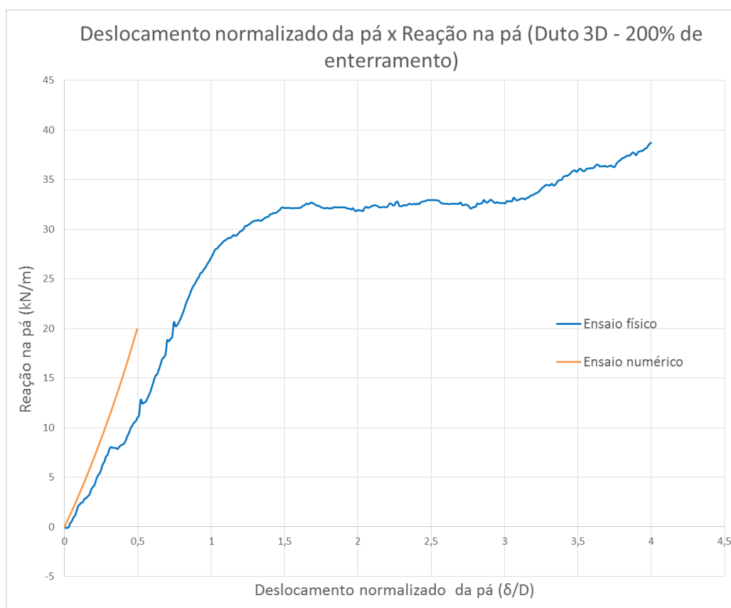
Figura 5-33 - Gráfico comparativo numérico-experimental para reação na pá com Duto 3D e 200% de enterramento (Cam-clay – modo implícito)
