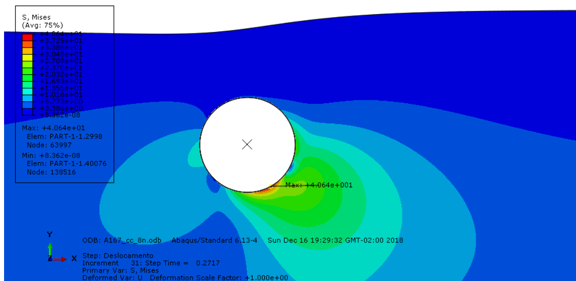
Figura 5-24 - Tensões de von Mises junto ao Duto 3D com 167% de enterramento após deslocamento de 0,248m da pá – Solo Cam-clay – Modo implícito
