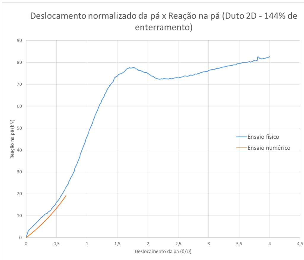
Figura 5-36 - Gráfico comparativo numérico-experimental para reação na pá com Duto 2D e 144% de enterramento (Cam-clay – modo implícito)
