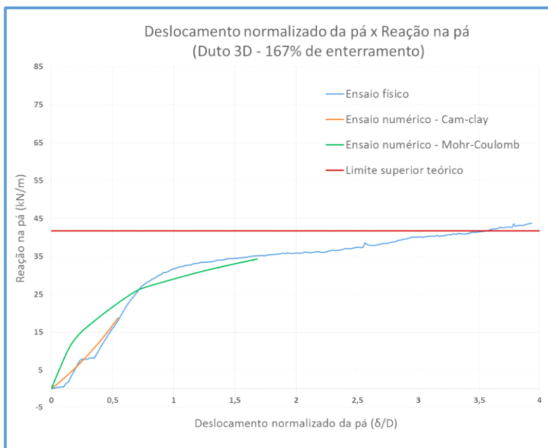
Figura 5-60 - Gráfico deslocamento versus reação na pá com Duto 3D e 167% de enterramento
