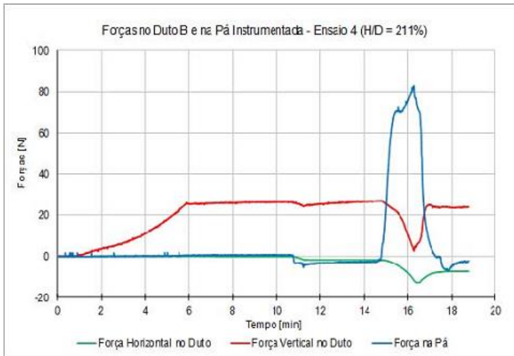
Figura 4-4 - Forças no Duto 2D e na Pá com enterramento de 211% (PEQUENO, 2013)
