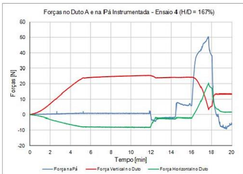
Figura 4-3 - Forças no Duto 2D e na Pá com enterramento de 167% (PEQUENO, 2013)
