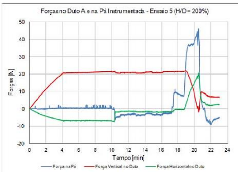
Figura 4-2 - Forças no Duto 3D e na Pá com enterramento de 200% (PEQUENO, 2013)
