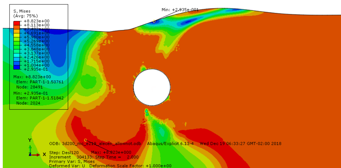
Figura 5-37 - Distribuição de tensões junto ao Duto 3D com 200% de enterramento após deslocamento de 0,531m da pá utilizando elemento de 3 nós (Mohr-Coulomb - modo explícito)
