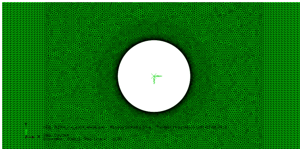
Figura 3-14 - Detalhe da malha junto ao duto com elementos de 3 nós.
