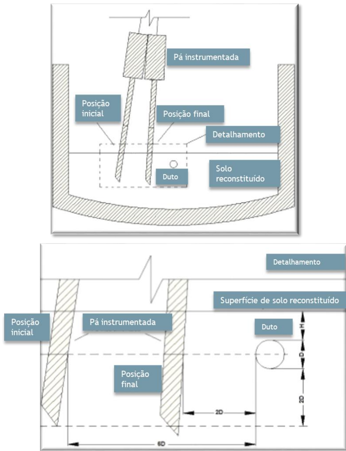
Figura 3-1 - Esquema de movimentação da Pá instrumentada em relação ao duto (PEQUENO, 2013)
