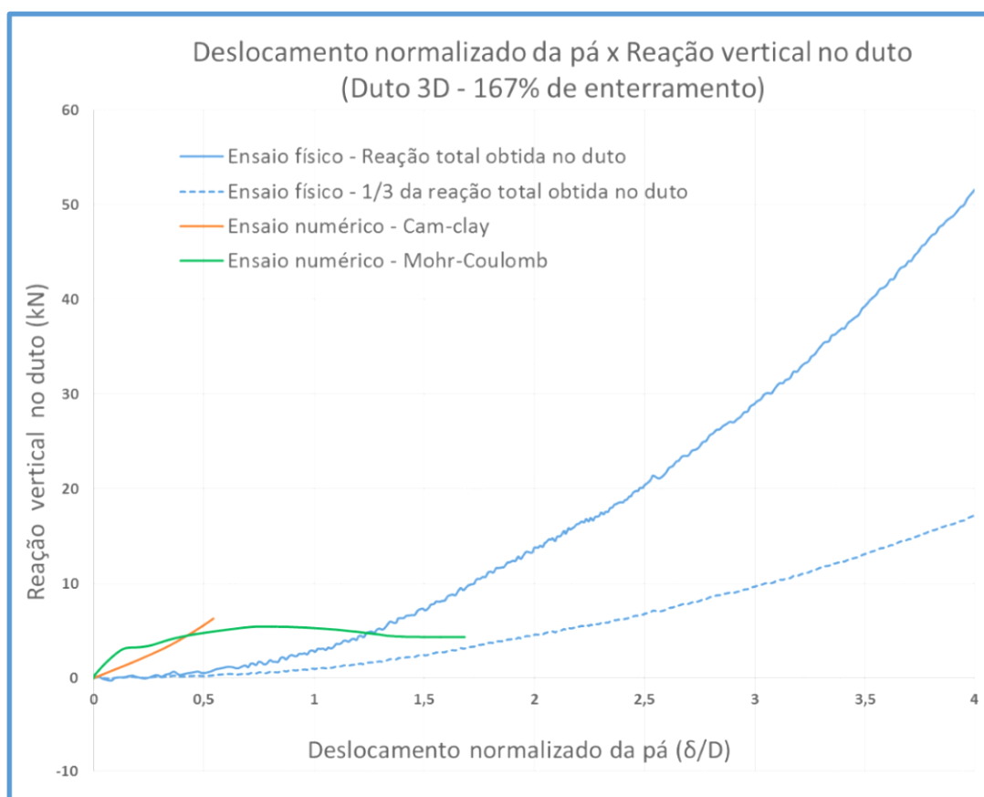
Figura 5-69 - Gráfico deslocamento versus reação vertical no duto com Duto 3D e 167% de enterramento
