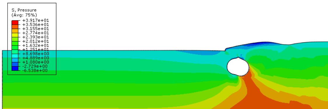
Figura 5-54 - Distribuição de tensões na massa de solo após deslocamento de 0,569m da pá contra Duto 2D com 144% de enterramento (Mohr-Coulomb - modo explícito)
