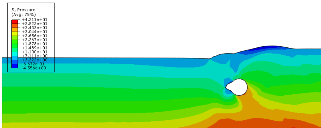
Figura 5-49 - Distribuição de tensões na massa de solo após deslocamento de 0,711m da pá contra Duto 2D com 211% de enterramento (Mohr-Coulomb - modo explícito)
