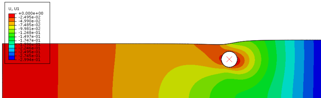
Figura 5-13 - Deslocamento horizontal para Duto 2D com 144% de enterramento – Solo Cam-clay – Modo implícito
