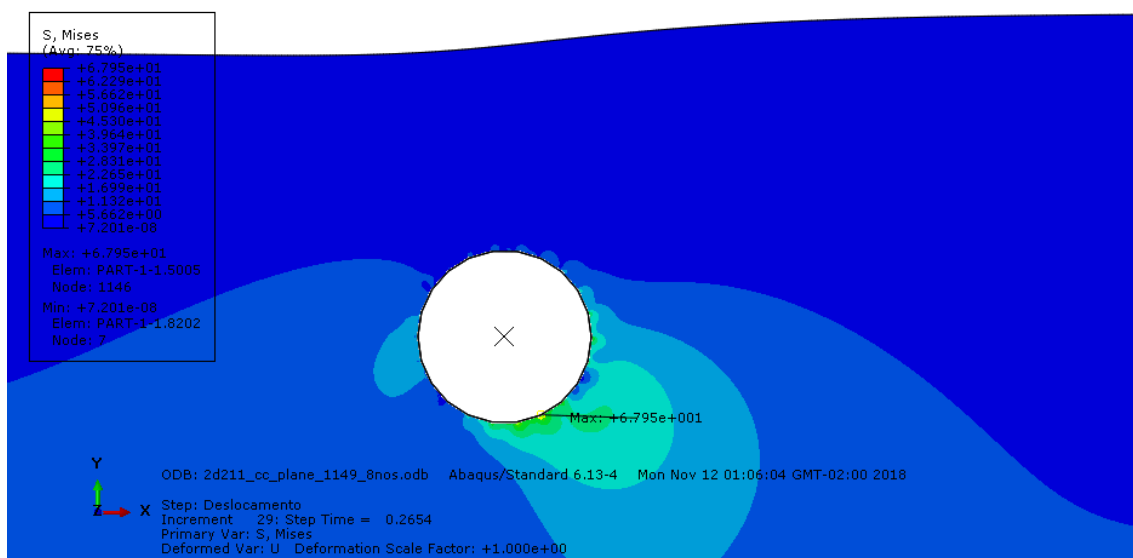
Figura 5-28 - Tensões de von Mises junto ao Duto 2D com 211% de enterramento após deslocamento de 0,243m da pá – Solo Cam-clay – Modo implícito
