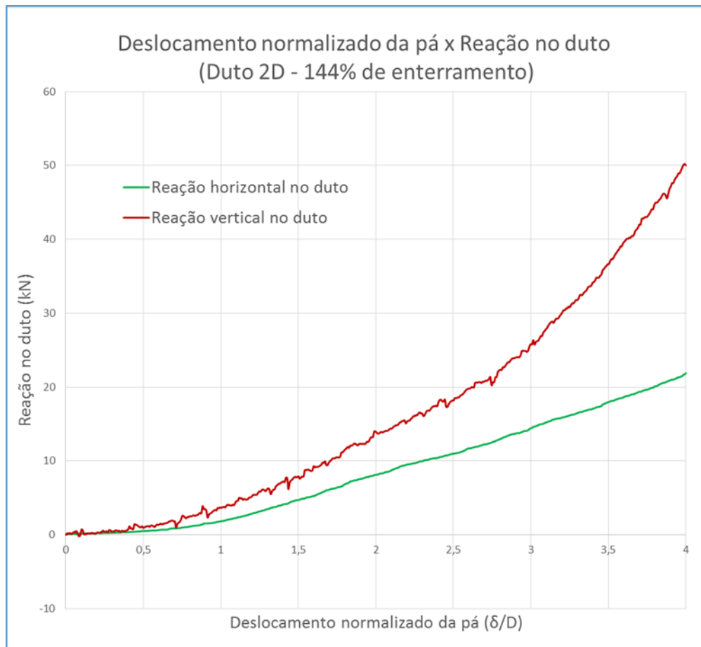
Figura 4-13 - Reação total no duto - Ensaio com duto 2D e 144% de enterramento
