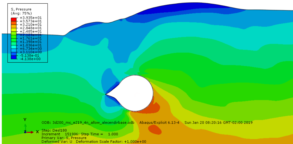
Figura 5-40 - Distribuição de tensões junto ao Duto 3D com 200% de enterramento após deslocamento de 0,869m da pá (Mohr-Culomb - modo explícito)
