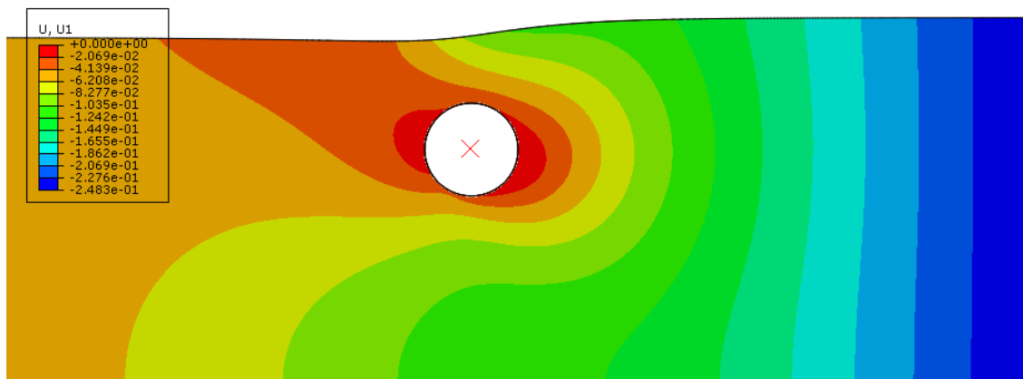
Figura 5-6 - Deslocamento horizontal ampliado para Duto 3D com 167% de enterramento – Solo Cam-clay – Modo implícito
