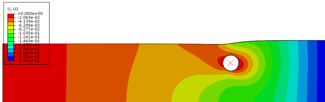
Figura 5-5 - Deslocamento horizontal para Duto 3D com 167% de enterramento – Solo Cam-clay – Modo implícito
