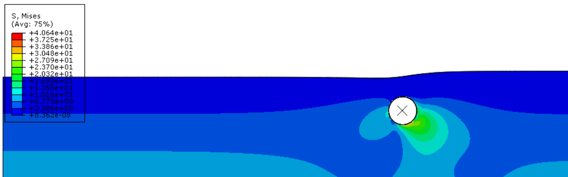
Figura 5-23 - Tensões de von Mises na massa de solo após deslocamento de 0,248m da pá contra Duto 3D com 167% de enterramento – Solo Cam-clay – Modo implícito
