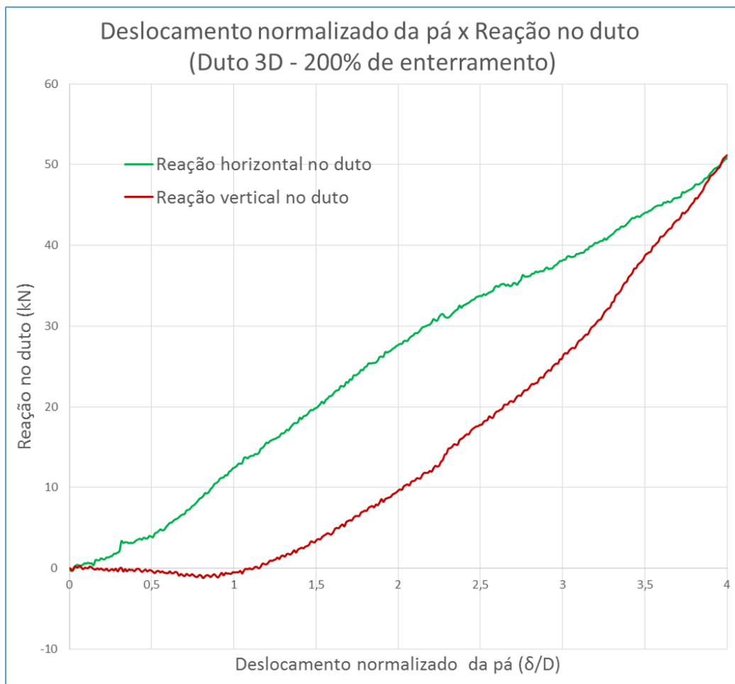
Figura 4-7 - Reação total no duto - Ensaio com duto 3D e 200% de enterramento
