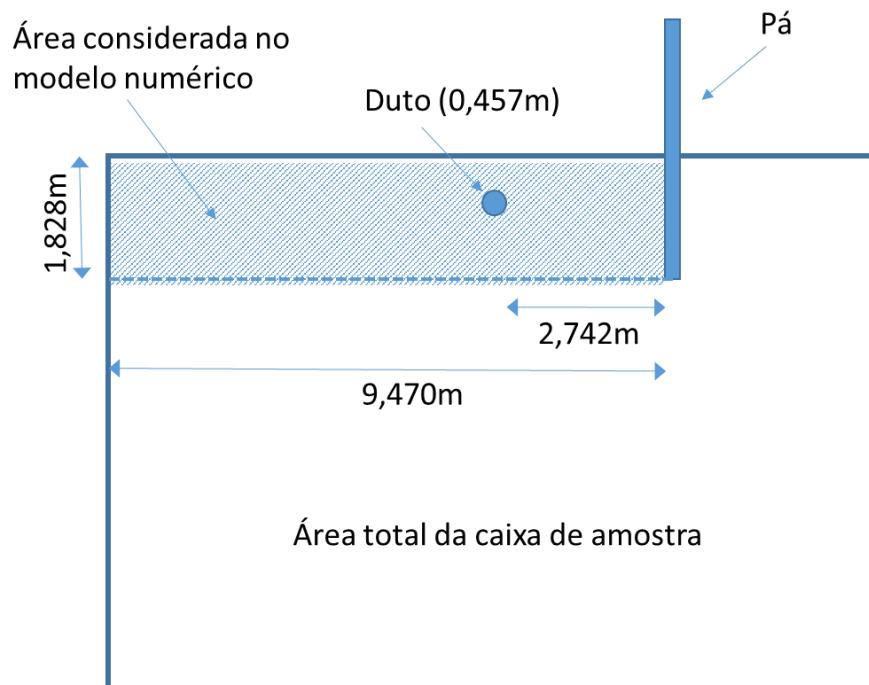
Figura 3-9 - Caixa de amostra e redução para simulação computacional.
