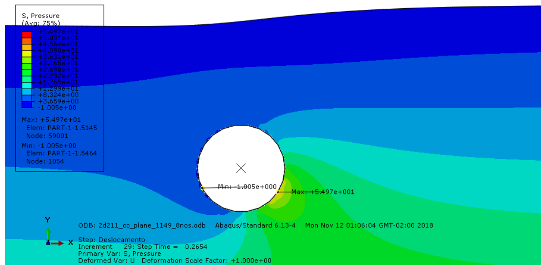
Figura 5-26 - Distribuição de tensões junto ao Duto 2D com 211% de enterramento após deslocamento de 0,243m da pá – Solo Cam-clay – Modo implícito
