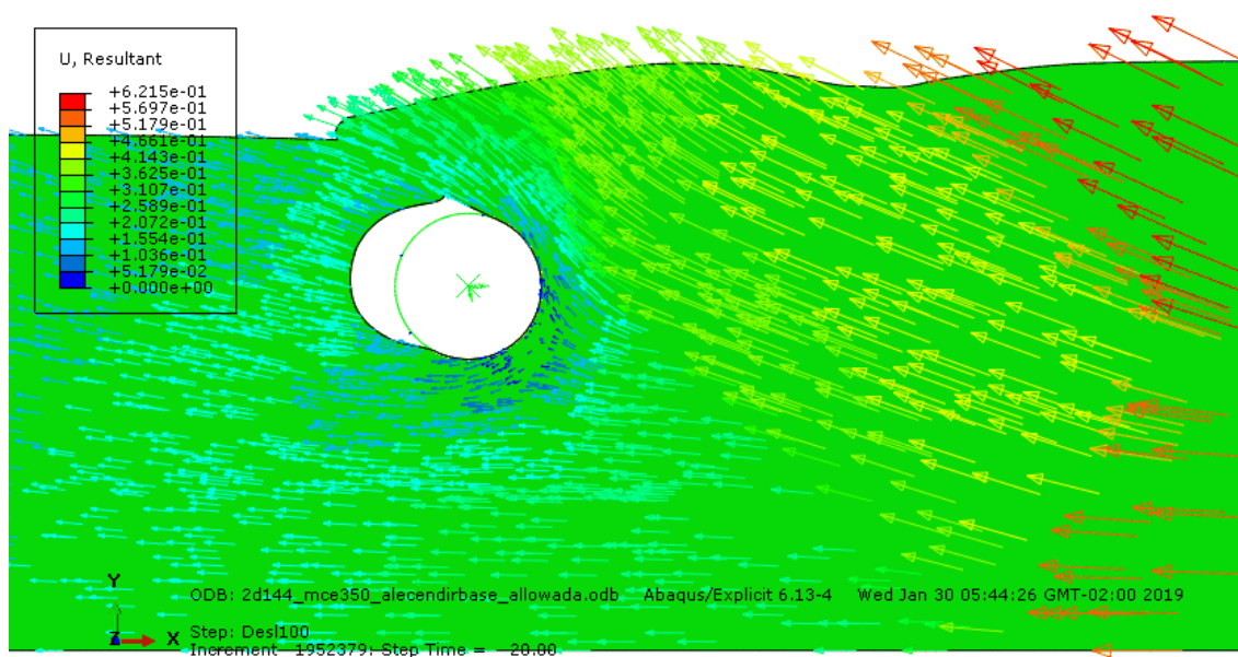
Figura 5-53 - Deslocamento total para Duto 2D com 144% de enterramento após deslocamento horizontal de 0,569m (Mohr-Coulomb - modo explícito)
