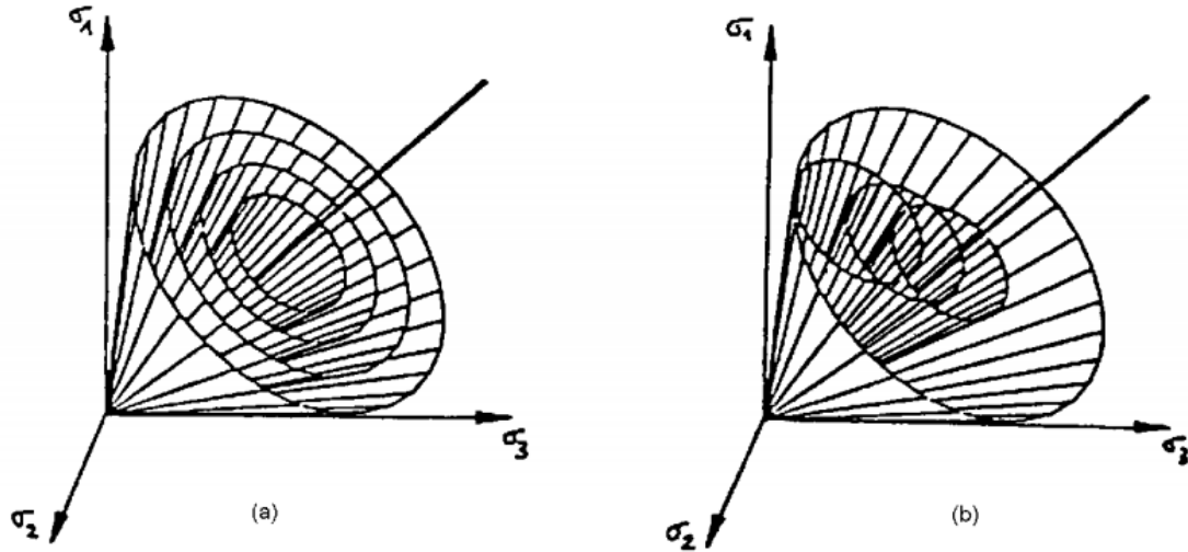
Figura 2-8 - Superfície de escoamento no espaço de tensões principais para escoamento isotrópico (a) e cinemático (b).
