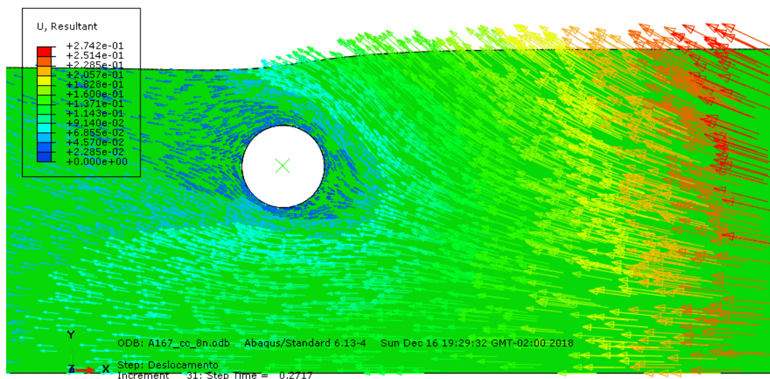
Figura 5-8 - Deslocamento total ampliado para Duto 3D com 167% de enterramento – Solo Cam-clay – Modo implícito
