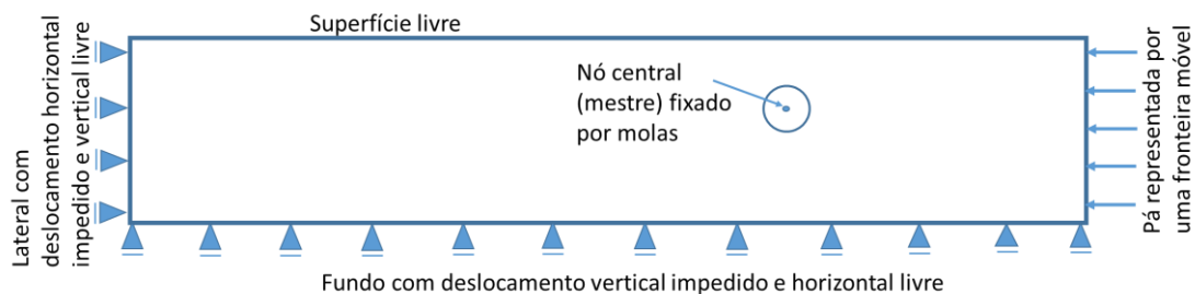
Figura 3-10 - Modelo numérico com condições de contorno e iniciais
