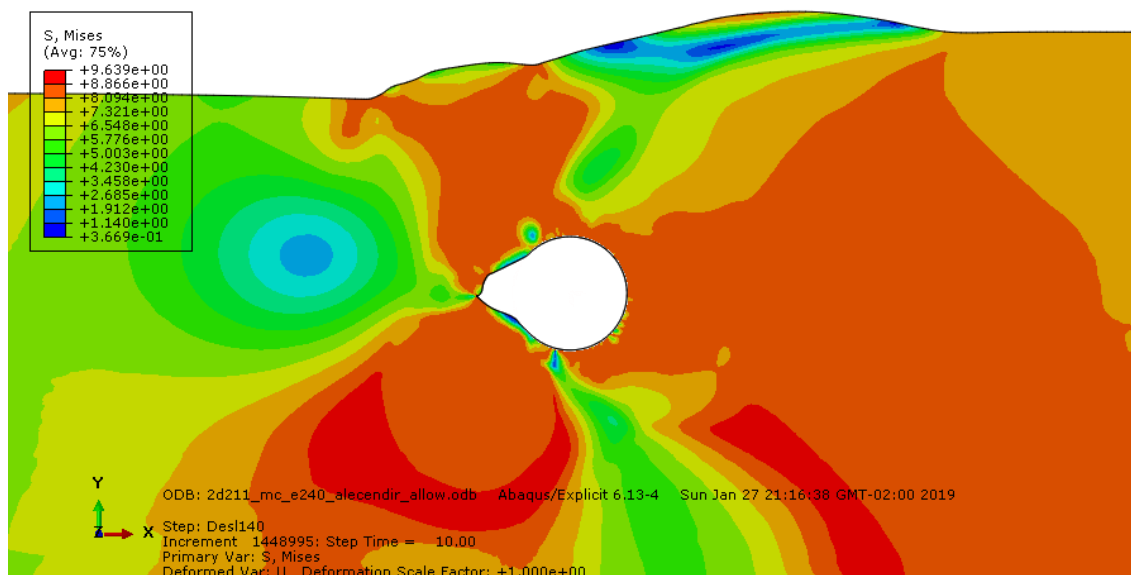
Figura 5-52 - Tensões de von Mises junto ao Duto 2D com 211% de enterramento após deslocamento de 0,711m da pá (Mohr-Coulomb - modo explícito)
