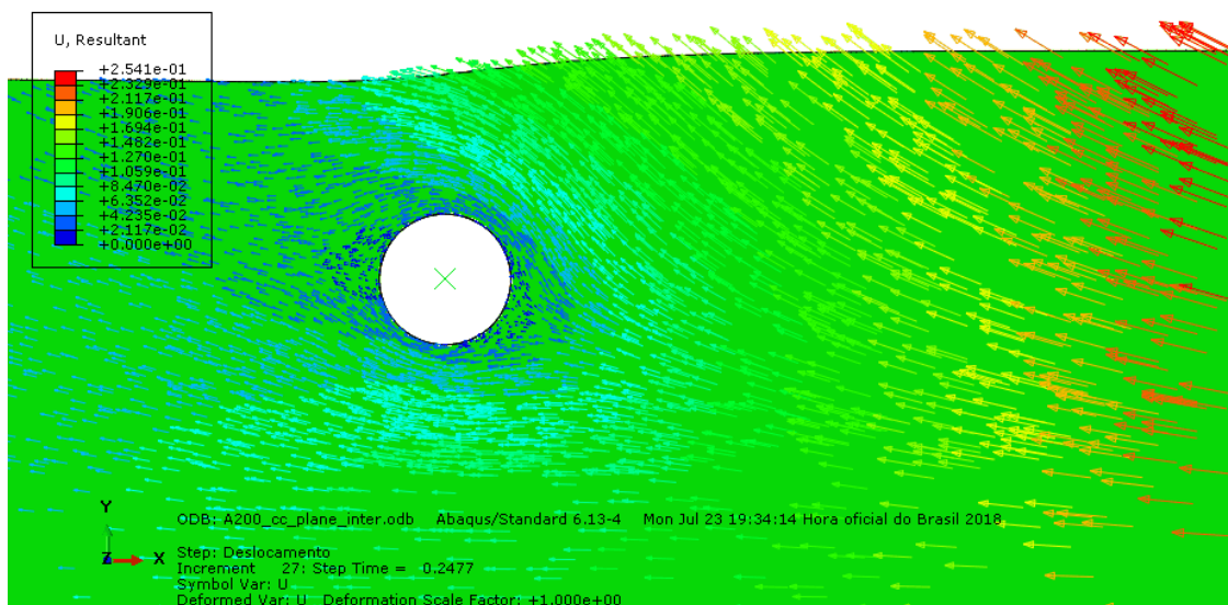
Figura 5-4 - Deslocamento total ampliado para Duto 3D com 200% de enterramento – Solo Cam-clay – Modo implícito
