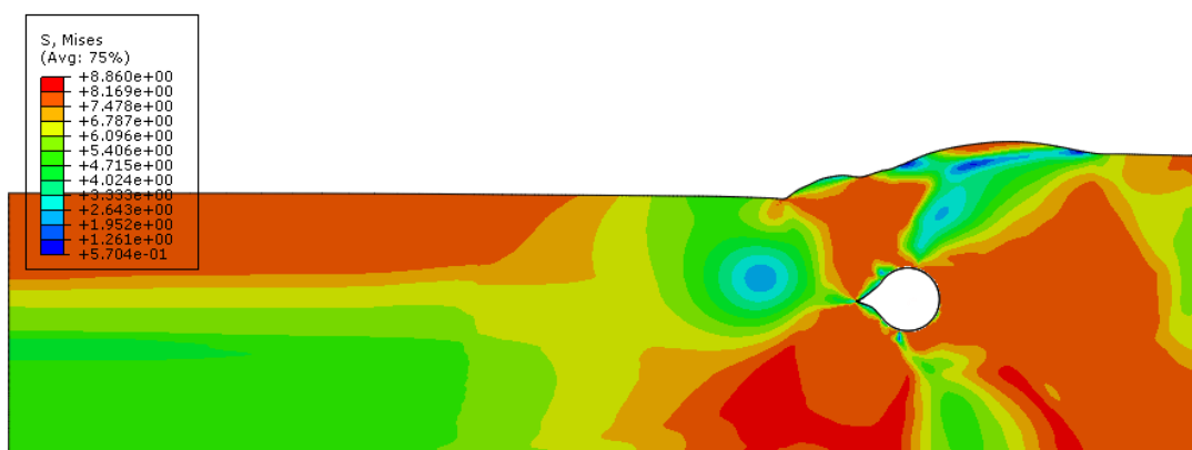
Figura 5-41 - Tensões de von Mises na massa de solo após deslocamento de 0,869m da pá contra Duto 3D com 200% de enterramento (Mohr-Coulomb - modo explícito)
