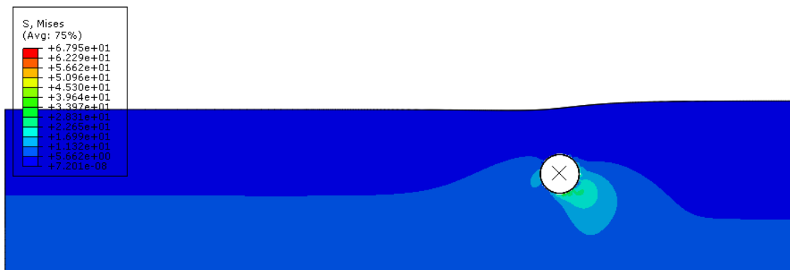
Figura 5-27 - Tensões de von Mises na massa de solo após deslocamento de 0,243m da pá contra Duto 2D com 211% de enterramento – Solo Cam-clay – Modo implícito
