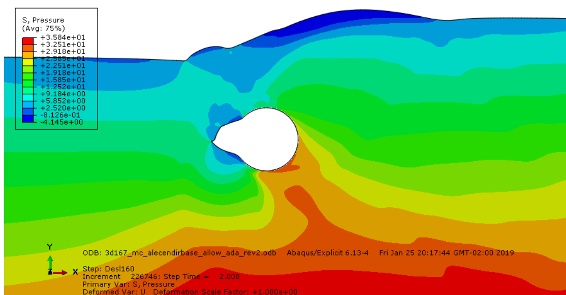
Figura 5-45 - Distribuição de tensões junto ao Duto 3D com 167% de enterramento após deslocamento de 0,769m da pá (Mohr-Culomb - modo explícito)
