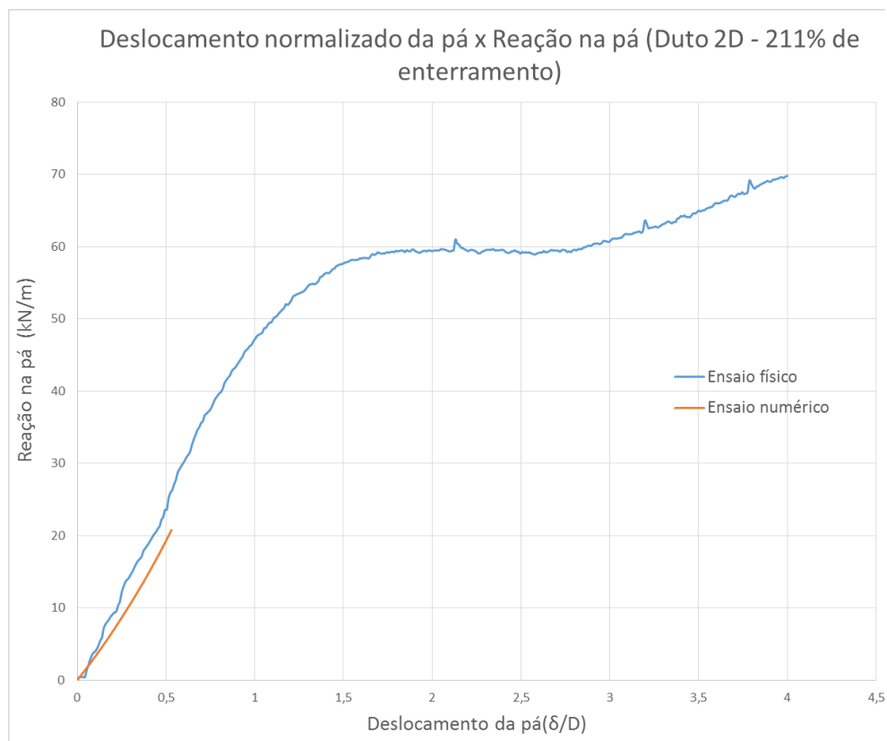
Figura 5-35 - Gráfico comparativo numérico-experimental para reação na pá com Duto 2D e 211% de enterramento (Cam-clay – modo implícito)
