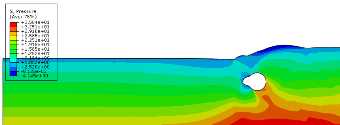
Figura 5-44 - Distribuição de tensões na massa de solo após deslocamento de 0,769m da pá contra Duto 3D com 167% de enterramento (Mohr-Coulomb - modo explícito)
