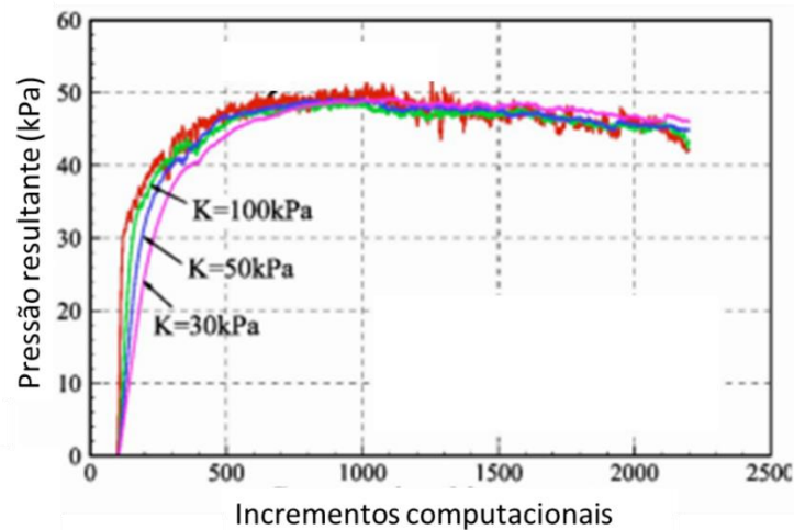
Figura 2-14 - Pressão resultante no duto ao longo da simulação numérica (ZHU, 2010)
