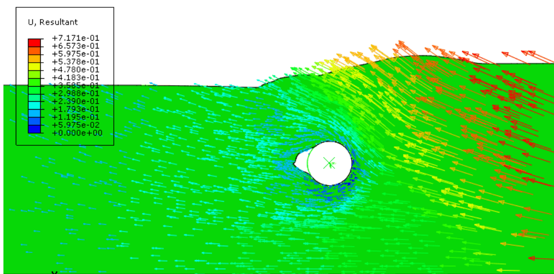
Figura 5-48 - Deslocamento parcial (0,656m) para Duto 2D com 211% de enterramento (Mohr-Coulomb - modo explícito)
