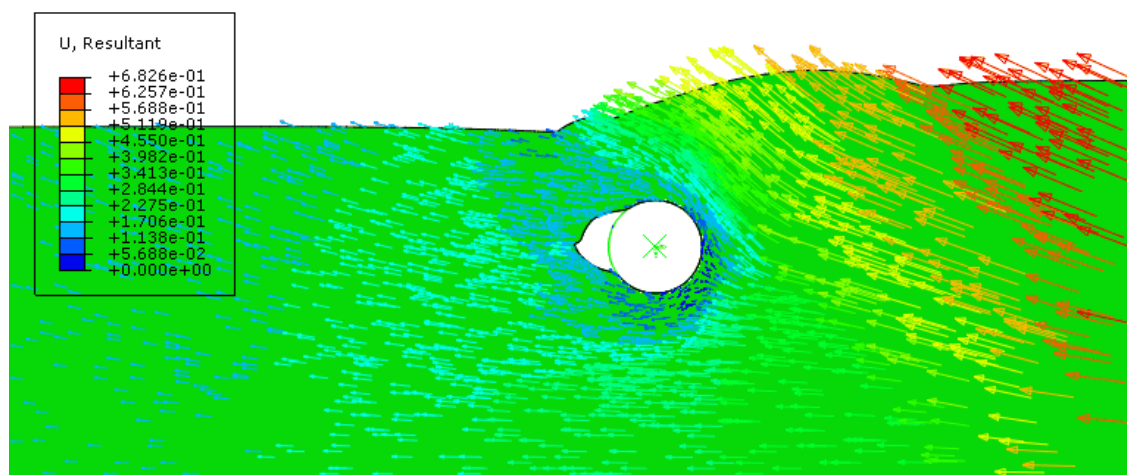
Figura 5-43 - Deslocamento parcial (0,622m) para Duto 3D com 167% de enterramento (Mohr-Coulomb - modo explícito)
