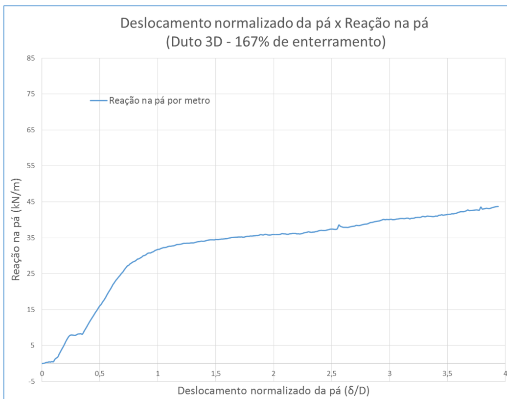
Figura 4-8 - Reação na pá por metro - Ensaio com duto 3D e 167% de enterramento
