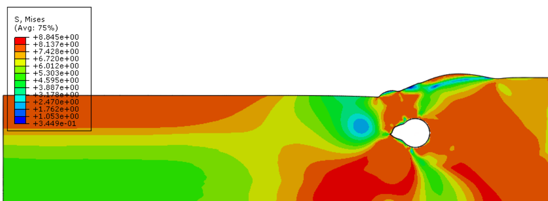
Figura 5-46 - Tensões de von Mises na massa de solo após deslocamento de 0,769m da pá contra Duto 3D com 167% de enterramento (Mohr-Coulomb - modo explícito)
