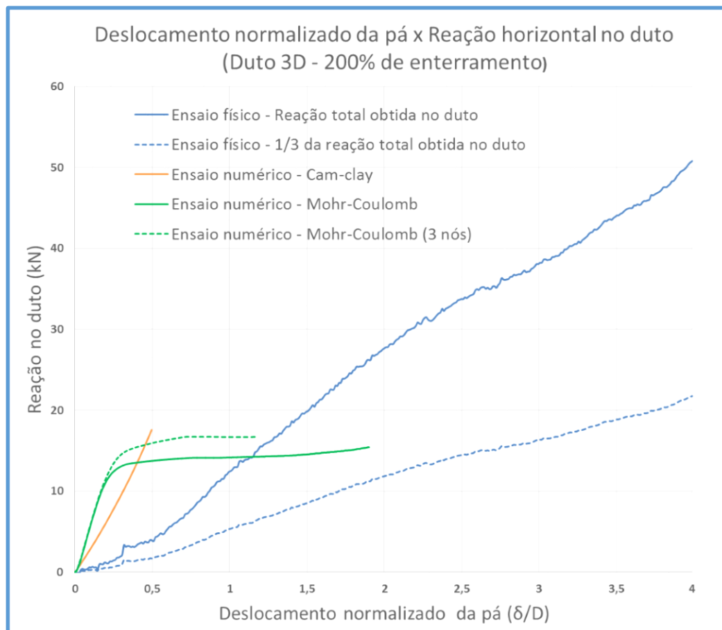
Figura 5-64 - Gráfico deslocamento versus reação horizontal no duto com Duto 3D e 200% de enterramento
