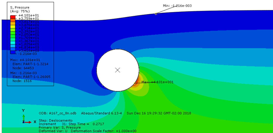
Figura 5-22 - Distribuição de tensões junto ao Duto 3D com 167% de enterramento após deslocamento de 0,248m da pá – Solo Cam-clay – Modo implícito
