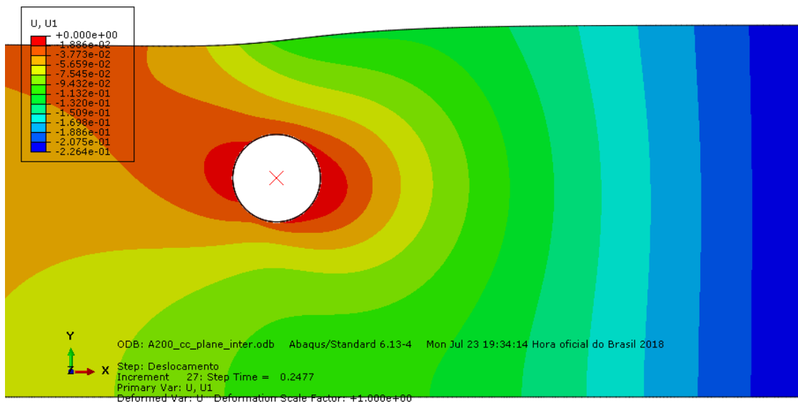
Figura 5-2 - Deslocamento horizontal ampliado para Duto 3D com 200% de enterramento – Solo Cam-clay – Modo implícito
