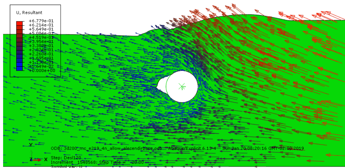
Figura 5-38 - Deslocamento parcial (0,624m) para Duto 3D com 200% de enterramento (Mohr-Coulomb - modo explícito)
