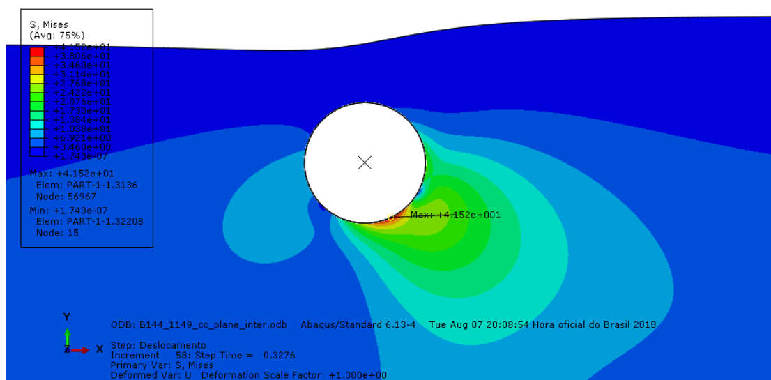
Figura 5-32 - Tensões de von Mises junto ao Duto 2D com 144% de enterramento após deslocamento de 0,299m da pá – Solo Cam-clay – Modo implícito
