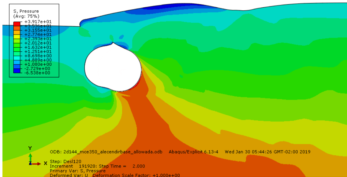
Figura 5-55 - Distribuição de tensões junto ao Duto 2D com 144% de enterramento após deslocamento de 0,569m da pá (Mohr-Culomb - modo explícito)
