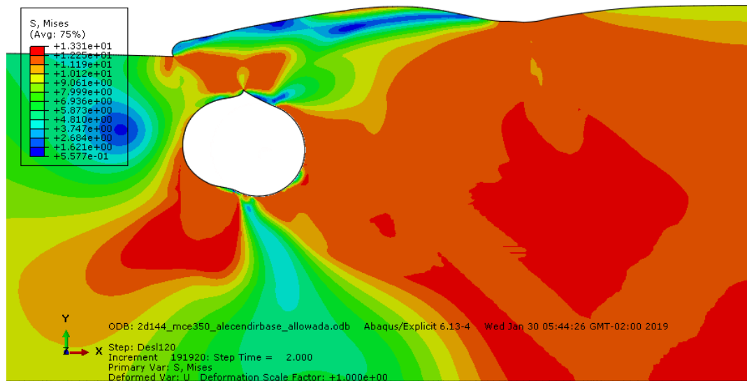
Figura 5-57 - Tensões de von Mises junto ao Duto 2D com 144% de enterramento após deslocamento de 0,569m da pá (Mohr-Coulomb - modo explícito)
