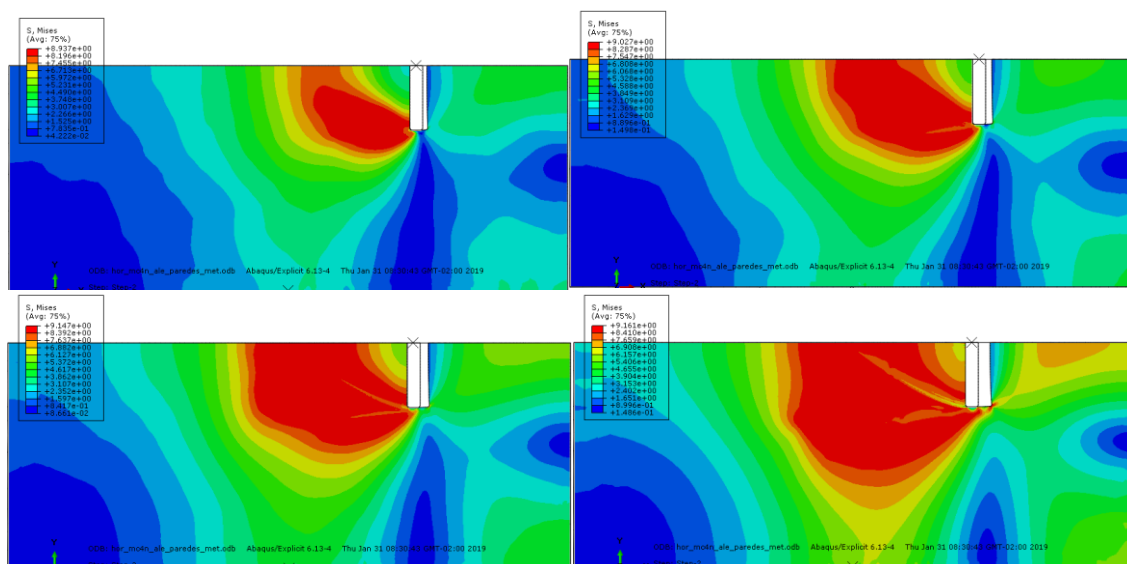
Figura 5-63 - Tensões de von Mises no plano horizontal após deslocamento da pá de 0,10m (esquerda superior); 0,15m (direita superior); 0,20m (esquerda inferior) e 0,30m (direita inferior)
