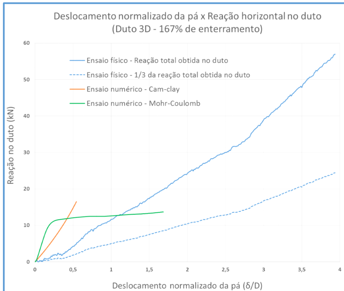
Figura 5-65 - Gráfico deslocamento versus reação horizontal no duto com Duto 3D e 167% de enterramento
