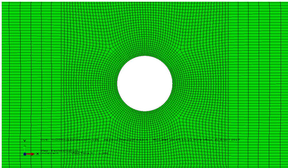
Figura 3-13 - Detalhe da malha junto ao duto com elementos de 8 nós.
