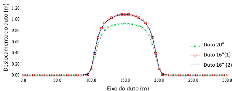
Figura 2-16 - Deslocamento transversal ao longo do eixo dos dutos ao longo do eixo (adaptado de SUSILA, 2018)
