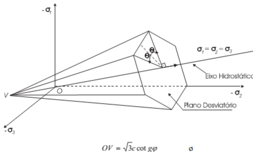
Figura 2-7- Superfície de escoamento de Mohr-Coulomb no espaço de tensões principais (CARDOSO, 2005)
