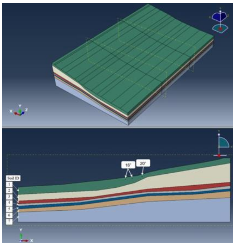
Figura 2-15 - Configuração da modelagem numérica tridimensional para movimentação de massa de solo transversal a grupo de dutos enterrados (adaptado de SUSILA, 2018)
