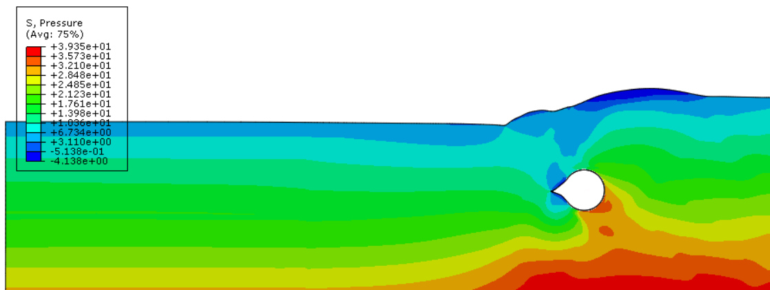
Figura 5-39 - Distribuição de tensões na massa de solo após deslocamento de 0,869m da pá contra Duto 3D com 200% de enterramento (Mohr-Coulomb - modo explícito)
