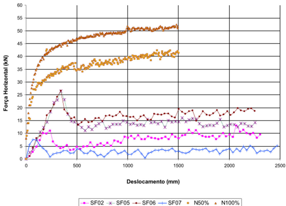
Figura 2-17 Comparação dos resultados físico e numérico para areia compacta (PACHECO, 2005)
