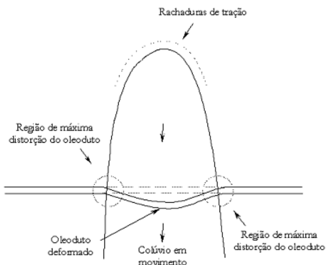
Figura 1-4 - Desenho esquemático de movimentação de solo transversal ao duto (SANDRONI et al , 2001)
