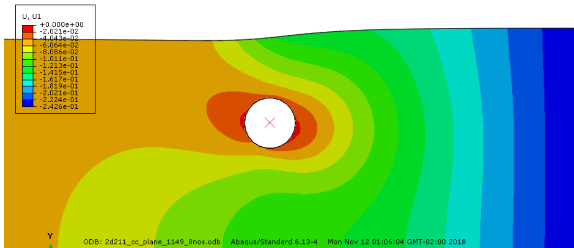
Figura 5-10 - Deslocamento horizontal ampliado para Duto 2D com 211% de enterramento – Solo Cam-clay – Modo implícito
