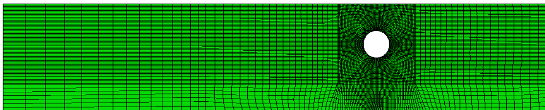
Figura 3-12 - Malha gerada pelo programa Abaqus com elementos de 8 nós
