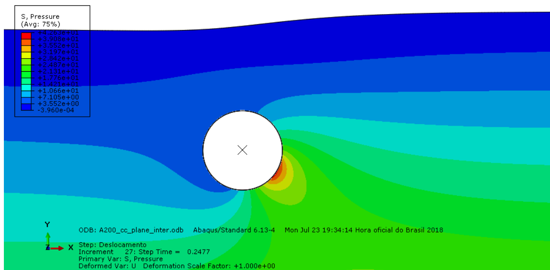
Figura 5-18 - Distribuição de tensões junto ao Duto 3D com 200% de enterramento após deslocamento de 0,226m da pá – Solo Cam-clay – Modo implícito
