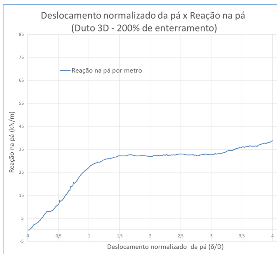
Figura 4-6 - Reação na pá por metro - Ensaio com duto 3D e 200% de enterramento
