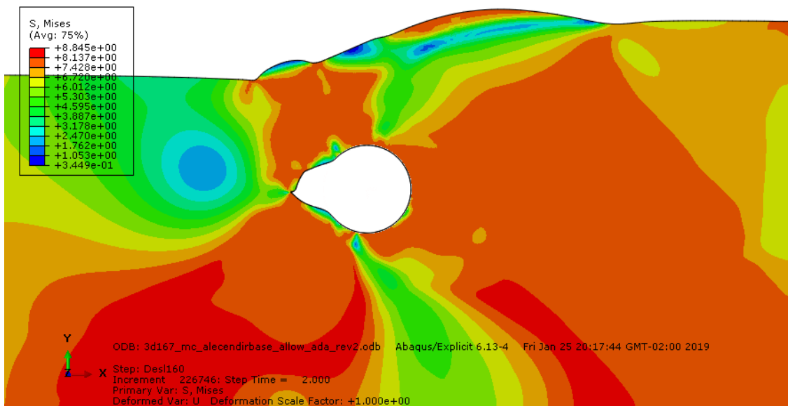
Figura 5-47 - Tensões de von Mises junto ao Duto 3D com 167% de enterramento após deslocamento de 0,769m da pá (Mohr-Coulomb - modo explícito)
