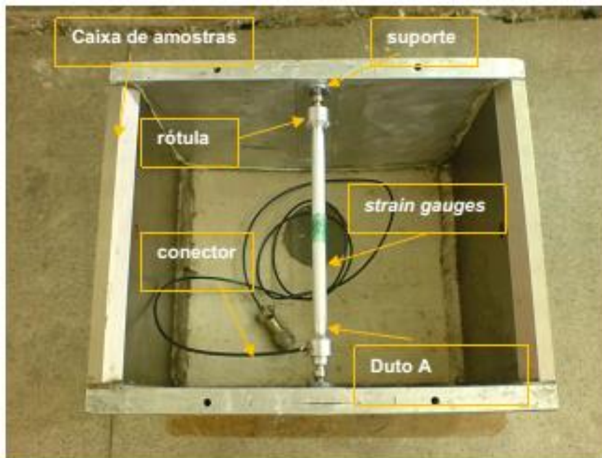
Figura 3-2 - Sistema Duto A posicionado na caixa de ensaio (PEQUENO, 2013)
