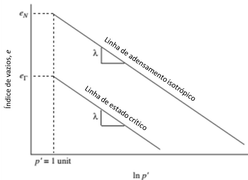
Figura 2-11 - Linha de adensamento isotrópico e linha de estado crítico no plano \ln p' \times e (adaptado de HELWANY, 2007)
