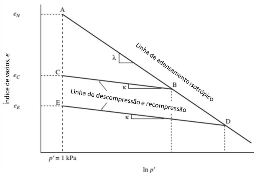
Figura 2-10 - Linha de adensamento isotrópico no plano \ln p' \times e (adaptado de HELWANY, 2007)
