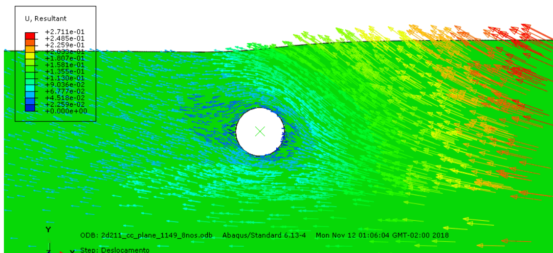
Figura 5-12 - Deslocamento total ampliado para Duto 2D com 211% de enterramento – Solo Cam-clay – Modo implícito
