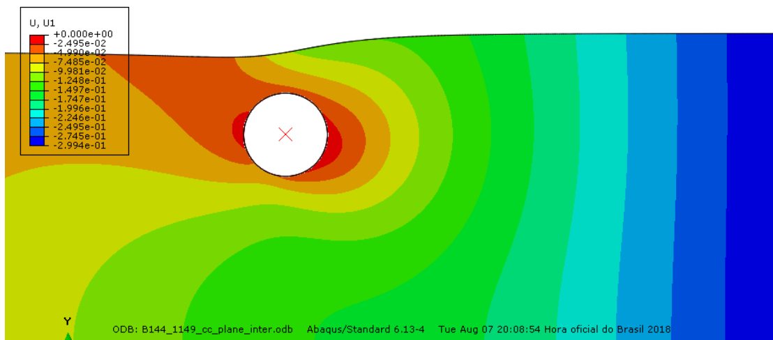
Figura 5-14 - Deslocamento horizontal ampliado para Duto 2D com 144% de enterramento – Solo Cam-clay – Modo implícito
