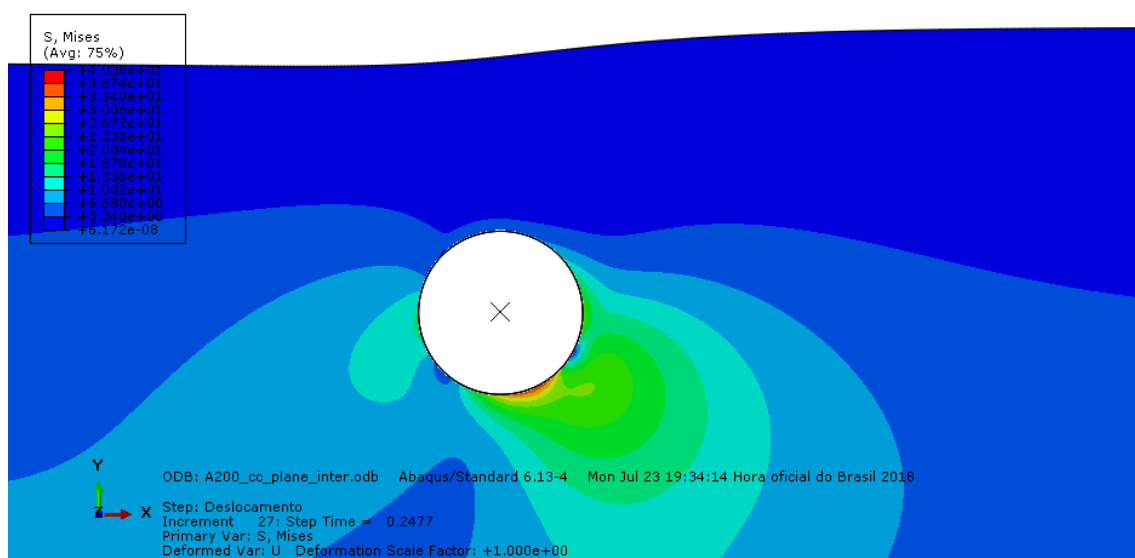
Figura 5-20 - Tensões de von Mises junto ao Duto 3D com 200% de enterramento após deslocamento de 0,226m da pá – Solo Cam-clay – Modo implícito
