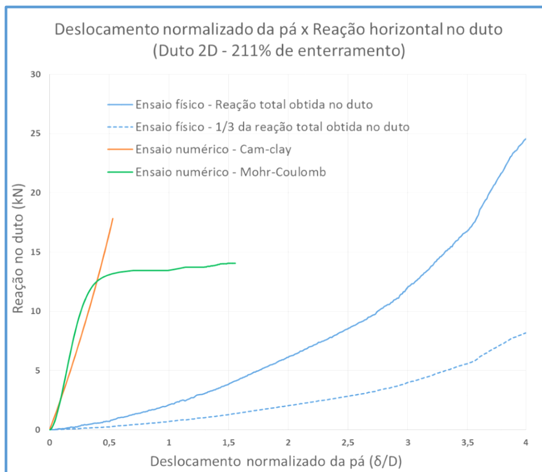
Figura 5-66 - Gráfico deslocamento versus reação horizontal no duto com Duto 2D e 211% de enterramento
