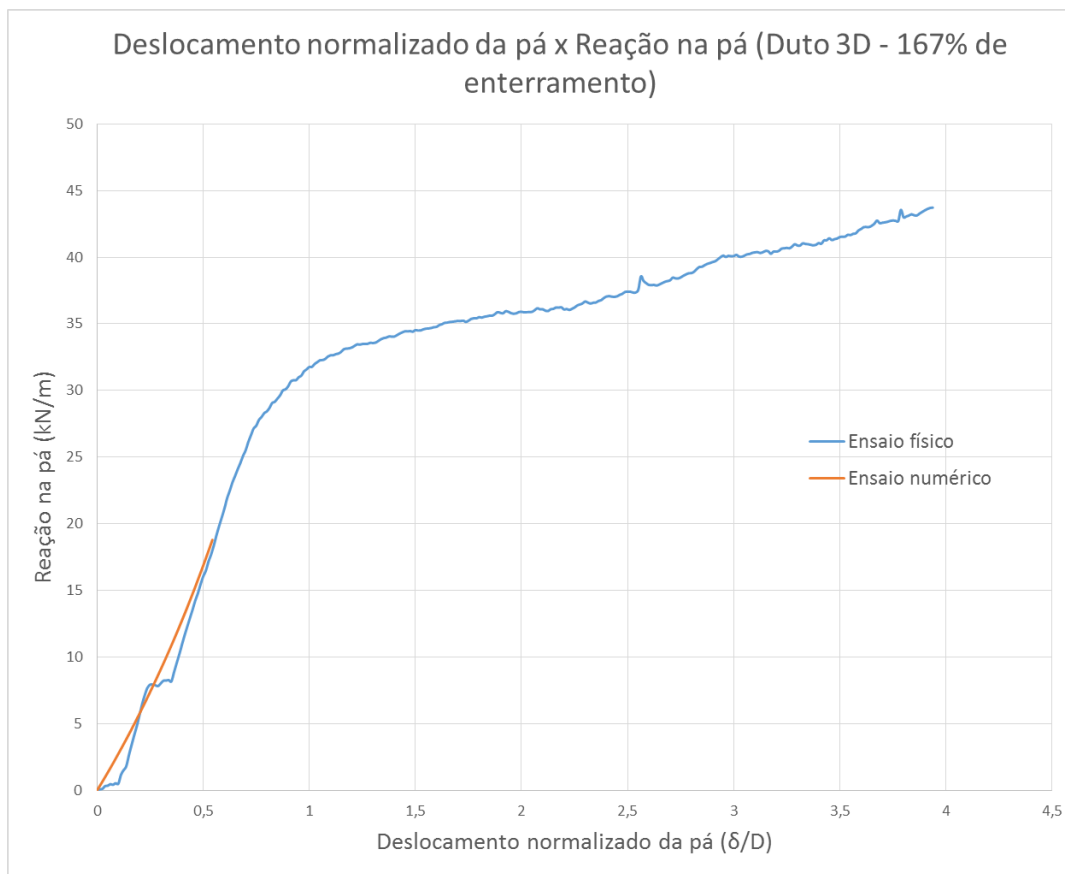
Figura 5-34 - Gráfico comparativo numérico-experimental para reação na pá com Duto 3D e 167% de enterramento (Cam-clay – modo implícito)
