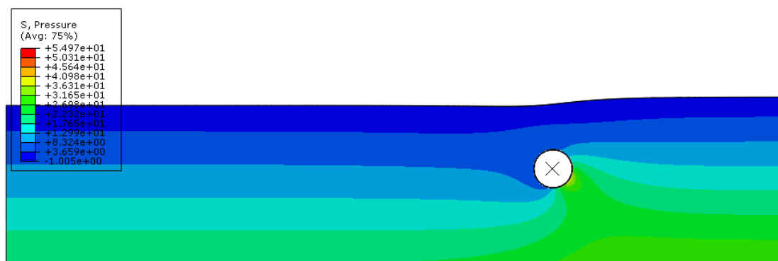
Figura 5-25 - Distribuição de tensões na massa de solo após deslocamento de 0,243m da pá contra Duto 2D com 211% de enterramento – Solo Cam-clay – Modo implícito
