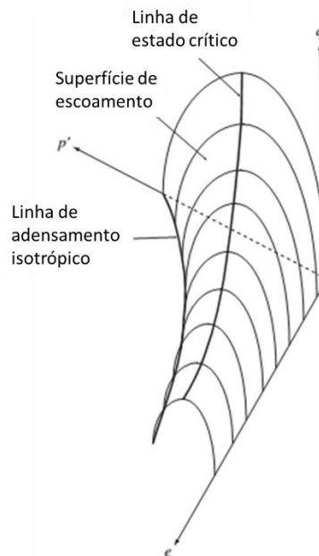
Figura 2-9 - Superfícies de escoamento no espaço p' , q , e (adaptado de HELWANY, 2007)
