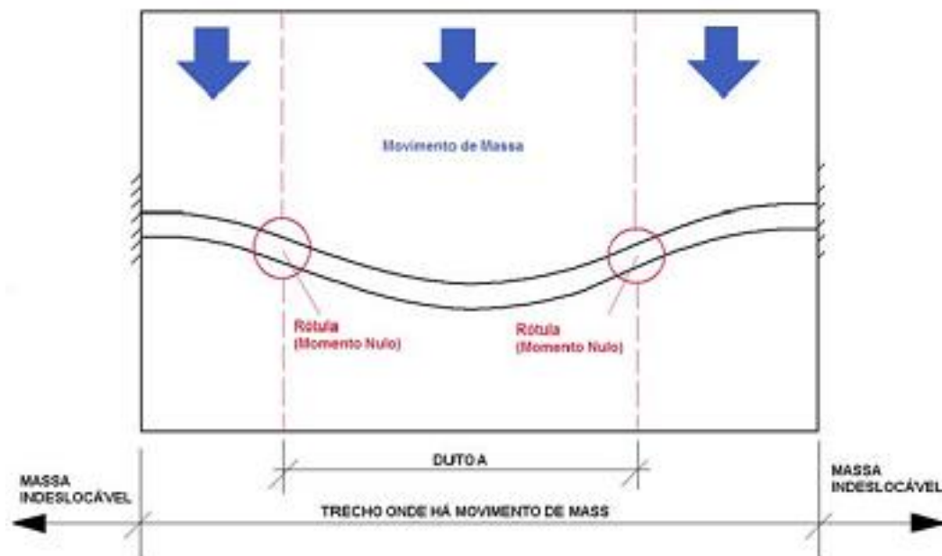
Figura 3-4 - Esquema da concepção do modelo Duto 3D (PEQUENO, 2013)
