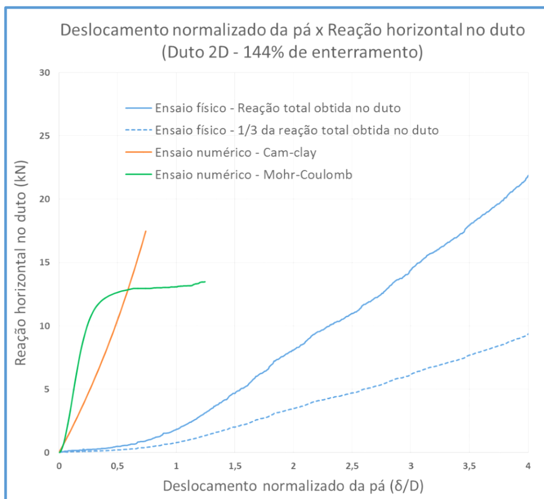
Figura 5-67 - Gráfico deslocamento versus reação horizontal no duto com Duto 2D e 144% de enterramento
