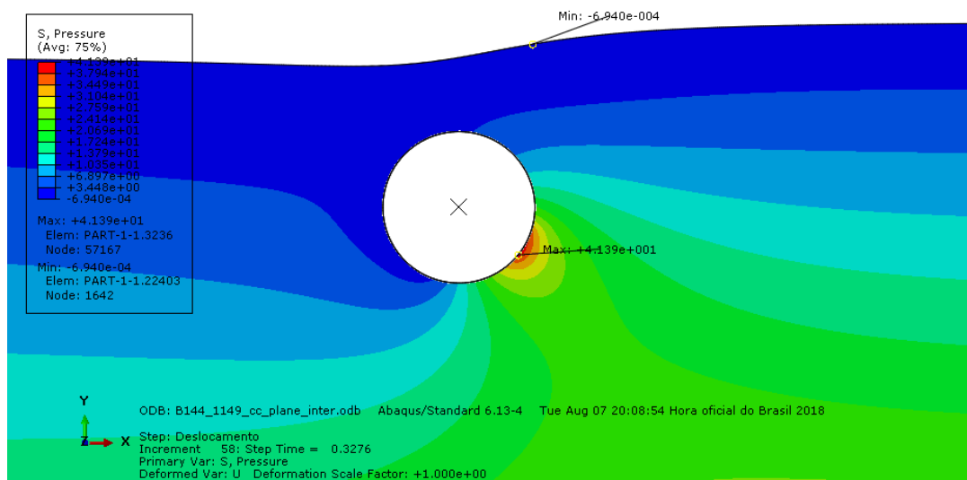
Figura 5-30 - Distribuição de tensões junto ao Duto 2D com 144% de enterramento após deslocamento de 0,299m da pá – Solo Cam-clay – Modo implícito
