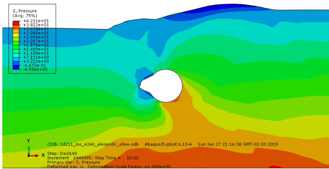
Figura 5-50 - Distribuição de tensões junto ao Duto 2D com 211% de enterramento após deslocamento de 0,711m da pá (Mohr-Culomb - modo explícito)
