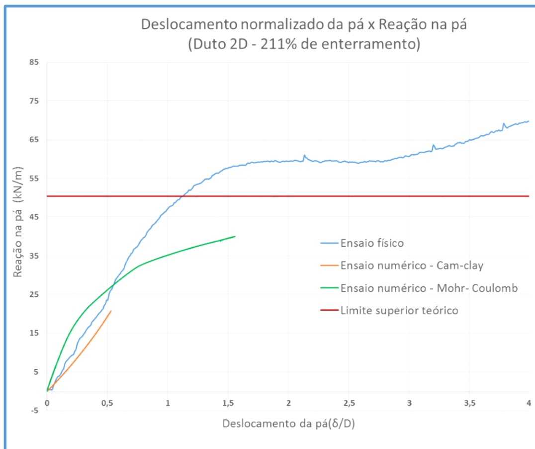
Figura 5-61 - Gráfico deslocamento versus reação na pá com Duto 2D e 211% de enterramento
