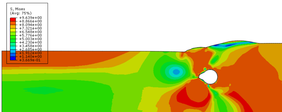
Figura 5-51 - Tensões de von Mises na massa de solo após deslocamento de 0,711m da pá contra Duto 2D com 211% de enterramento (Mohr-Coulomb - modo explícito)
