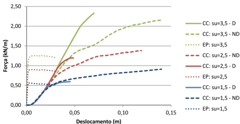
Figura 2-18 Gráfico comparativo dos modelos constitutivos Cam-clay (MCC) e “elasto-plástico” (MEP) para vários valores de resistência não drenada ( S_u ) (THOMAZ, 2015)
