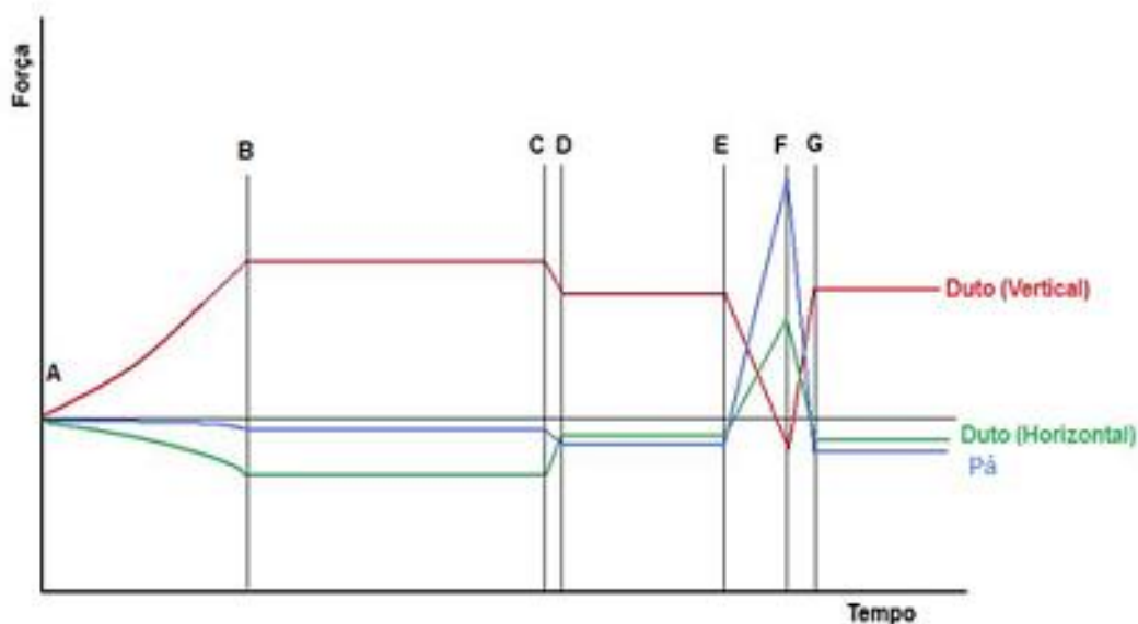
Figura 4-1 - Esquema para o entendimento das fases do ensaio da centrífuga (Pequeno, 2013)
