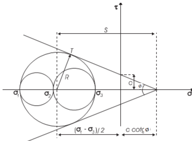
Figura 2-6 - Representação do estado limite para o critério de Mohr-Coulomb (CARDOSO, 2005)
